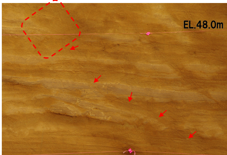
拡大写真② (②小断層延長部)
