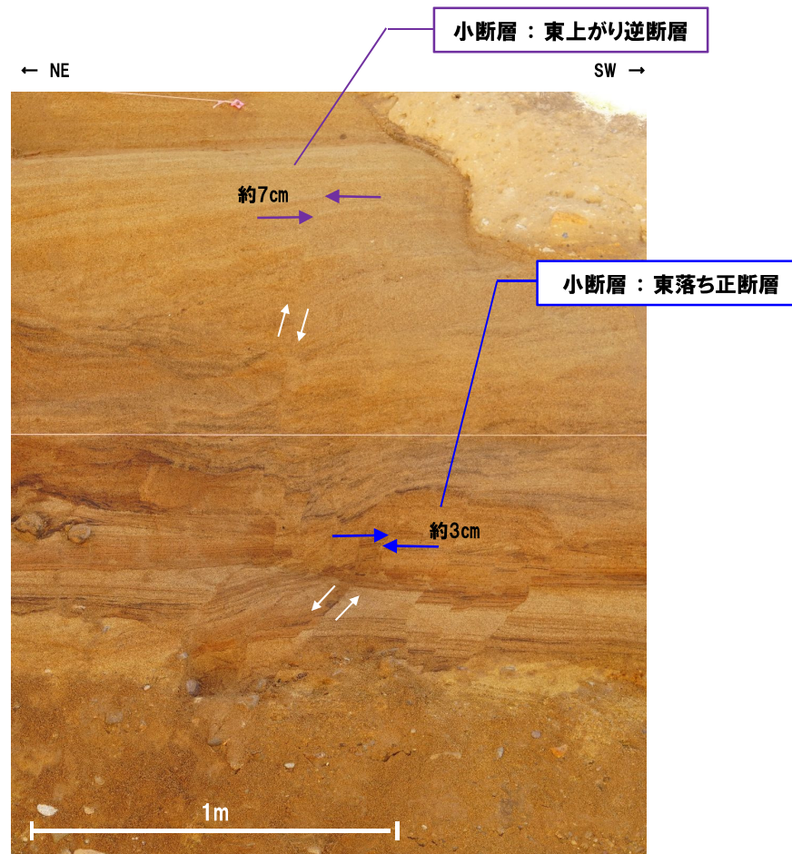
東上がり逆断層及び東落ち正断層センスの小断層 見かけ鉛直変位量計測箇所
