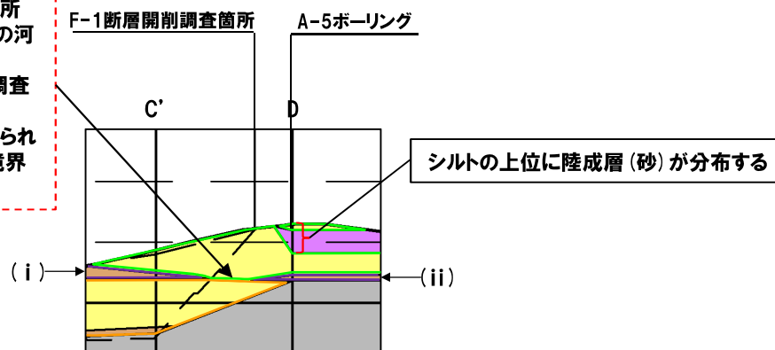
拡大図
