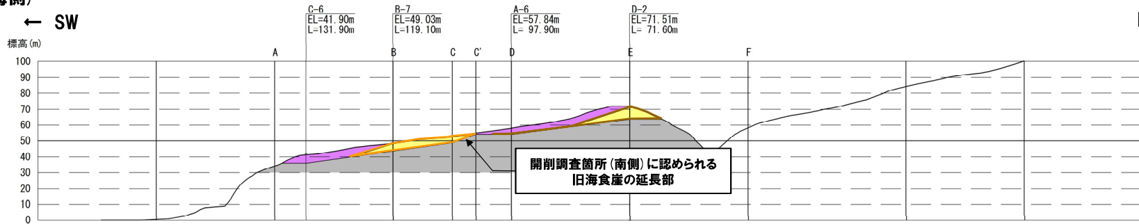
④断面図
