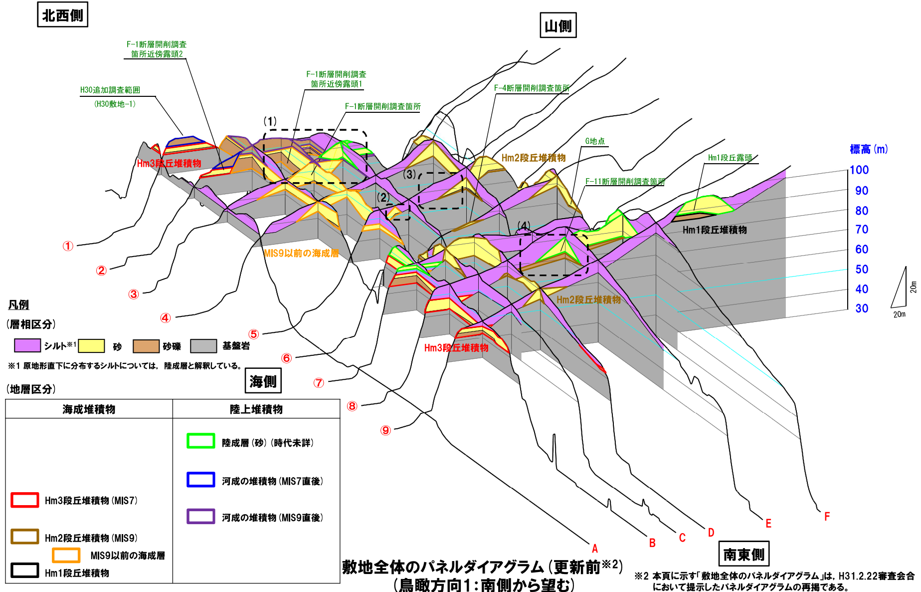
敷地全体のパネルダイアグラムにおける層相区分及び地層区分の主な変更箇所 (2/5)
