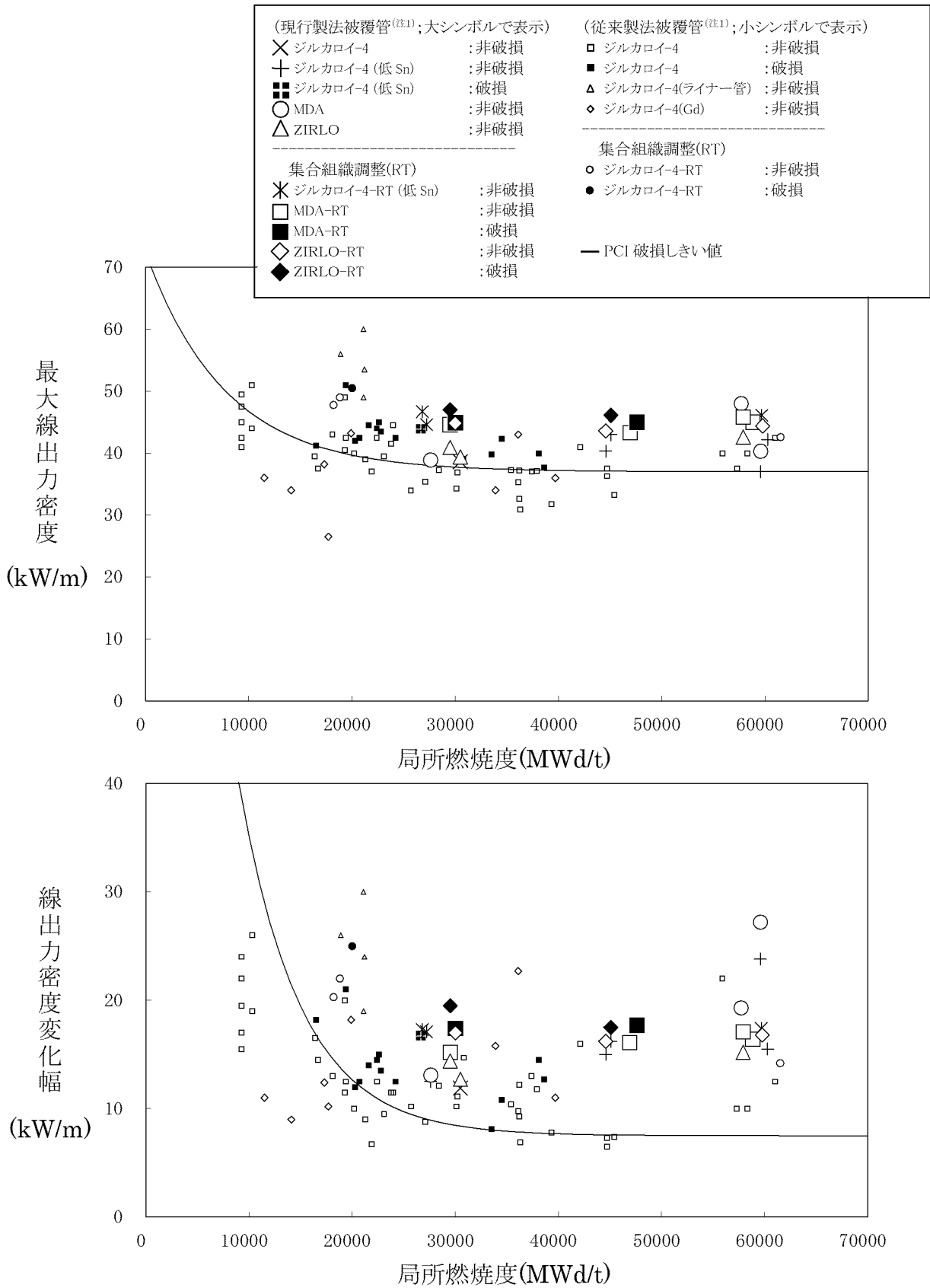
第5-11図 MDA及びZIRLO被覆管の耐PCI性 (10)(26)(53)(54)
