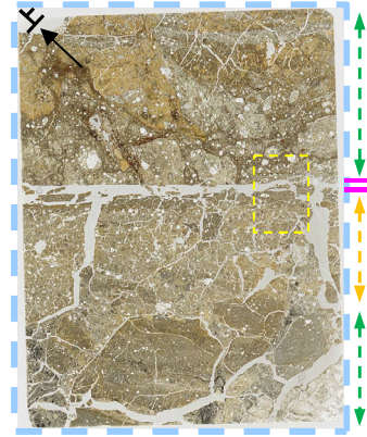
オープンニコル 10mm
