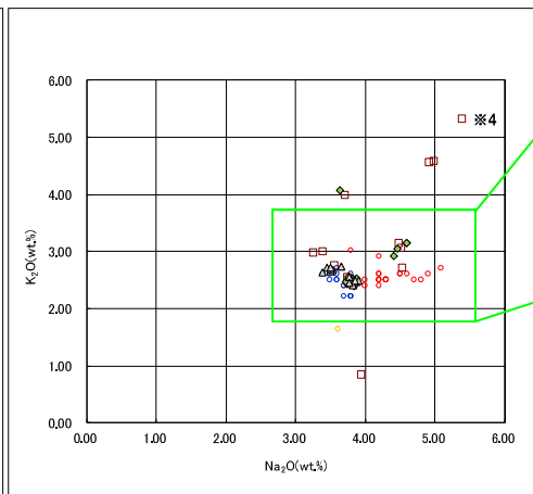
D-2-a 火山ガラスのK 2 O-TiO 2 図(左図), K 2 O-Na 2 O図(右図)
