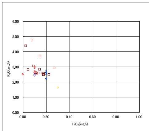
F-2-c 火山ガラスのK 2 O-TiO 2 図(左図), K 2 O-Na 2 O図(右図)
