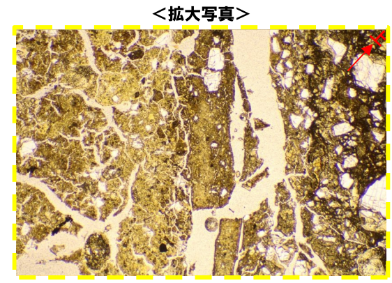
オープンニコル(右に90°回転) 1mm
