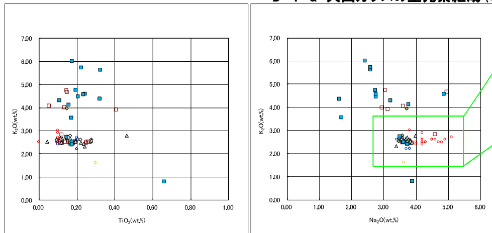
D-1-a 火山ガラスのK 2 O-TiO 2 図※4(左図), K 2 O-Na 2 O図(右図)
