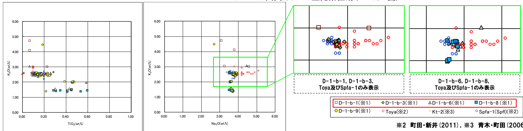
D-1-b 火山ガラスのK 2 O-TiO 2 図(左図), K 2 O-Na 2 O図(右図)
