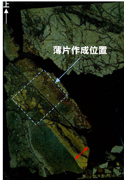
傾斜方向研磨片 ※研磨片, 薄片ともに左右反転
