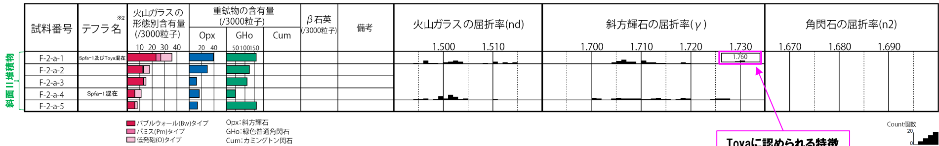
F-2-a 火山ガラス及び重鉱物の屈折率測定結果
