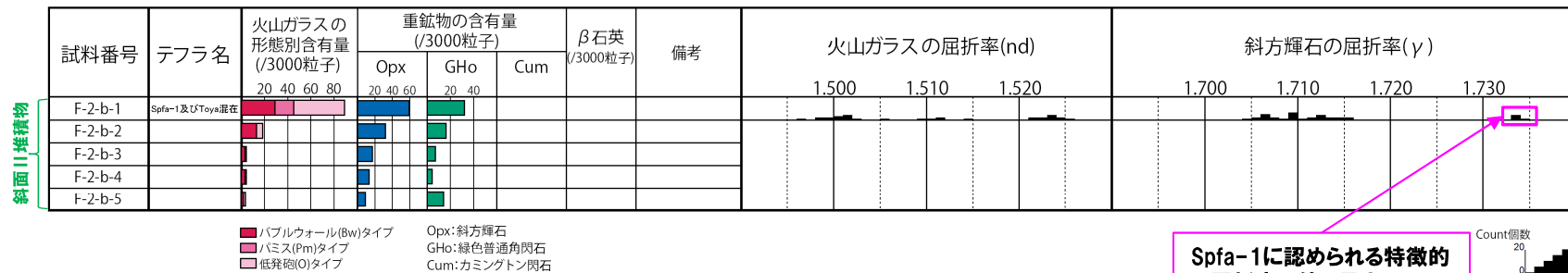
F-2-b 火山ガラス及び重鉱物の屈折率測定結果
