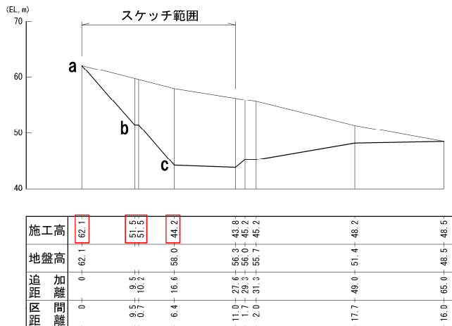
東側壁面中央部の縦断面図 (A-A') (F-1断層開削調査箇所)
