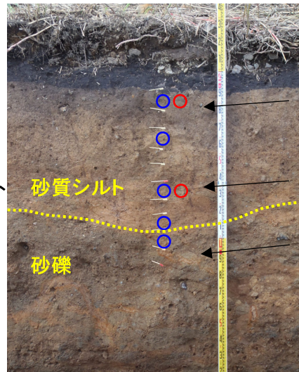
測線D-1-b 拡大写真
