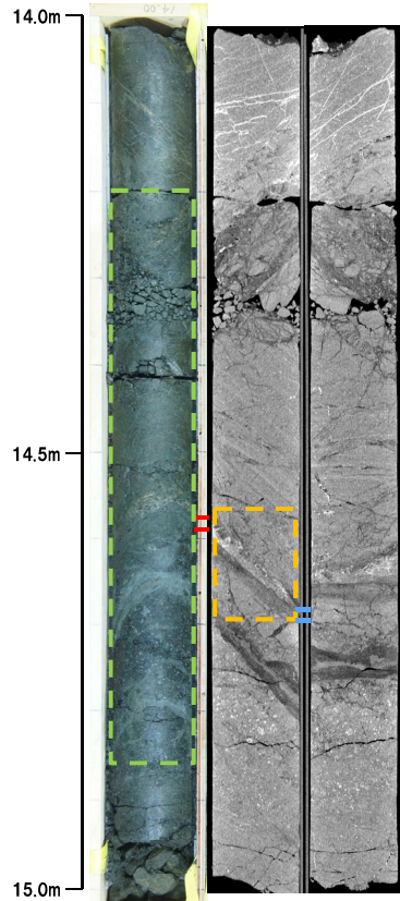
傾斜方向研磨片 ※研磨片, 薄片ともに左右反転
