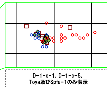
D-1-c 火山ガラスの主元素組成(ハーカー図)
