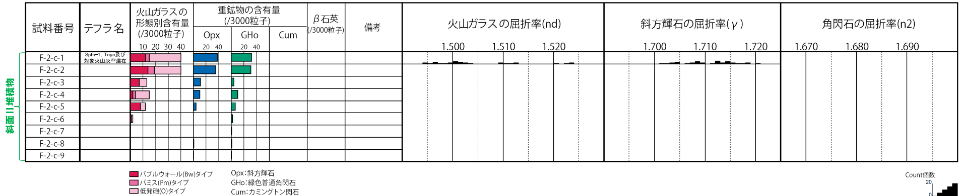
F-2-c 火山ガラス及び重鉱物の屈折率測定結果
