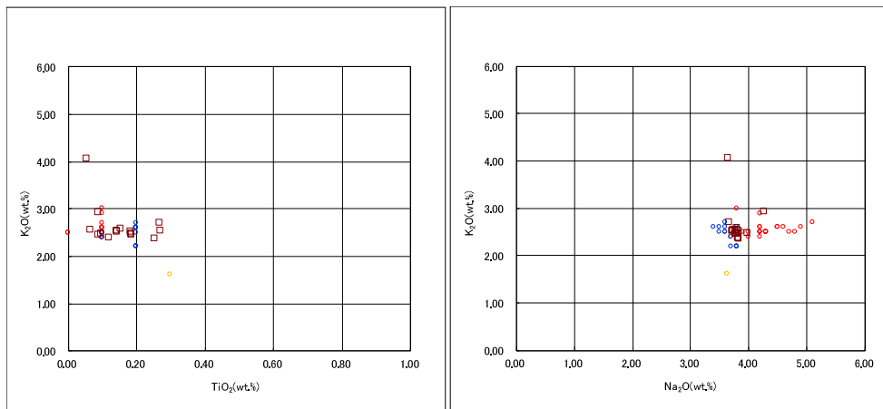
D-2-b 火山ガラスのK 2 O-TiO 2 図(左図), K 2 O-Na 2 O図(右図)
