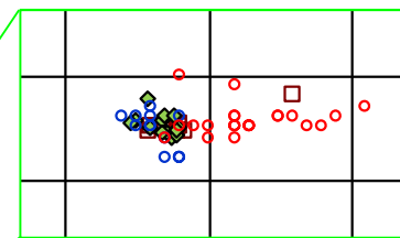
D-1-a-1, D-1-a-4, Toya及びSpfa-1のみ表示
