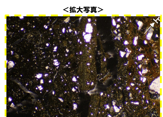
クロスニコル(右に90°回転) 1mm
