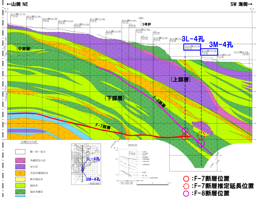
地質断面図 (4断面)
