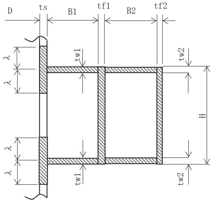
C-C 断面
