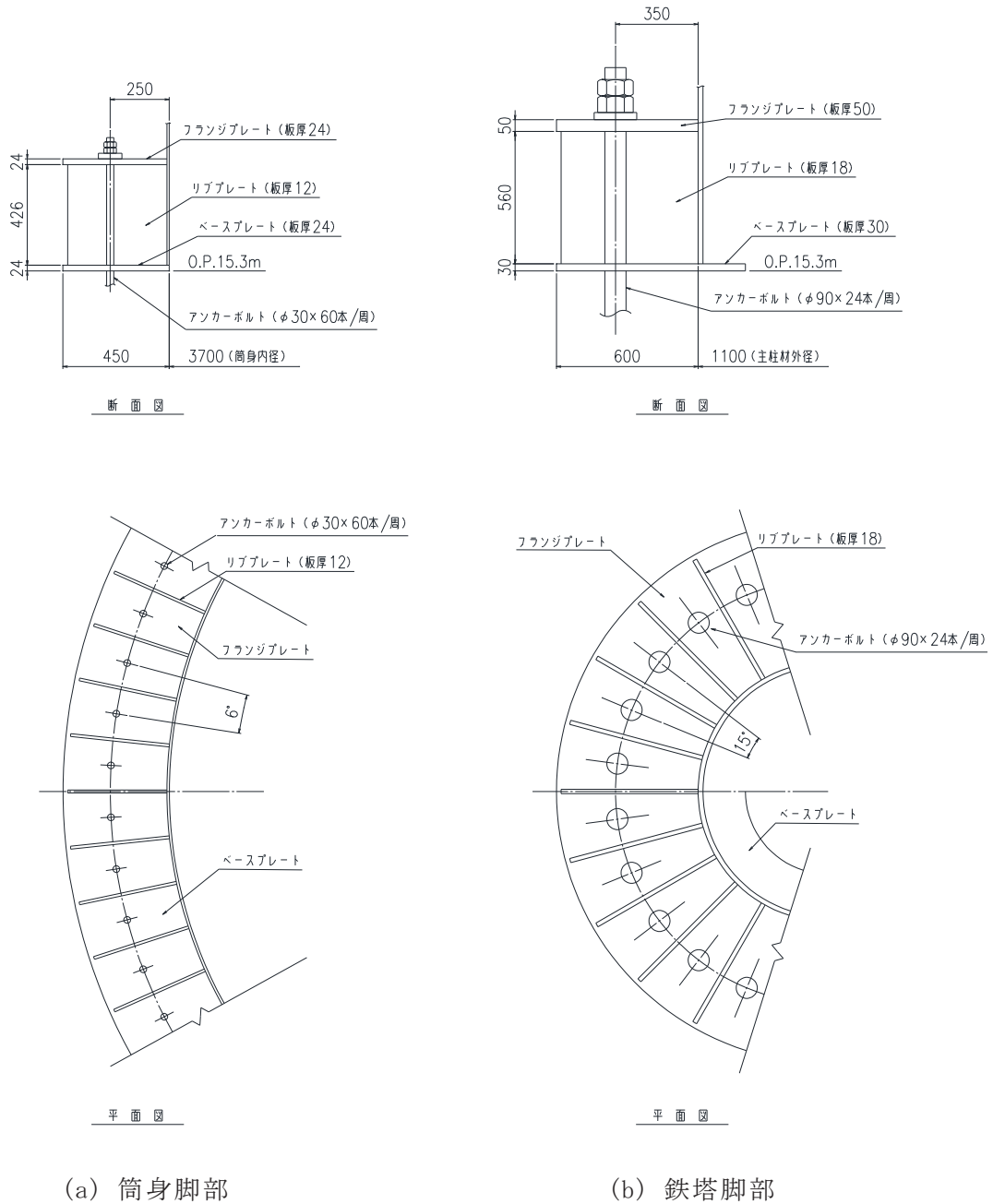
図 5-1 脚部の概要図（単位：mm）
