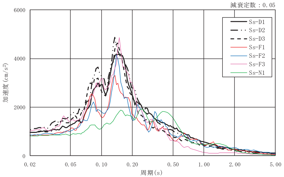
図 3-6(1) 入力地震動の加速度応答スペクトル (基準地震動 S_s , NS 断面 並進成分)
