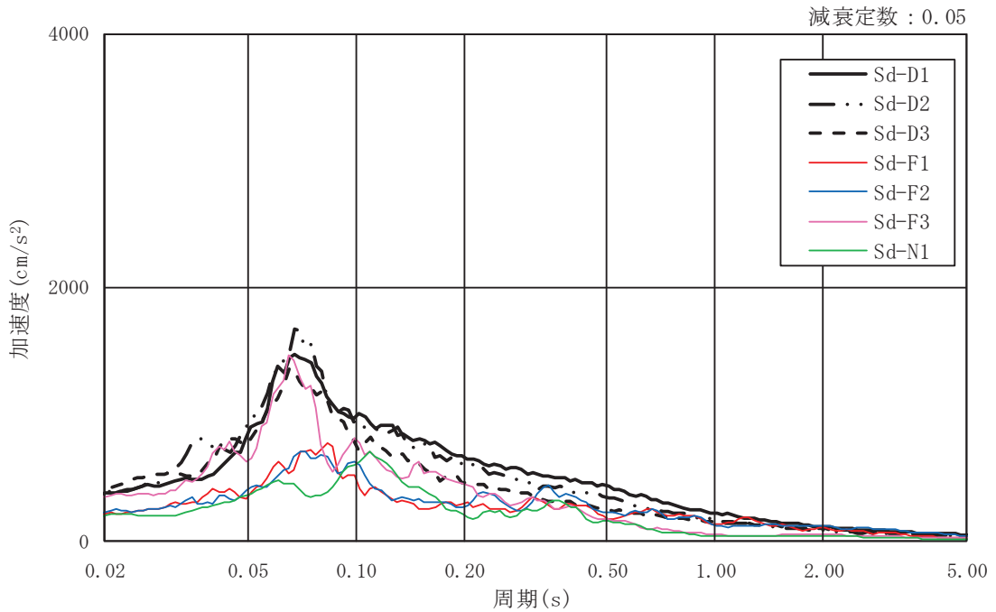
図 3-7(2) 入力地震動の加速度応答スペクトル (弾性設計用地震動 S d , NS 断面 鉛直成分)
