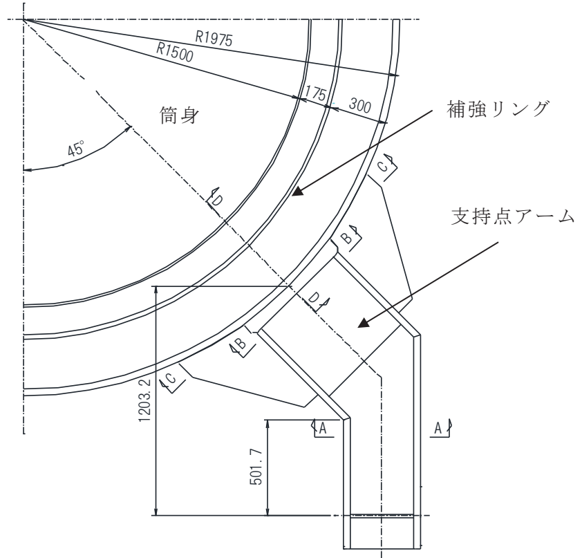
図 1-5 第 4 支持点部拡大図 (単位 : mm)
