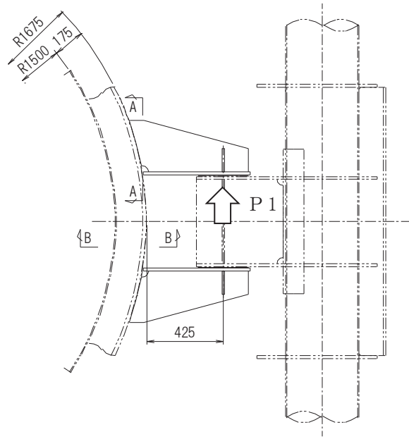
a 部詳細
