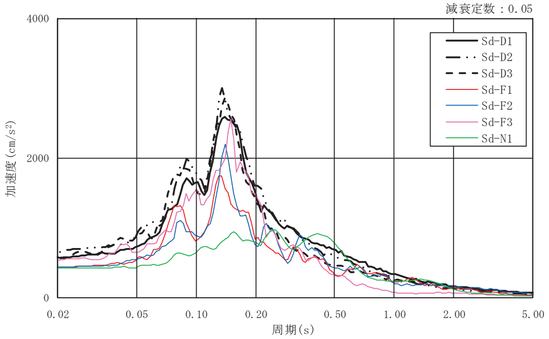
図 3-7(1) 入力地震動の加速度応答スペクトル (弾性設計用地震動 S d , NS 断面 並進成分)
