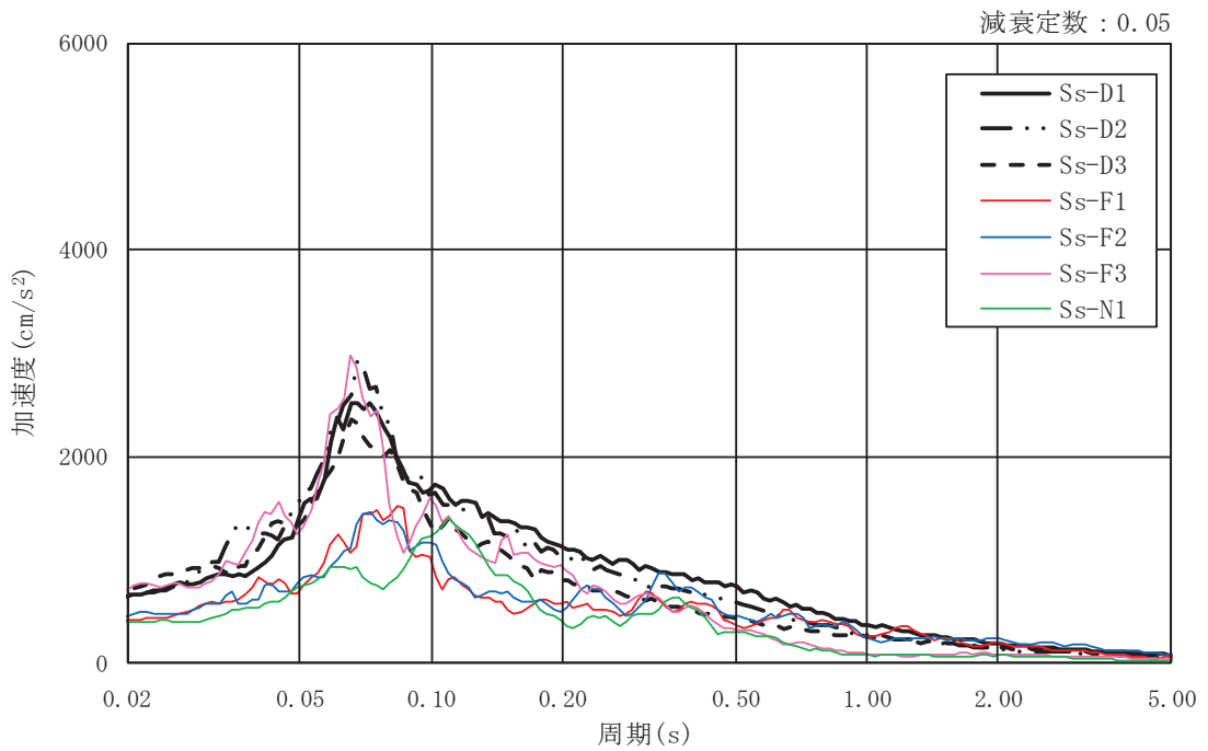
図 3-6(2) 入力地震動の加速度応答スペクトル (基準地震動 S_s , NS 断面 鉛直成分)
