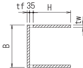
A-A 断面
