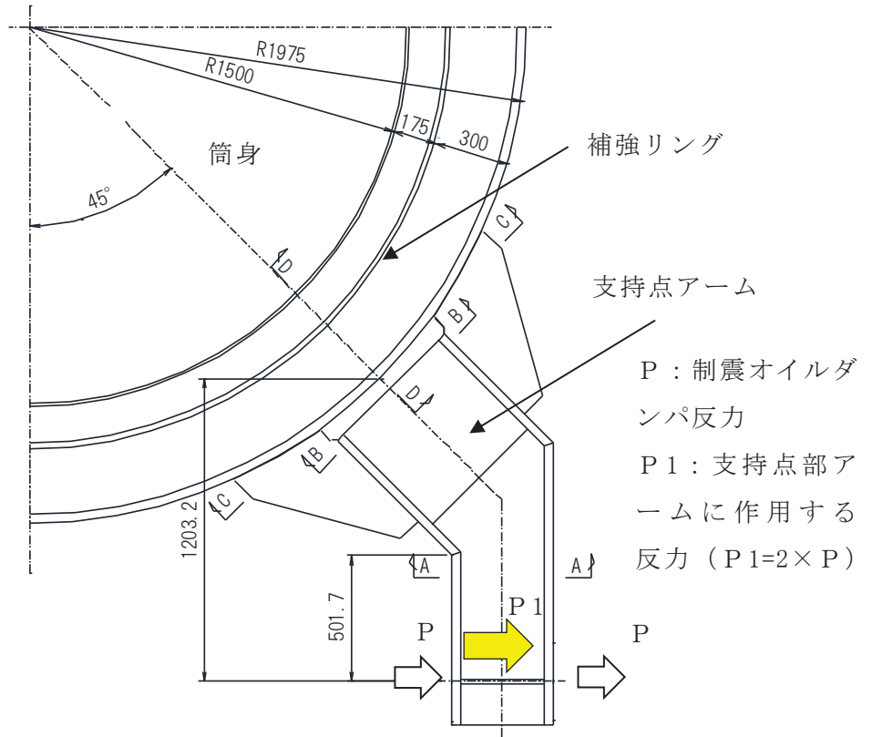
図 4-1(2) 制震オイルダンパ支持点平面図及び支持点荷重
