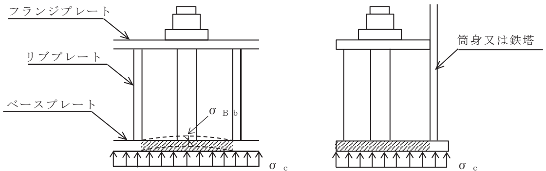
(a) 正面図
