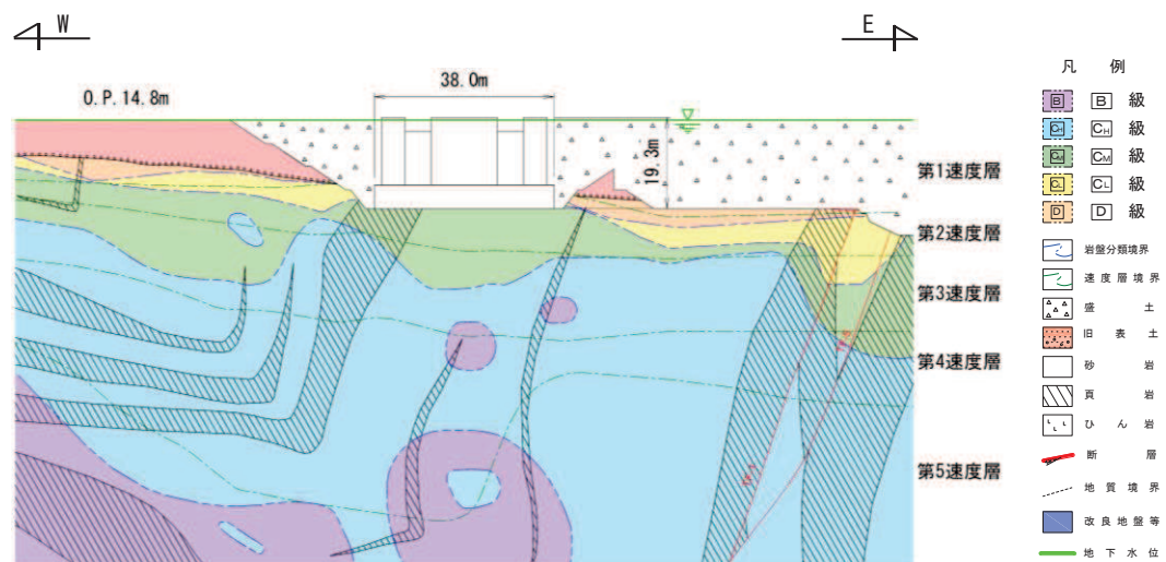
图 3-7 排气筒基础 地震时荷重算出用地质断面图 (EW 断面)
