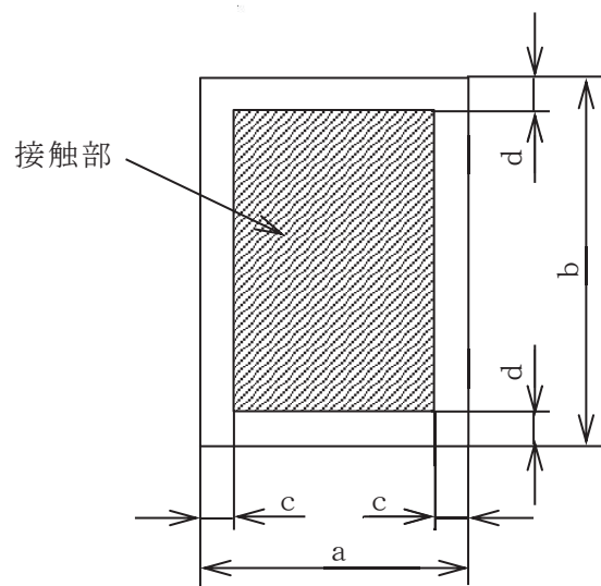
接触部詳細
