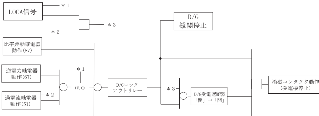
図 6.8 インターロック図 (概要) (1/2)
