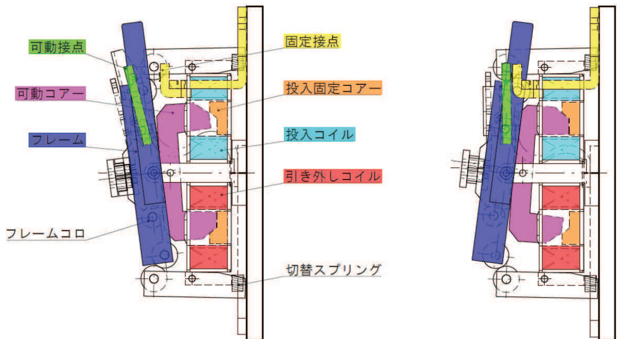
図 6.10 消磁コンタクタ構成図
