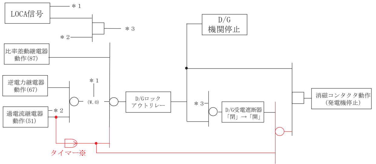
図 6.8 インターロック図 (概要) (2/2) (HEAF 対策後)
