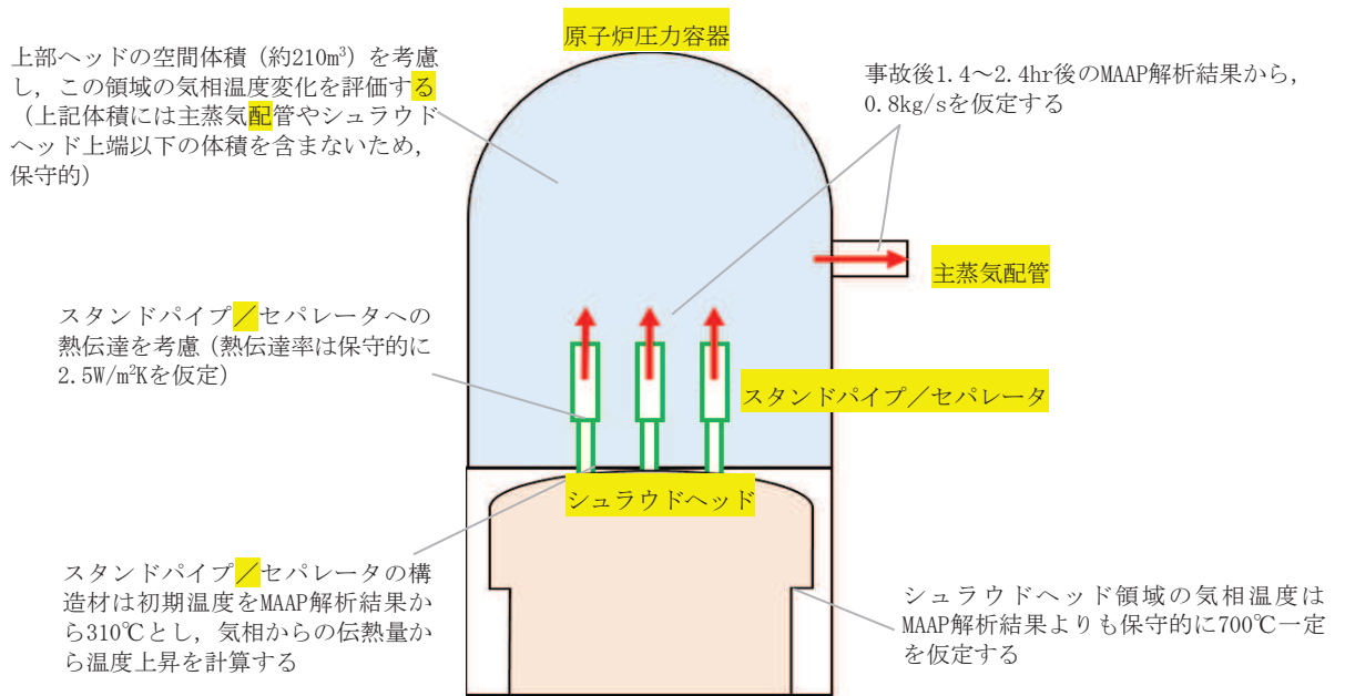
図2 簡易評価の計算体系
