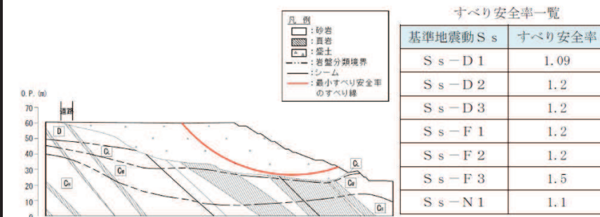
図2.3.2-8 斜面Bのすべり安定性評価結果
