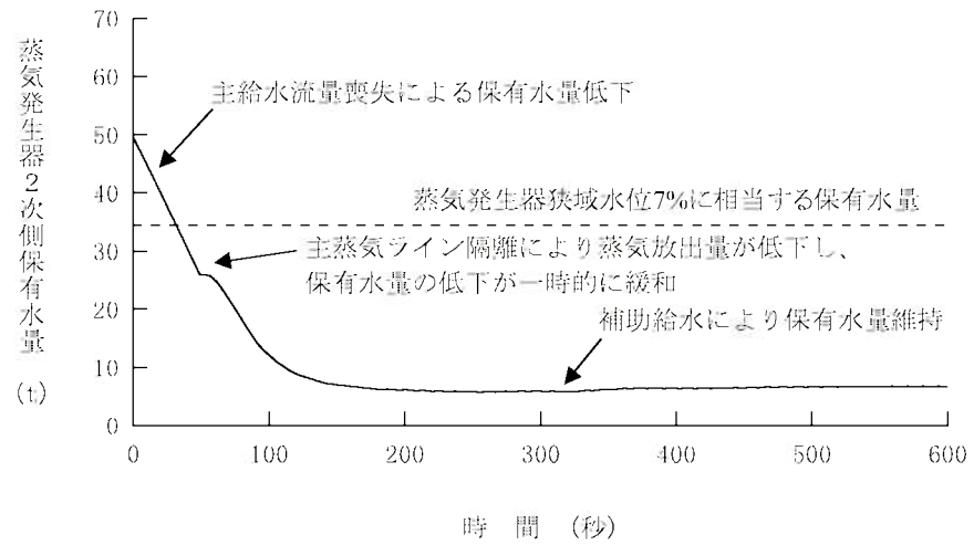
第1.15-239図 蒸気発生器2次側保有水量の推移 (主給水流量喪失時に原子炉トリップ機能が喪失する事故)
