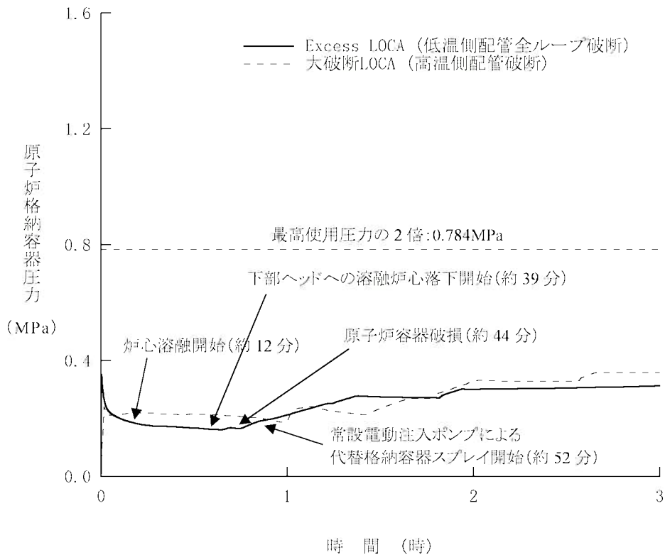
第1.15-399図 原子炉格納容器圧力の推移 (低温側配管全ループ破断時の影響確認)
