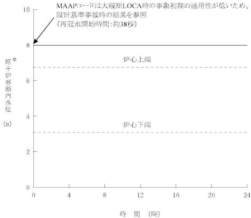
第1.15-217図 原子炉容器内水位の推移
