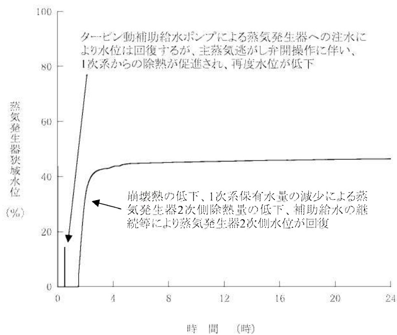
第1.15-185図 蒸気発生器狭域水位の推移 (RCPシールLOCAが発生する場合)
