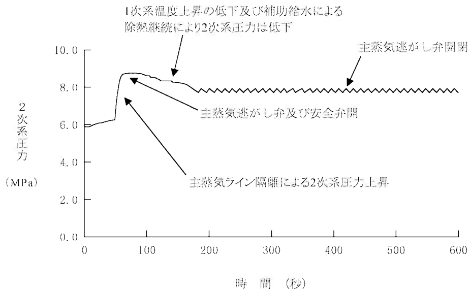
第1.15-238図 2次系圧力の推移 (主給水流量喪失時に原子炉トリップ機能が喪失する事故)
