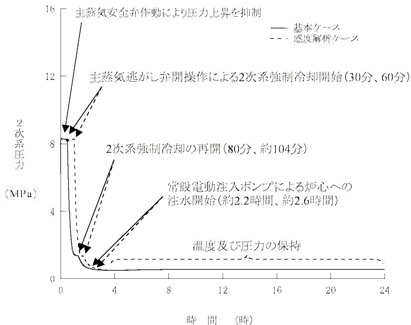
第1.15-208図 2次系圧力の推移比較 (RCPシールLOCAが発生する場合) (主蒸気逃がし弁操作時間余裕確認)
