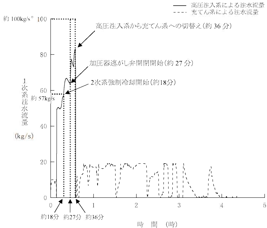
第1.15-348図 1次系注水流量(高圧及び充電)の推移 (インターフェイスシステムLOCA)(操作時間余裕確認)
