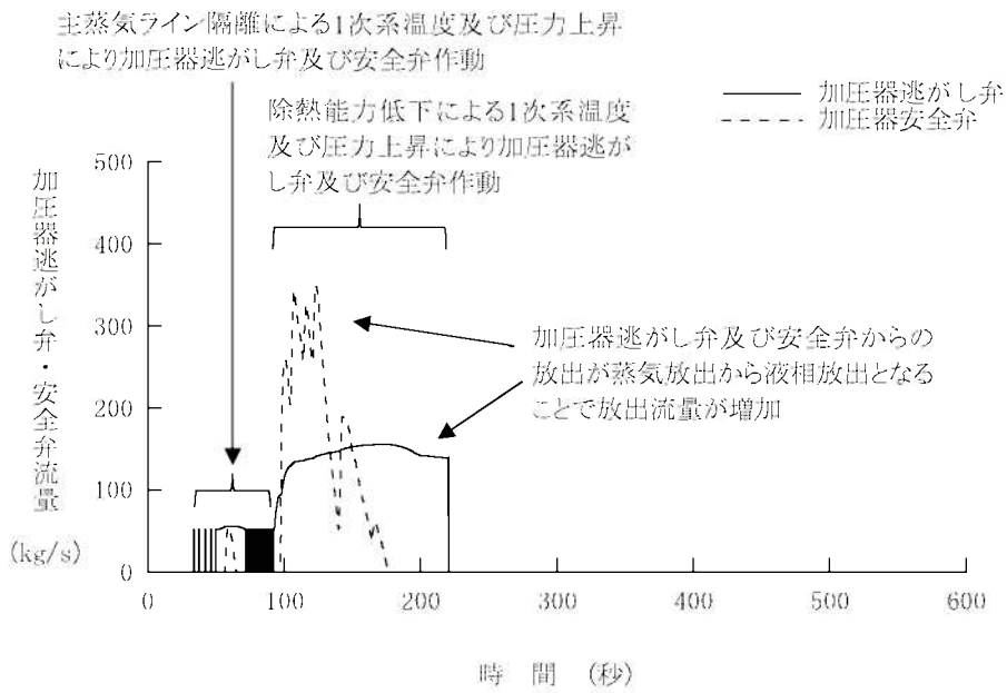
第1.15-232図 加圧器逃がし弁・安全弁流量の推移 (主給水流量喪失時に原子炉トリップ機能が喪失する事故)
