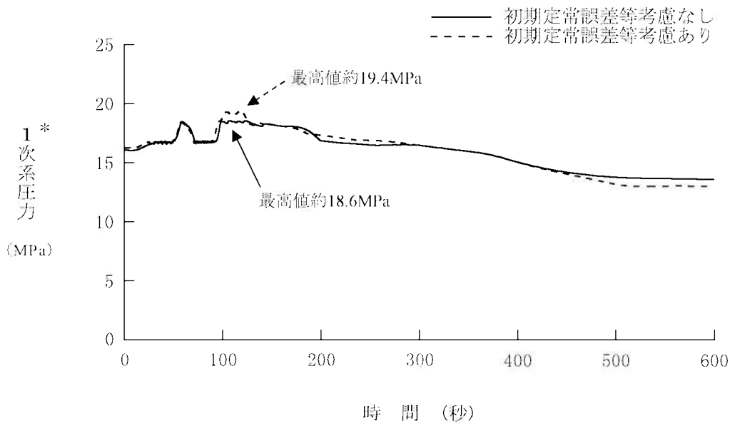
第1.15-255図 1次系圧力の推移比較 (主給水流量喪失時に原子炉トリップ機能が喪失する事故) (初期定常誤差及びドブブラ特性の感度確認)
