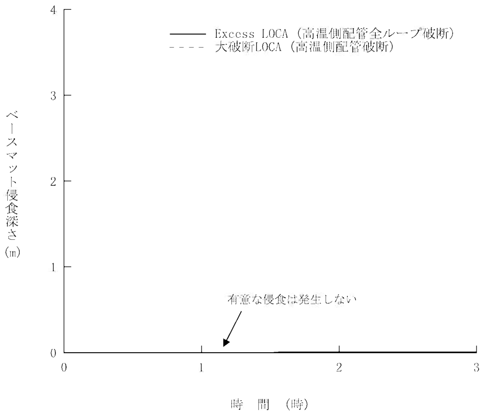
第1.15-444図 ベースマツト侵食深さの推移 (高温側配管全ループ破断時の影響確認)
