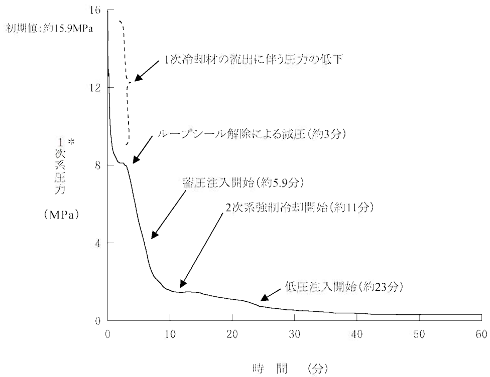
第1.15-257図 1次系圧力の推移(6inch破断)
