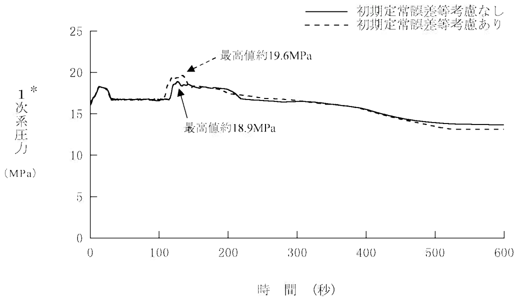
第1.15-256図 1次系圧力の推移比較 (負荷の喪失時に原子炉トリップ機能が喪失する事故) (初期定常誤差及びドブブラ特性の感度確認)
