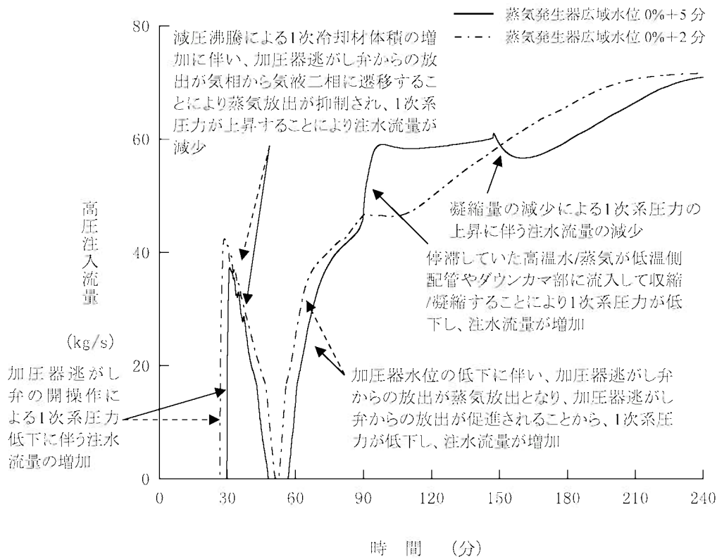
第1.15-161図 高圧注水流量の推移(開始が早くなる場合)
