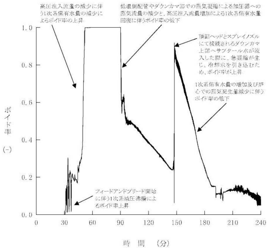
第1.15-145図 高圧側配管・加圧器サージライン接続部ボイド率の推移
