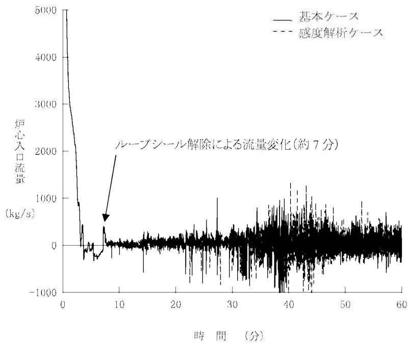
第1.15-301図 炉心入口流量の推移(4inch破断) (2次系強制冷却操作時間余裕確認)
