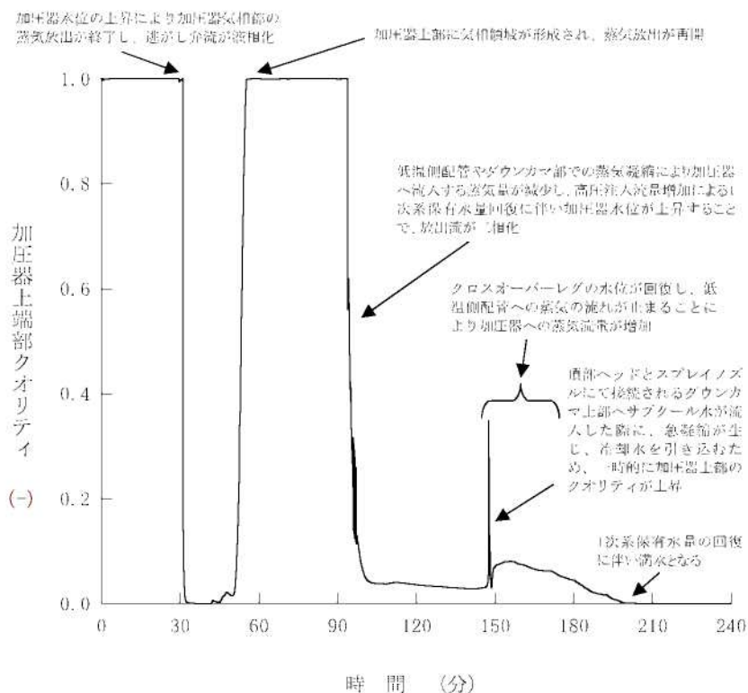
第1.15-143図 加圧器上端部クオリティの推移
