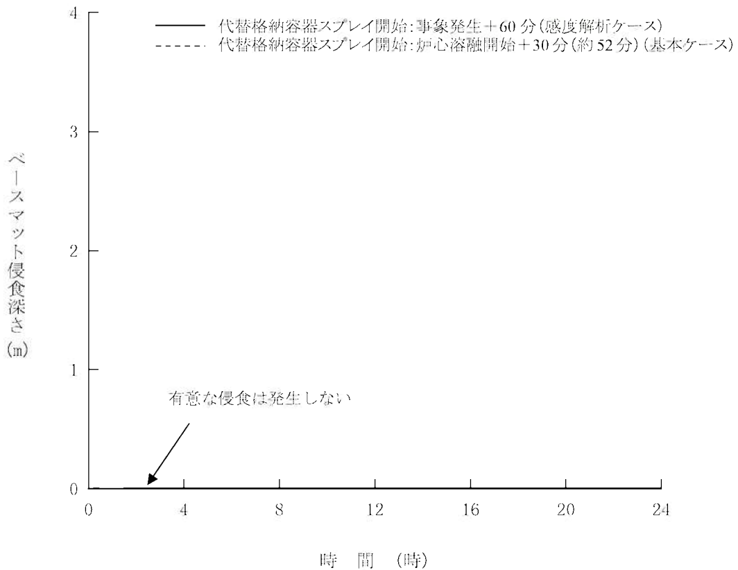
第1.15-450図 ベースマツト侵食深さの推移 (代替格納容器スプレイ操作時間余裕確認)
