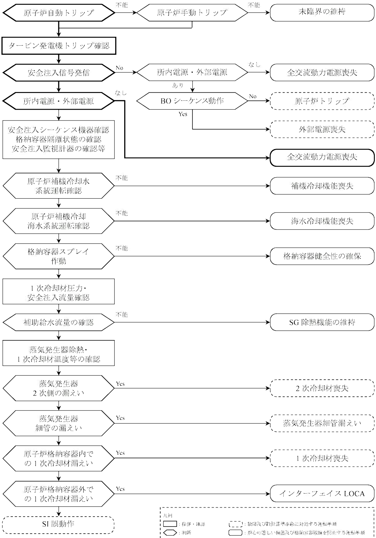
第1.15-382図 「雰囲気圧力・温度による静的負荷(格納容器過圧破損)」の事象進展 (事象判別プロセス) (大破断LOCA時に低压注入機能、高压注入機能及び格納容器スプレイ注入機能が喪失する事故)
