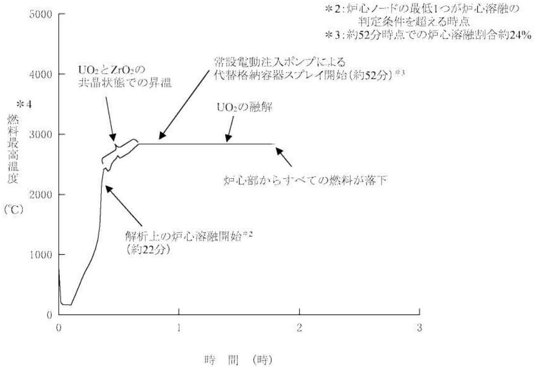
第1.15-386図 燃料最高温度の推移
