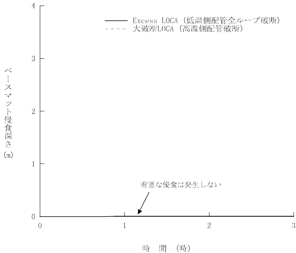
第1.15-446図 ベースマツト侵食深さの推移 (低温側配管全ループ破断時の影響確認)
