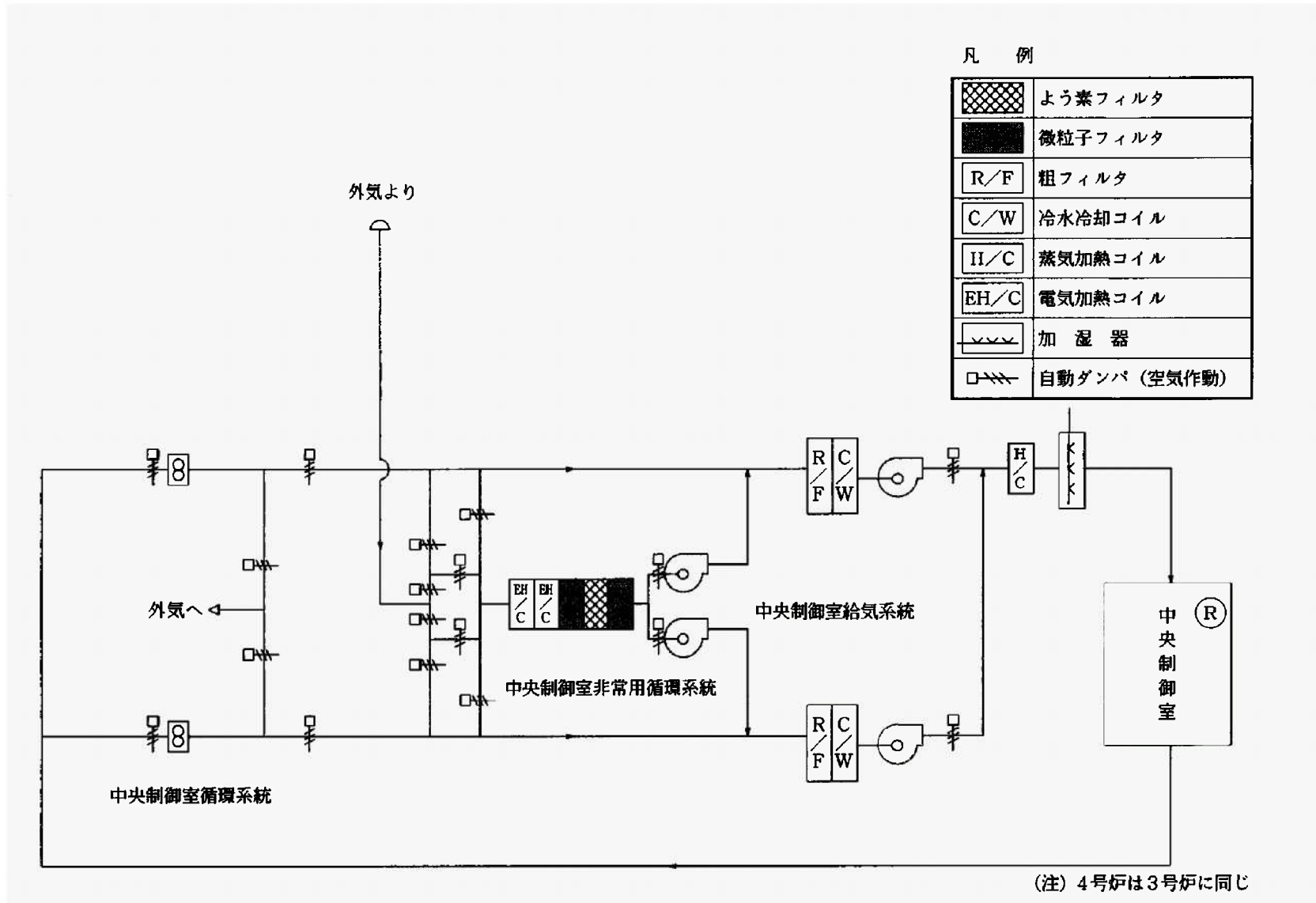
第1.12-24図 補助建屋換気空調設備系統説明図(中央制御室)
