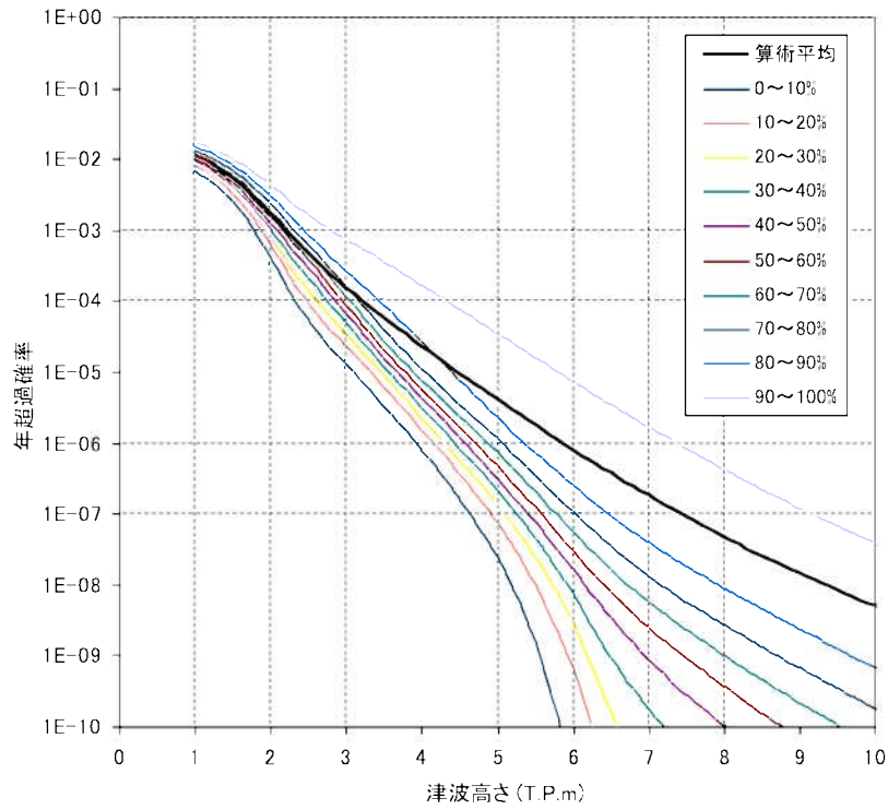
第 3.1.3.4-22 図 取水口位置におけるフラクタイルハザード曲線 (1/2)
