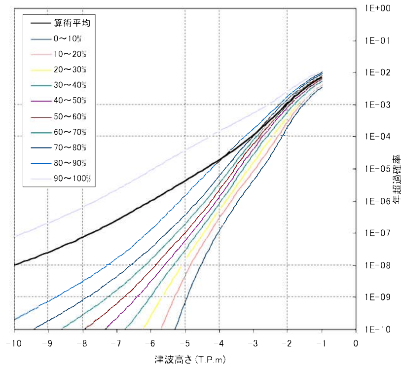
第 3.1.3.4-22 図 取水口位置におけるフラクタイルハザード曲線 (2/2)
