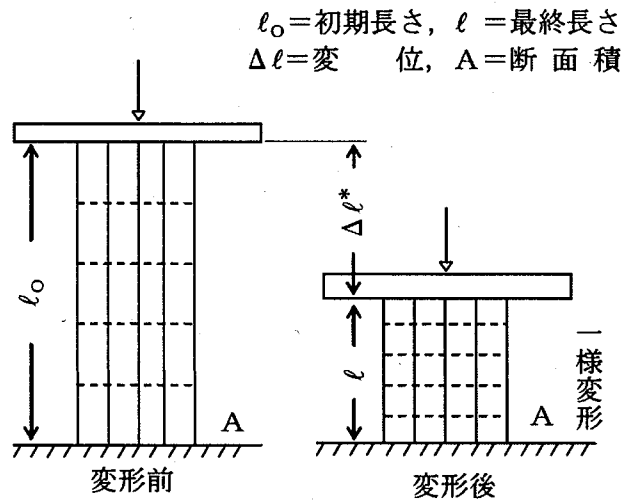
(a) - 第 A. 102 図 一次元変形法による解析モデル
