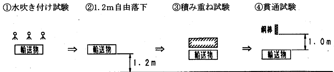
(ロ)－第A.98図 一般の試験条件
