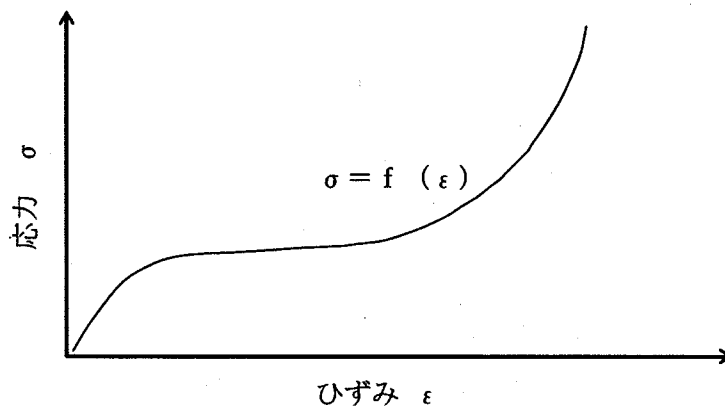
(a) - 第 A. 103 図 材料の圧縮応力-圧縮ひずみ関係
