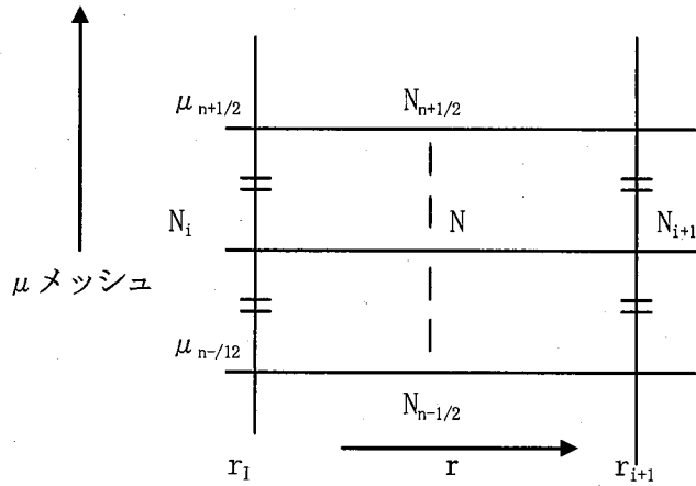
(D.5) 図 D.5 図 メッシュ分割図
