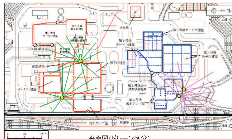
平面図(ドレーン区分)
