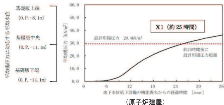
(原子炉建屋)
