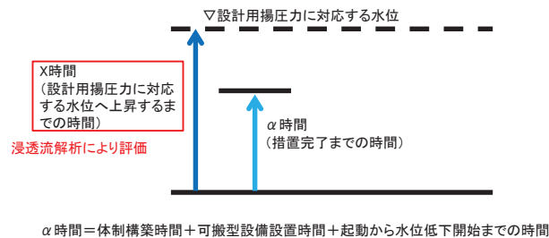
図3-5 到達時間と措置の概念
