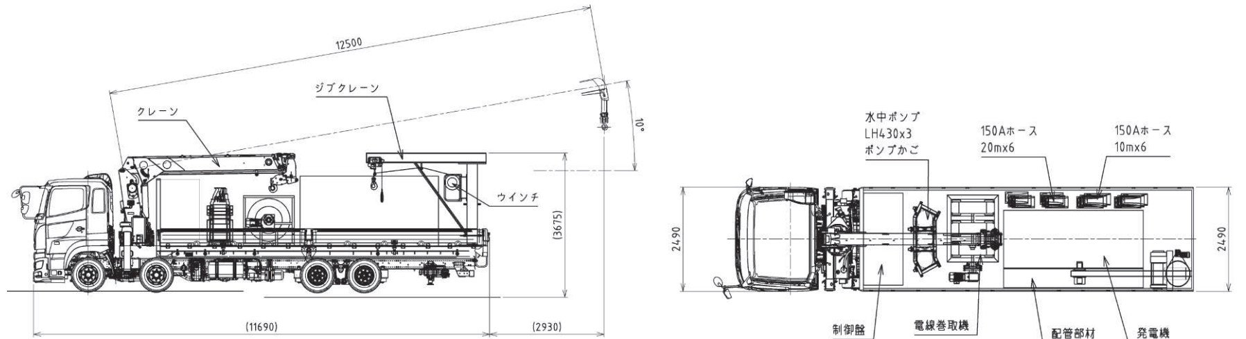
参考図4-1 可搬ポンプユニット
