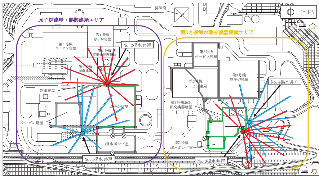
図4-2 原子炉建屋・制御建屋エリアの揚水井戸配置
