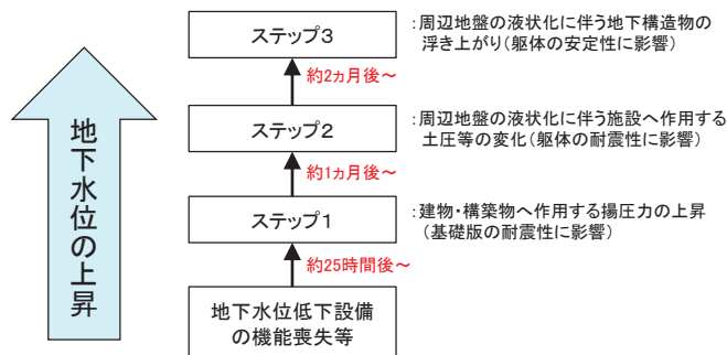
図3-6 地下水水位上昇時に施設に段階的に生じる影響(時間軸)
