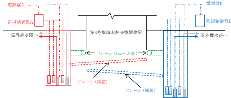
図4-3 第3号機海水熱交換器建屋エリアの揚水井戸配置
