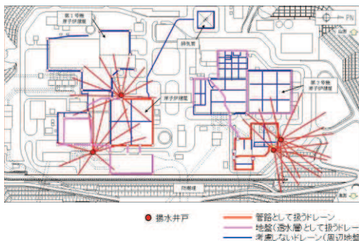
(a) 通常の運転状態に対応するドレーン範囲(④水位上昇評価モデル)
