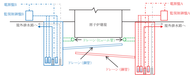
図4-2 原子炉建屋・制御建屋エリアの揚水井戸配置
