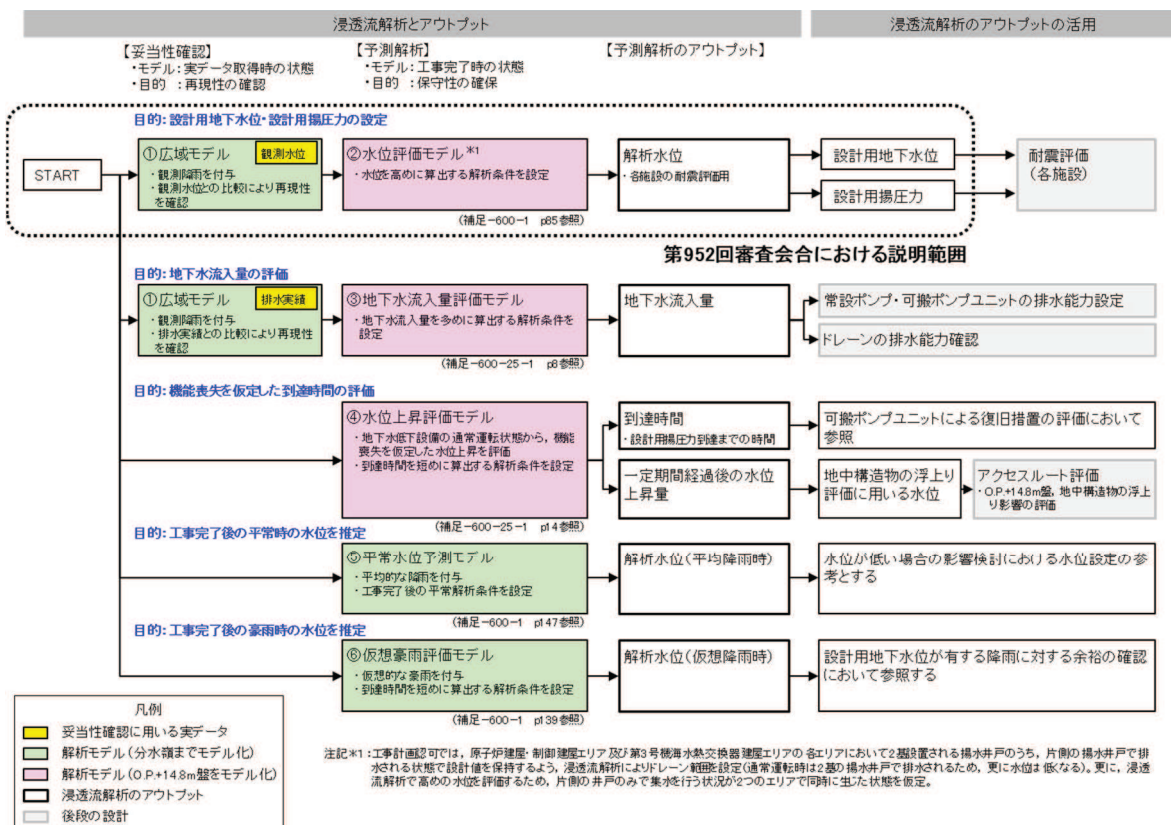
図1-1 浸透流アウトプットと反映事項について
