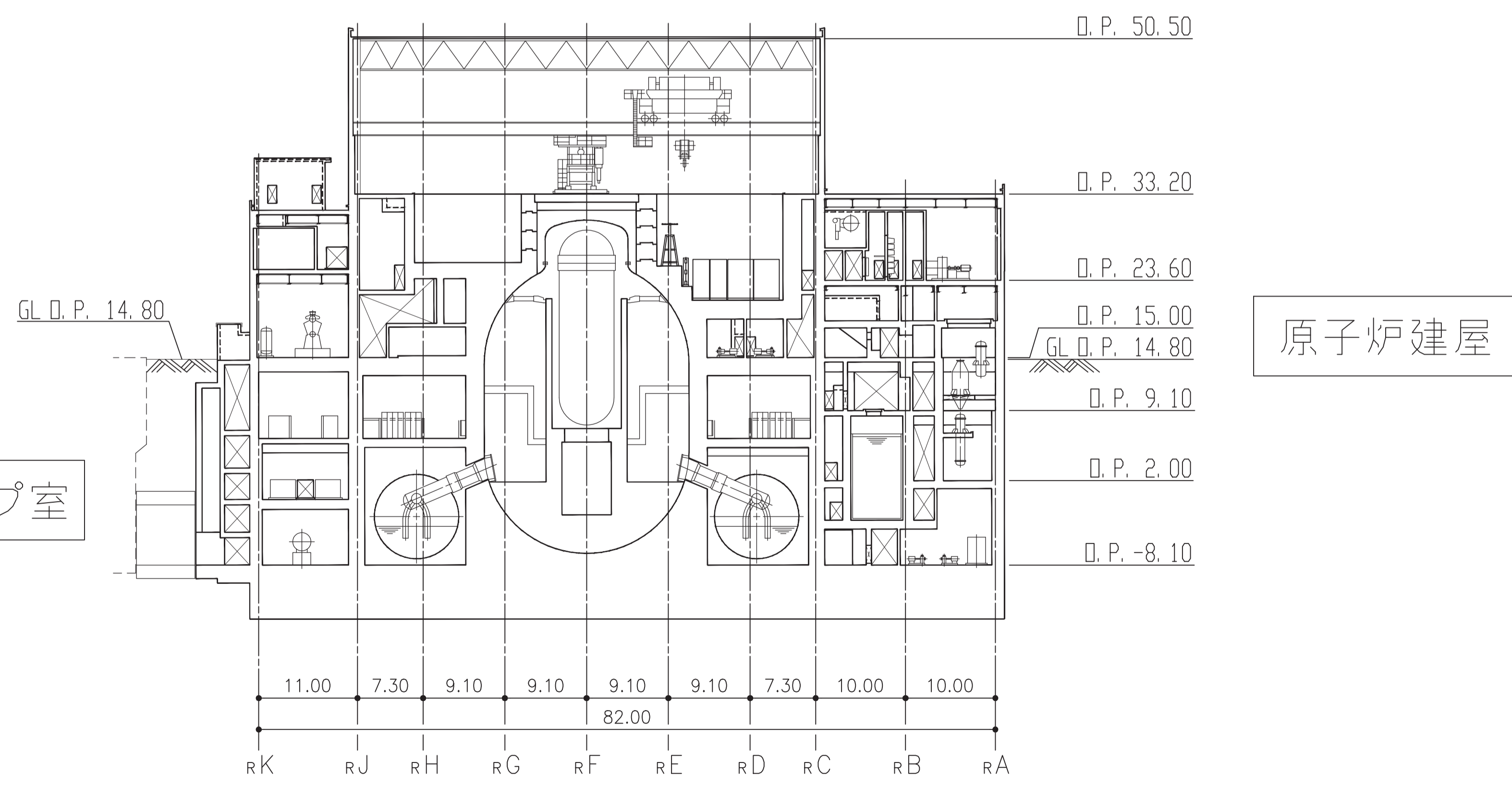
C-C断面図
