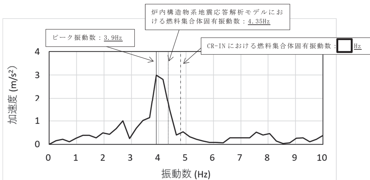
別添 2 図 3 炉心支持板の加速度時刻歴(S s - D 2)より作成したフーリエスペクトル
