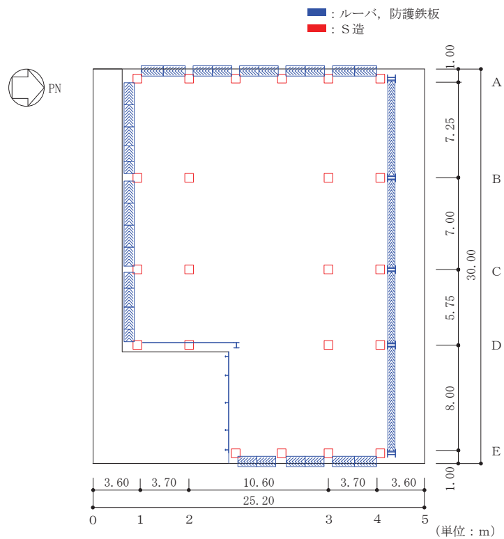
図 2-2(2) 緊急用電気品建屋の概略平面図 (O. P. 62.9 m)
