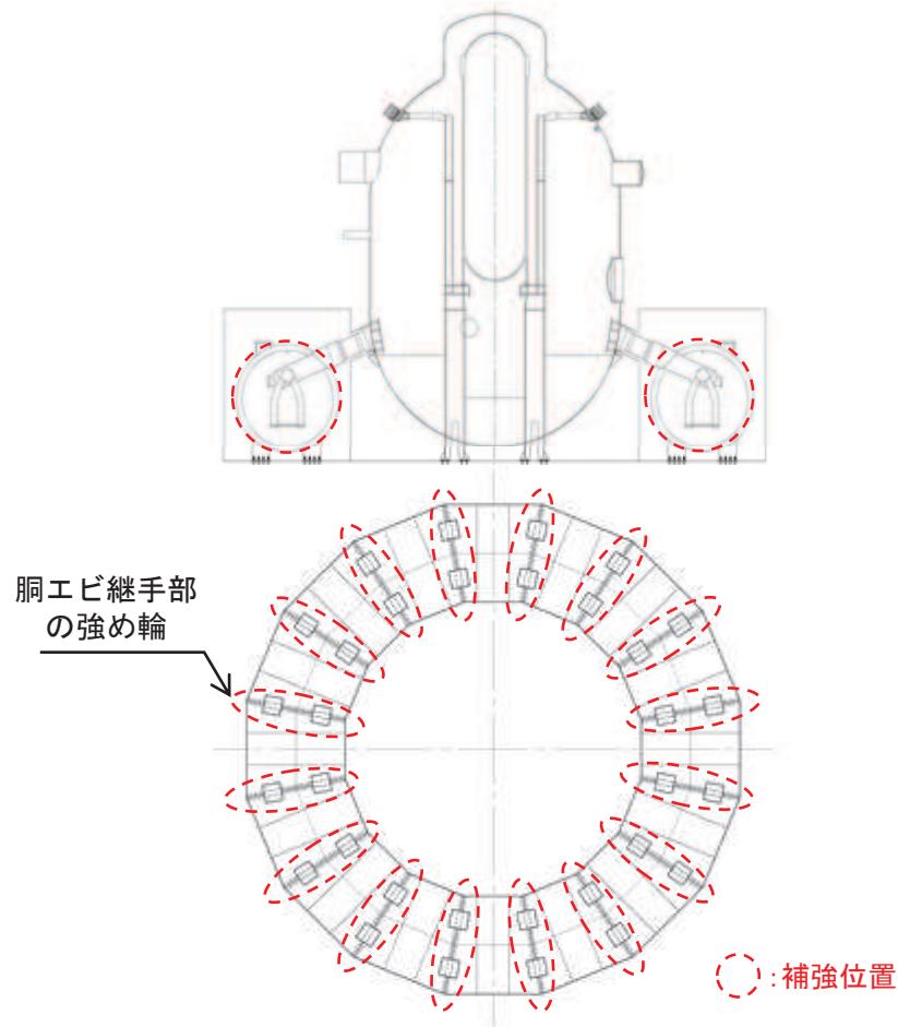
サプレッションチェンバ本体の補強位置
