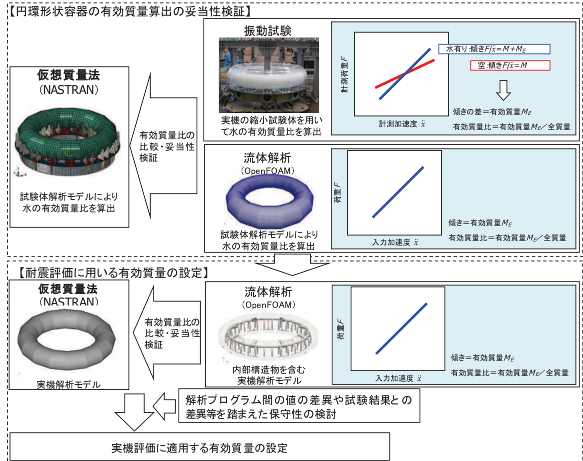
有効質量算定に係る妥当性確認フロー
