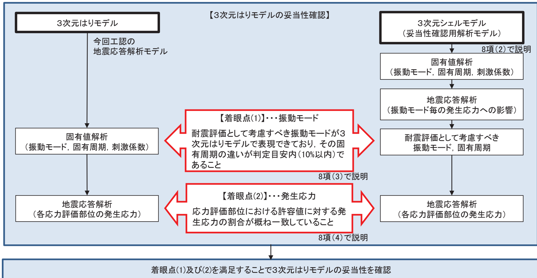
今回工認の地震応答解析モデル(3次元はりモデル)の妥当性確認フロー
