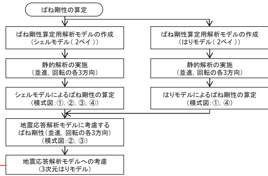
図B ボックスサポート取付部のばね剛性算定フロー
