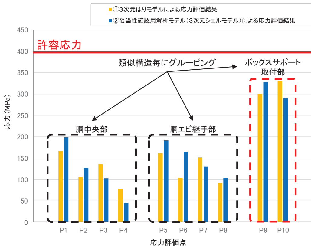
サブレーションチェンバ本体の応力比較結果
