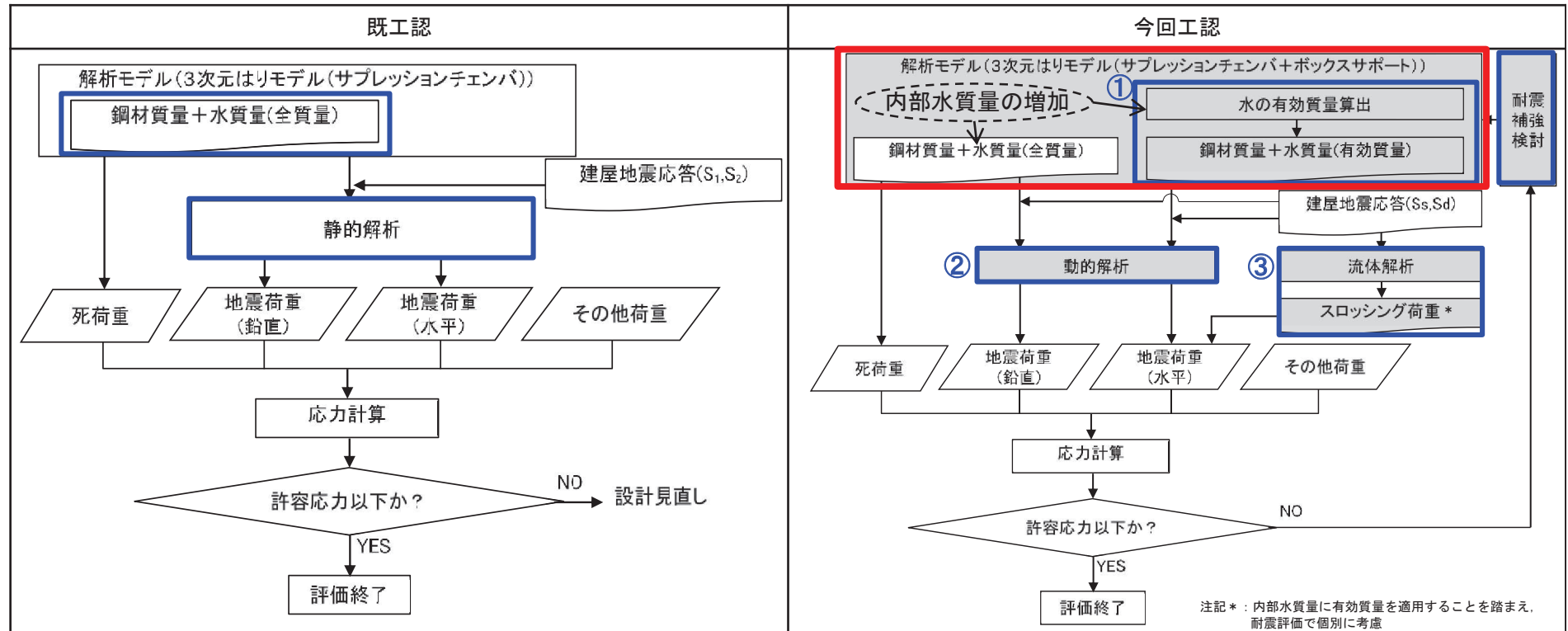
既工認及び今回工認における耐震評価フロー
