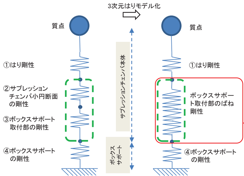
図A サプレッションチェンバとボックスサポートの質量・剛性模式図
