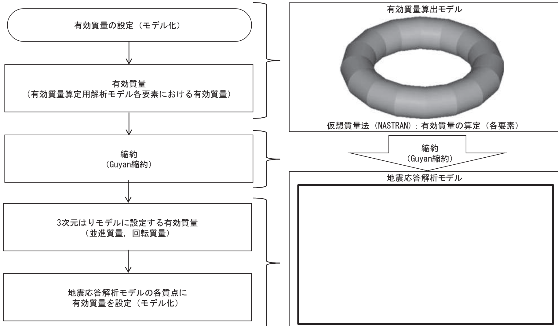
地震応答解析モデルに対する有効質量の設定フロー
