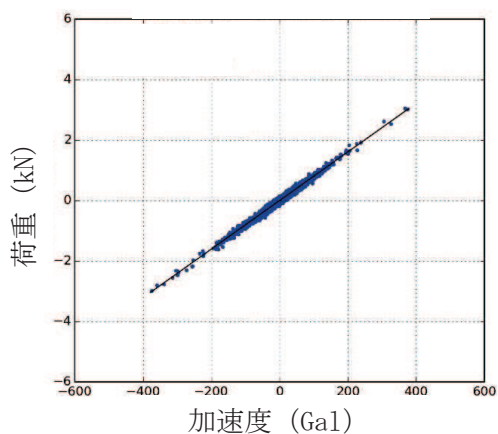
(a) 水位高, 入力倍率 1.0 倍, スロッシング周期成分有りし
