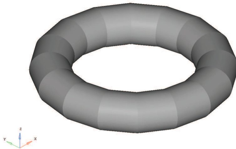
図 4.1-2 内部水の有効質量算定用解析モデル
