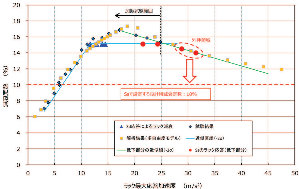
図8 燃料ラックの減衰挙動に係る解析結果と試験結果 (解析結果の横軸を -3\text{m/s}^2 シフト)
