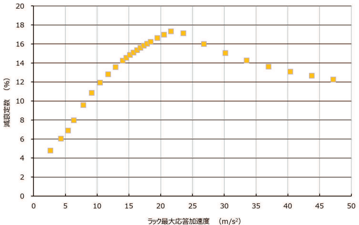
図7 燃料ラックの減衰挙動に係る解析結果 (多自由度モデル)
