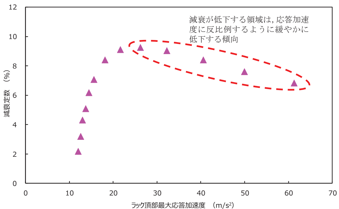
図 5 燃料ラックの減衰挙動に係る解析結果 (構造減衰及び摩擦減衰のみに着目した 1 質点系解析)
