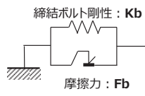
滑り変位と摩擦力の関係
