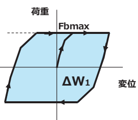
滑り変位と摩擦力の関係
