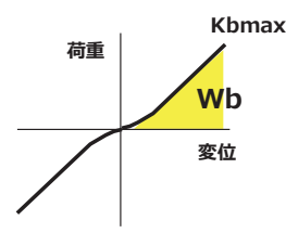
滑り変位とばね力の関係
