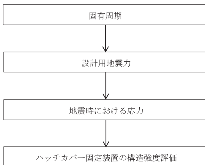
図 1.1.1-1 ハッチカバー固定装置の強度評価フロー
