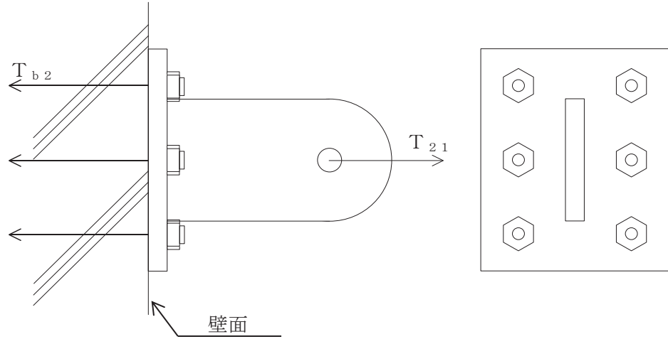
図 1.3.6-2 計算モデル
