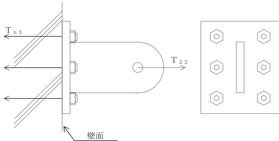
図 1.3.6-3 計算モデル
