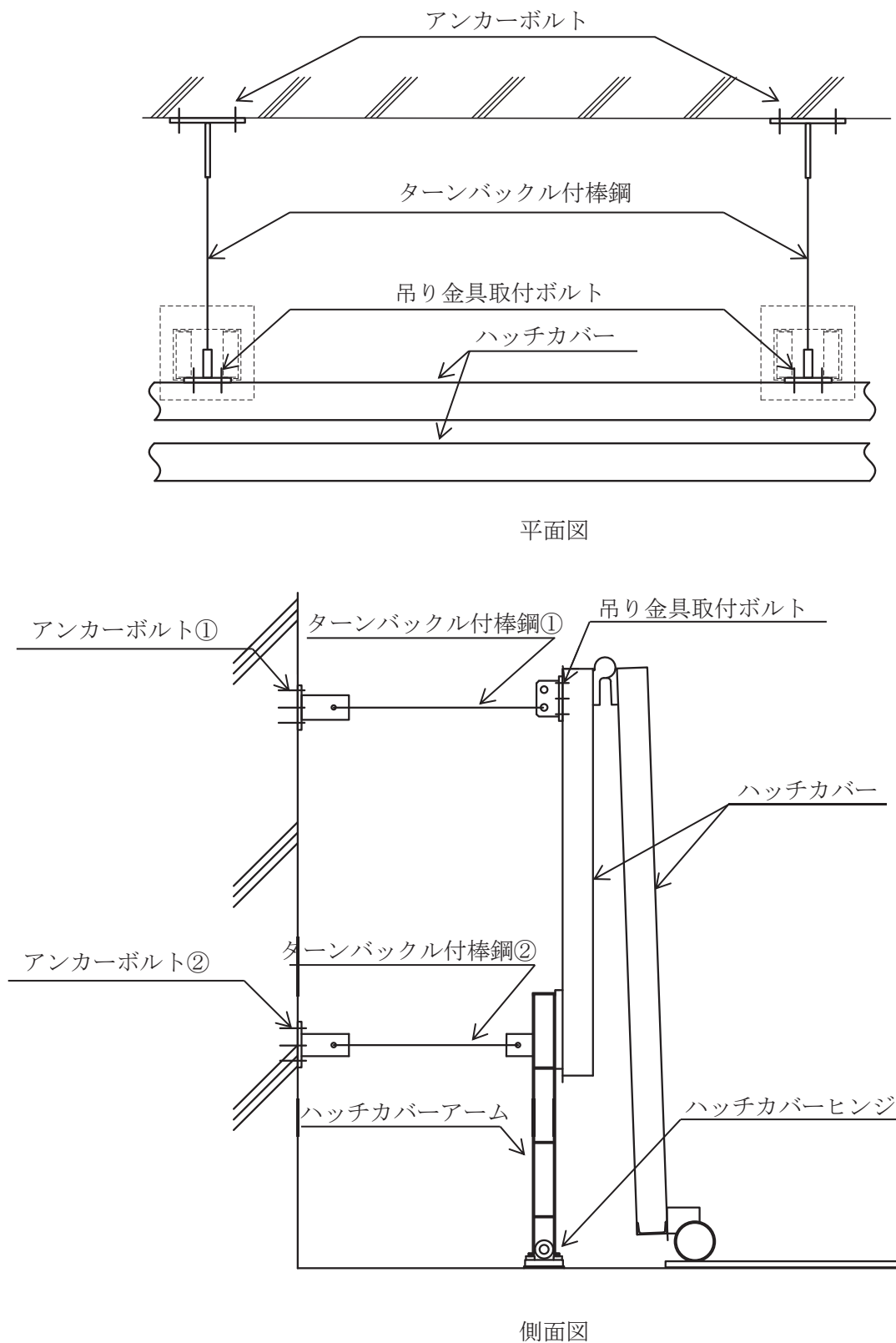
図 1.2-1 ハッチカバー固定装置の概略構造図
