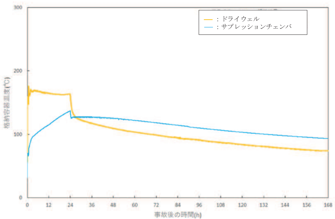
図2 原子炉格納容器温度(有効性評価シナリオ条件(代替循環冷却系を使用する場合), 感度解析)
