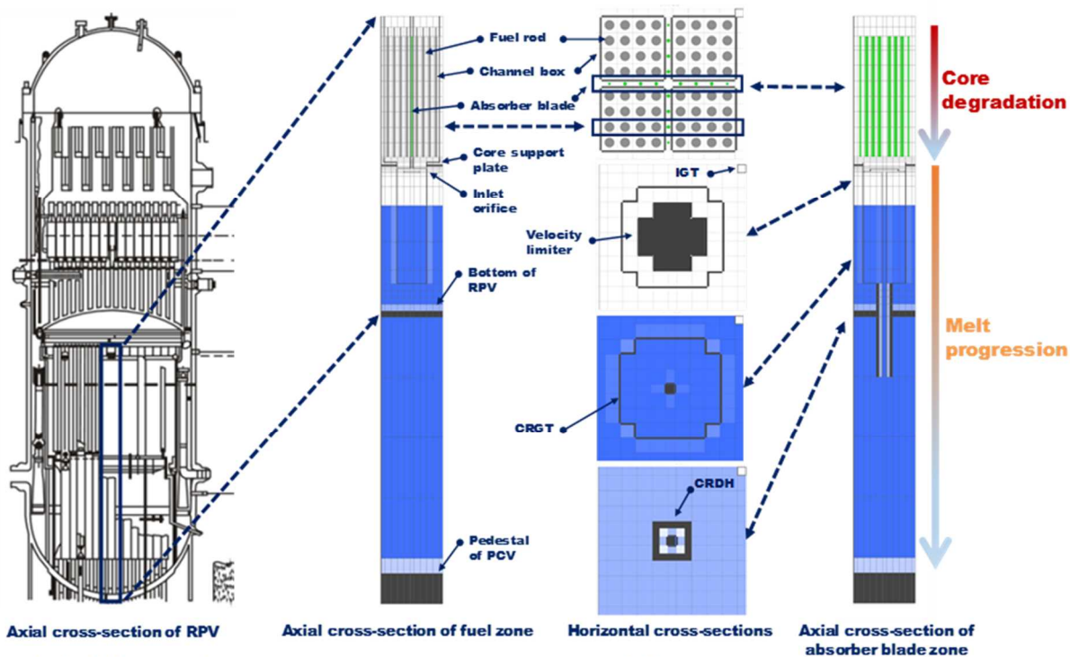
図1 BWR 原子炉圧力容器下部を対象とした詳細幾何形状モデルの縦断面と水平断面
