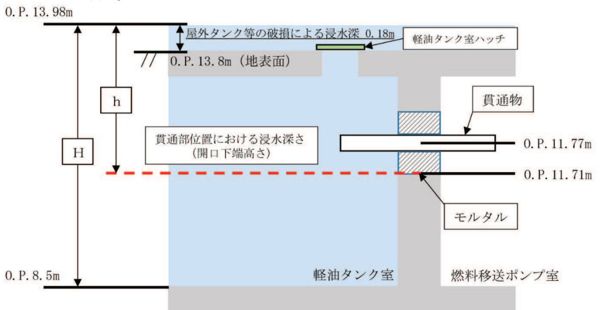
図 4-5 貫通部止水処置 (モルタル) に加わる荷重の概要
