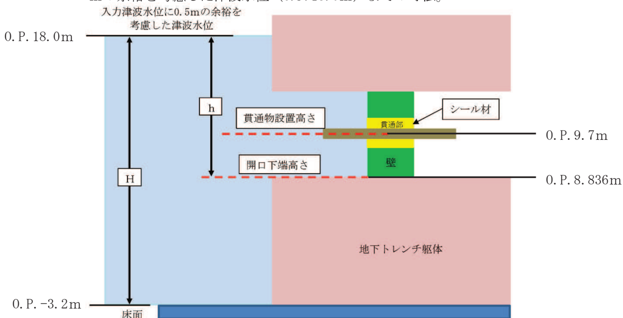
図 4-3 貫通部止水処置（貫通軸：水平）に加わる津波の概要
