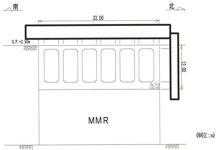
図 2-4 取水口断面図 (A-A 断面, 南北 (標準部))
