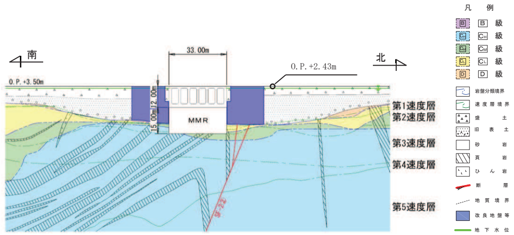
图 2-14 取水口，貯留堰 地震時荷重算出用地質断面図 (A-A 断面，南北 (標準部))
