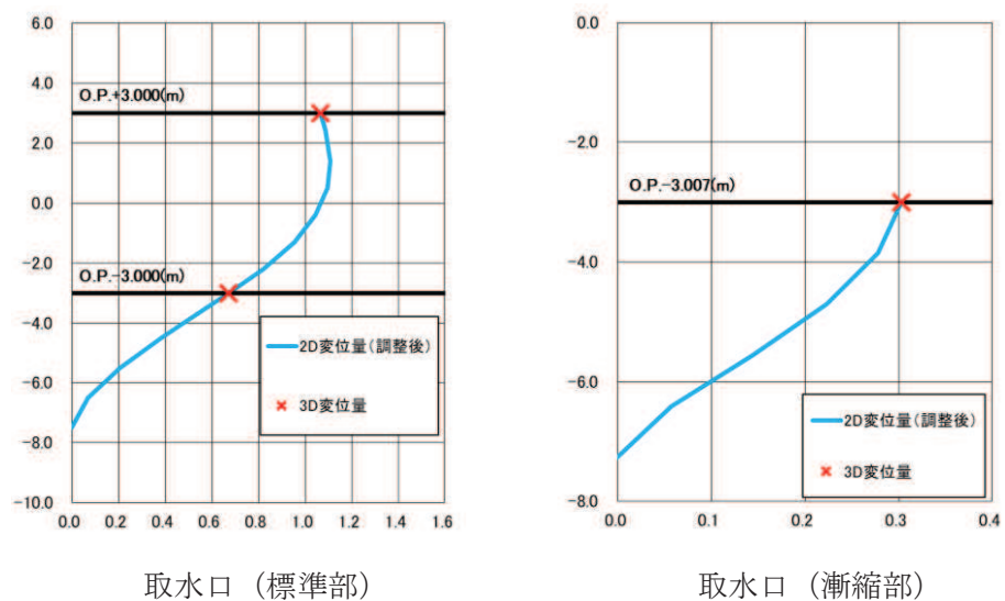
図 3-15 剛性調整結果
