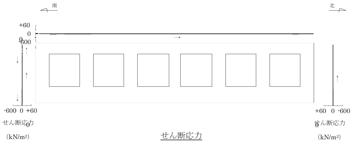
図 6-3 作用荷重分布図 (直応力及びせん断応力) (解析ケース①, S s - D 2 (-+), B-B 断面 (漸縮部), t = 25.06s)
