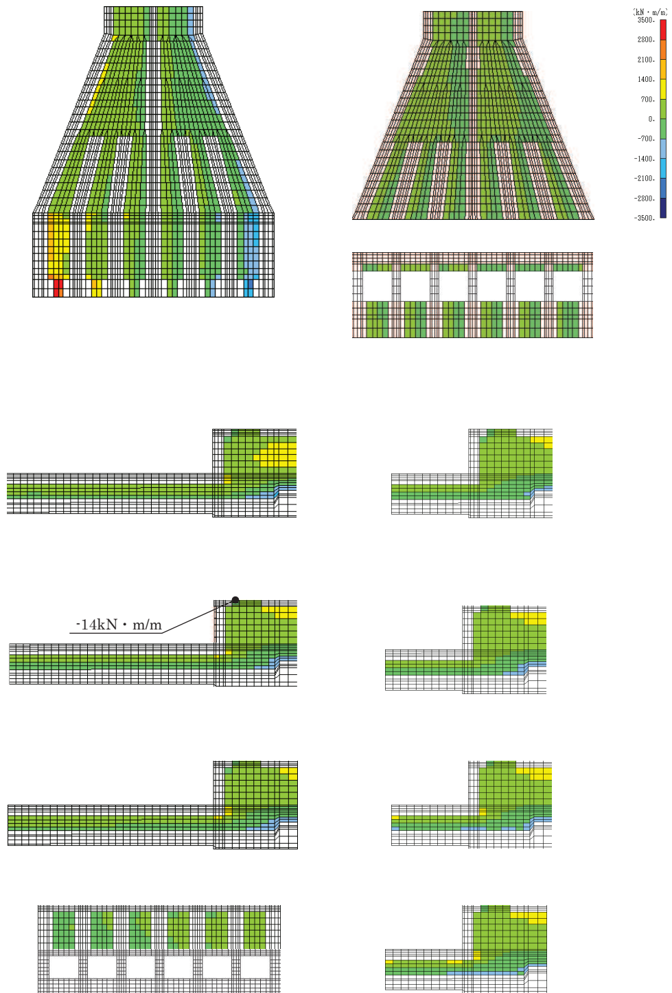
図 6-18 せん断破壊に対する照査値最大時の断面力分布図 (曲げモーメント (kN・m/m) : M_x ) (導流壁, 解析ケース①, 地震動 S_s - D2 (-+)) (標準部 t = 25.07s , 漸縮部 t = 25.06s )
