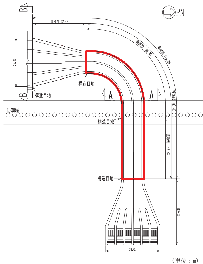
図 2-3 取水路（標準部）平面図
