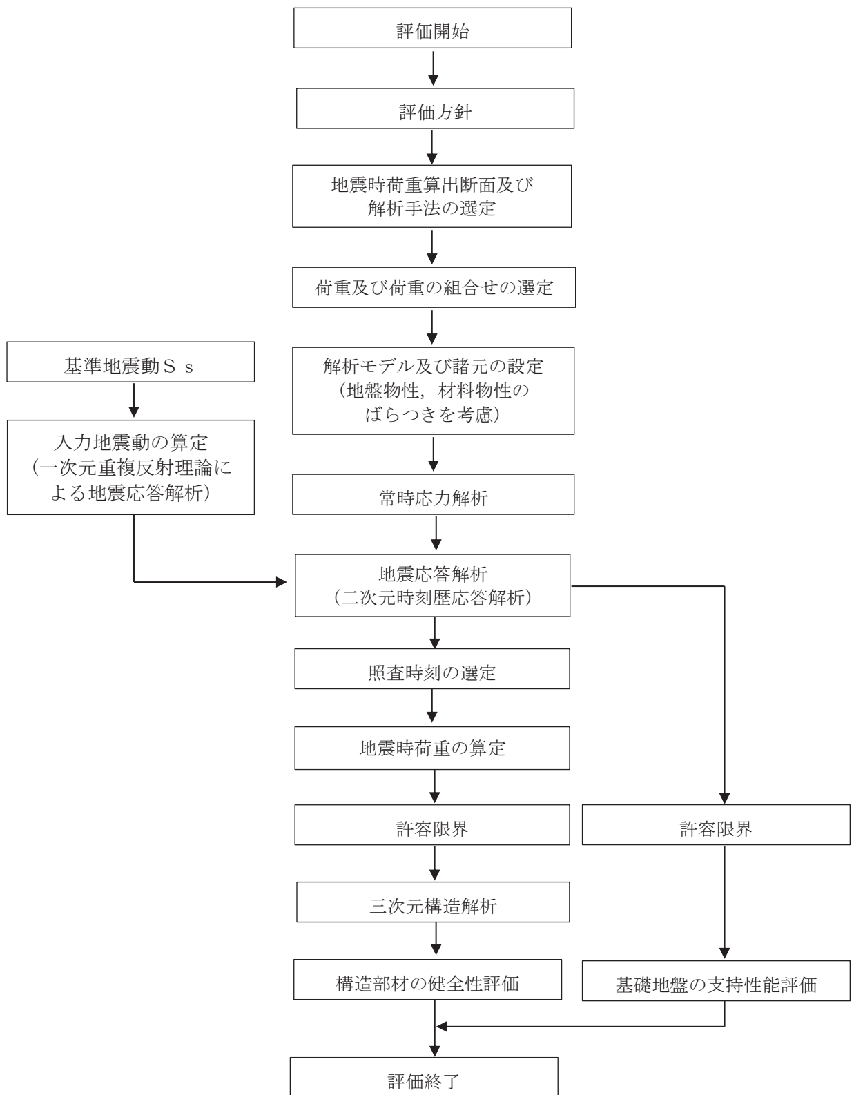
図 2-1 取水口，貯留堰の耐震評価フロー
