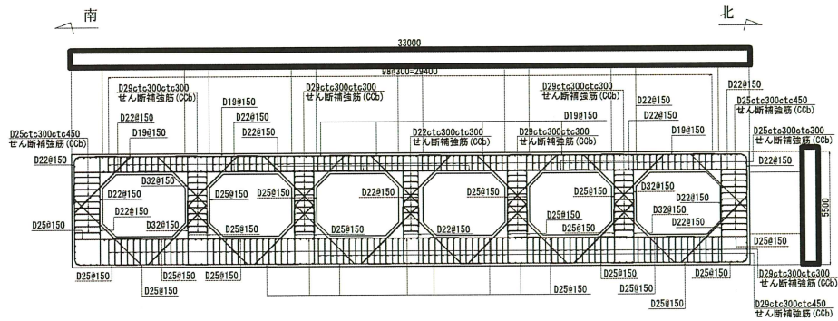
図 2-10 取水口，貯留堰概略配筋図（B-B 断面，南北（漸縮部））
