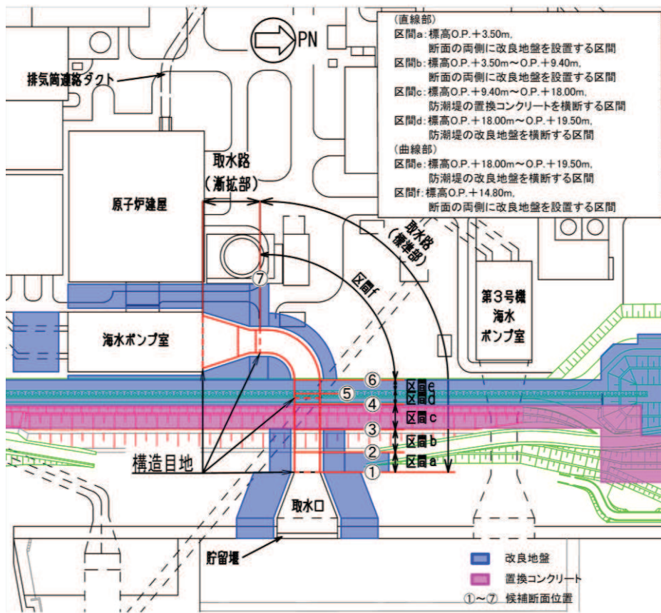
図 2-6 取水路平面図 (区間及び地震時荷重断面位置)
