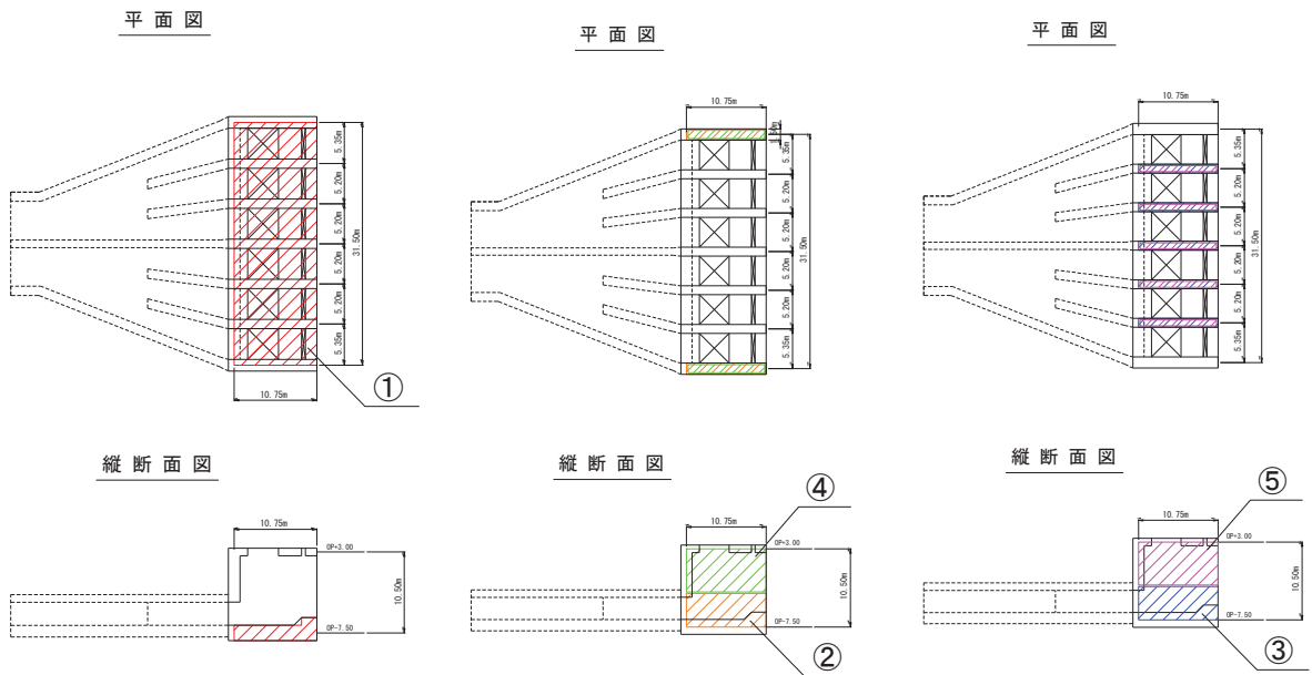
図3-11(2) 取水口の等価剛性モデル (はり部材番号①, ②, ③, ④, ⑤) (2/3)
