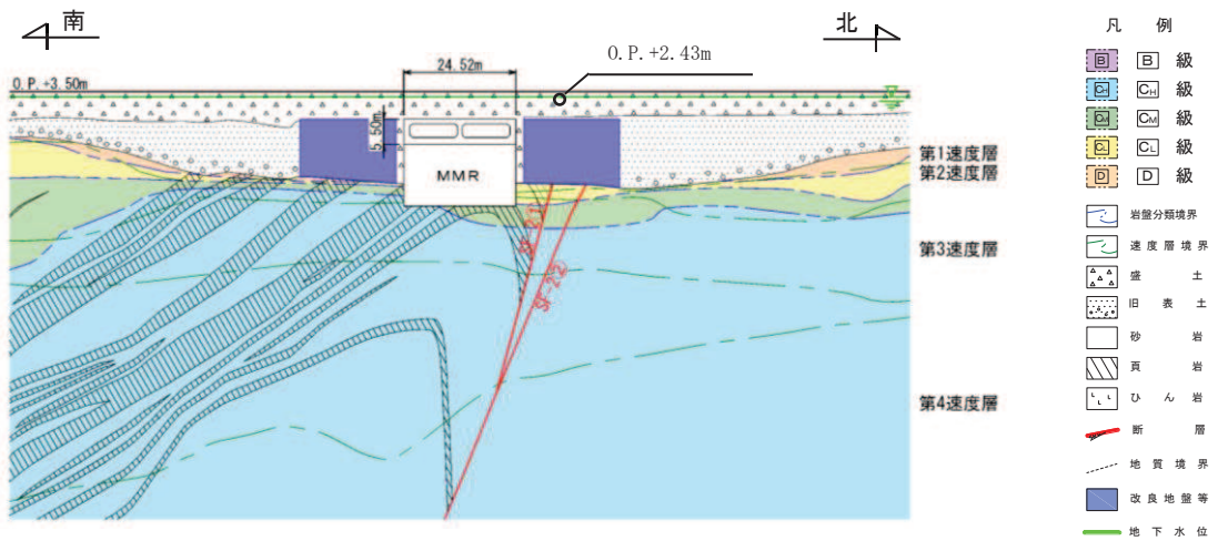
图 2-15 取水口，貯留堰 地震時荷重算出用地質断面図 (C-C 断面，南北 (漸縮部))
