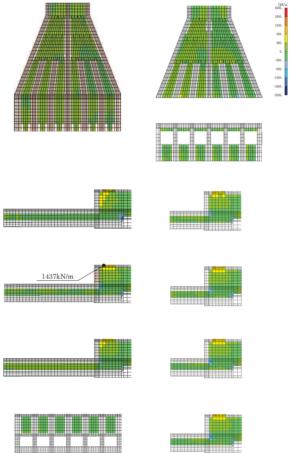
図 6-23 せん断破壊に対する照査値最大時の断面力分布図 (せん断力 (kN/m) : Q_y ) (導流壁, 解析ケース①, 地震動 S_s - D2 (-+)) (標準部 t = 25.07s , 漸縮部 t = 25.06s )
