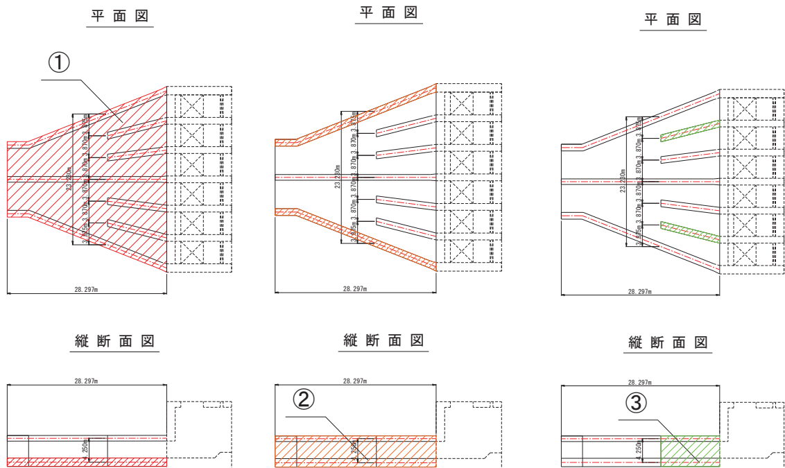
図3-12(2) 取水口の等価剛性モデル (はり部材番号①, ②, ③) (2/3)
