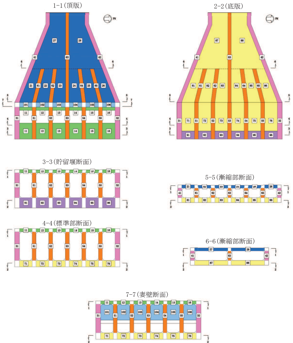
図 6-17 評価位置図 (曲げ・軸力系の破壊及びせん断破壊)
