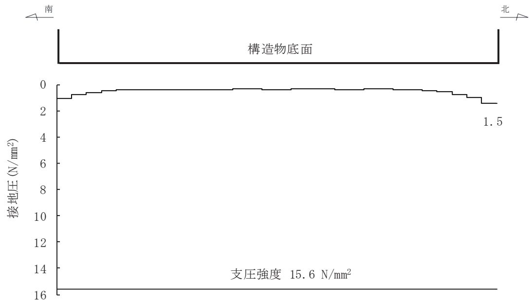
図 6-28 MMR (既設) の最大接地圧分布図 (解析ケース②, S s -D 2 (-+), A-A断面 (標準部))
