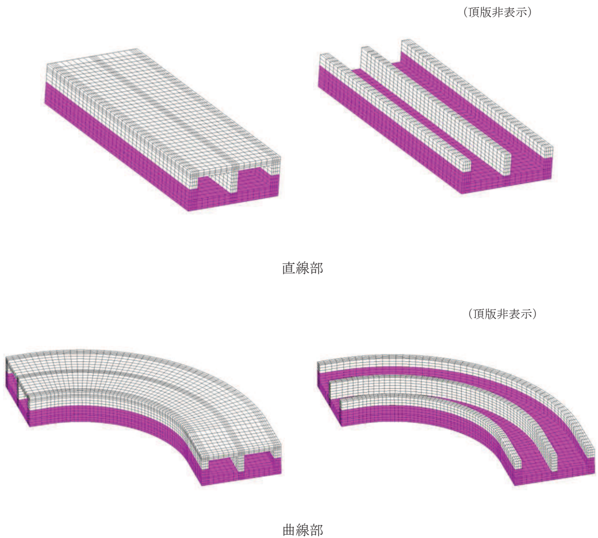
図2-17 貯水機能が要求される部材の範囲
