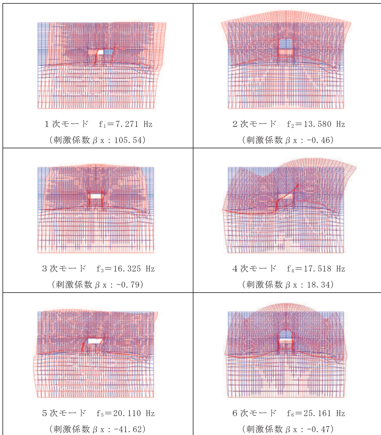
図 3-28(1) 固有値解析結果 (モード図) (断面④) (1/2)
