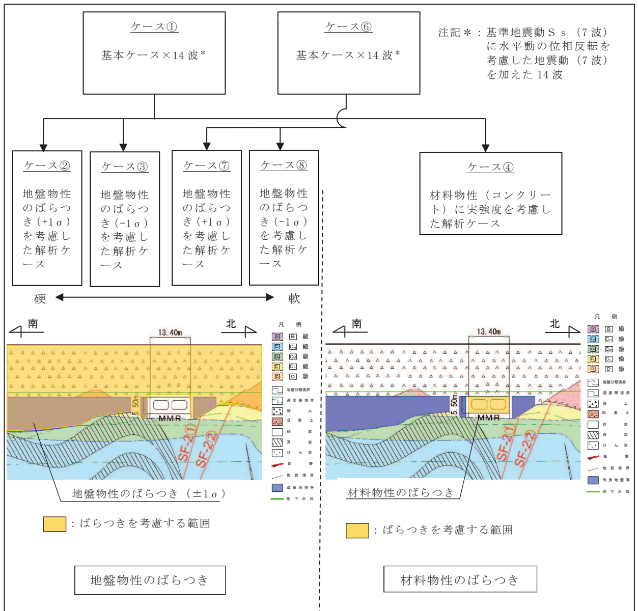
図 3-49 耐震評価における解析ケース
