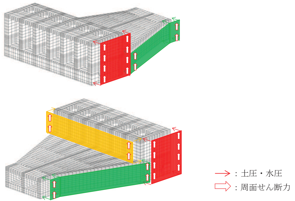
図 4-21 地震時土圧・水圧及び周面せん断力の概念図
