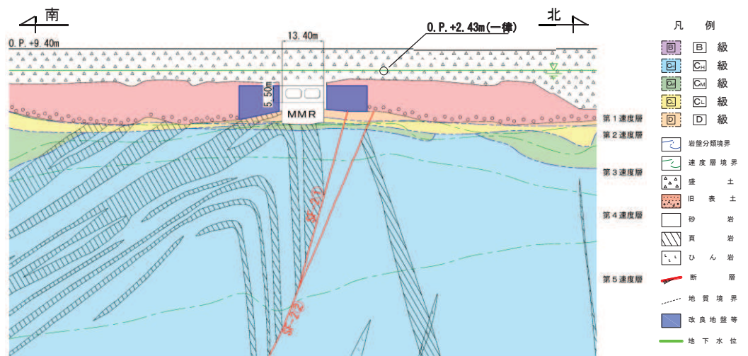
图 2-19 设计用地下水位 (断面③)
