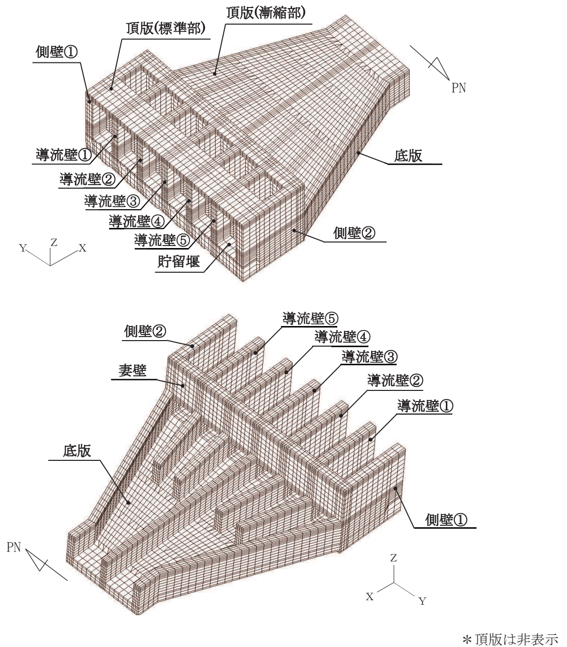
図6-9 各部材位置
