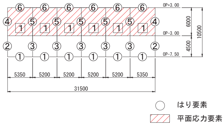
図3-11(1) 取水口の等価剛性モデル (はり部材番号①, ②, ③) (1/3)
