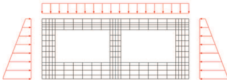
図4-14 静止土圧及び外水圧の载荷概念図
