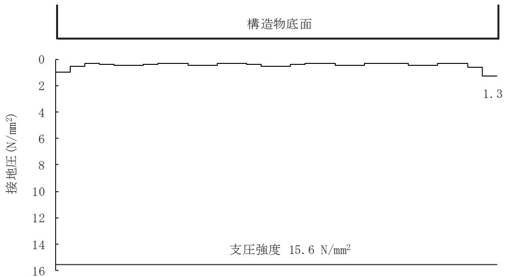
図 6-29 MMR (既設) の最大接地圧分布図 (解析ケース①, S s -D 2 (++) , B-B 断面 (漸縮部))
