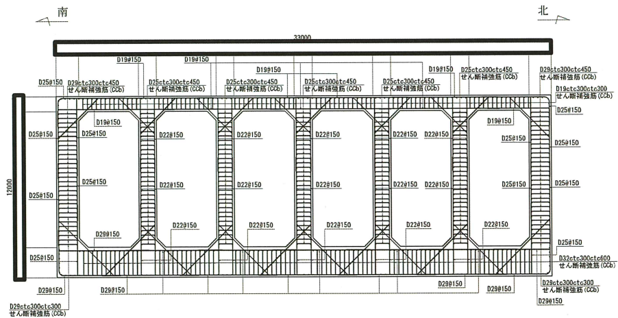
図 2-9 取水口, 貯留堰概略配筋図 (A-A 断面, 南北 (標準部))
