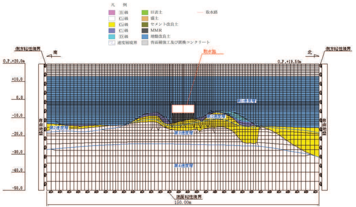
(b) 地震応答解析モデル図
