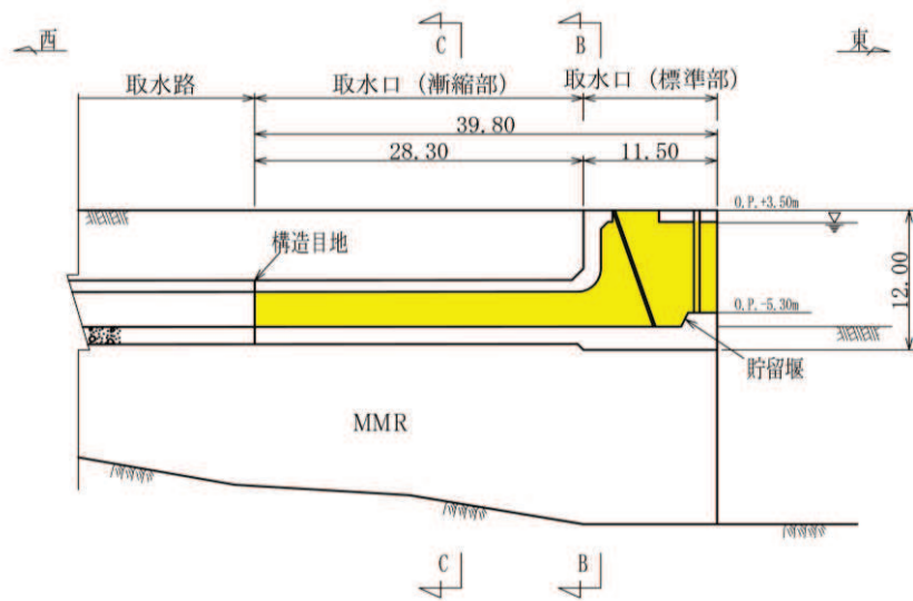
図 5-16(1) Ccb 工法を用いる部材 (平面図)
