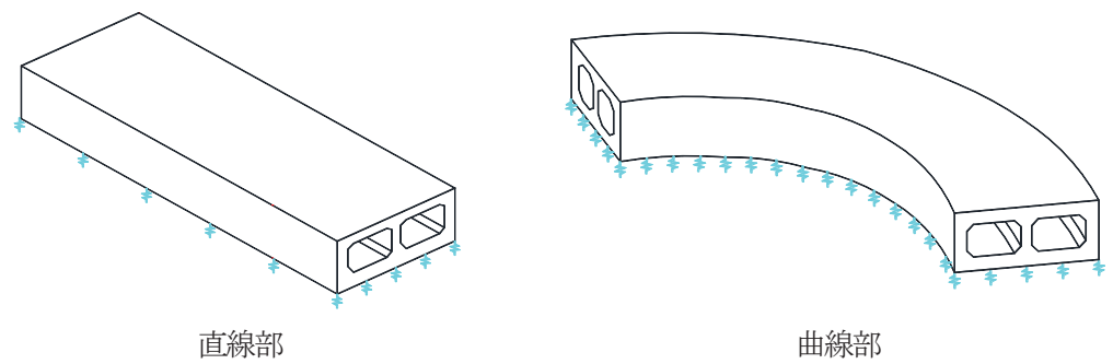
図4-5 地盤ばねの設定イメージ図
