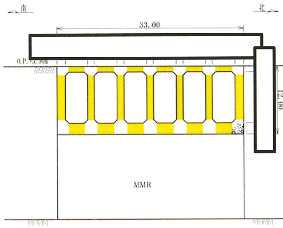
図 5-16(3) Ccb工法を用いる部材 (B-B断面)
