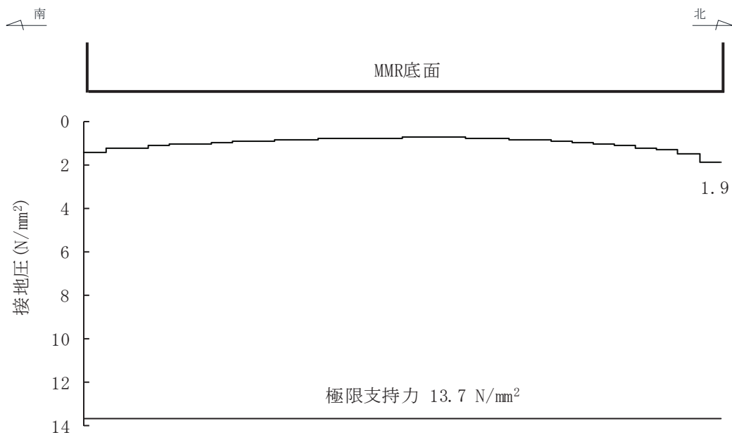
図 6-27 基礎地盤の最大接地圧分布図 (解析ケース③, S s -N 1 (++) , B-B 断面 (漸縮部))
