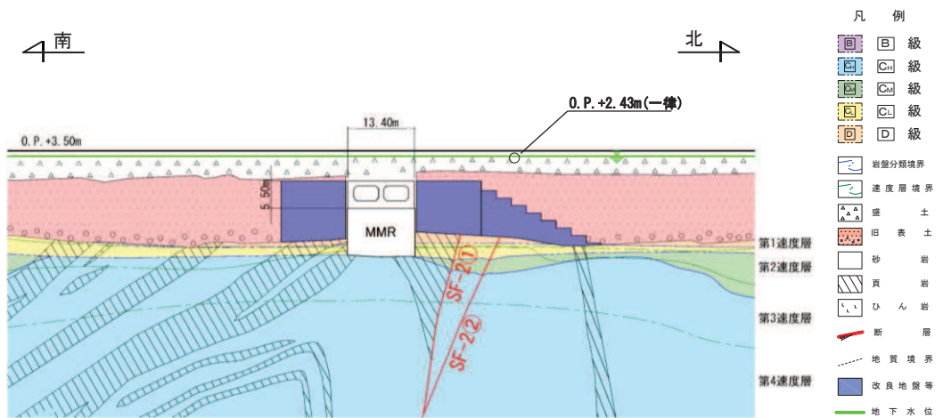
図 2-9 取水路（標準部） 地震時荷重算出用地質断面図（断面②）
