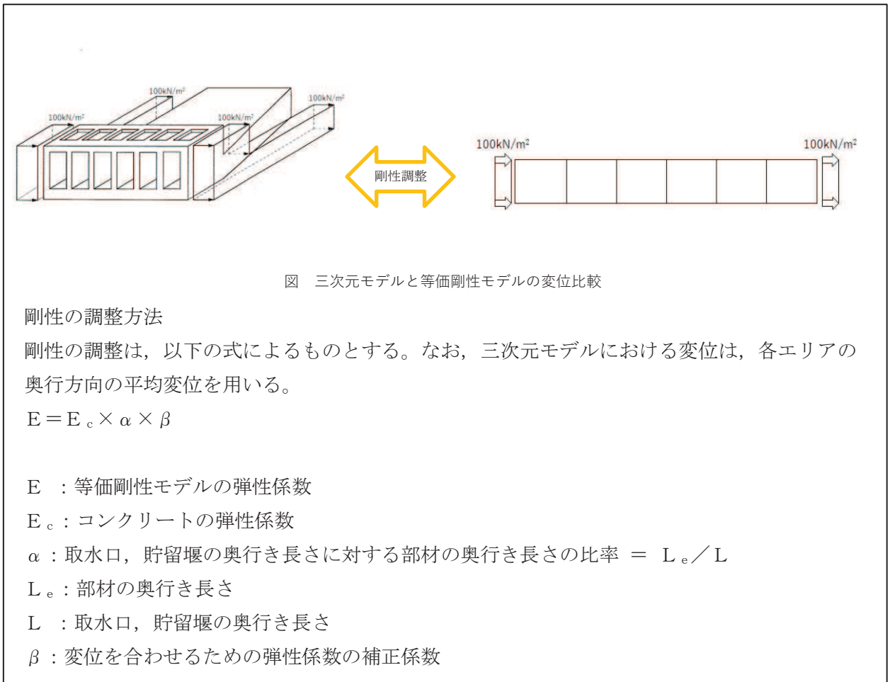
図 3-14 剛性の調整方法
