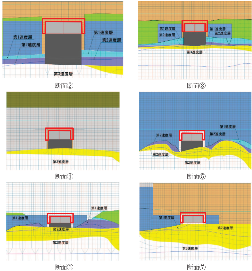
図4-19 地震時土圧・水圧及び周面せん断力の抽出位置
