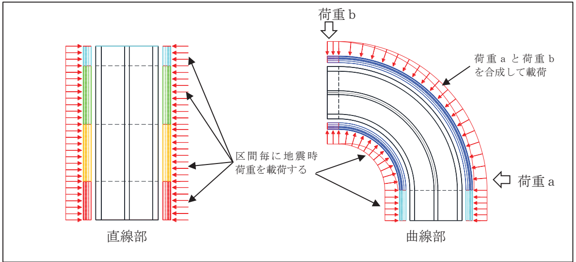
図 2-2 地震時荷重載荷イメージ図
