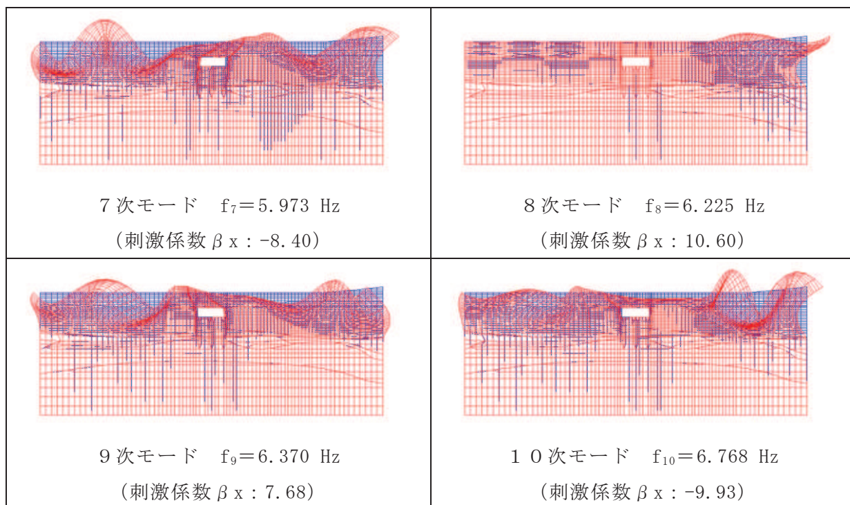
図 3-26(2) 固有値解析結果 (モード図) (断面②) (2/2)
