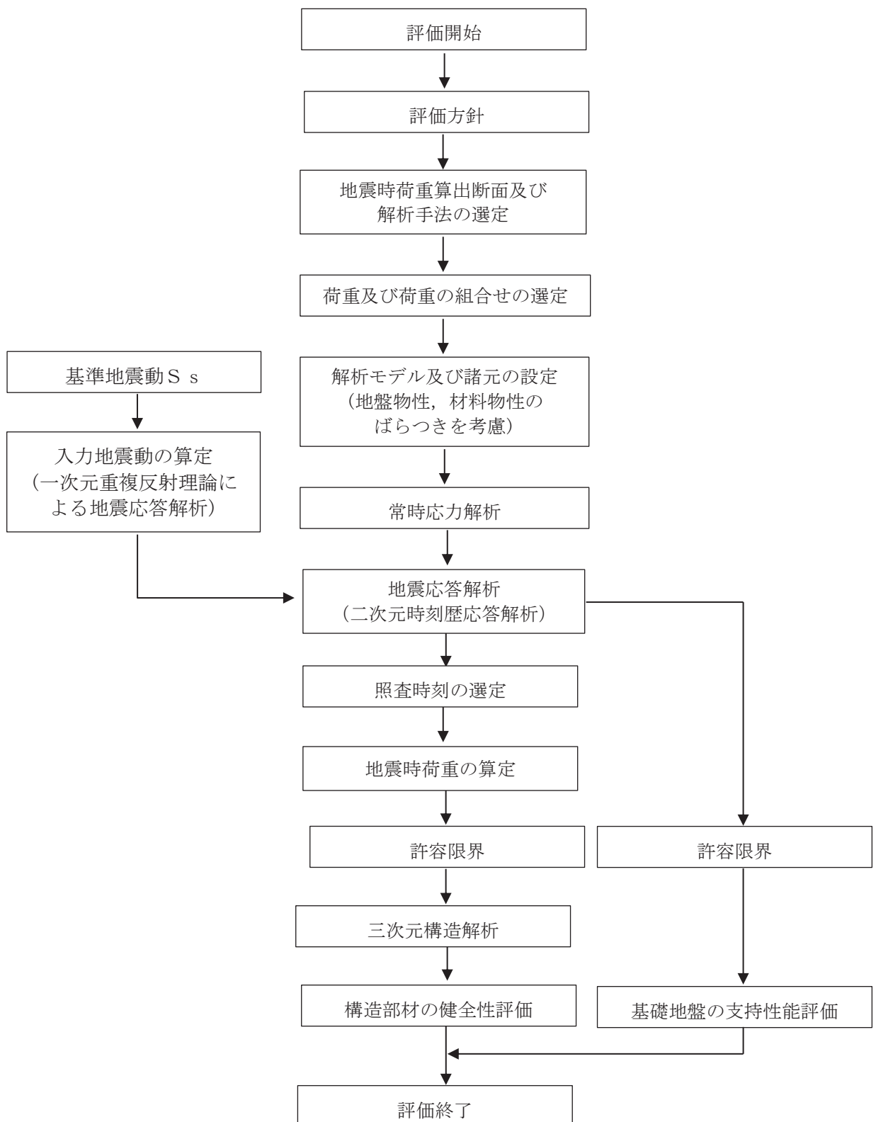
図 2-1 取水路（標準部）の耐震評価フロー
