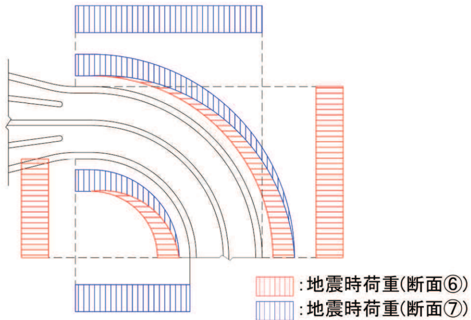
図 2-7 曲線部における荷重載荷イメージ図
