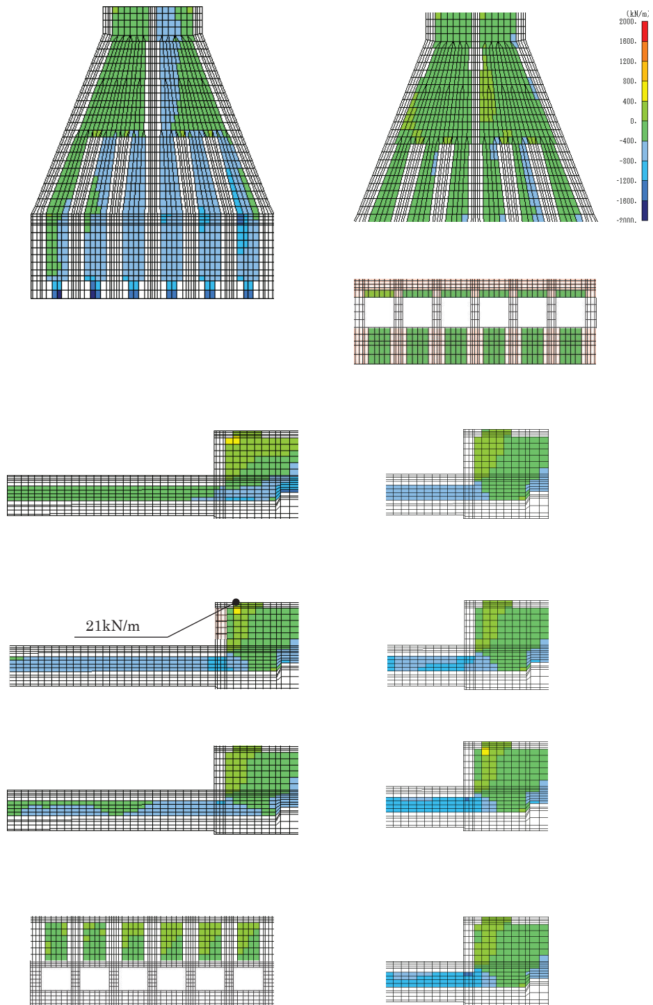
図 6-22 せん断破壊に対する照査値最大時の断面力分布図 (せん断力 (kN/m) : Q_x ) (導流壁, 解析ケース①, 地震動 S_s - D2 (-+)) (標準部 t = 25.07s , 漸縮部 t = 25.06s )
