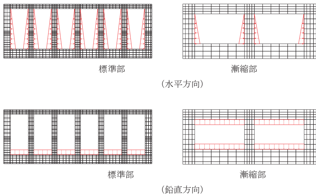
図 4-14 内水圧の概念図 (南北方向)
