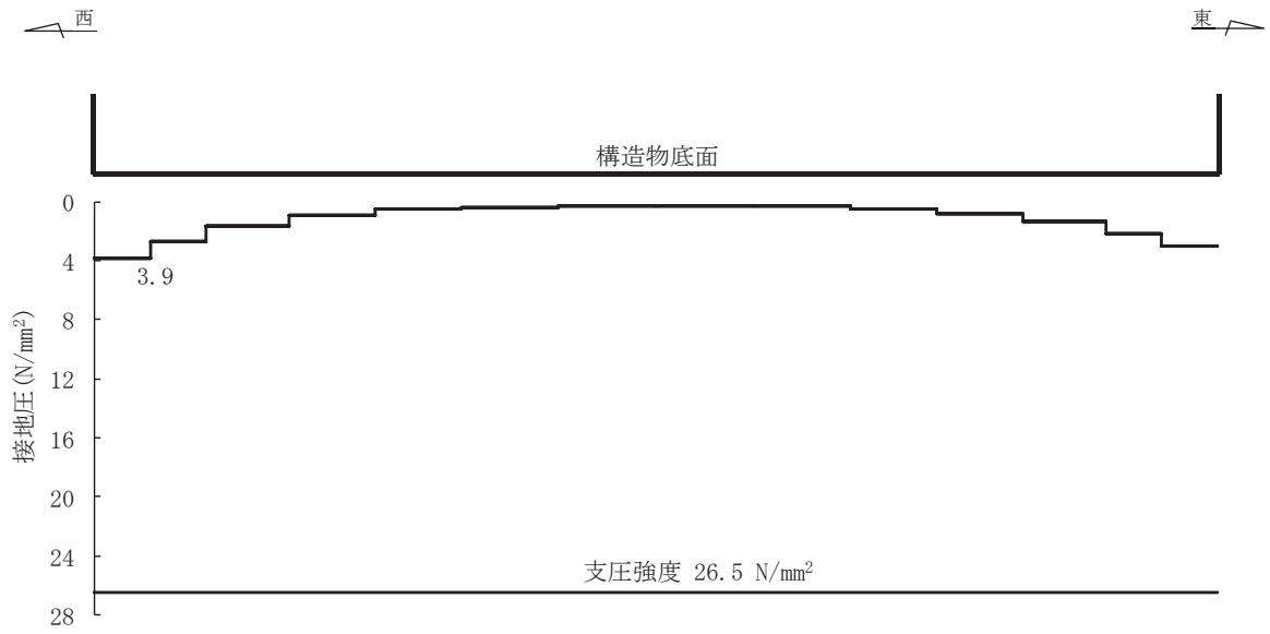
図 6-16 MMR (新設) の最大接地圧分布図 (解析ケース③, S s - D 2 (++) )
