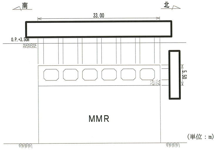
図 2-5 取水口断面図 (B-B 断面, 南北 (漸縮部))
