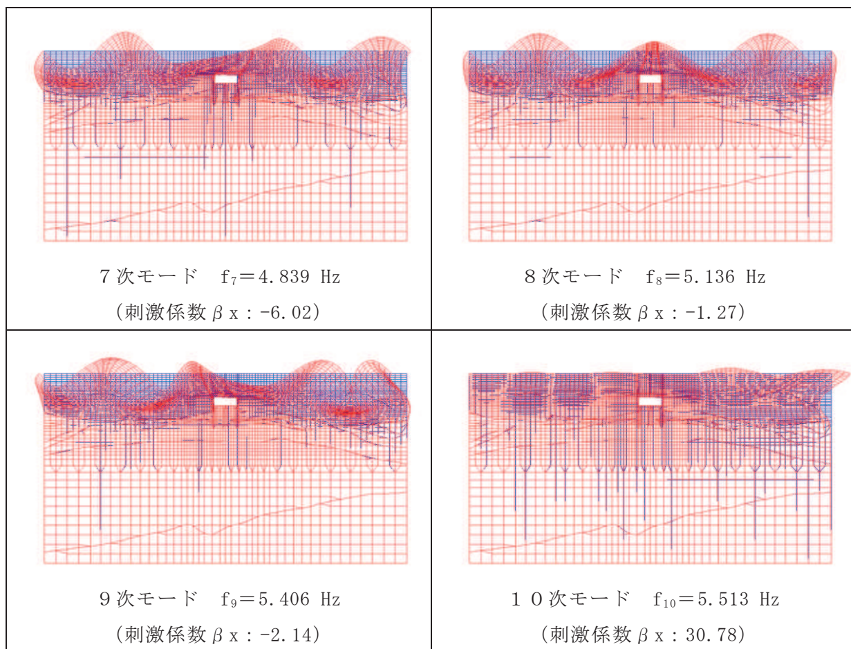
図 3-27(2) 固有値解析結果 (モード図) (断面③) (2/2)
