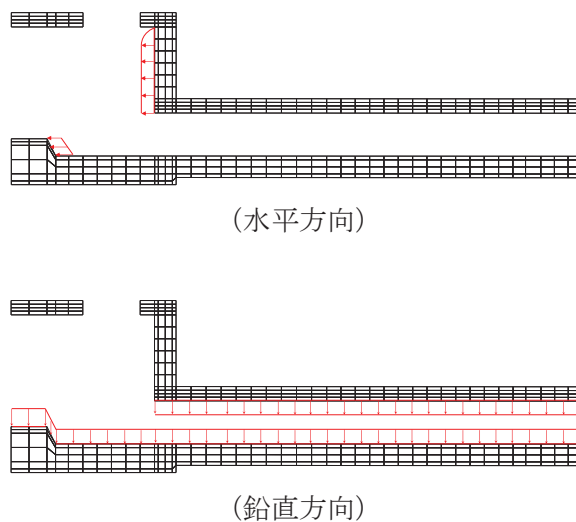
図4-19 動水圧の概念図（東西方向）
