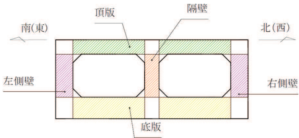
断面図
