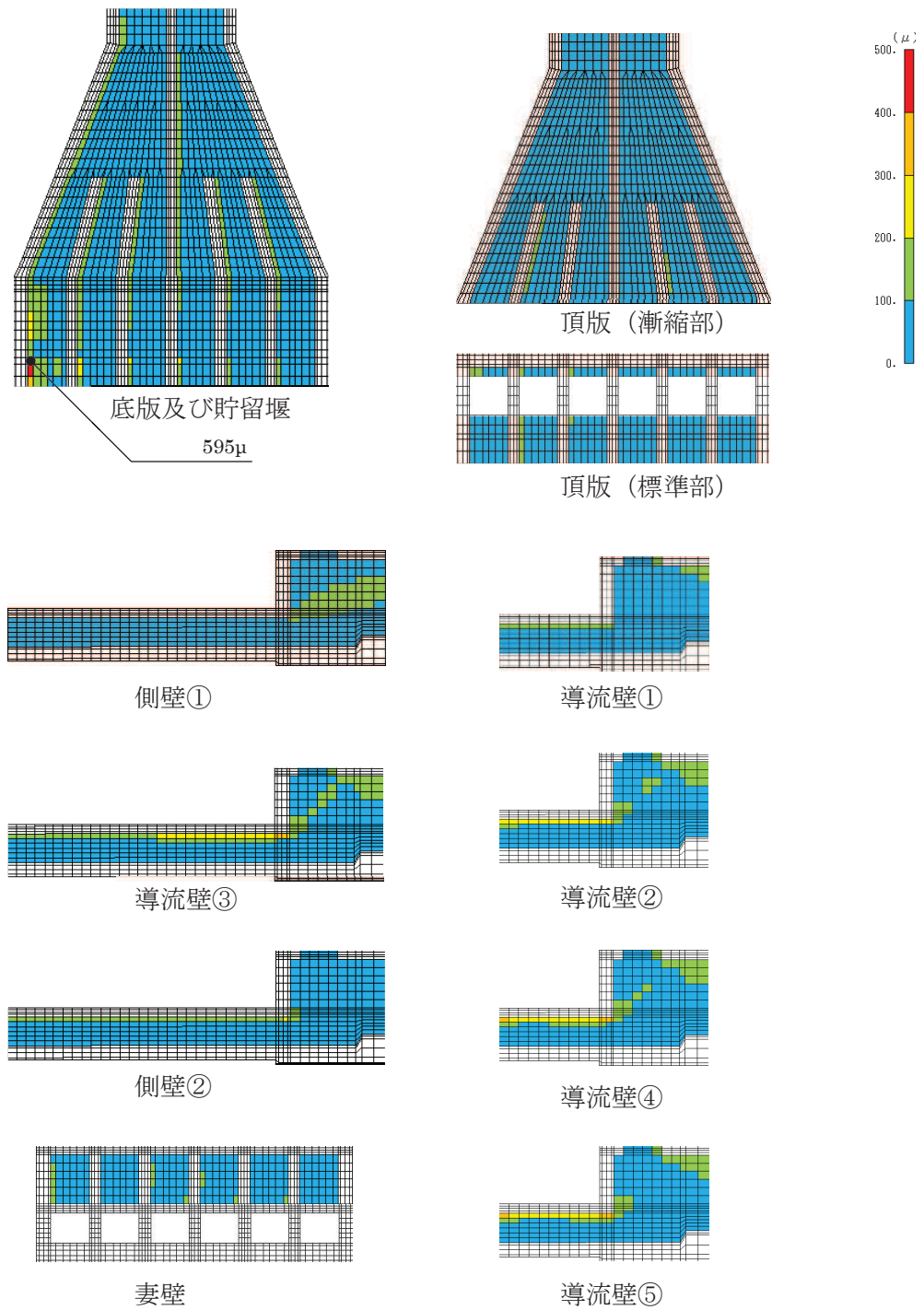
図 6-14 曲げ・軸力系の破壊に対する照査値最大時のひずみ分布図 (コンクリートの圧縮縁ひずみ) (貯留堰, 解析ケース③, 地震動 S s - D 2 (-+)) (標準部 t = 25.08s , 漸縮部 t = 25.06s )
