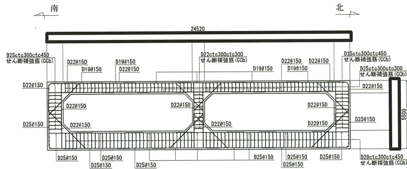
図 2-11 取水口概略配筋図（C-C 断面，南北（漸縮部））
