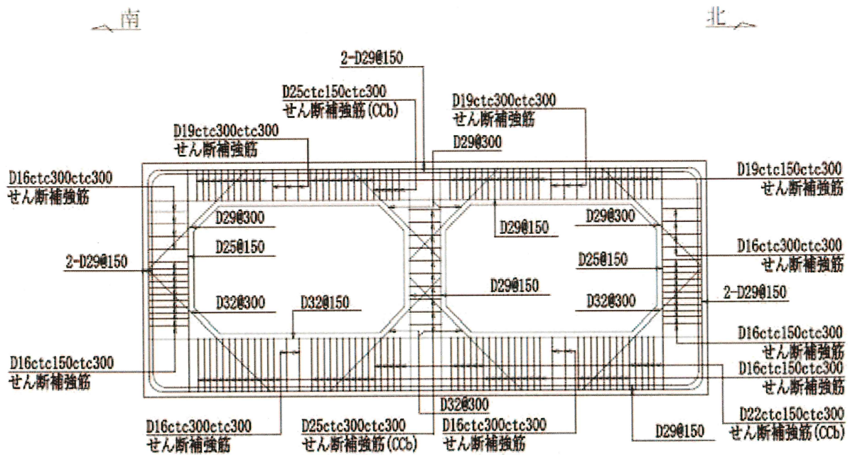
図 2-5 取水路（標準部）概略配筋図（A-A 断面）
