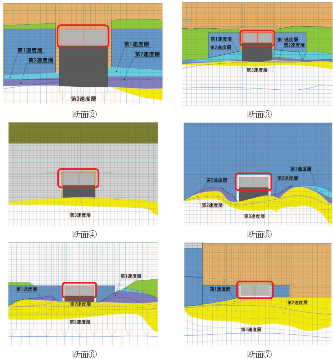
図4-16 応答加速度の抽出位置
