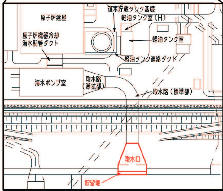
図 2-2 取水口位置図
