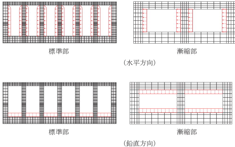
図4-18 動水圧の概念図（南北方向）
