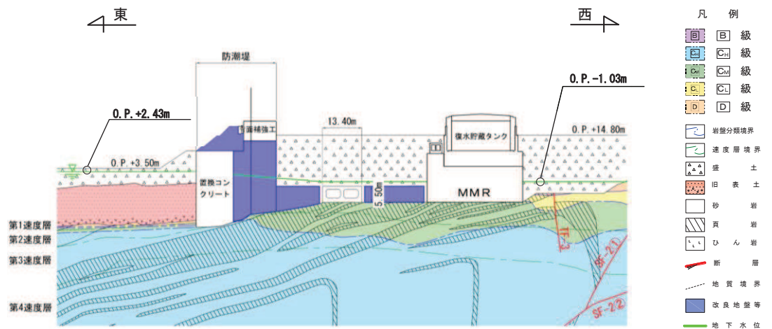
図 2-23 設計用地下水位 (断面⑦)
