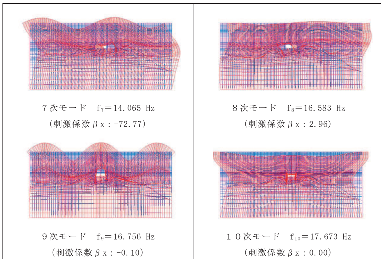
図 3-29(29) 固有値解析結果 (モード図) (断面⑤) (2/2)
