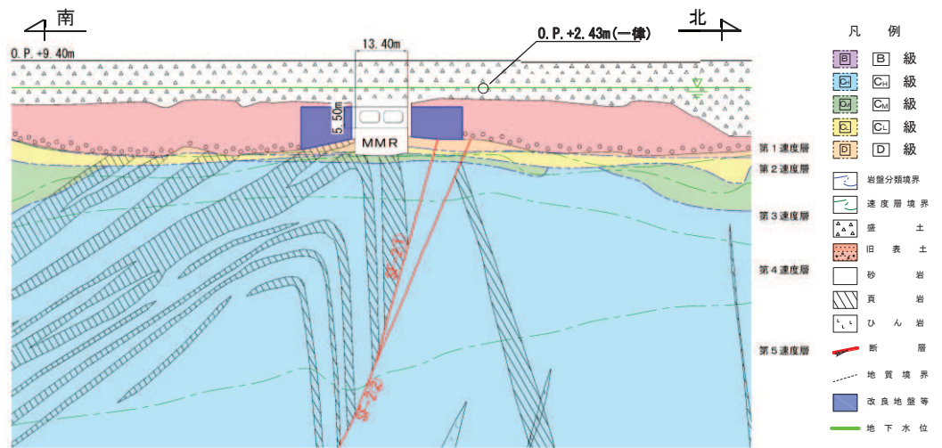
図 2-10 取水路（標準部） 地震時荷重算出用地質断面図（断面③）
