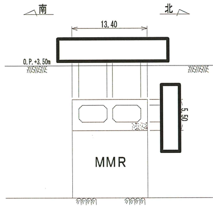
図 2-7 取水口断面図 (D-D 断面, 南北 (漸縮部))
