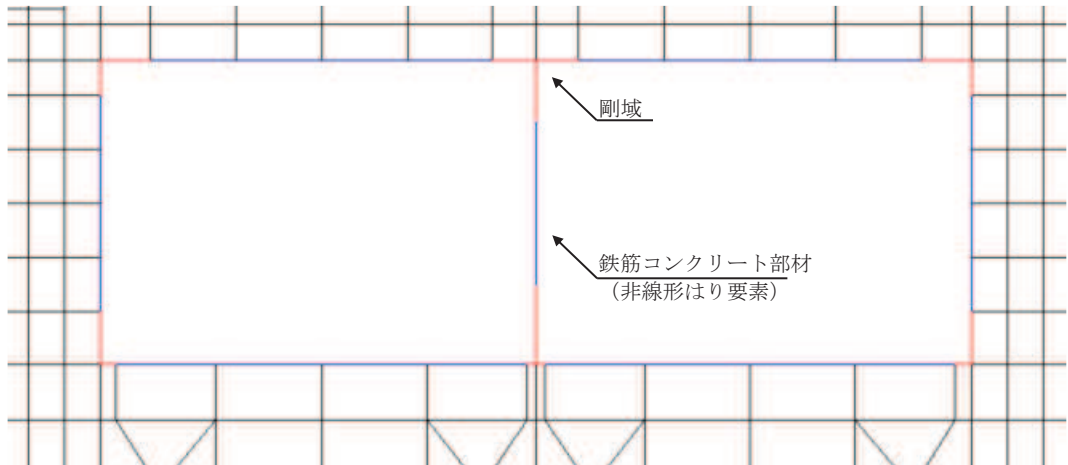
図 3-13 取水路（標準部）の地震応答解析モデル図 （構造物部分拡大）
