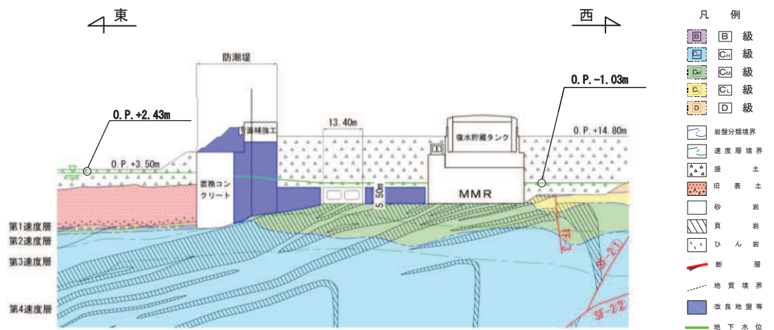
図 2-14 取水路（標準部） 地震時荷重算出用地質断面図（断面⑦）
