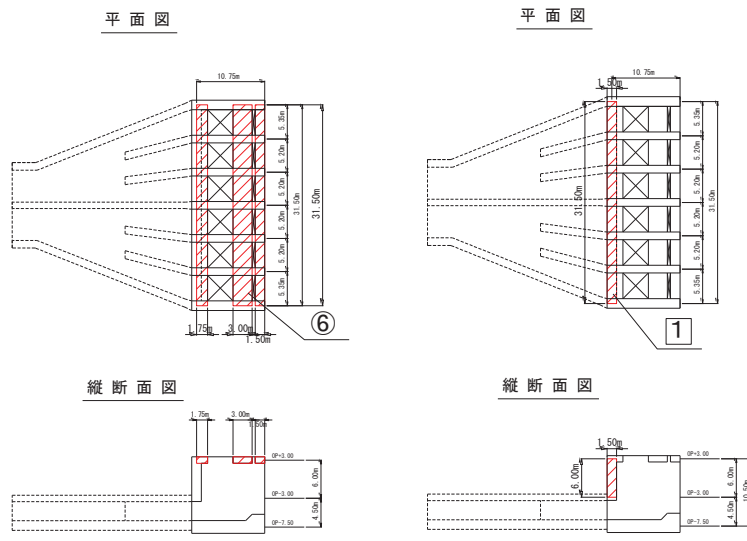
図3-11(3) 取水口の等価剛性モデル (はり部材番号⑥, 平面応力要素1) (3/3)
