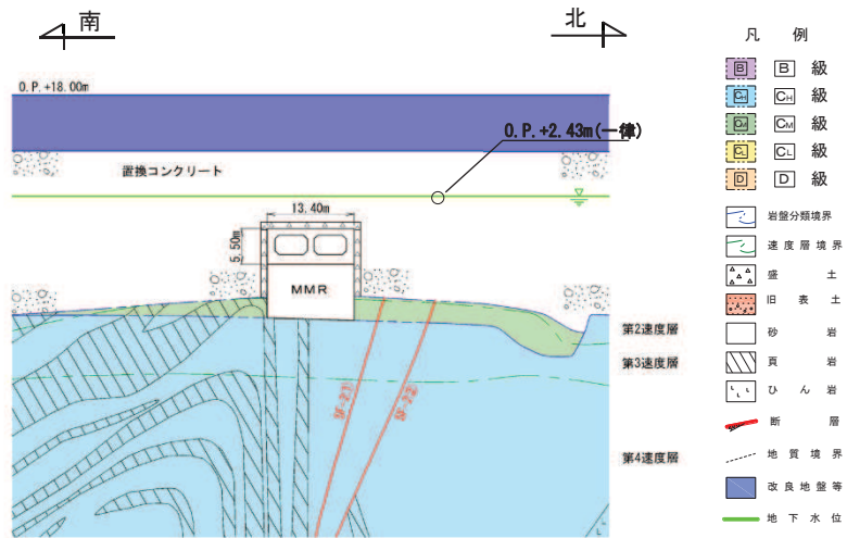
(a) 地震時荷重算出用地質断面図
