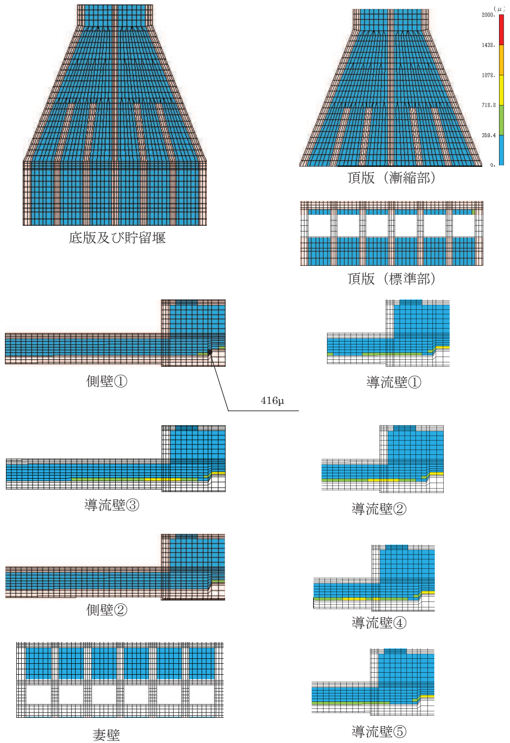
図 6-16 曲げ・軸力系の破壊に対する照査値最大時のひずみ分布図 (鉄筋) (側壁, 解析ケース③, 地震動 S s - D 2 ( - + ) ) (標準部 t = 25.08s , 漸縮部 t = 25.06s )
