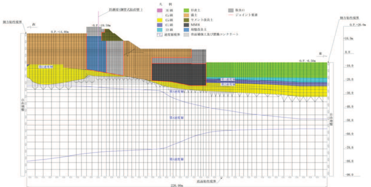
図 3-20 取水口，貯留堰（縦断）のジョイント要素の配置
