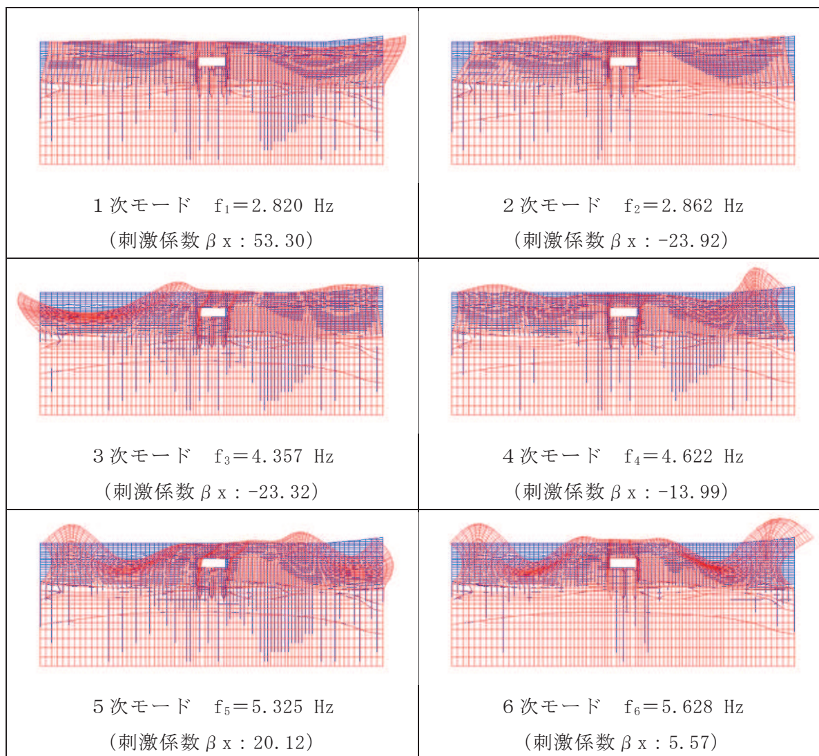
図 3-26(1) 固有値解析結果 (モード図) (断面②) (1/2)
