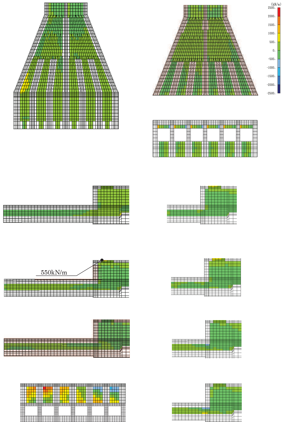
図 6-21 せん断破壊に対する照査値最大時の断面力分布図
