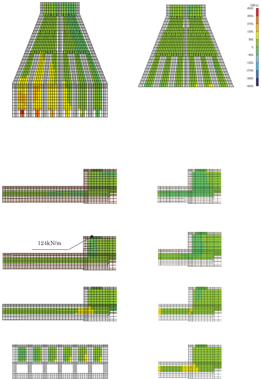
図 6-20 せん断破壊に対する照査値最大時の断面力分布図
