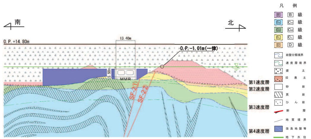
図 2-22 設計用地下水位 (断面⑥)
