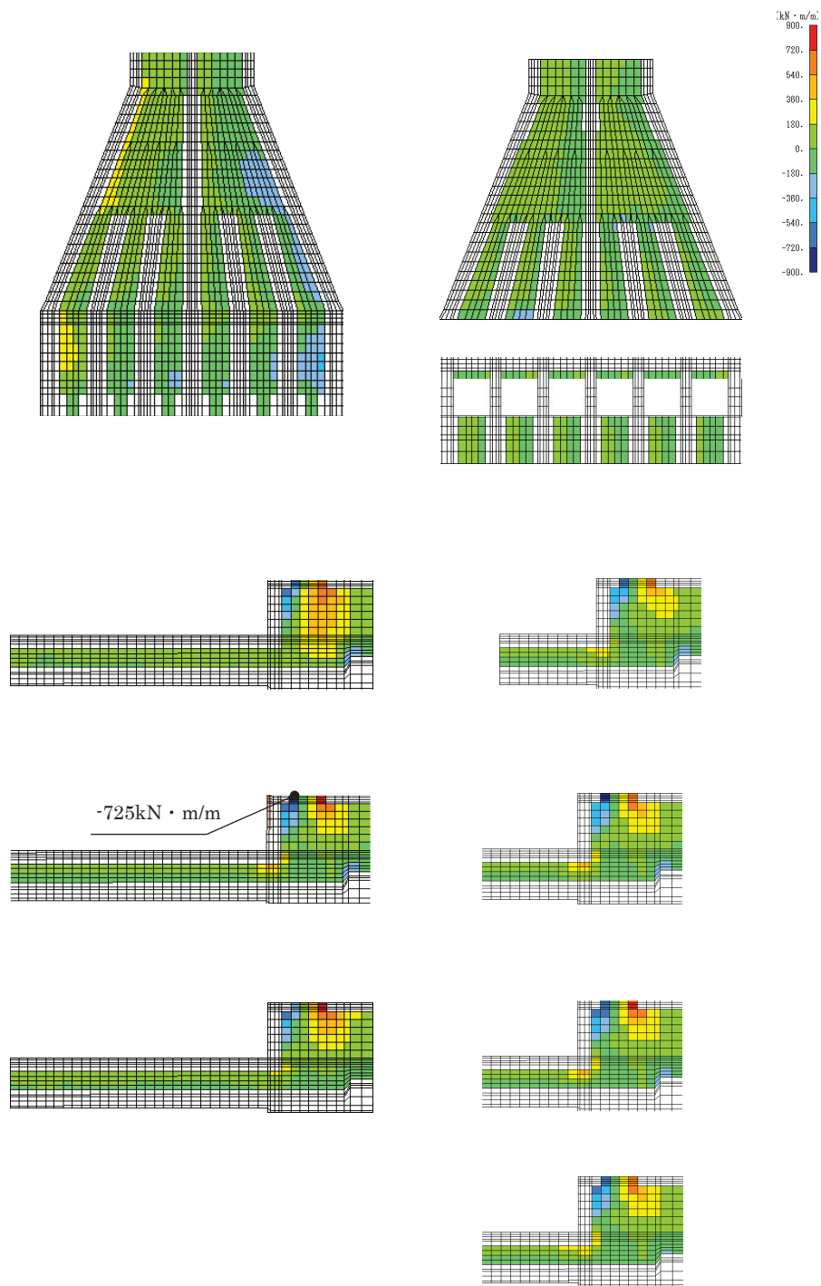
図 6-19 せん断破壊に対する照査値最大時の断面力分布図 (曲げモーメント (kN · m/m) : M_y ) (導流壁, 解析ケース①, 地震動 S_s - D2 (-+)) (標準部 t = 25.07s , 漸縮部 t = 25.06s )
