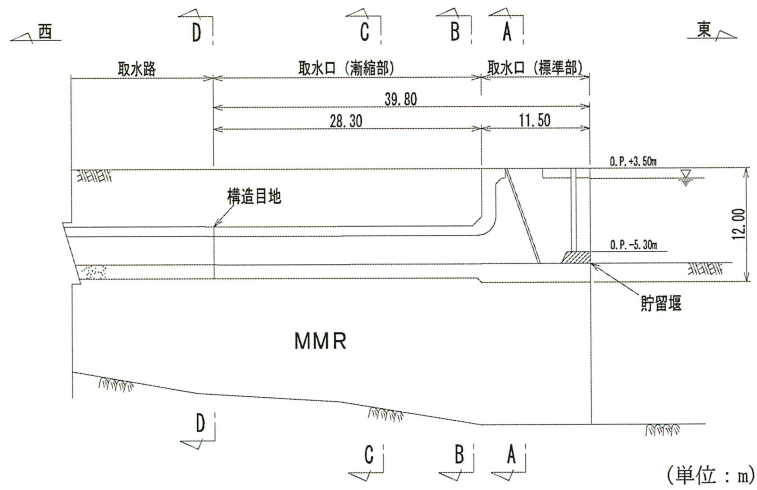
図 2-8 取水口断面図 (E-E 断面, 東西)
