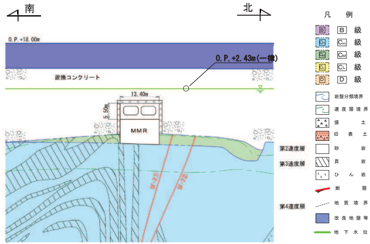
図 2-20 設計用地下水位 (断面④)
