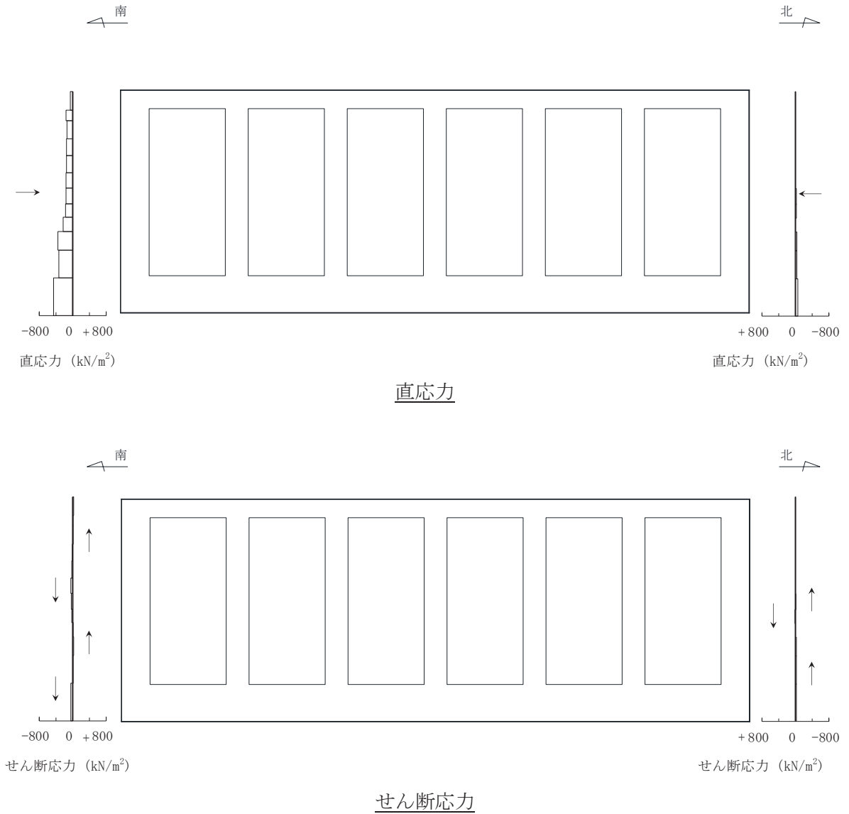
図6-1 作用荷重分布図（直応力及びせん断応力） (解析ケース①, S s - D 2 (一+), A-A断面 (標準部), t = 25.07s)
