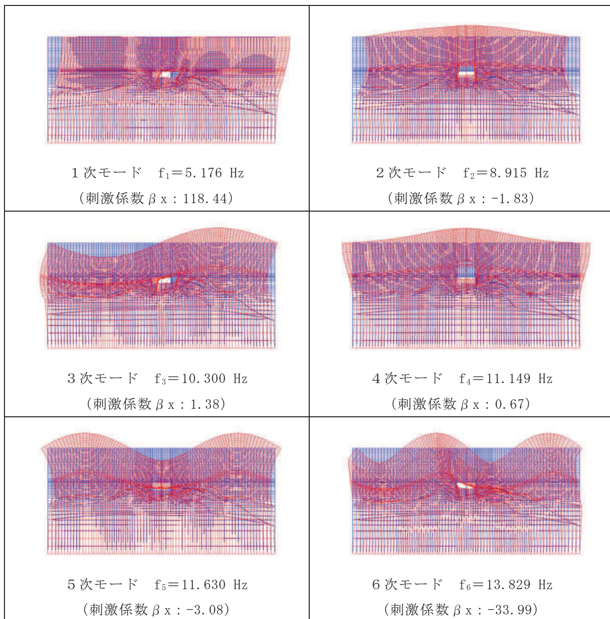
図 3-29(1) 固有値解析結果 (モード図) (断面⑤) (1/2)
