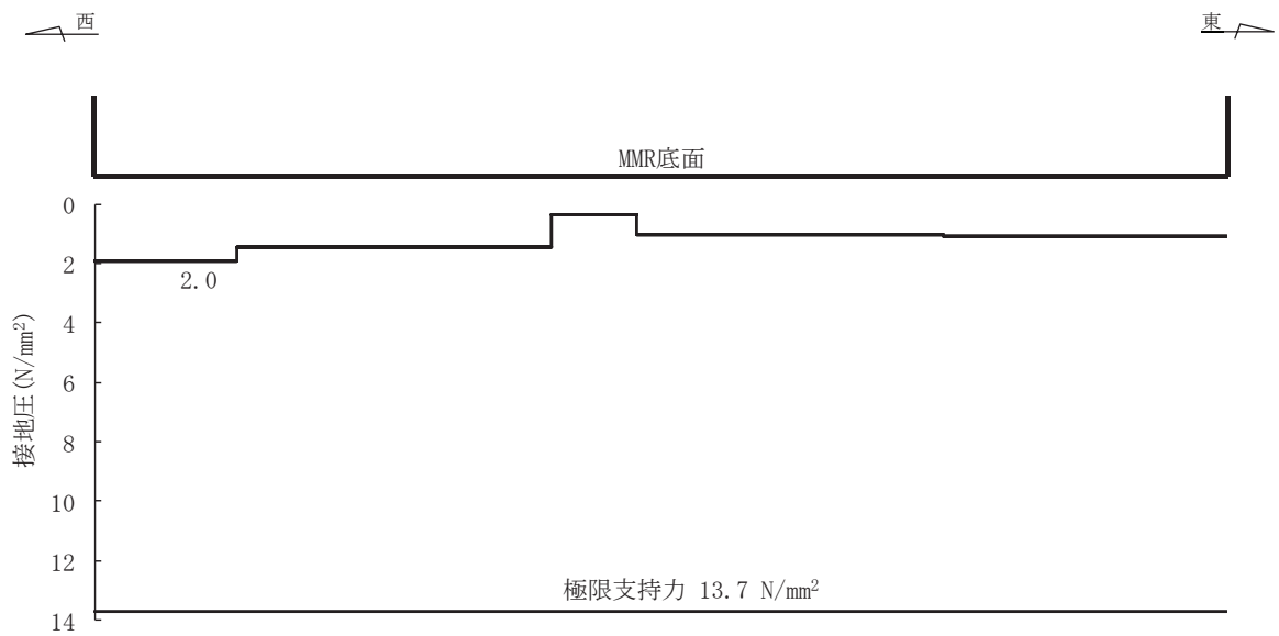
図 6-15 基礎地盤の最大接地圧分布図 (解析ケース①, S s - D 1 (++) )
