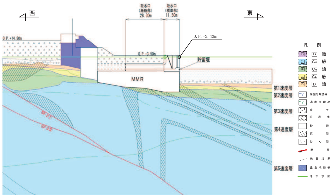
图 2-16 取水口，貯留堰 地震時荷重算出用地質断面図 (D-D 断面，東西)
