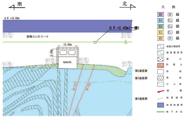
図 2-11 取水路（標準部） 地震時荷重算出用地質断面図（断面④）
