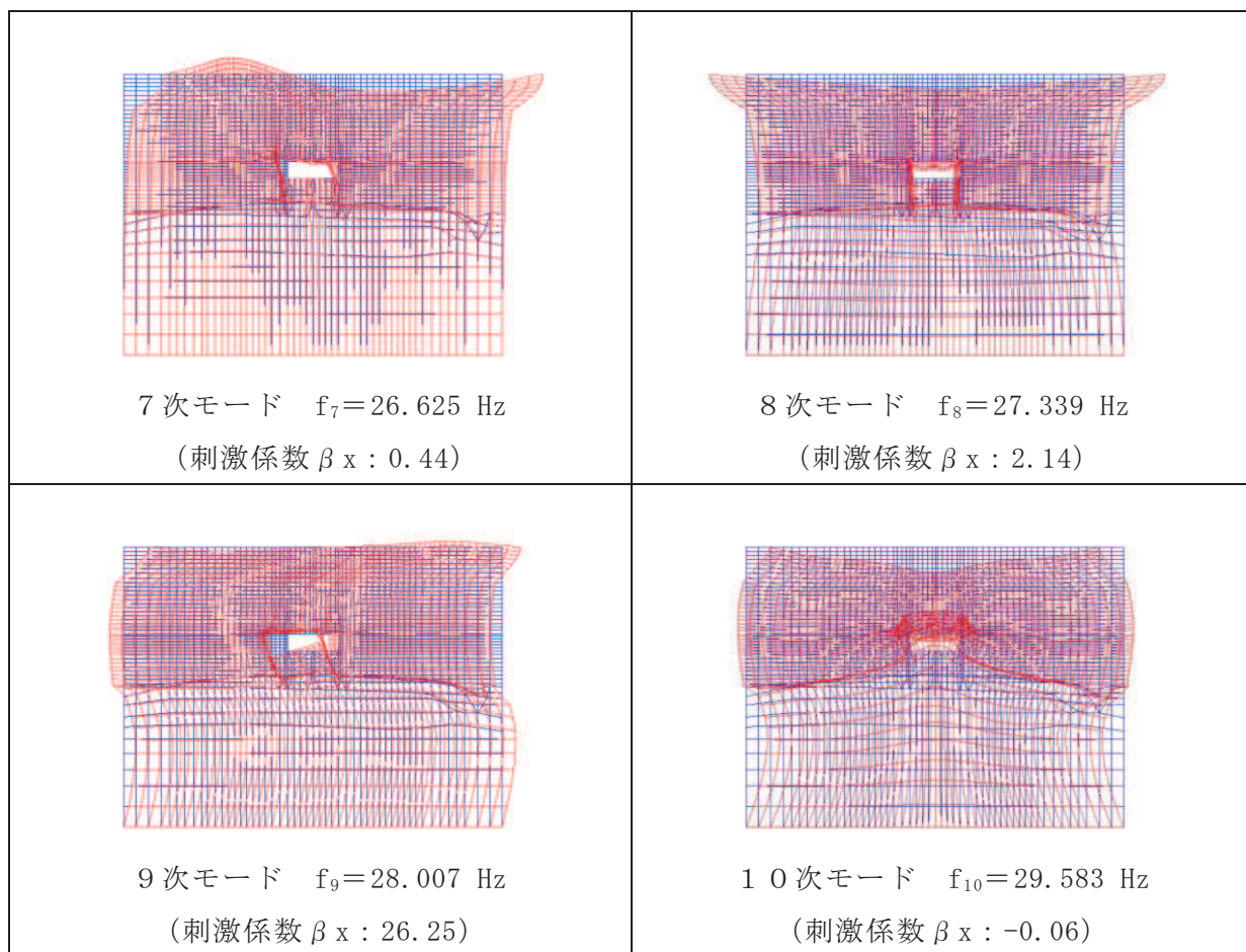
図 3-28(2) 固有値解析結果 (モード図) (断面④) (2/2)
