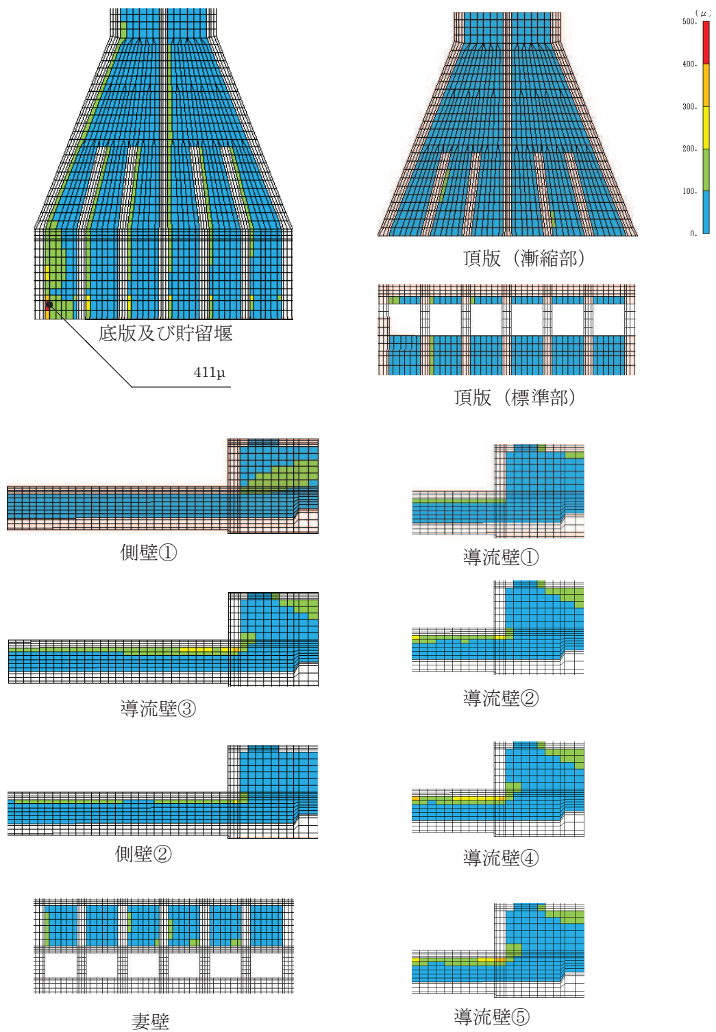
図 6-15 曲げ・軸力系の破壊に対する照査値最大時のひずみ分布図 (コンクリートの圧縮ひずみ) (貯留堰, 解析ケース③, 地震動 S_s - D2 (—+)) (標準部 t = 25.08s , 漸縮部 t = 25.06s )
