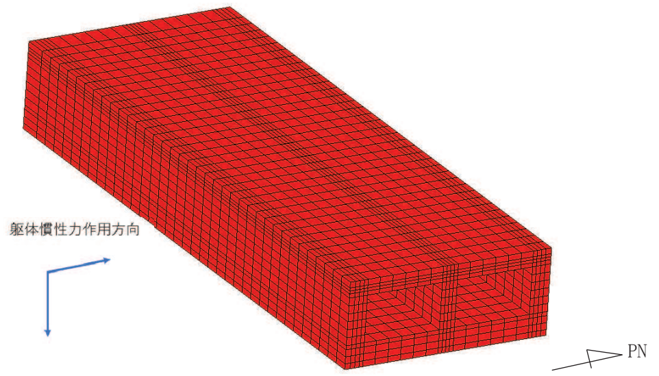
図 4-17 三次元構造解析モデルに入力する慣性力（躯体）の概念図
