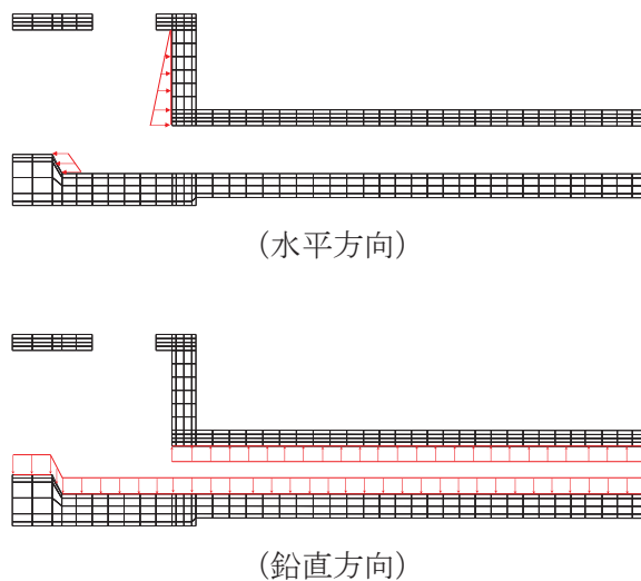
図 4-15 内水圧の概念図 (東西方向)
