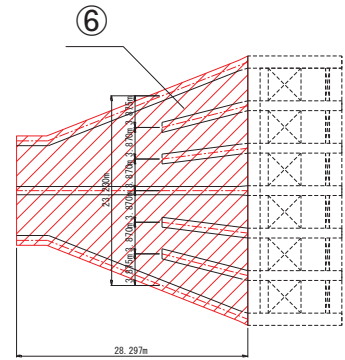
縦断面図
