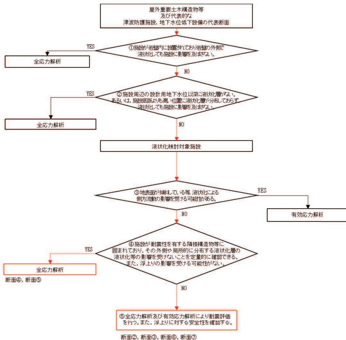
図 3-1 解析手法の選定フロー
