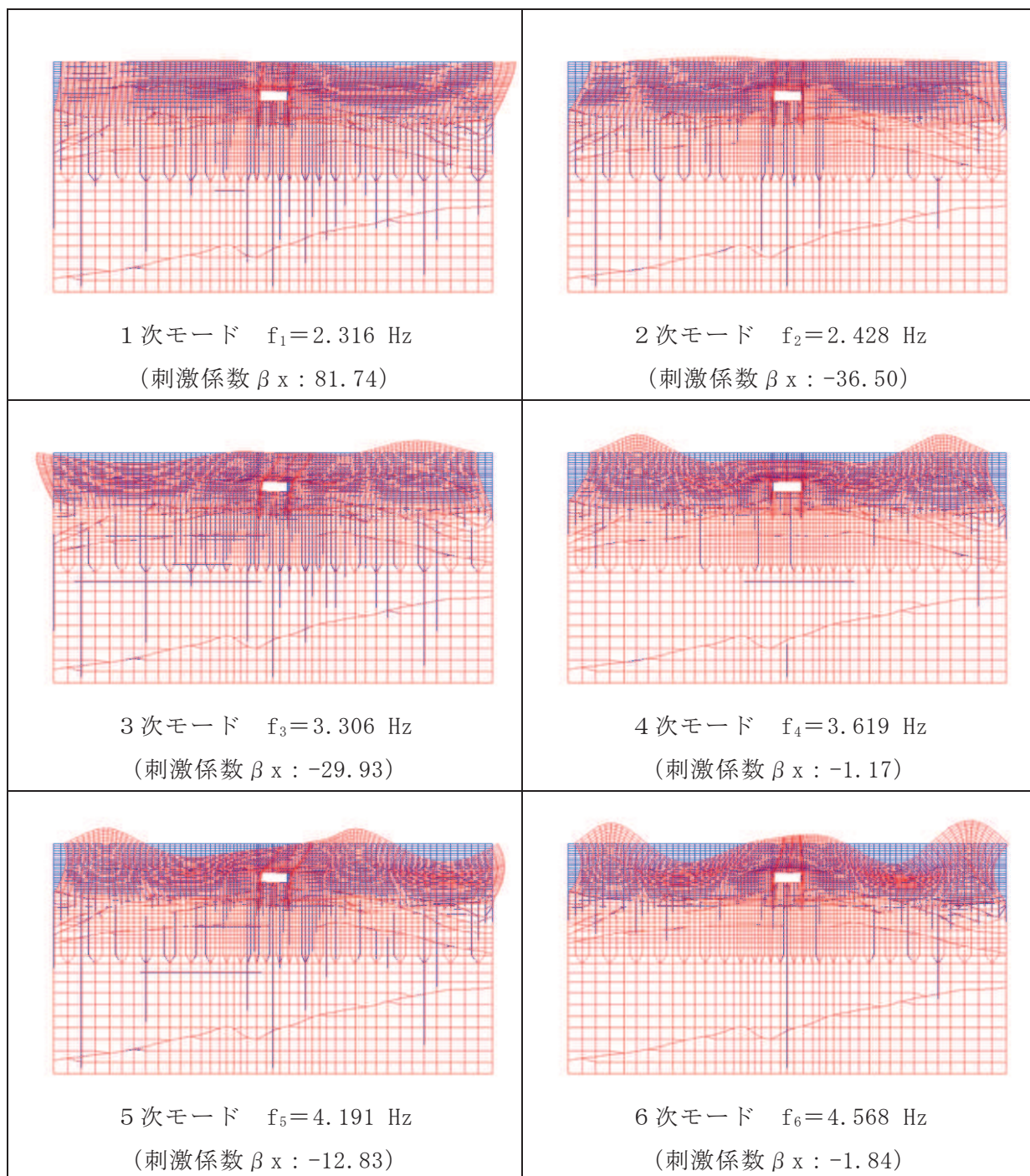
図 3-27(1) 固有値解析結果 (モード図) (断面③) (1/2)
