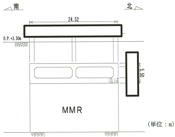
図 2-6 取水口断面図 (C-C 断面, 南北 (漸縮部))
