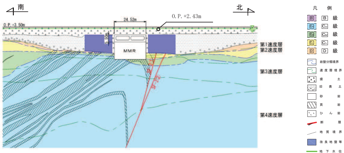
図 2-22 設計用地下水位（C-C 断面，漸縮部）
