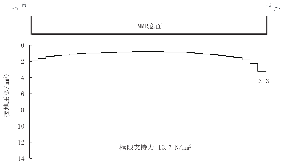
図 6-26 基礎地盤の最大接地圧分布図 (解析ケース①, S s -D 1 (++) , A-A 断面 (標準部))
