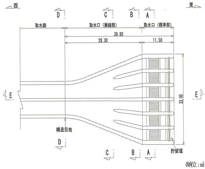
図 2-3 取水口平面図
