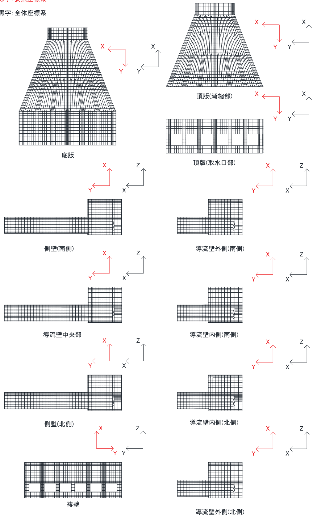
図 6-10 各部材の要素座標系
