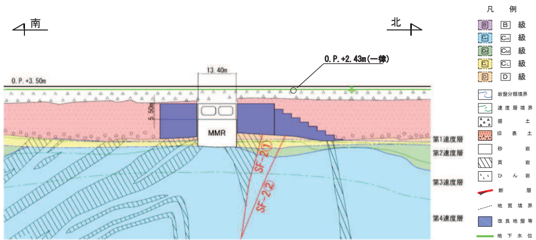
图 2-18 设计用地下水位 (断面②)
