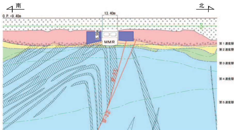
(a) 地震時荷重算出用地質断面図
