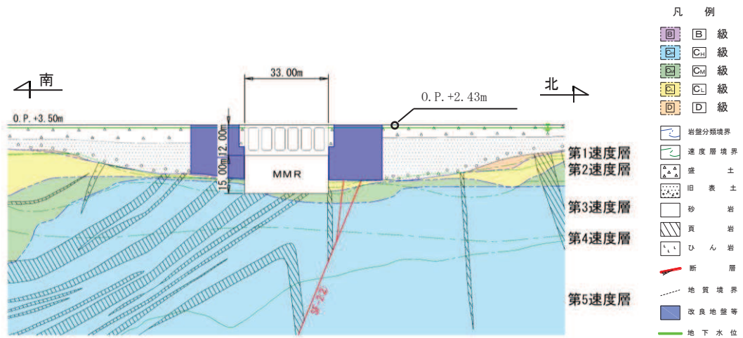
図 2-21 設計用地下水位（A-A 断面，標準部）
