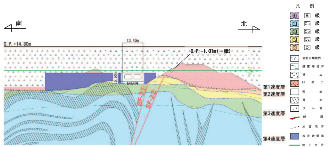
図 2-13 取水路（標準部） 地震時荷重算出用地質断面図（断面⑥）
