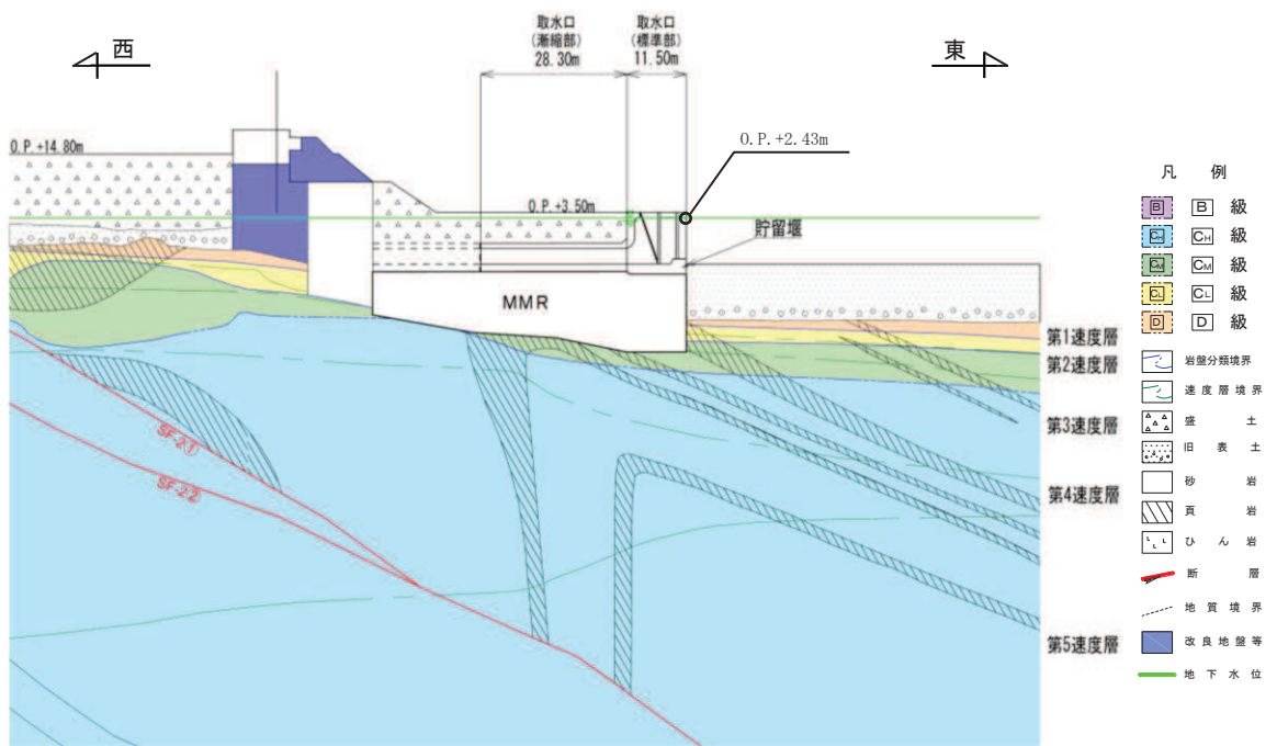
图 2-23 设计地下水位 (D-D 断面, 纵断)
