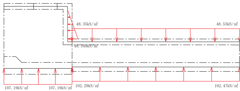
図3-28 外水圧図 (縦断)
