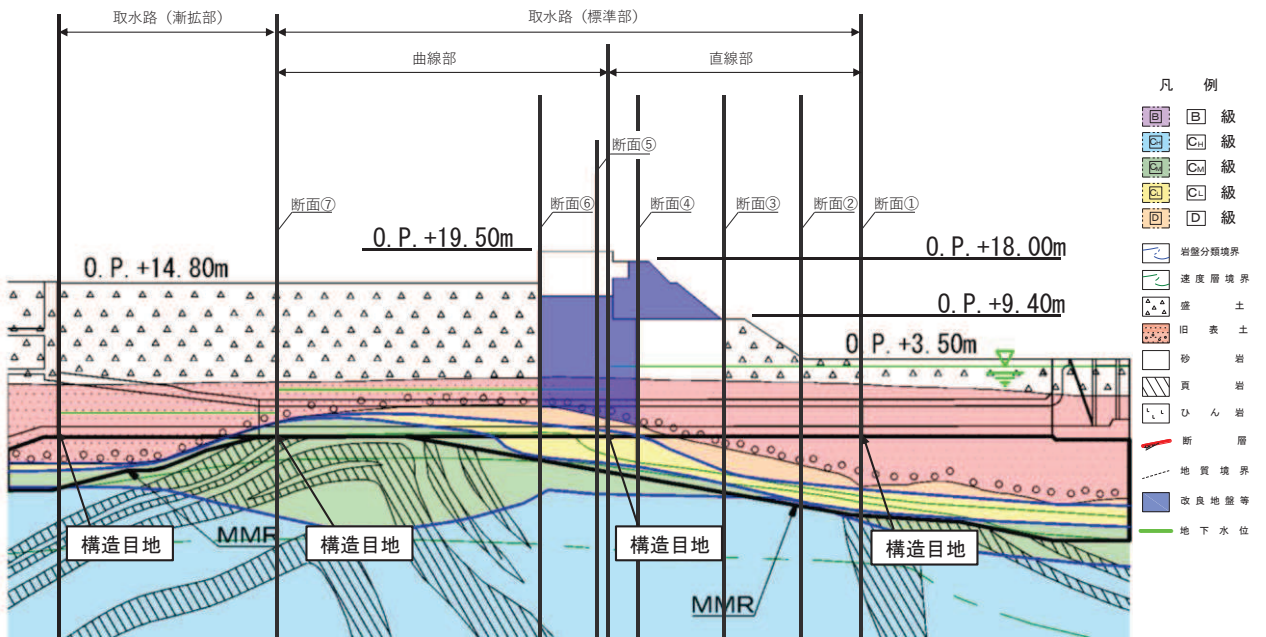
図 2-8 取水路 (標準部) の地震時荷重算出断面位置図
