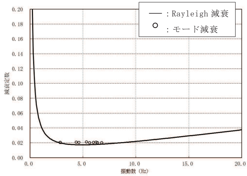
図 3-30 設定した Rayleigh 減衰 (断面②)
