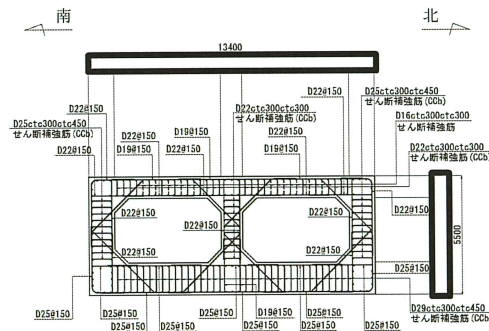
図 2-12 取水口概略配筋図（D-D 断面，南北（漸縮部））
