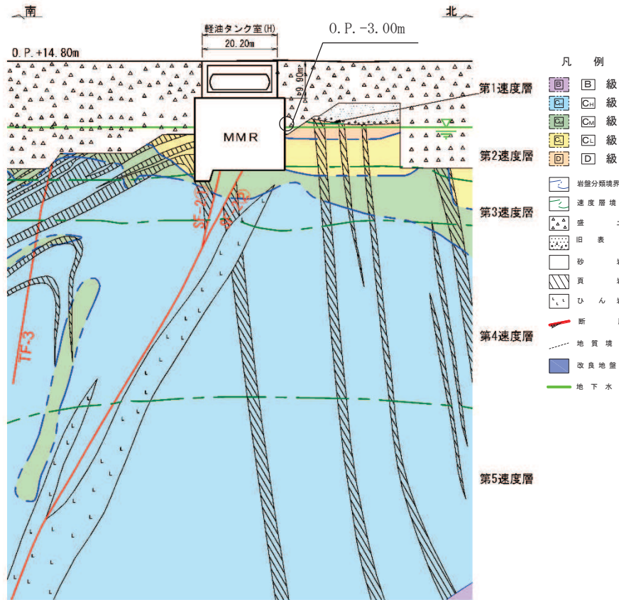
図3-2 軽油タンク室 (H) 地震時荷重算出用地質断面図 (A-A 断面, 南北)
