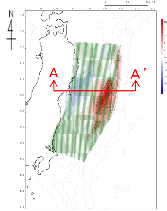
地殻変動量分布 (合計)
