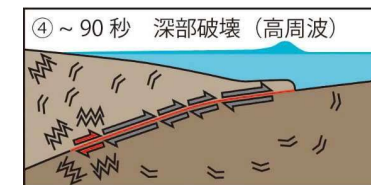
時間毎の破壊過程の模式図 井出 (2011) (25)
