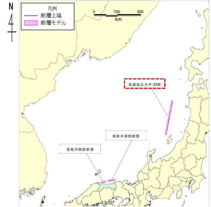
想定地震位置図 鳥取県 (2012) (10) に一部加筆
