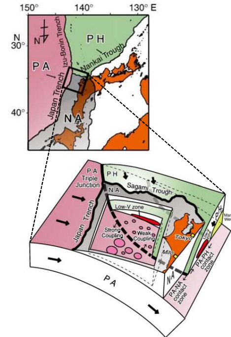
太平洋プレート上面のプレート間カップリング模式図 Uchida et al. (2009) (33)
