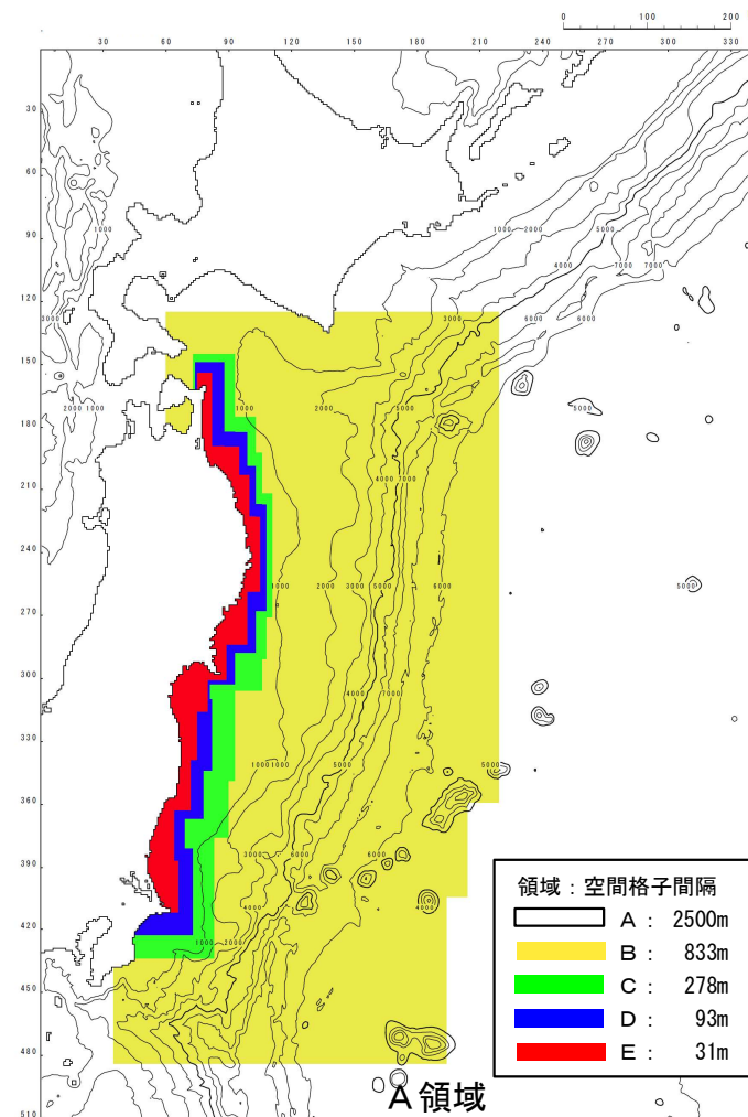
計算領域とその水深及び格子分割
