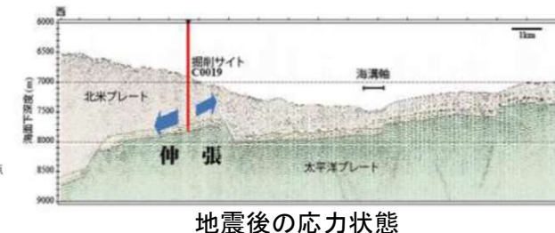
2011年東北地方太平洋沖地震震源域の応力状態変化模式図 JAMSTEC (2013) (18)
