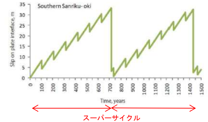
宮城県沖及び三陸沖南部における地震発生サイクルのモデル 佐竹 (2011) (19) に一部加筆
