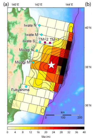
藤井・佐竹55枚モデル
