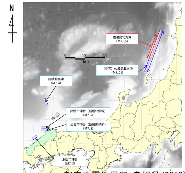
想定地震位置図 島根県 (2012) (11)
