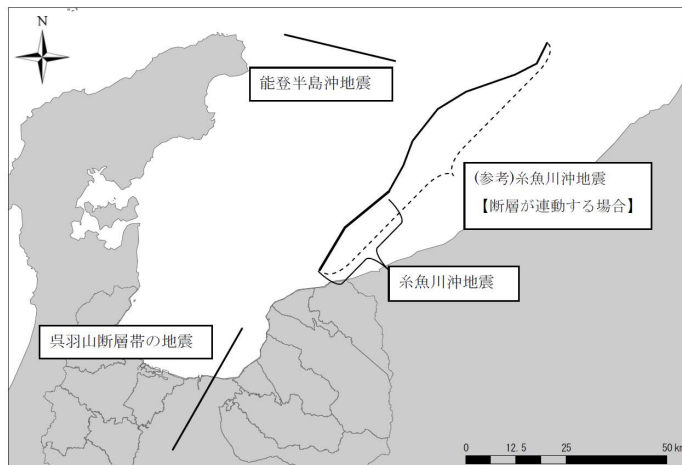
想定地震位置図 富山県(2012) (7)
