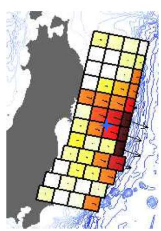
JNESモデル (杉野ほか (2013) (36))
