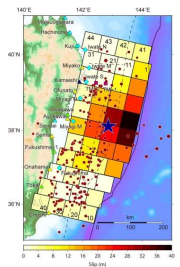
藤井・佐竹44枚モデル
