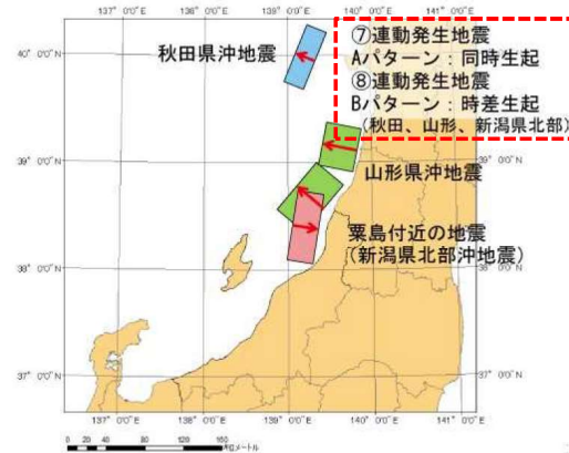
新潟県(2016) (6) に一部加筆
