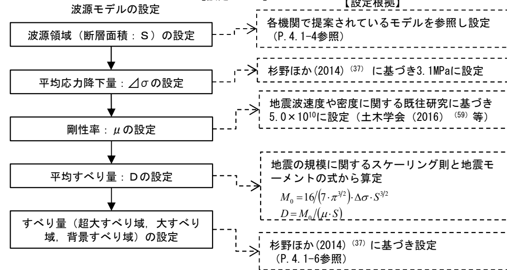
3. 11地震における広域の津波特性を考慮した特性化モデルのパラメータ
