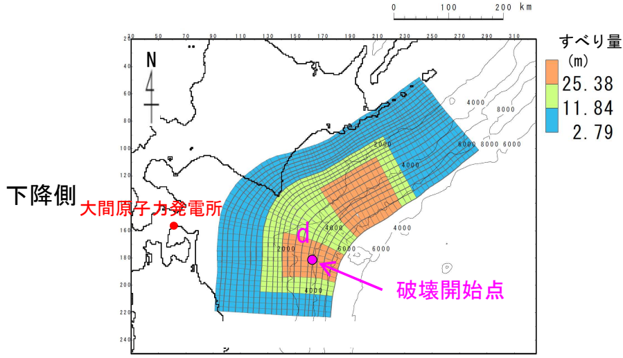
最大ケース波源モデル (基準波源モデル①-1)
