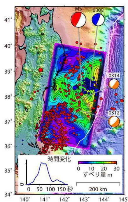
(左図) コンター: 総すべり量の分布, 0309: 前震 (Mw7.3) のメカニズム, MS: 本震のメカニズム, 0312及び0314: 余震 (それぞれMw6.5, Mw6.1) のメカニズム, 青点: 前震の震央, 赤点: 余震の震央, グラフ: 地震モーメントの放出速度の推移
