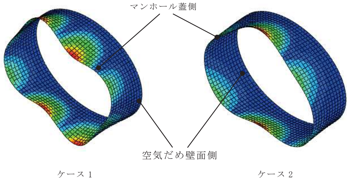
図 4-1 座屈モード
