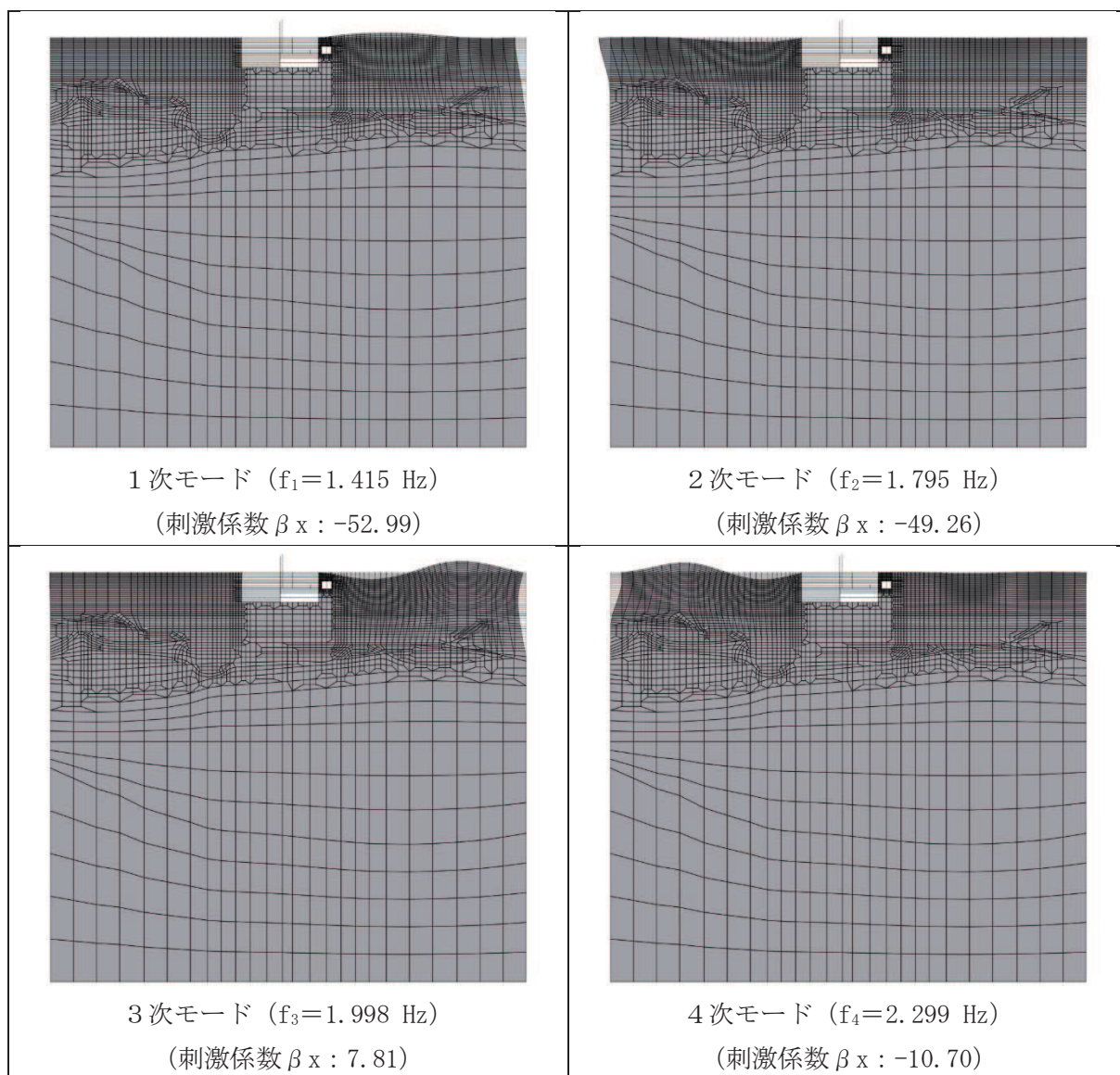
図 3-14(1) 固有値解析結果 (モード図) (1/3)
