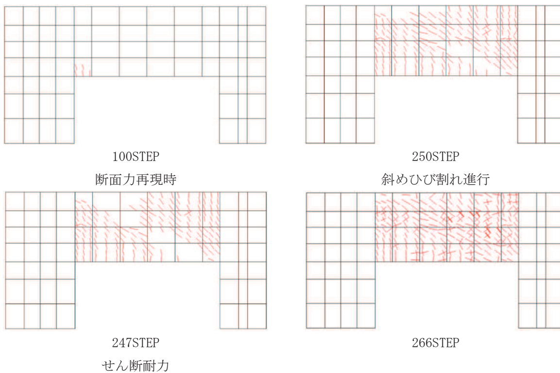
図 5-18 各ステップにおけるひび割れ図 (頂版, 解析ケース③, S_s - D3 (++) )
