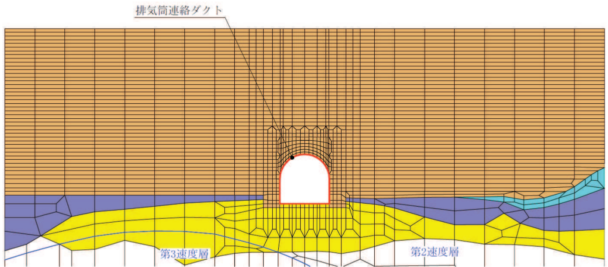
図 3-10(1) ジョイント要素の配置 (断面①)
