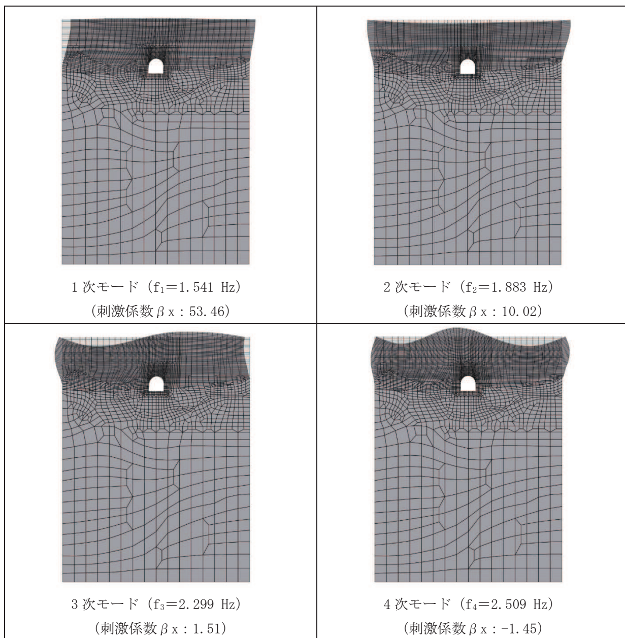
図 3-18(4) 固有値解析結果 (モード図) (断面③) (1/3)
