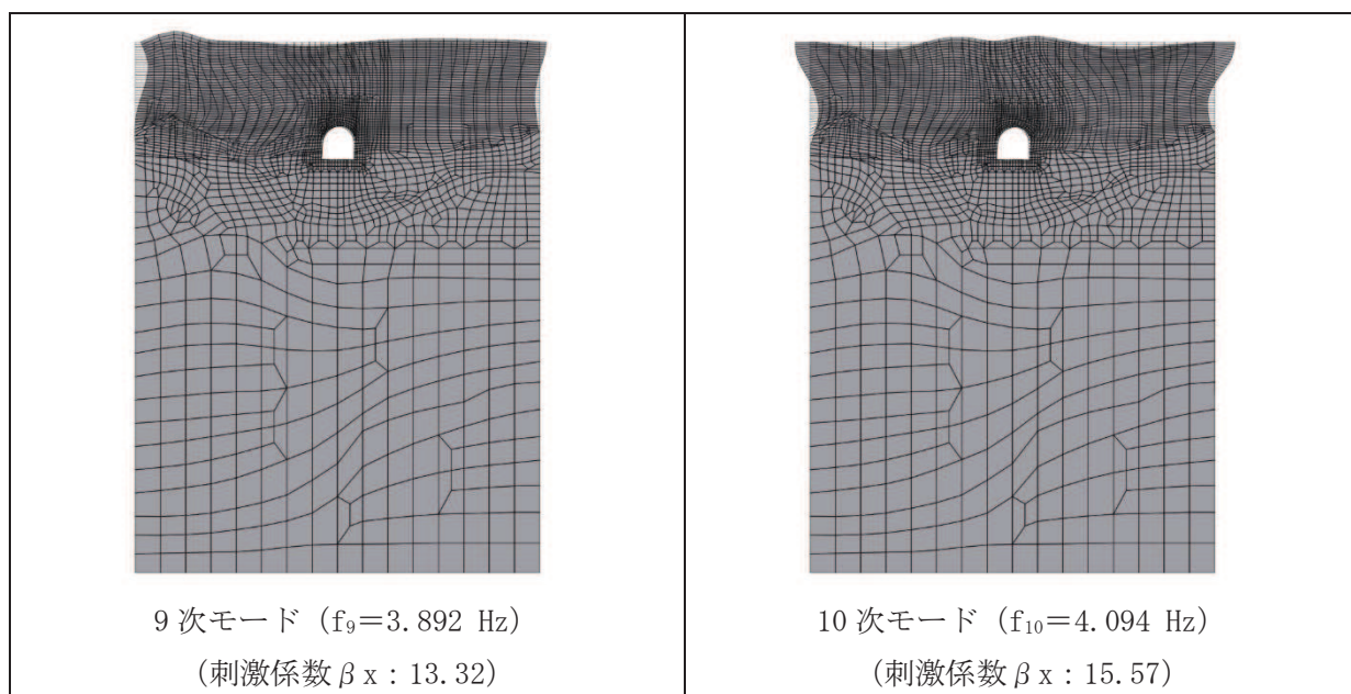
図 3-18(6) 固有値解析結果 (モード図) (断面③) (3/3)
