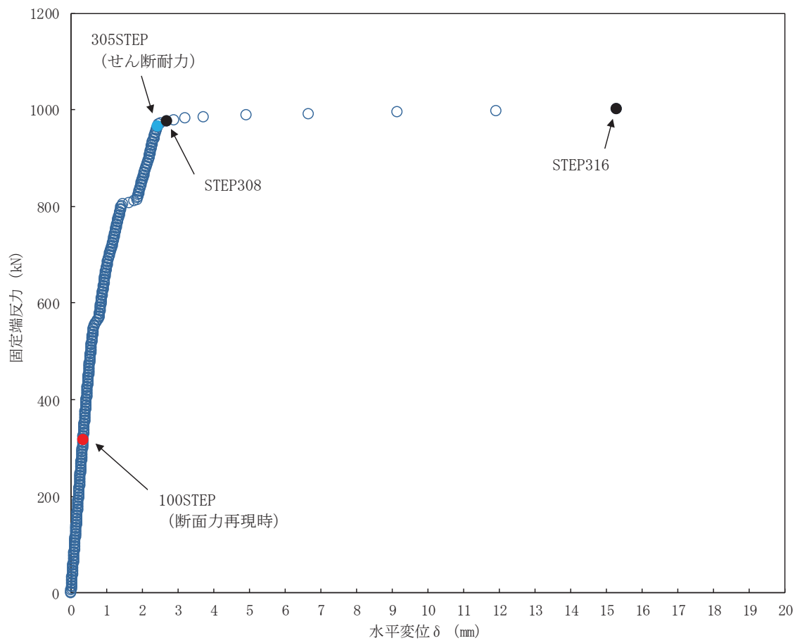
図 5-20 荷重-変位曲線 (側壁, 解析ケース②, S_s - D_2 (-+) )
