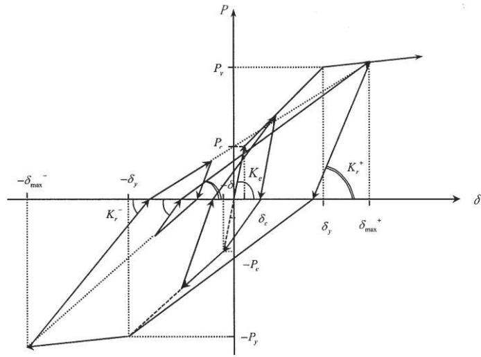
図 3-14 M-φ モデルに用いる鉄筋コンクリート部材の履歴特性（修正武田モデル） （道路橋示方書（V耐震設計編）・同解説（平成 14 年 3 月）より引用）
