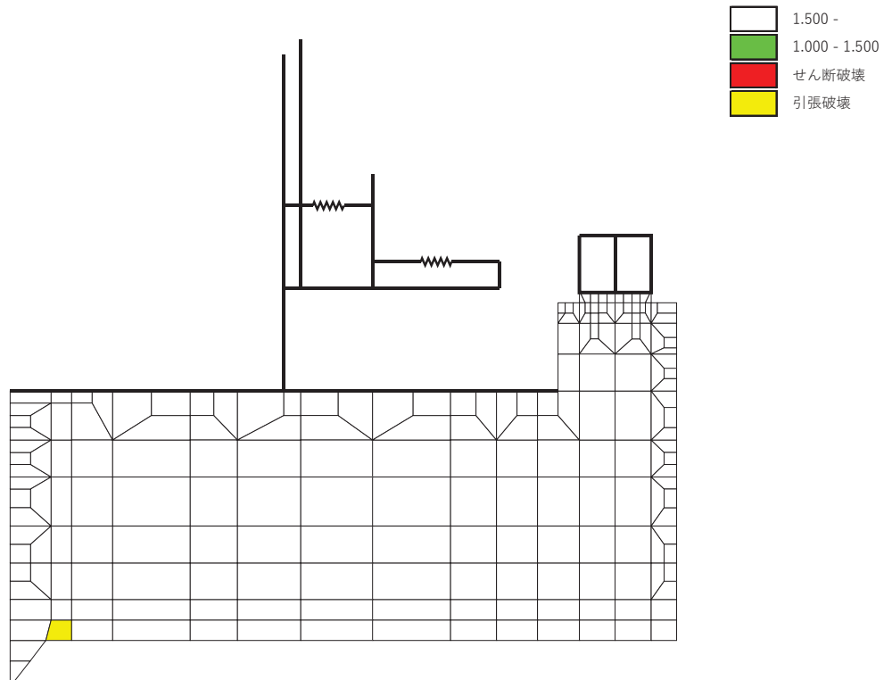
図 5-30(1) MMR (既設) の引張応力最大時刻の局所安全係数 (解析ケース① : 基本ケース, S_s - D 1 (-+) , t=25.22s )
