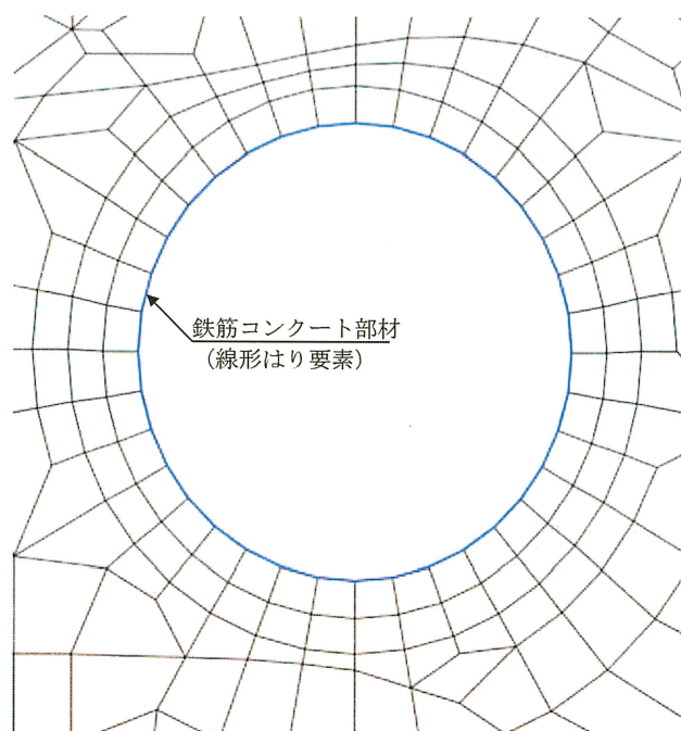
図3-8(2) 排気筒連絡ダクトの地震応答解析モデル（構造物部分拡大，岩盤部）
