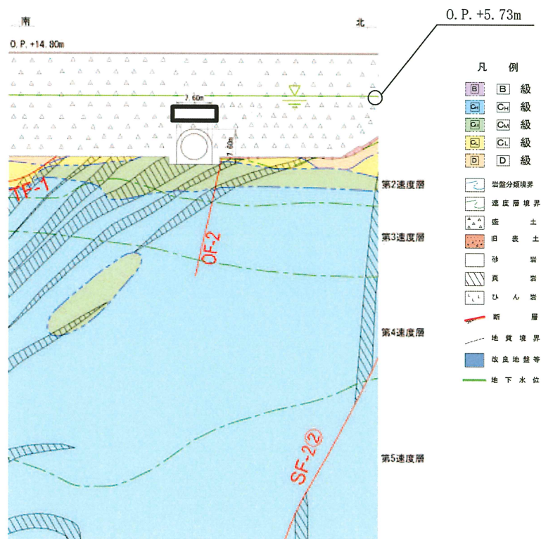
図 2-5(2) 排気筒連絡ダクト 評価対象地質断面図 (断面①)
