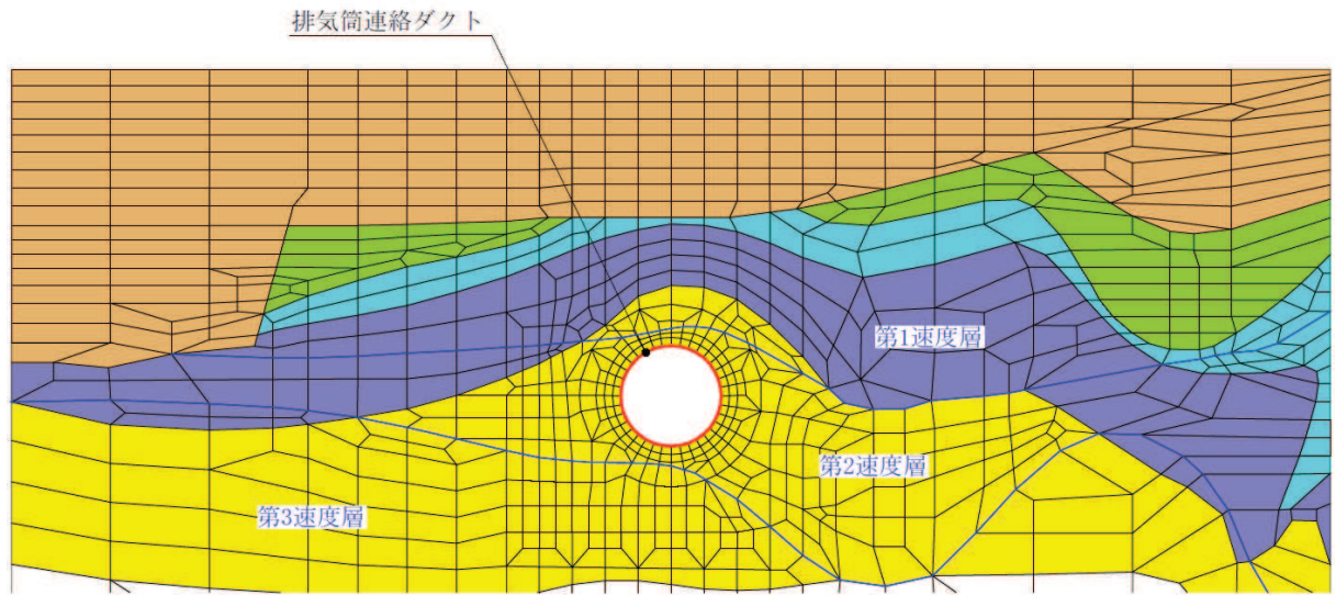
図 3-10(3) ジョイント要素の配置 (断面⑤)
