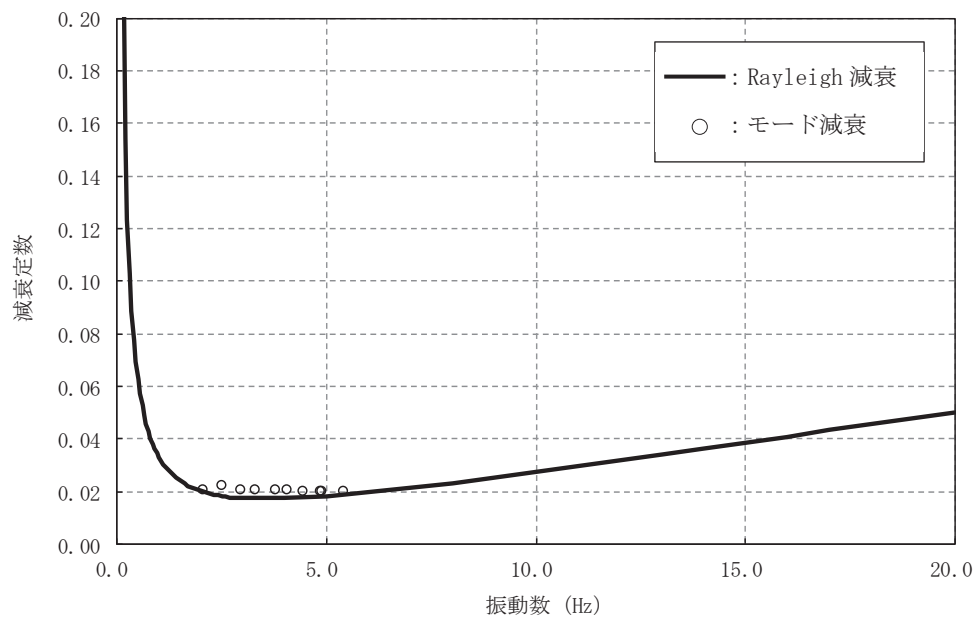
図 3-19(3) 設定した Rayleigh 減衰 (断面⑤)
