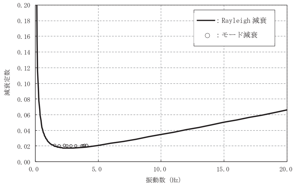
図 3-19(2) 設定した Rayleigh 減衰 (断面③)
