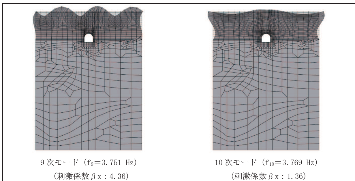
図 3-18(3) 固有値解析結果 (モード図) (断面①) (3/3)
