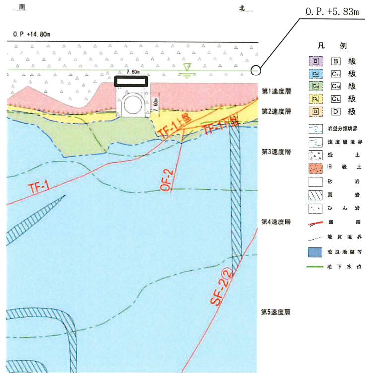
図 2-9 排気筒連絡ダクトの設計用地下水位 (断面③)
