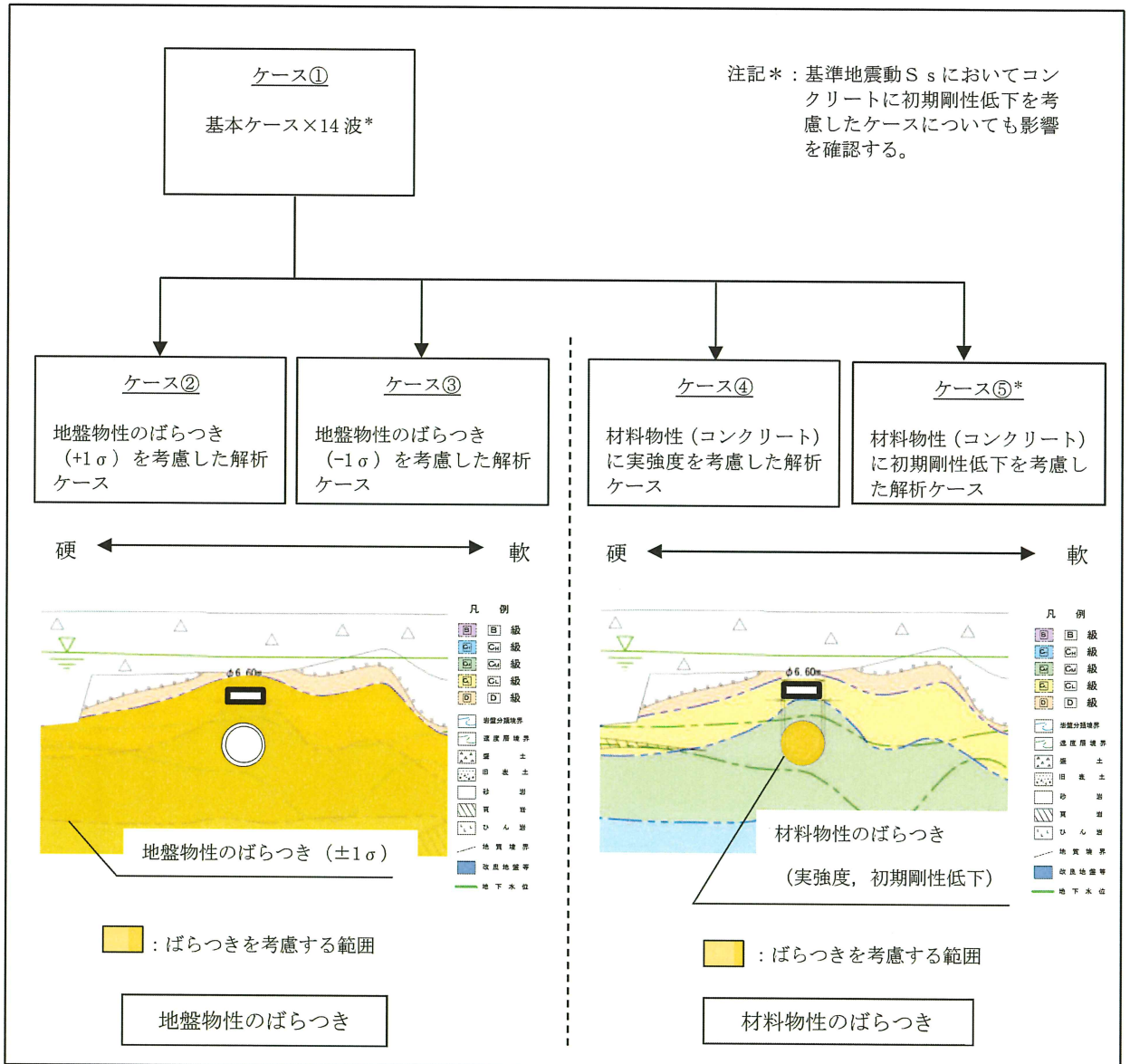
図 3-25(2) 機器・配管系の耐震評価に適用する解析ケース (岩盤部)
