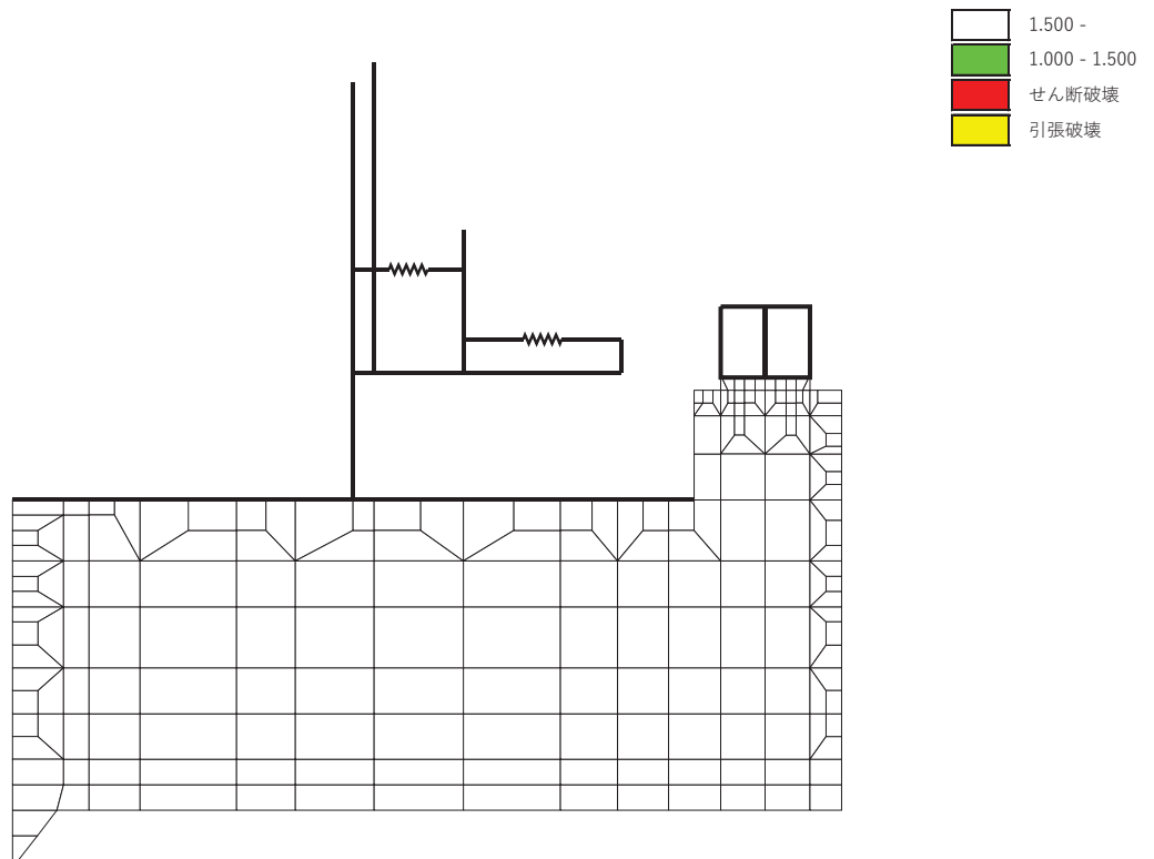
図 5-29(1) MMR (既設) のせん断応力最大時刻の局所安全係数 (解析ケース①: 基本ケース, S_s - D 1 (-+) , t=37.19s )
