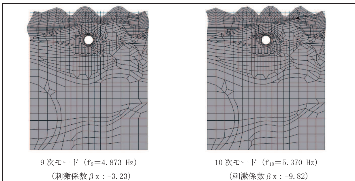
図 3-18(9) 固有値解析結果 (モード図) (断面⑤) (3/3)
