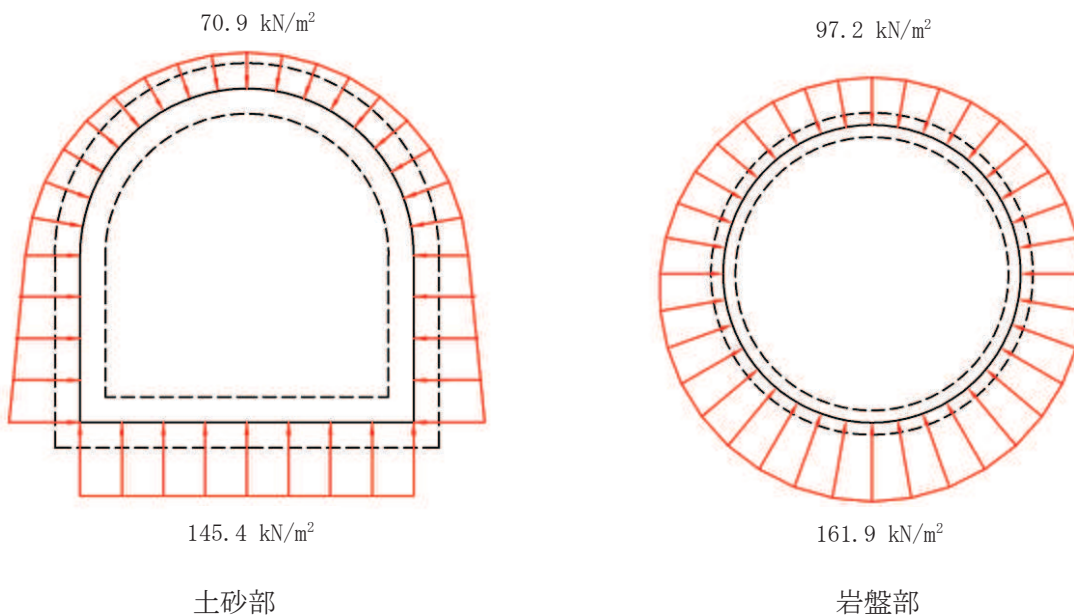
図3-21 外水圧図
