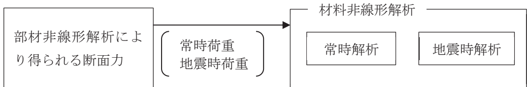
図 5-16 荷重の作用手順
