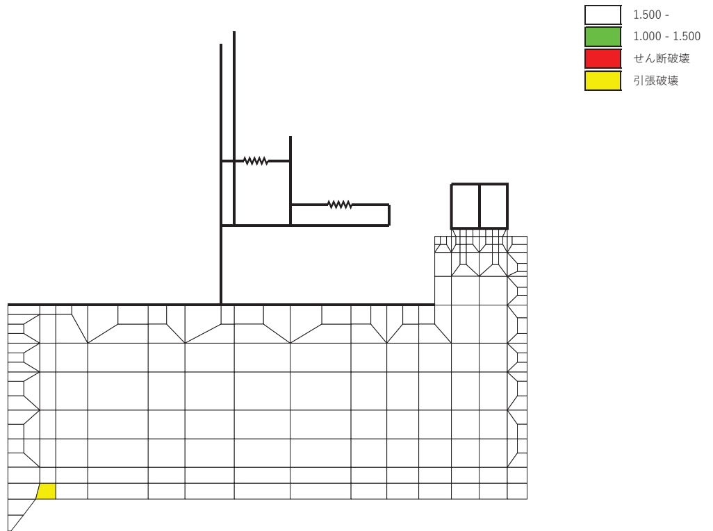
図 5-30(1) MMR (既設) の引張応力最大時刻の局所安全係数 (解析ケース① : 基本ケース, S_s - D 1 (-+) , t=25.22s )
