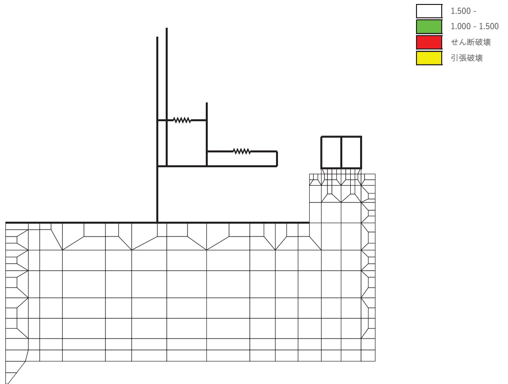
図 5-29(3) MMR (既設) のせん断応力最大時刻の局所安全係数 (解析ケース①: 基本ケース, S_s - N_1 (-+) , t=7.55s )
