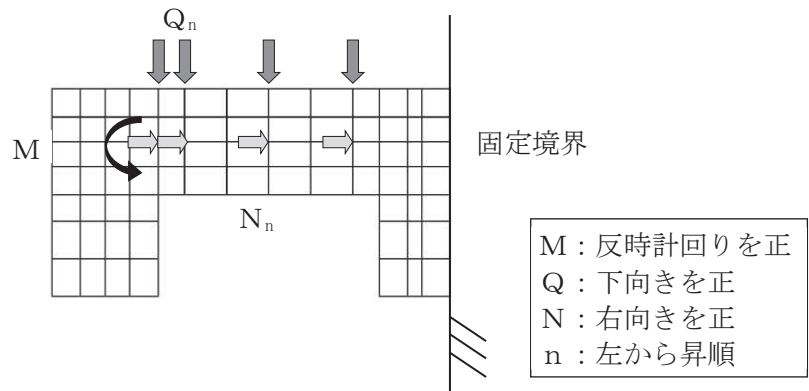
図 5-13 材料非線形解析における載荷状況（頂版）
