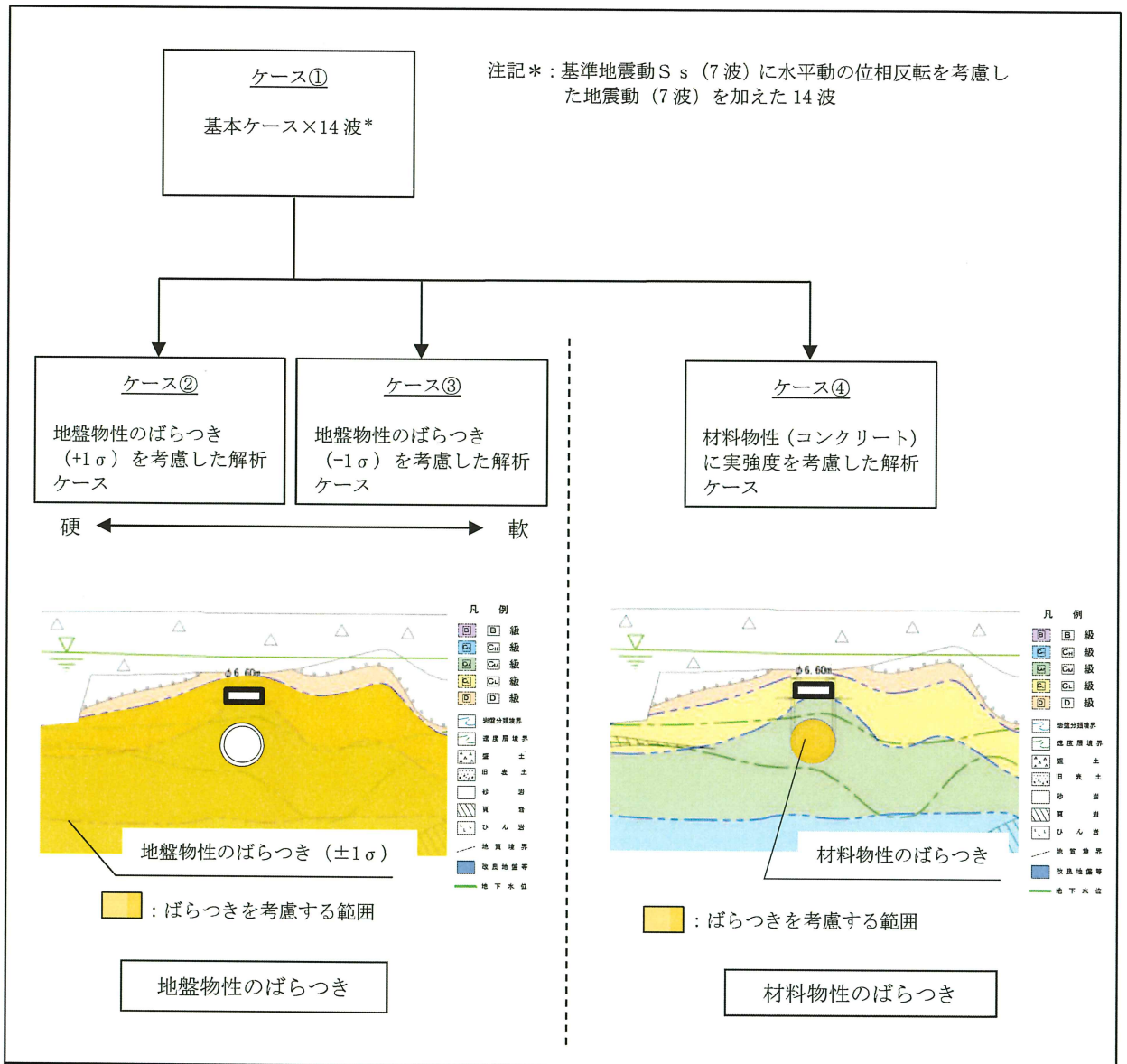
図 3-23(2) 耐震評価における解析ケース (岩盤部)
