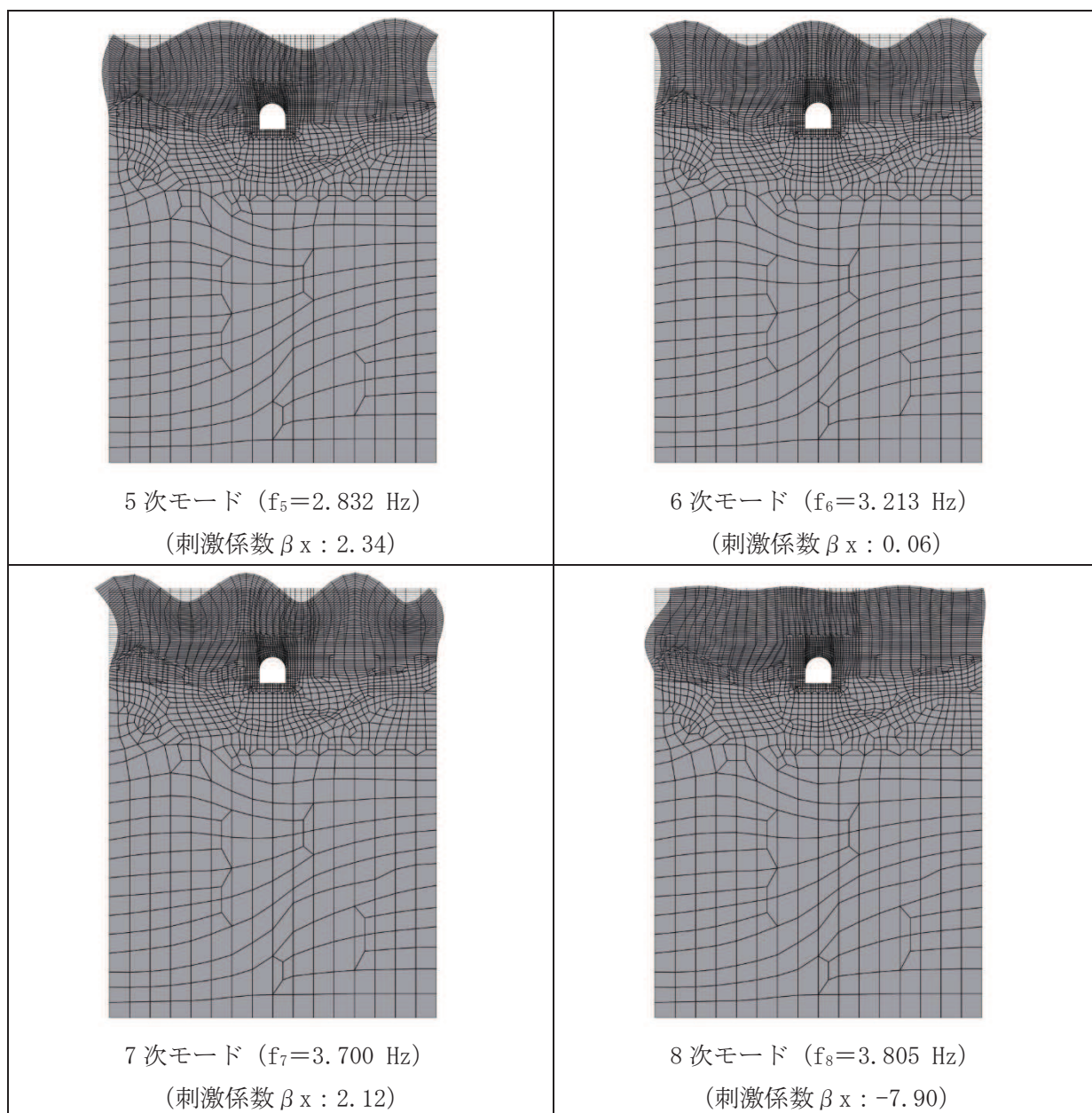
図 3-18(5) 固有値解析結果 (モード図) (断面③) (2/3)
