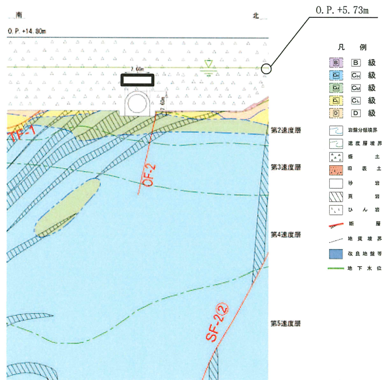
図 2-8 排気筒連絡ダクトの設計用地下水位 (断面①)
