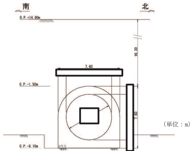
図 2-3(1) 排気筒連絡ダクト断面図 (A-A 断面, 土砂部)
