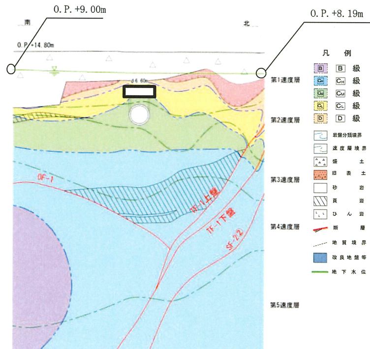
図 2-10 排気筒連絡ダクトの設計用地下水位 (断面⑤)
