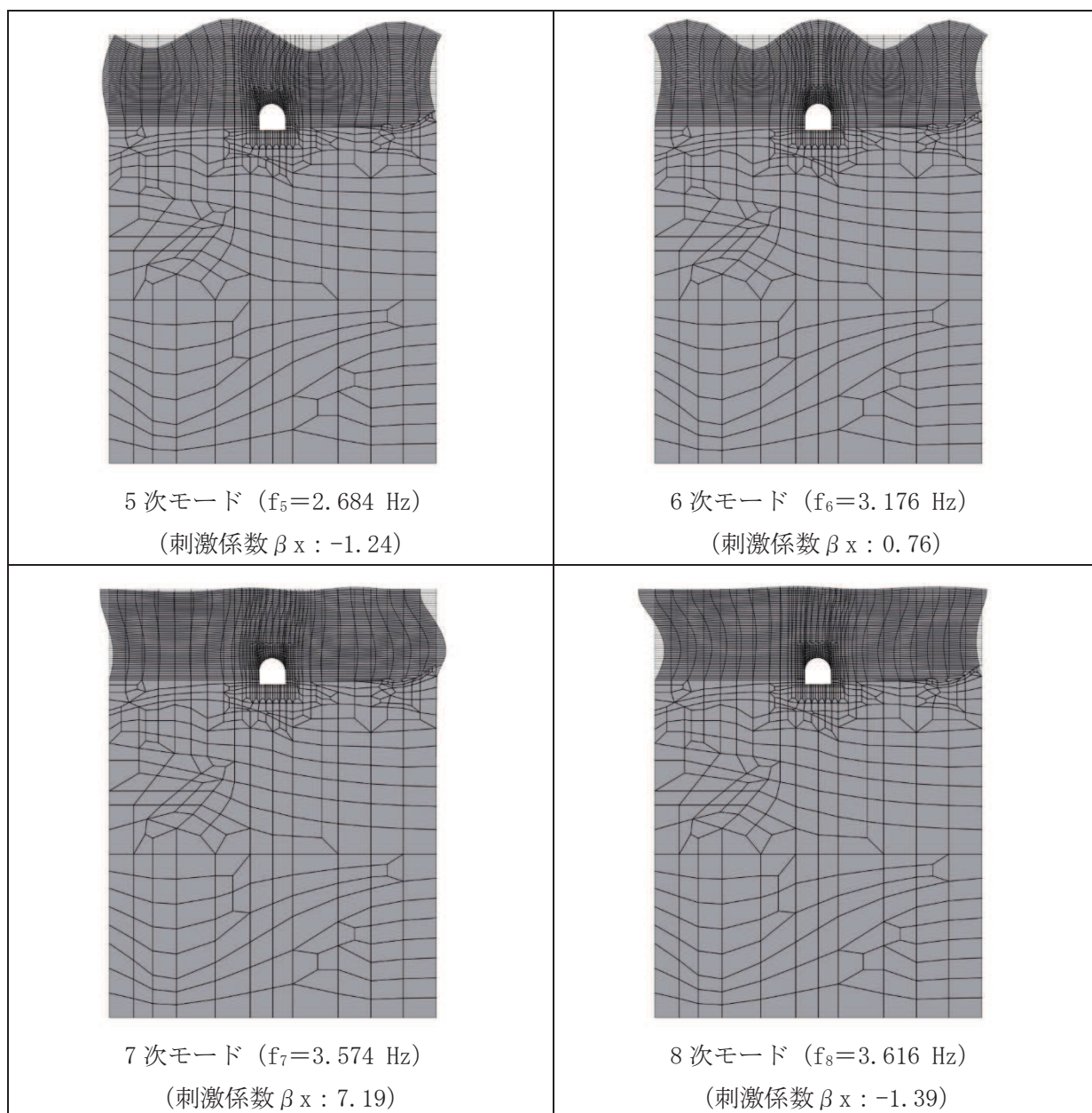
図 3-18(2) 固有値解析結果 (モード図) (断面①) (2/3)
