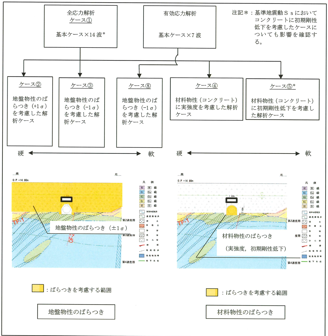
図 3-25(1) 機器・配管系の耐震評価に適用する解析ケース (土砂部)
