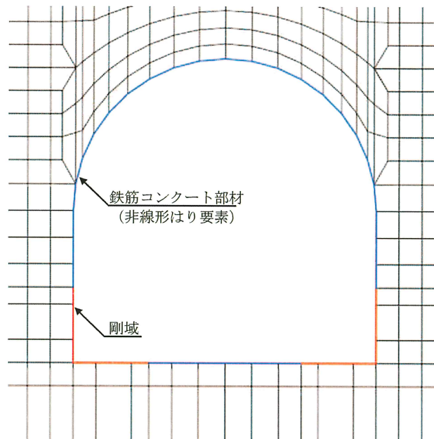
図3-8(1) 排気筒連絡ダクトの地震応答解析モデル（構造物部分拡大，土砂部）
