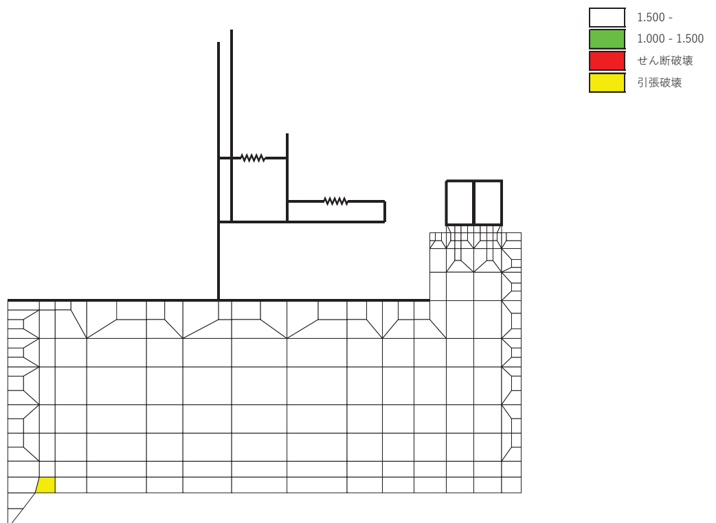
図 5-30(3) MMR (既設) の引張応力最大時刻の局所安全係数 (解析ケース①: 基本ケース, S_s - N_1 (-+) , t=7.36s )
