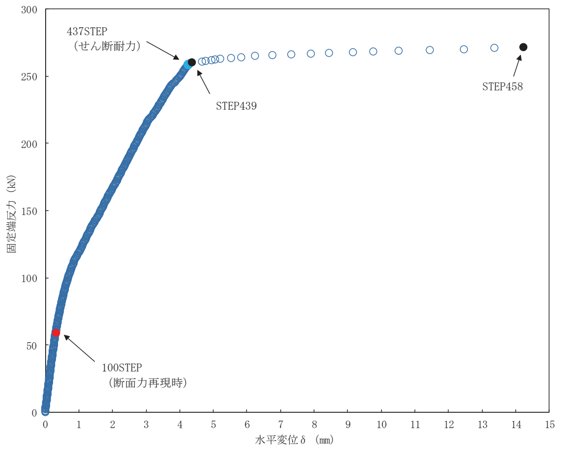
図 5-23 荷重-変位曲線 (隔壁, 解析ケース①, S s -D2 (++) )
