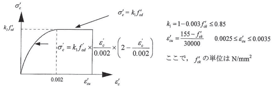
図 3-15 構造部材の非線形特性（M-φ モデルに用いるコンクリートの応力-ひずみ関係） （コンクリート標準示方書より引用）
