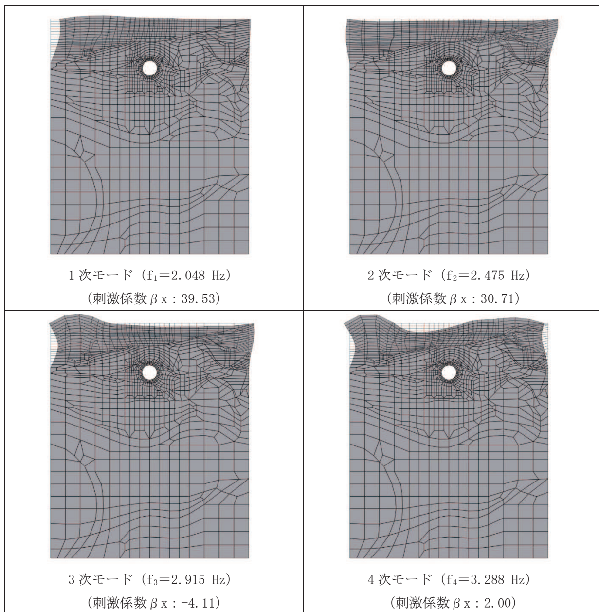
図 3-18(7) 固有値解析結果 (モード図) (断面⑤) (1/3)
