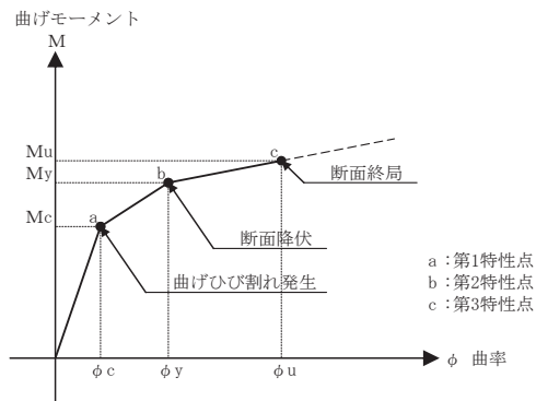
図 3-13 鉄筋コンクリート部材のM-φ関係 (土木学会マニュアルより引用)
