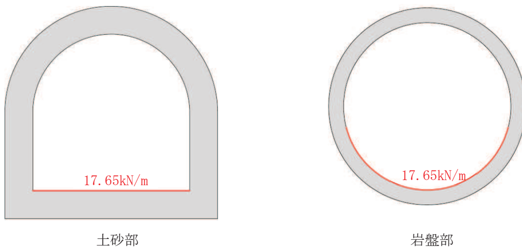
図3-20 機器・配管系の荷重図
