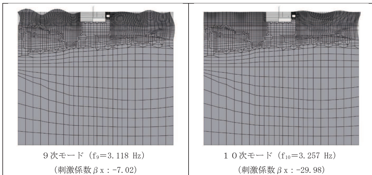
図 3-14(3) 固有値解析結果 (モード図) (3/3)
