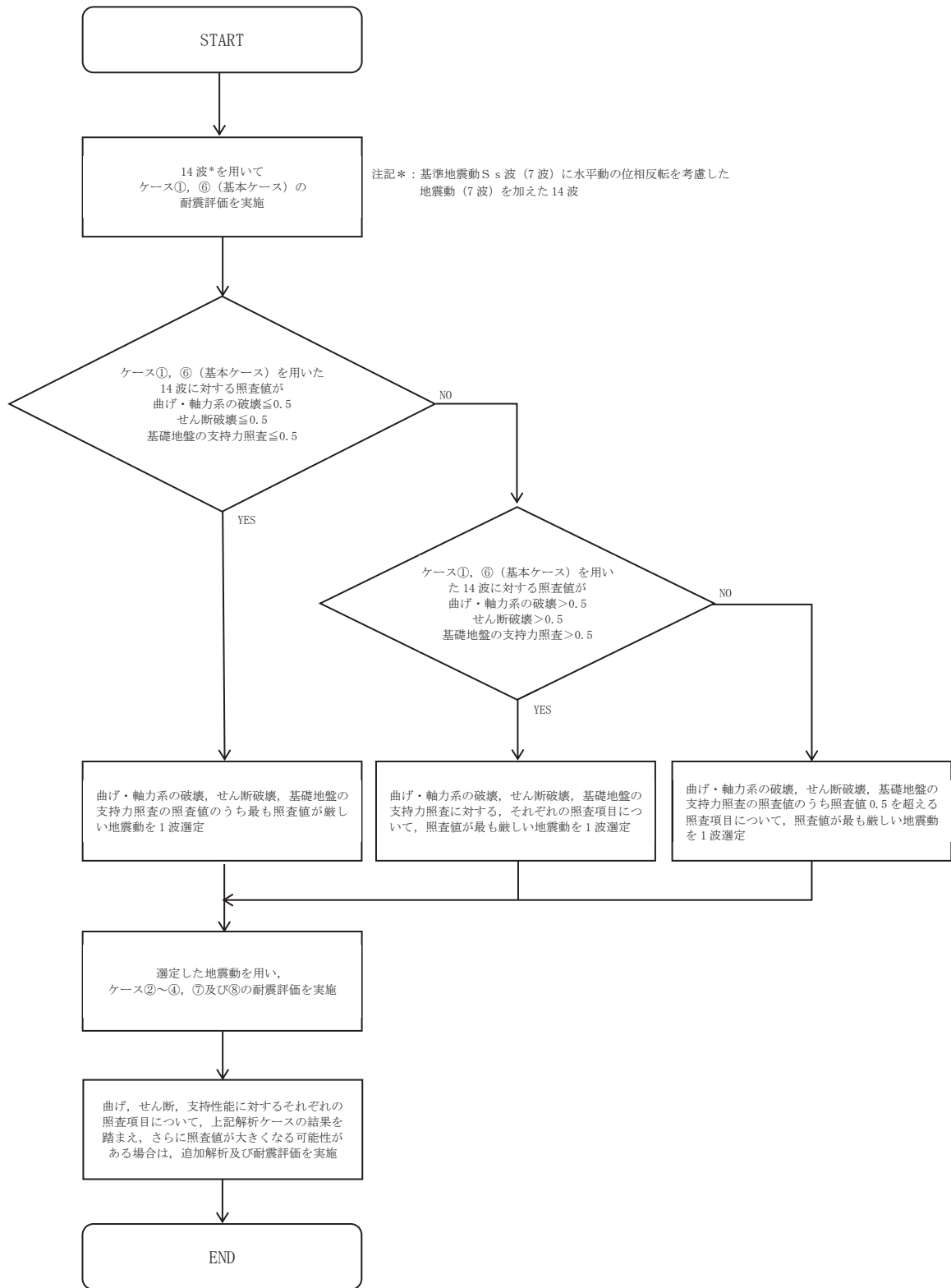
図 3-24(1) 追加解析を実施する地震動の選定フロー（土砂部）
