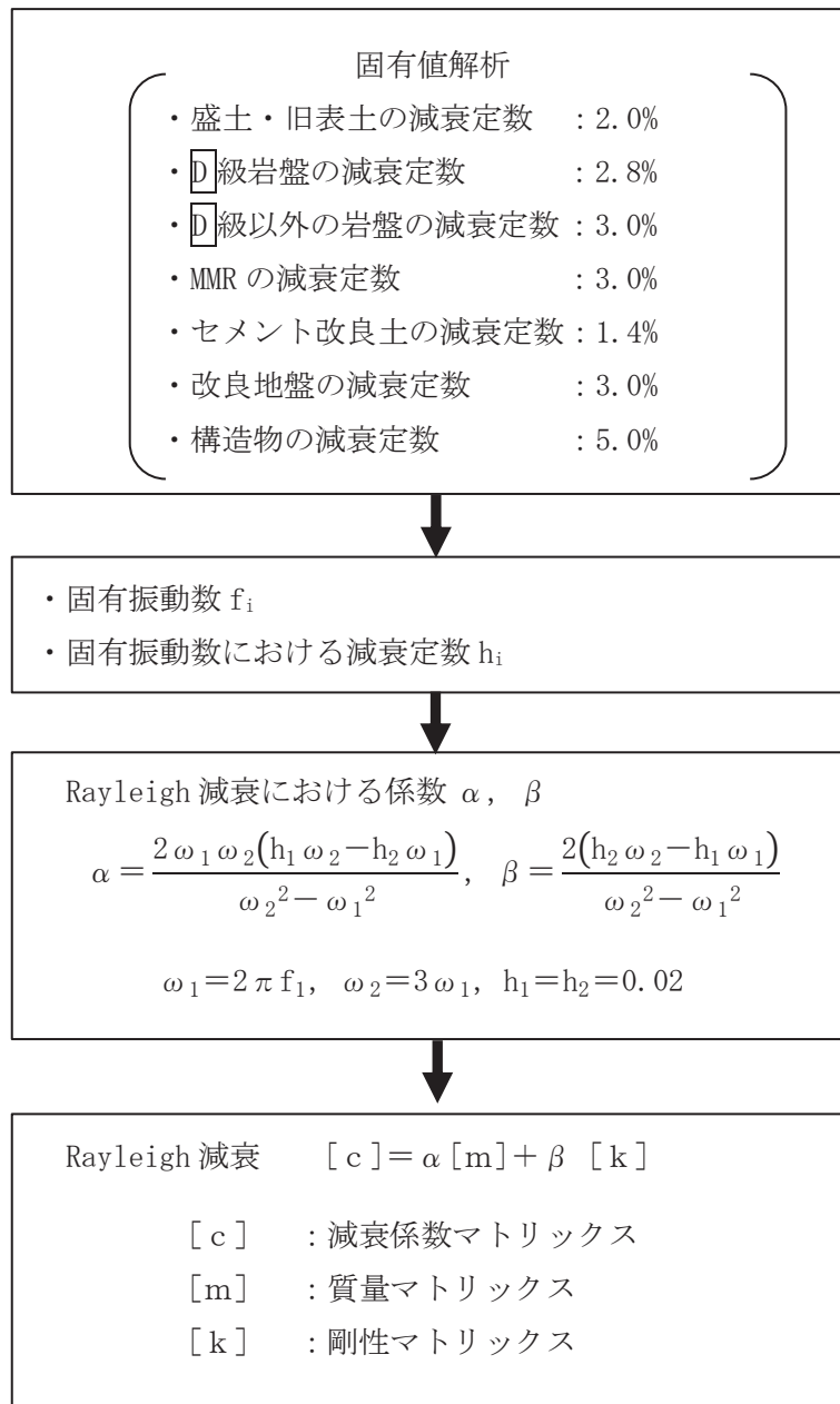
図 3-17 Rayleigh 減衰の設定フロー
