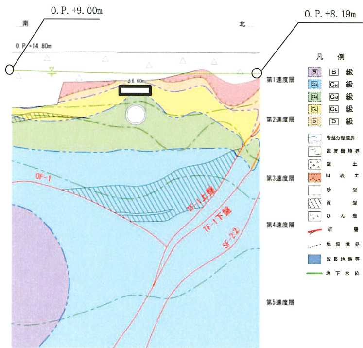
図 2-5(4) 排気筒連絡ダクト 評価対象地質断面図 (断面⑤)
