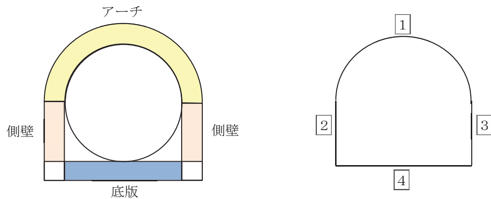
図 2-6 評価部位（土砂部）
