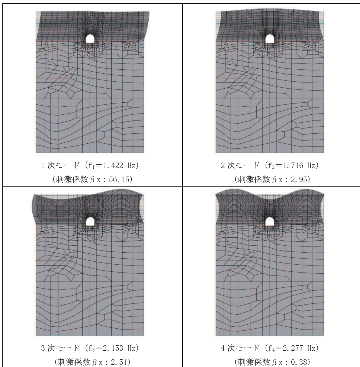
図 3-18(1) 固有値解析結果 (モード図) (断面①) (1/3)
