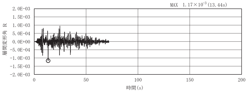
図5-1 曲げ・軸力系の破壊に対する照査が最も厳しくなるケースの層間変形角時刻歴波形（解析ケース②，S s - D 2 (++)）
