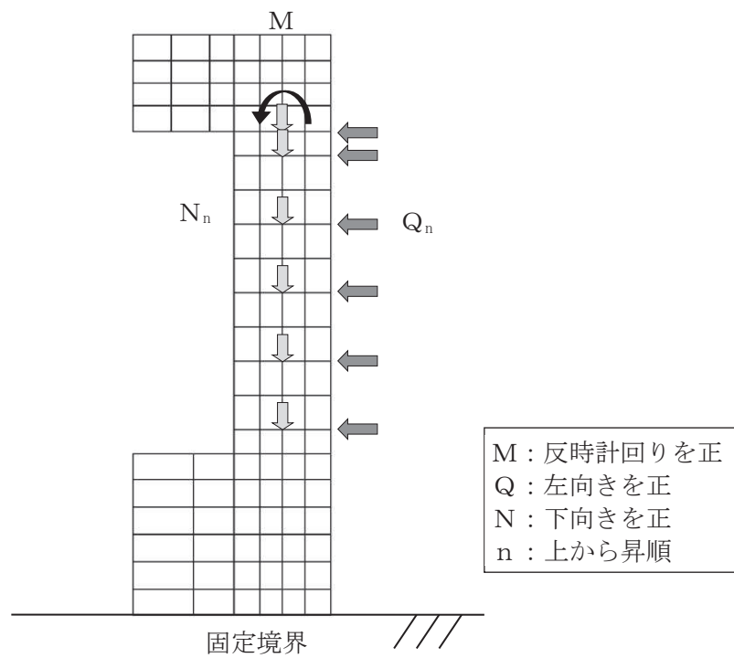
図 5-14 材料非線形解析における載荷状況（側壁）
