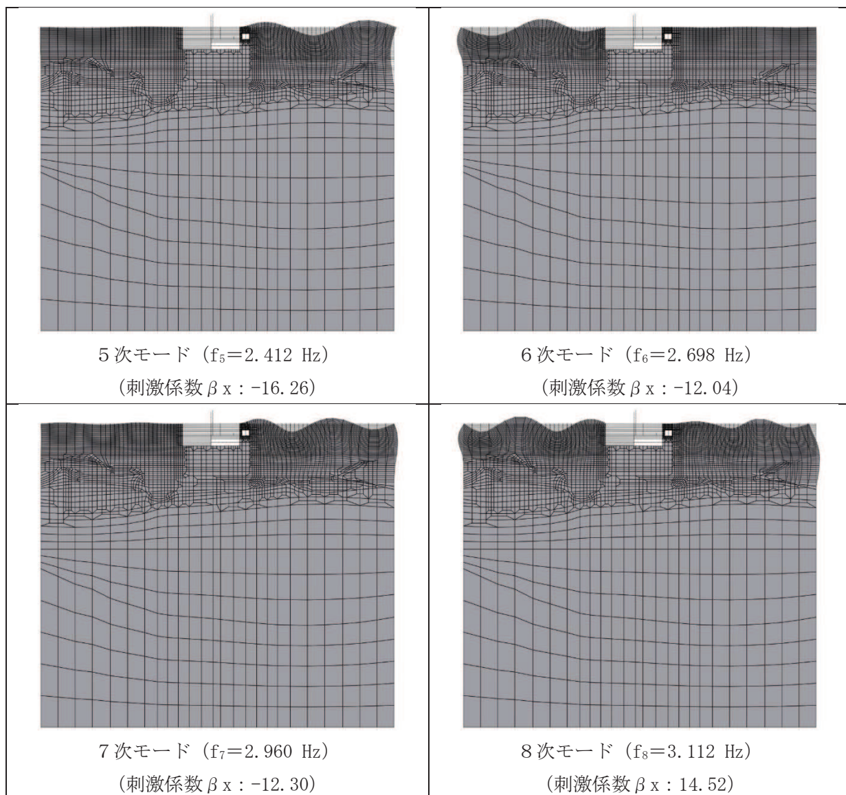
図 3-14(2) 固有値解析結果 (モード図) (2/3)
