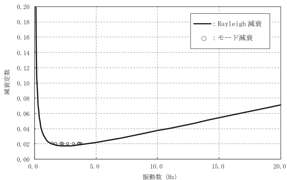
図 3-19(1) 設定した Rayleigh 減衰 (断面①)
