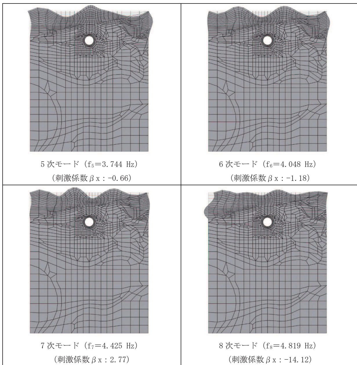
図 3-18(8) 固有値解析結果 (モード図) (断面⑤) (2/3)
