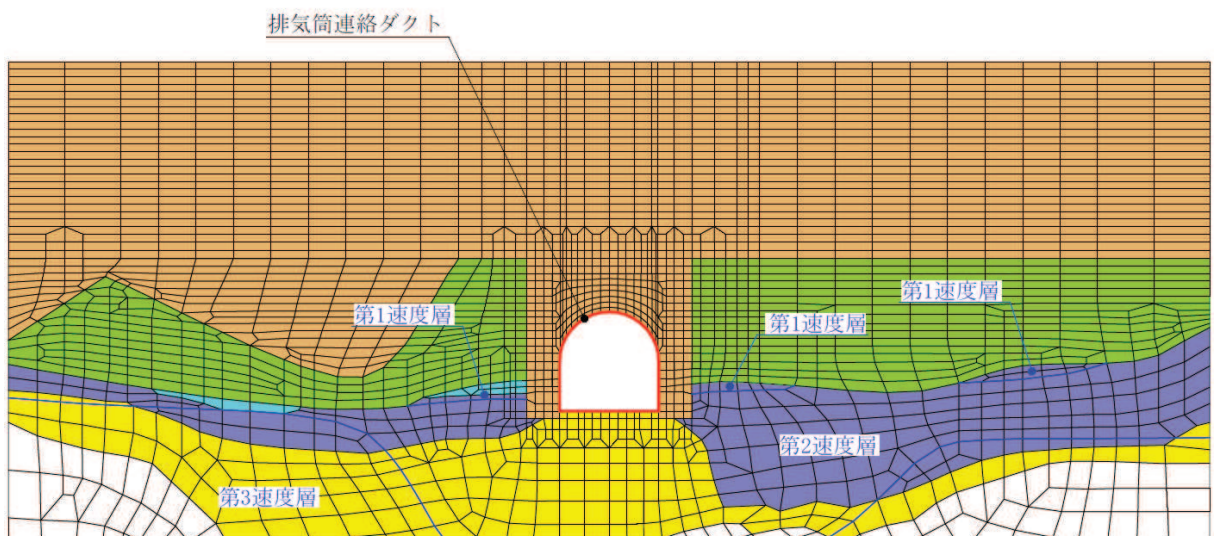
図 3-10(2) ジョイント要素の配置 (断面③)
