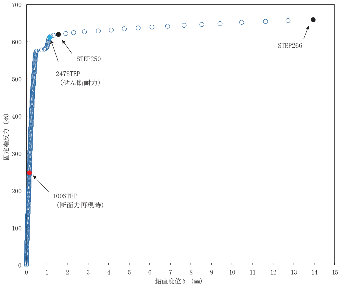
図 5-17 荷重-変位曲線 (頂版, 解析ケース③, S_s - D3 (++) )
