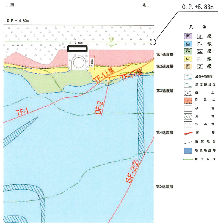
図 2-5(3) 排気筒連絡ダクト 評価対象地質断面図 (断面③)
