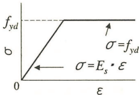
図 3-16 鉄筋の応力-ひずみ関係 （コンクリート標準示方書より引用）
