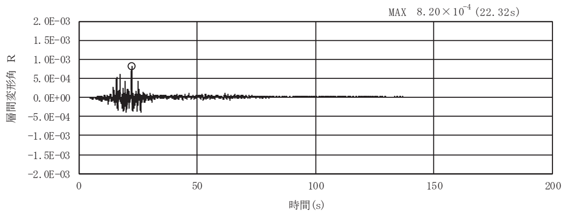
図5-1 曲げ・軸力系の破壊に対する照査が最も厳しくなるケースの層間変形角時刻歴波形（解析ケース①，S s - F 1 (-+)）
