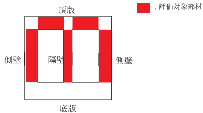
図 5-8 材料非線形解析における評価対象部材
