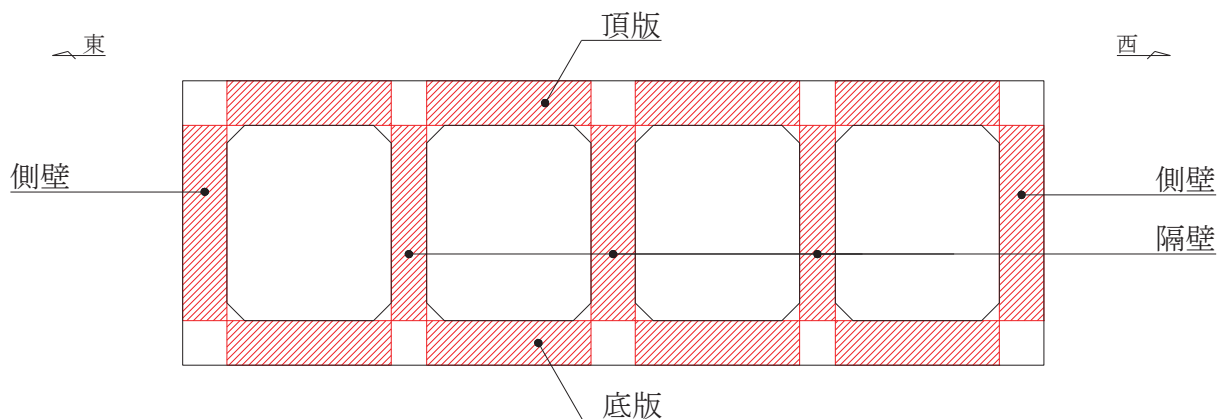
図 5-5 通水機能が要求される部材の範囲
