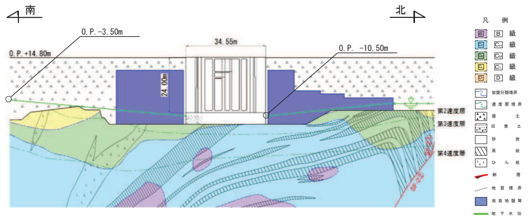
図 2-19 設計用地下水位 (A-A 断面)
