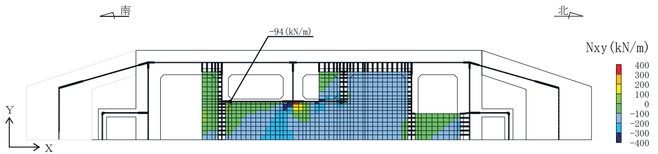
図 6-7 曲げ・軸力系の破壊に対する照査値最大時の断面力分布図 (面内せん断力 (kN/m) : N_{xy} ) (頂版, 解析ケース④, S_s - D_2 (++) )
