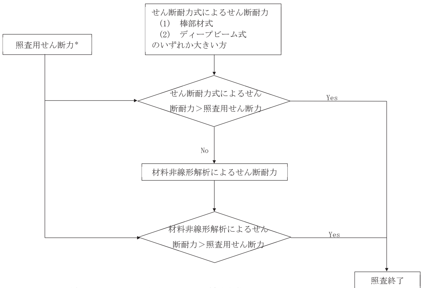
図4-18 せん断破壊に対する照査フロー
