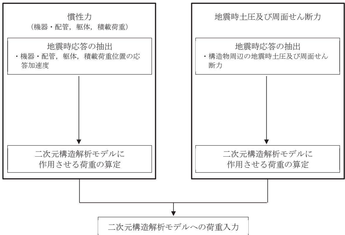
図4-10 各入力荷重の算定フロー
