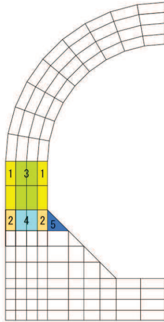
図 5-14 要素プロパティ番号図 (側壁)
