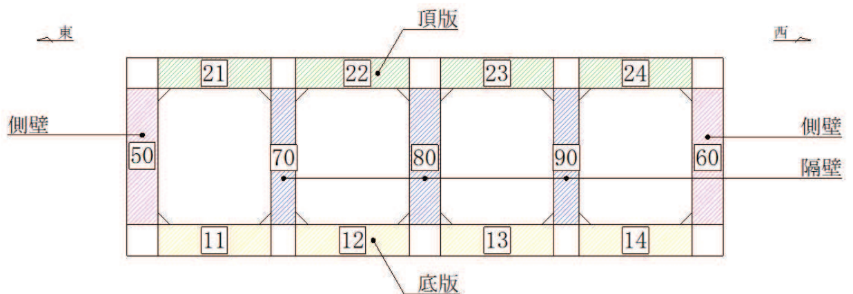
図5-2 評価位置図
