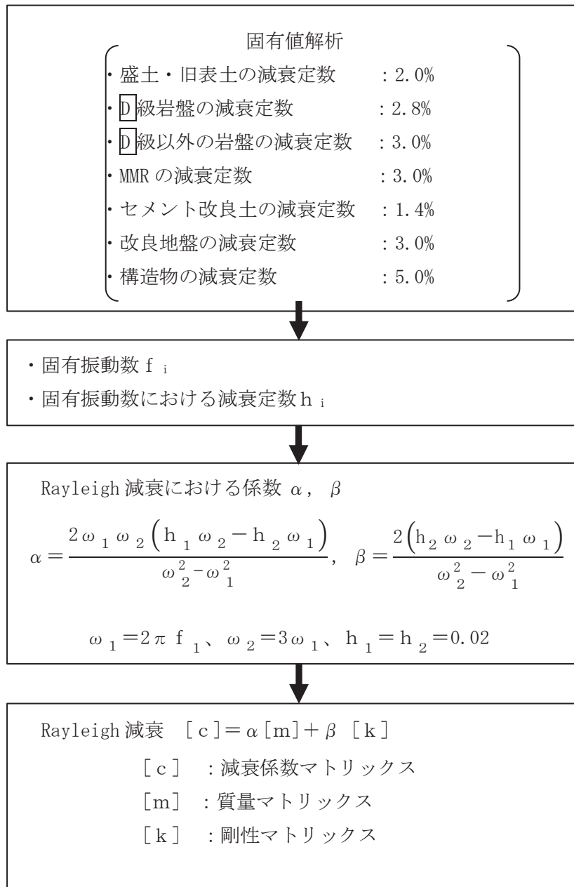
図 3-13 Rayleigh 減衰の設定フロー
