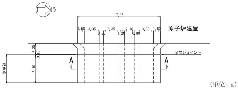
図 2-2 原子炉機器冷却海水配管ダクト（水平部）平面図
