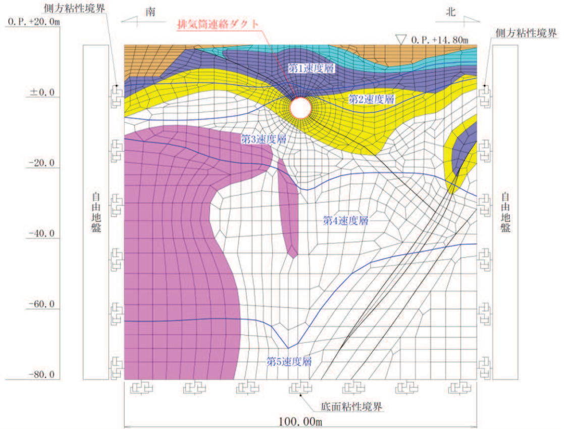
図 3-2 排気筒連絡ダクト (岩盤部) の地震応答解析モデル図
