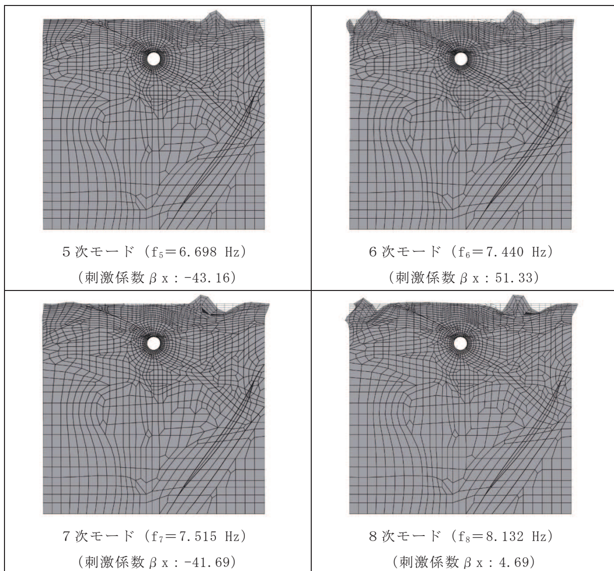
図 3-3(5) 固有値解析結果 (モード図) (断面⑦) (2/3)
