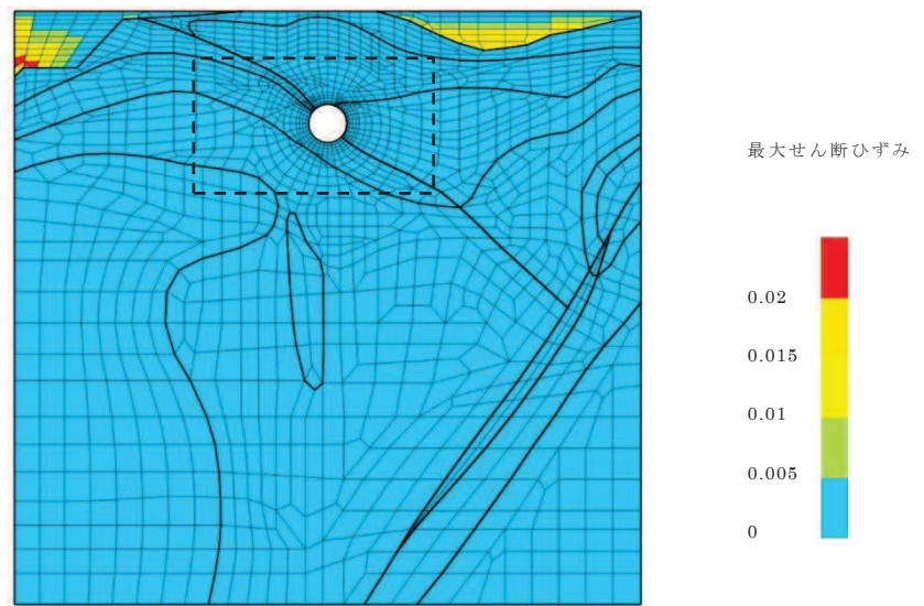
(a) 全体図
