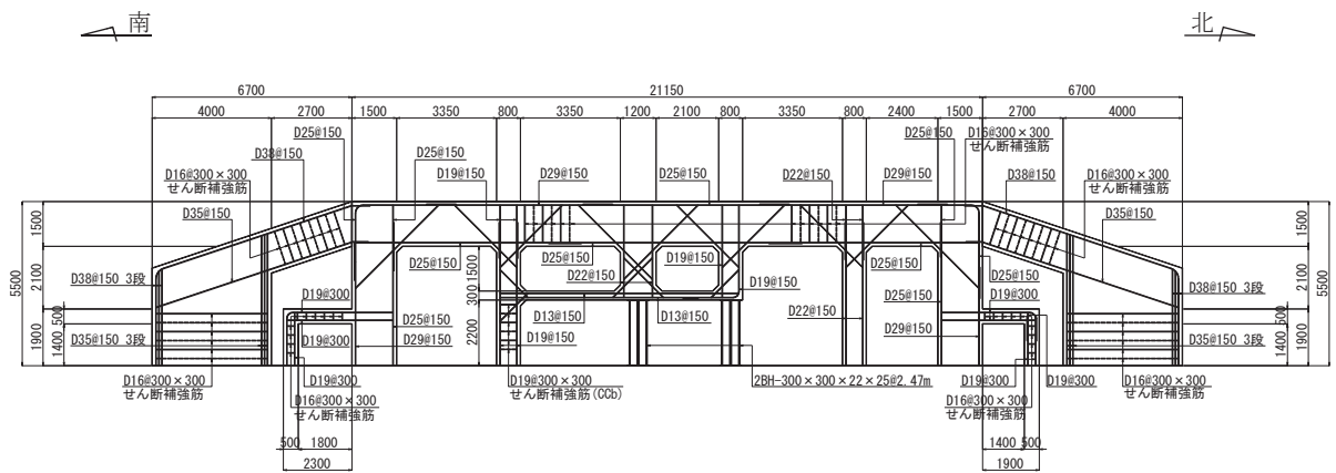
図 2-12 原子炉機器冷却海水配管ダクト（鉛直部）概略配筋図（断面②）
