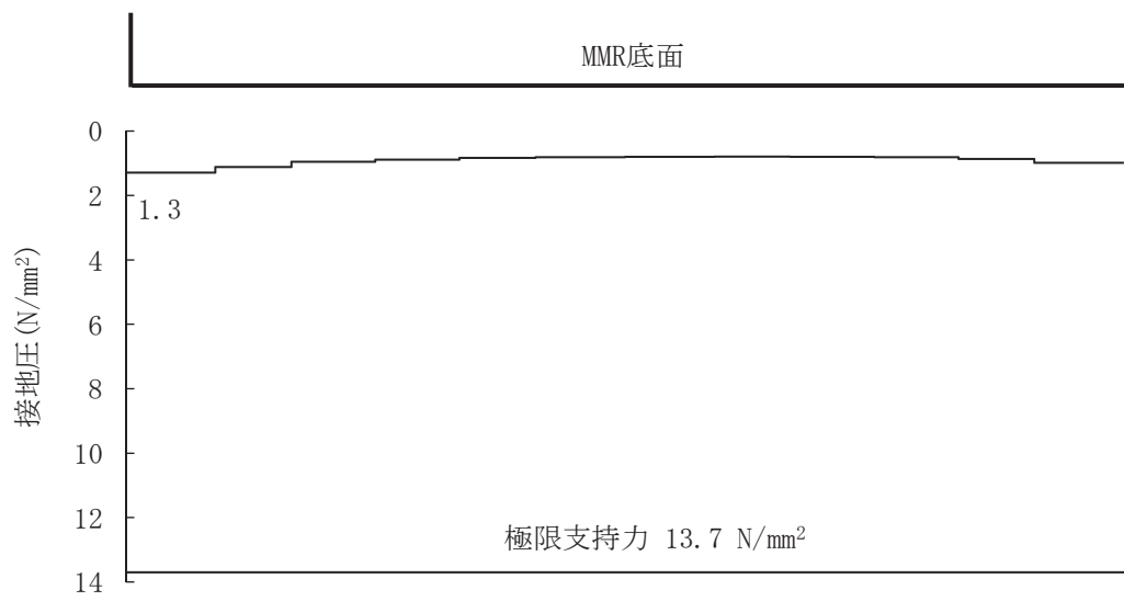
図 5-7 基礎地盤の最大接地圧分布図 (解析ケース②, S s - F 2 (-+))
