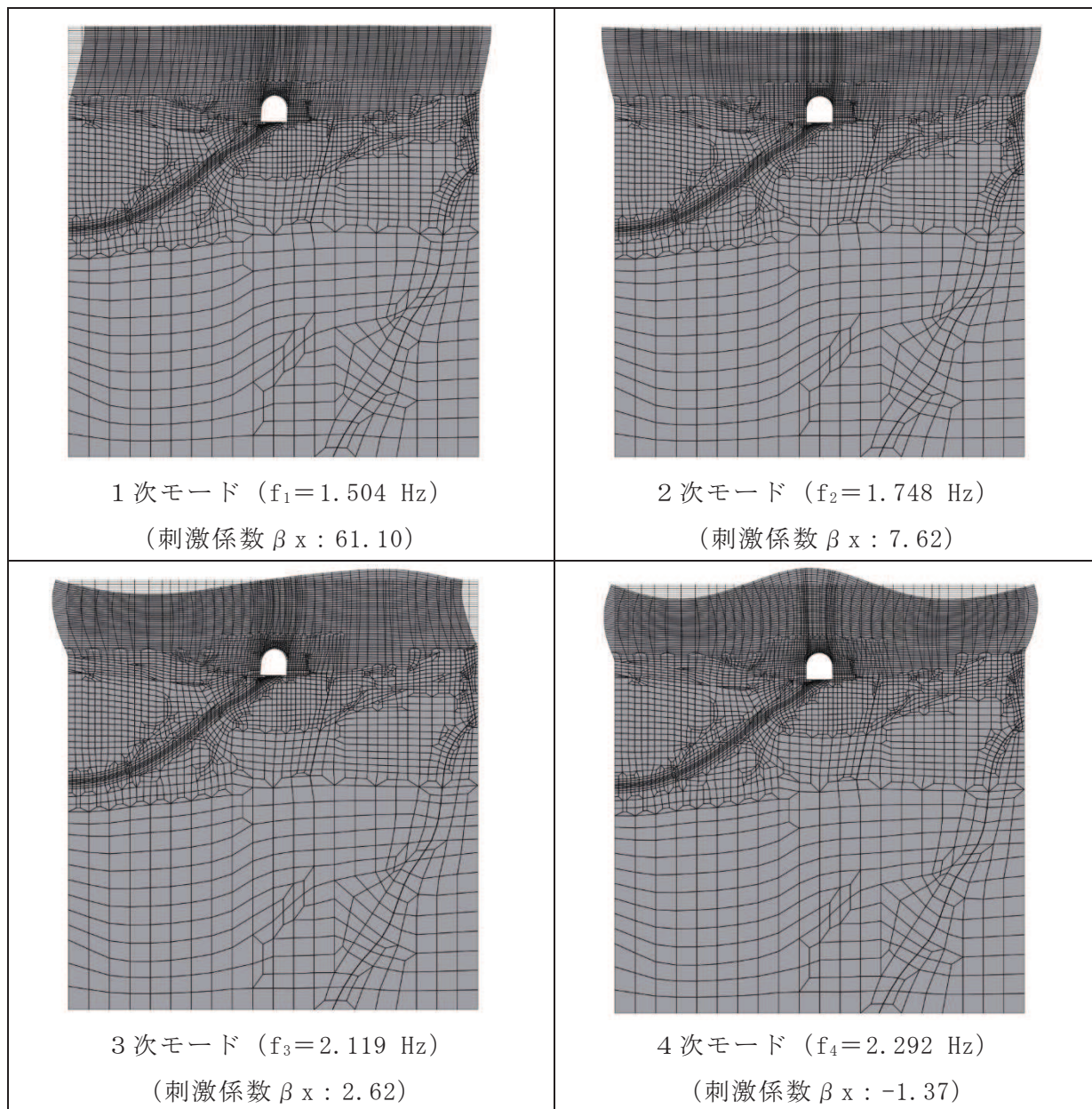
図 3-3(1) 固有値解析結果 (モード図) (断面②) (1/3)
