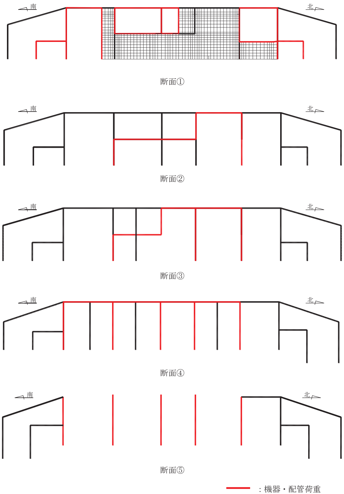
图 4-11 機器・配管荷重図
