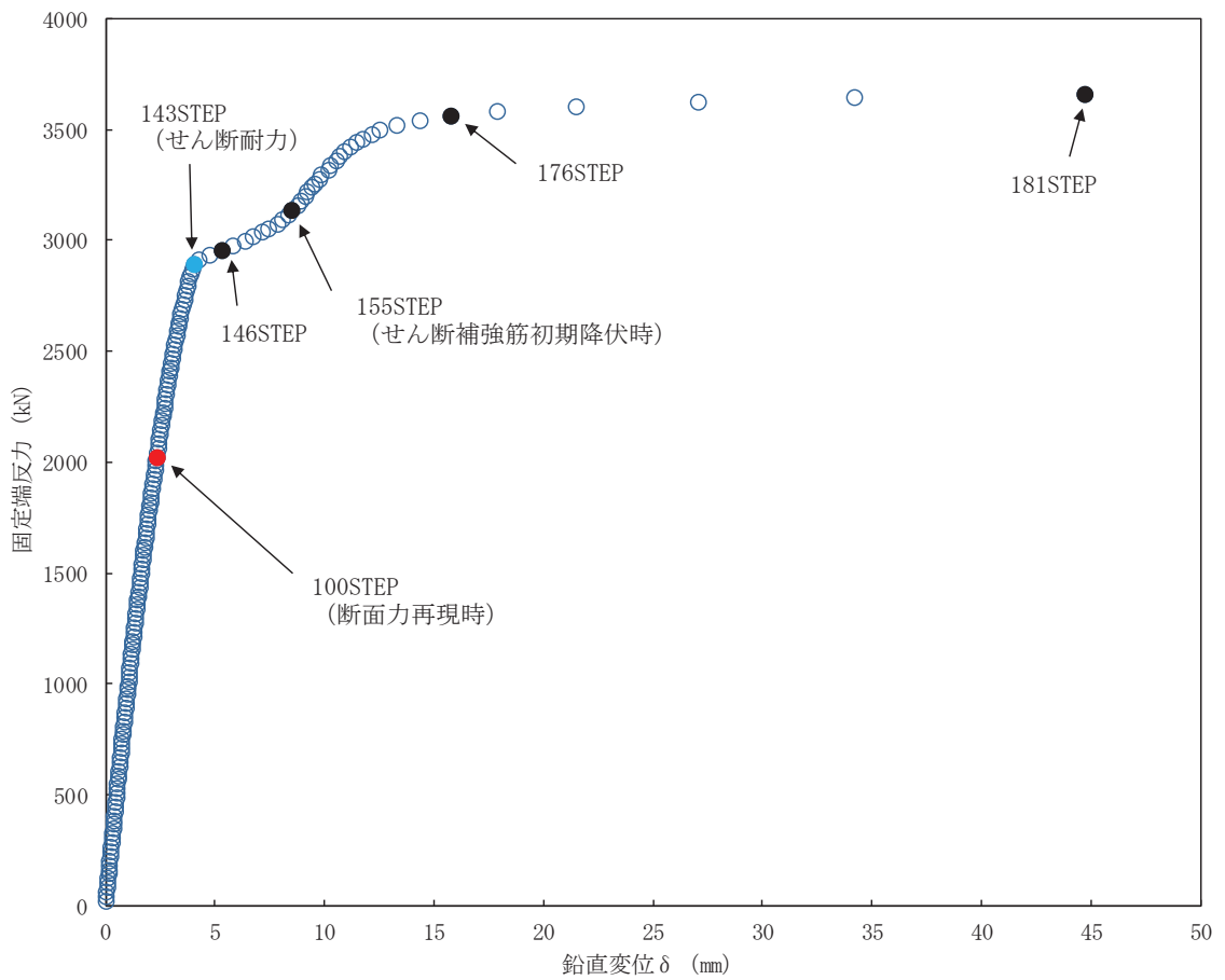
図 5-23 荷重-変位曲線 (底版, 解析ケース④, S_s - N1 (++) )
