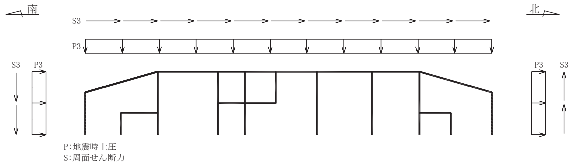
図 4-16(3) 土圧及び周面せん断力の载荷概念図 (断面③)
