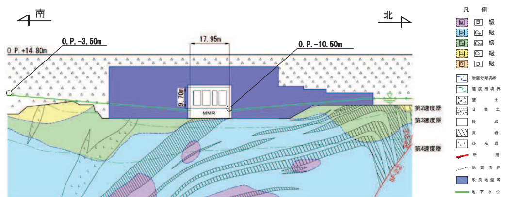
図 2-7 原子炉機器冷却海水配管ダクト（水平部）の設計用地下水位
