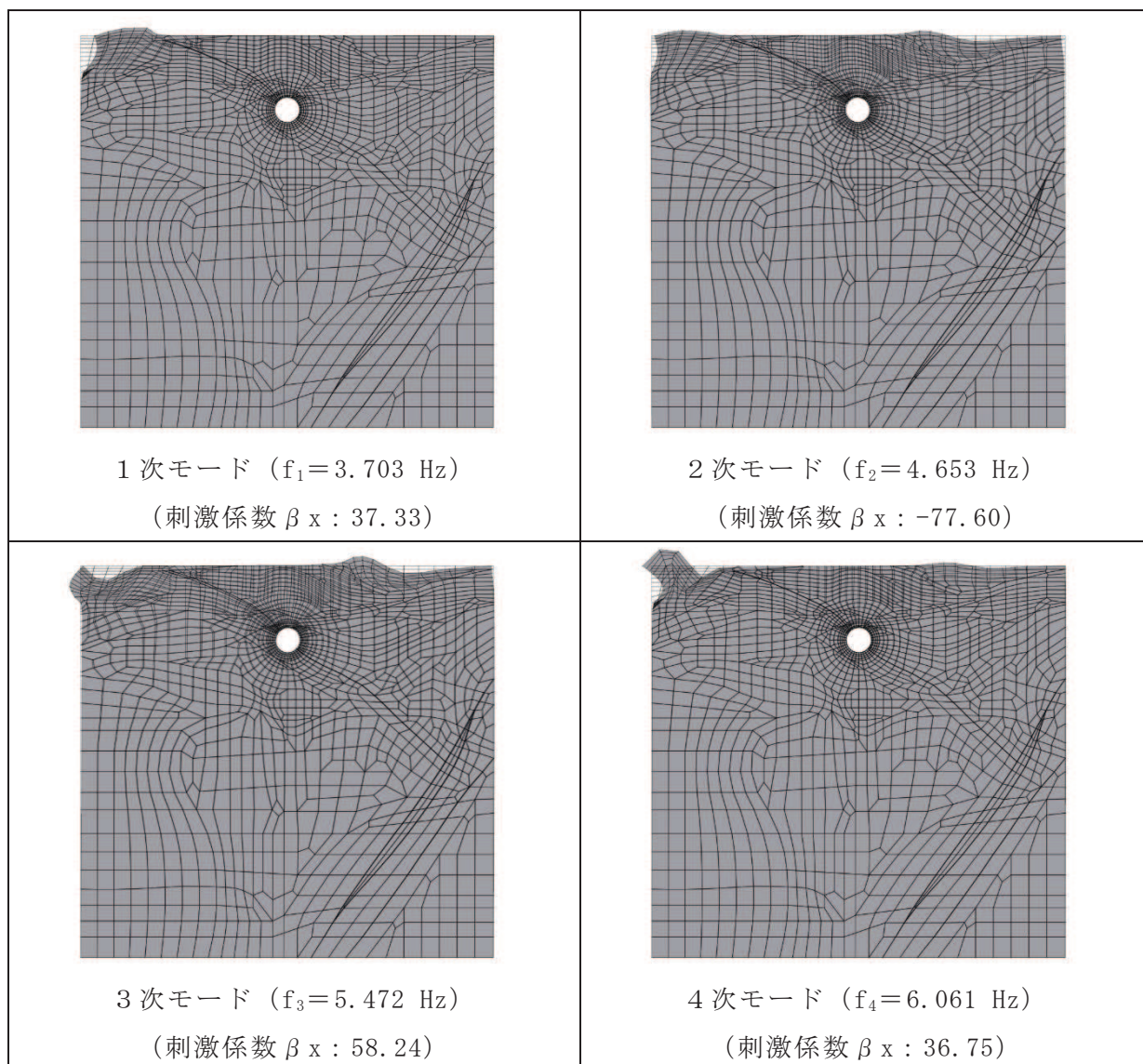
図 3-3(4) 固有値解析結果 (モード図) (断面⑦) (1/3)
