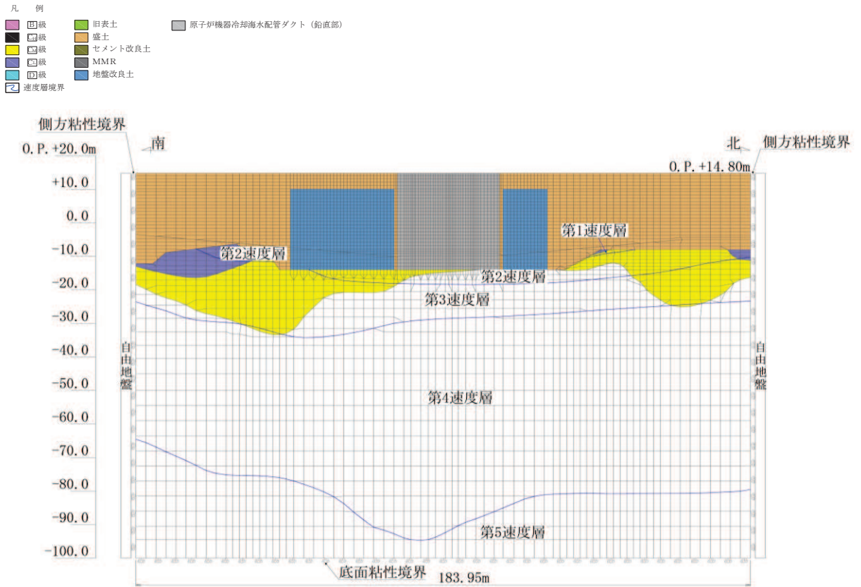
(b) 地震応答解析モデル図 (A-A 断面)
