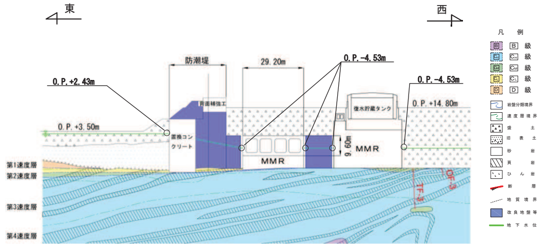
図 2-5 取水路（漸拡部）評価対象地質断面図（A-A 断面）
