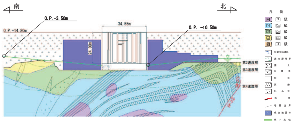
図 2-16 原子炉機器冷却海水配管ダクト(鉛直部) 地震時荷重算出用地質断面図(A-A断面:南北)
