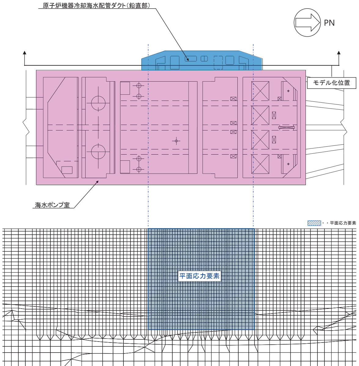
図3-9 原子炉機器冷却海水配管ダクト（鉛直部）の地震応答解析モデル （構造物部分拡大，A-A断面）
