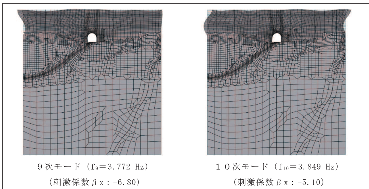
図 3-3(3) 固有値解析結果 (モード図) (断面②) (3/3)
