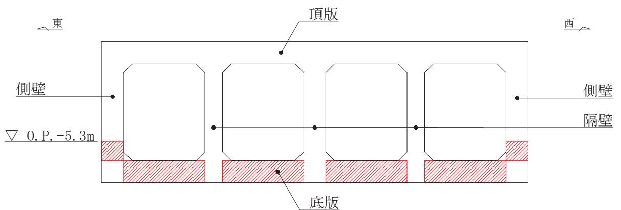
図 5-6 貯水機能が要求される部材の範囲
