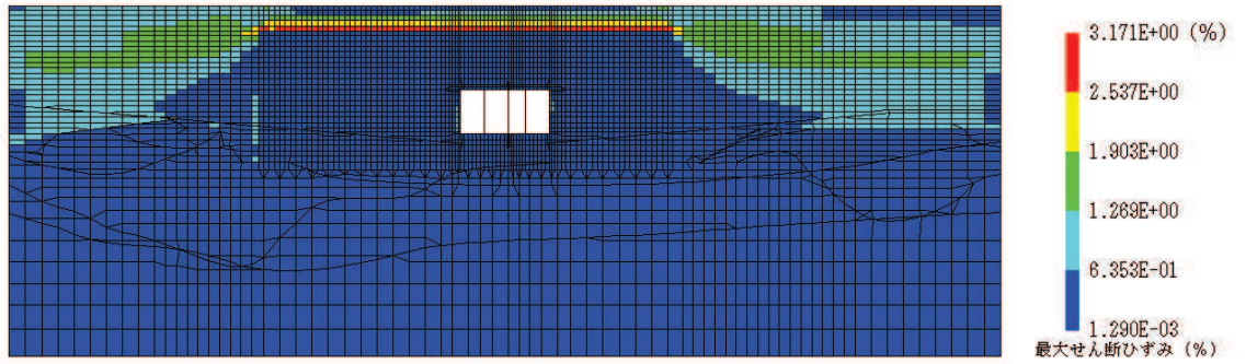
(a) 全体図
