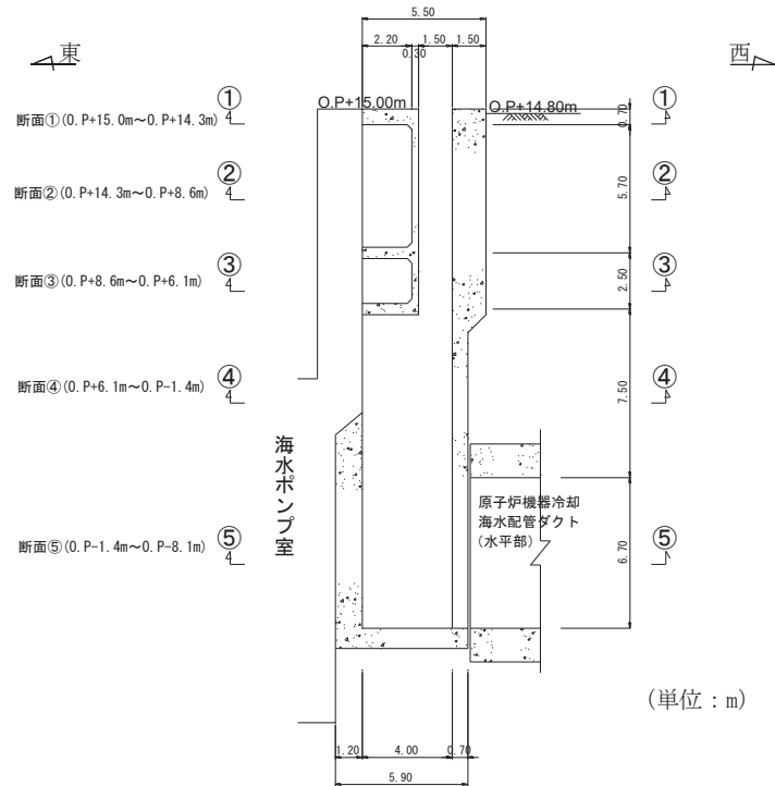
図 2-4 原子炉機器冷却海水配管ダクト（鉛直部）正面図（A-A 断面）
