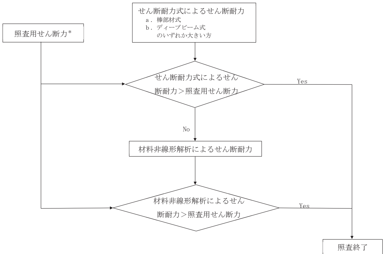
図5-30 せん断破壊に対する照査フロー
