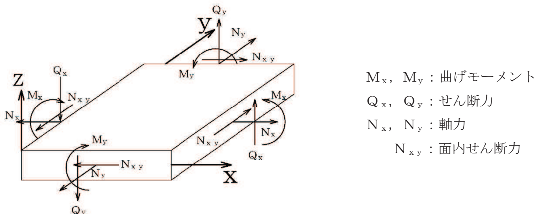
図4-6 シェル要素の各要素における断面力の方向
