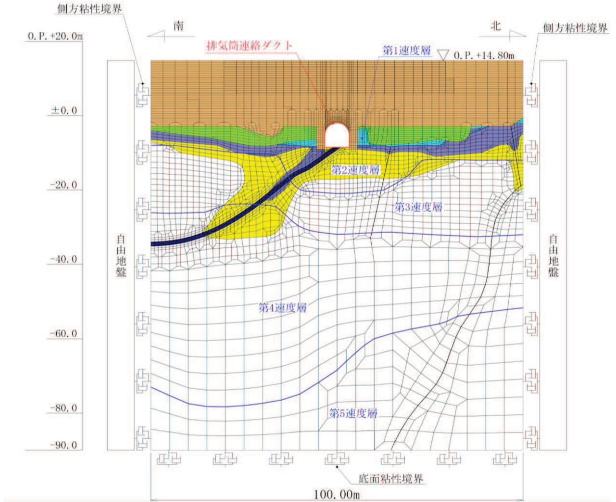
図 3-1 排気筒連絡ダクト (土砂部) の地震応答解析モデル図
