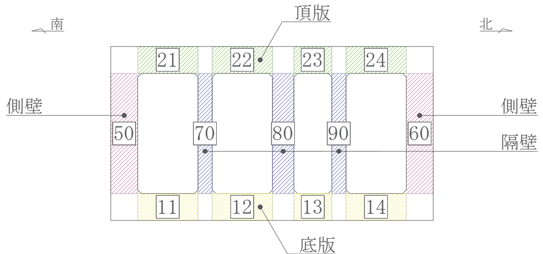
図5-2 評価位置図
