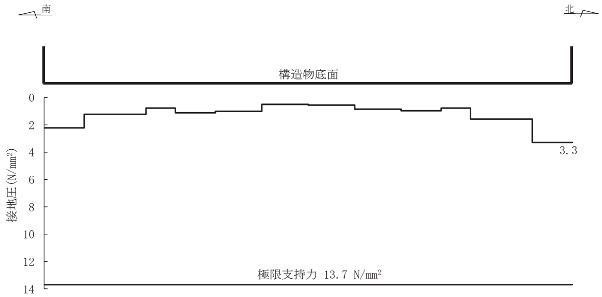
図 5-29 基礎地盤の最大接地圧分布図 (断面①) (解析ケース①, S s - F 2 (-+))
