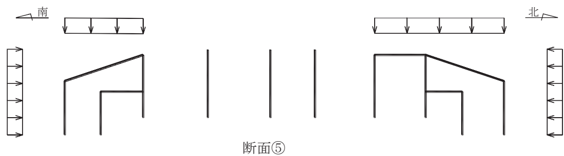
図 4-12 常時土圧の載荷概念図
