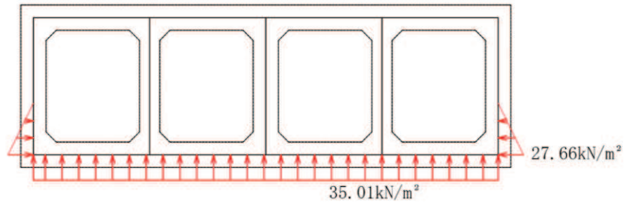
図3-18 外水圧図
