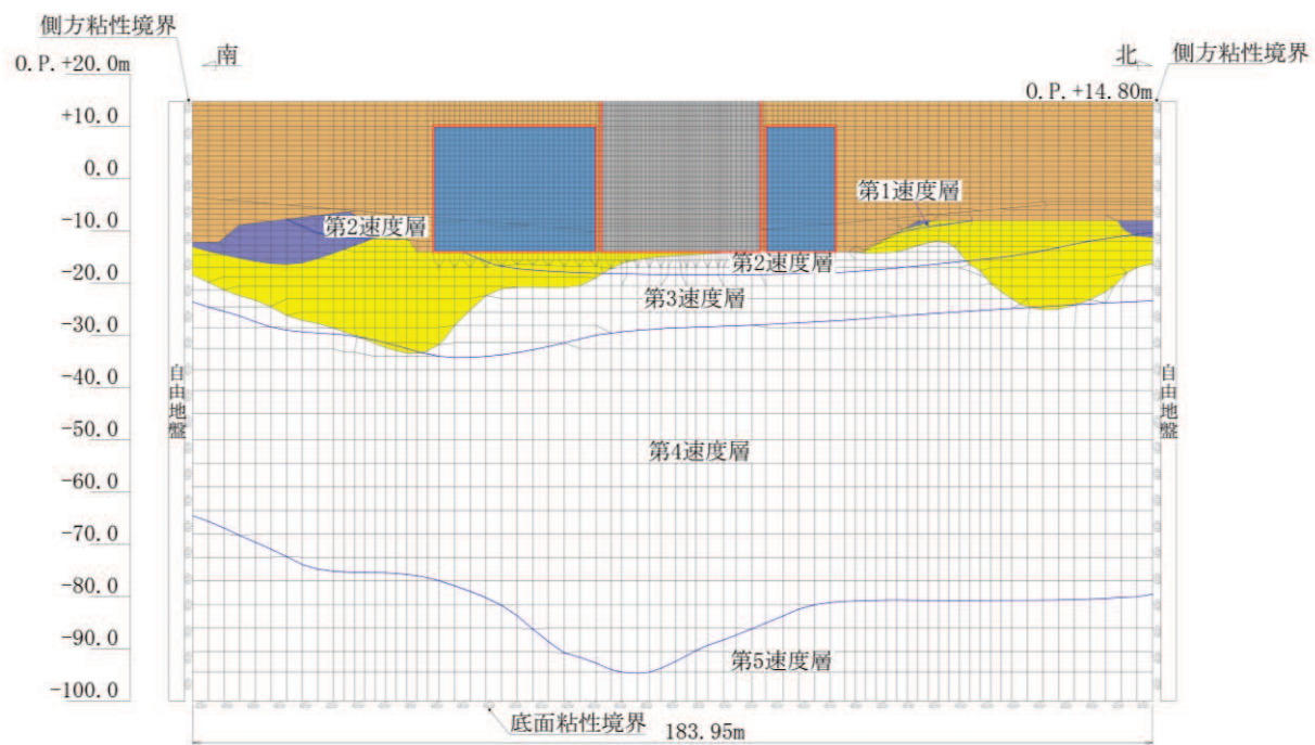
図 3-11 ジョイント要素の配置 (A-A 断面：南北)
