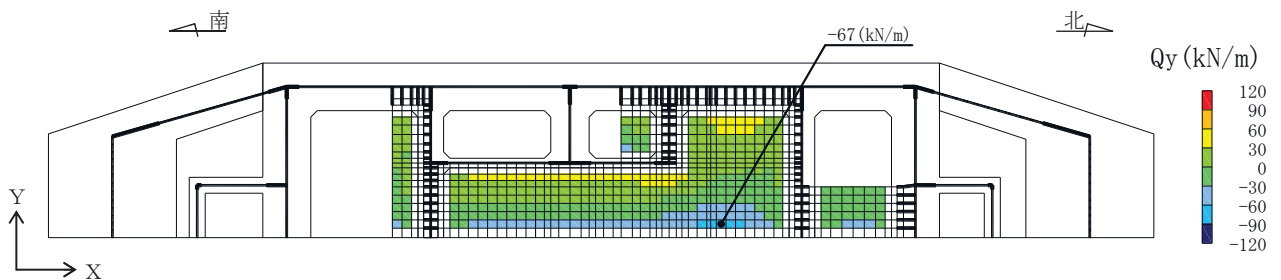
図6-18 せん断破壊に対する照査における照査値最大時の断面力分布図
