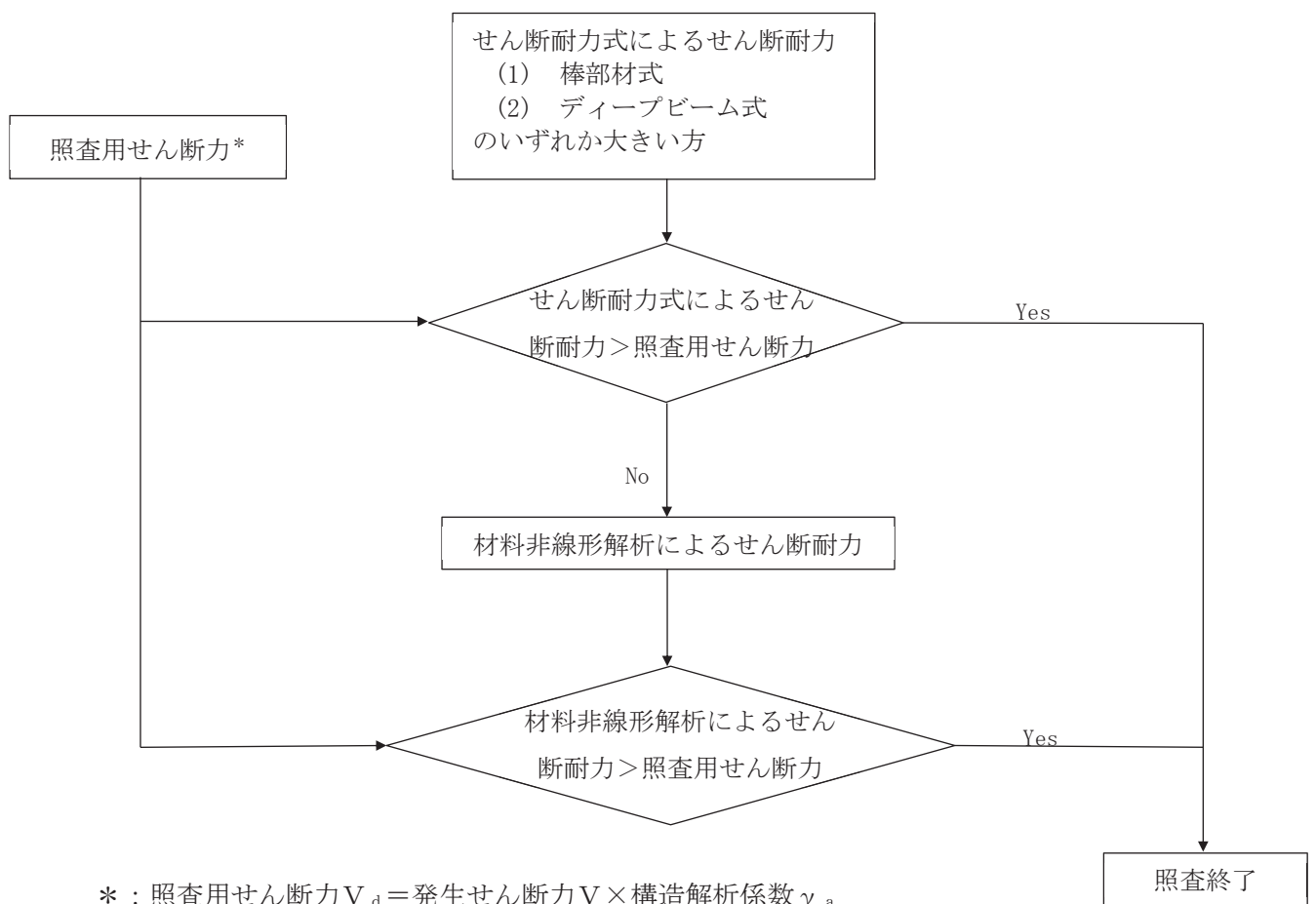
図4-31 せん断破壊に対する照査フロー
