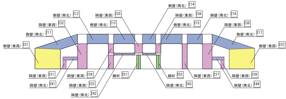
断面②
