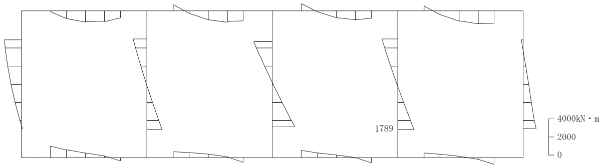
(a) 曲げモーメント (kN・m)
