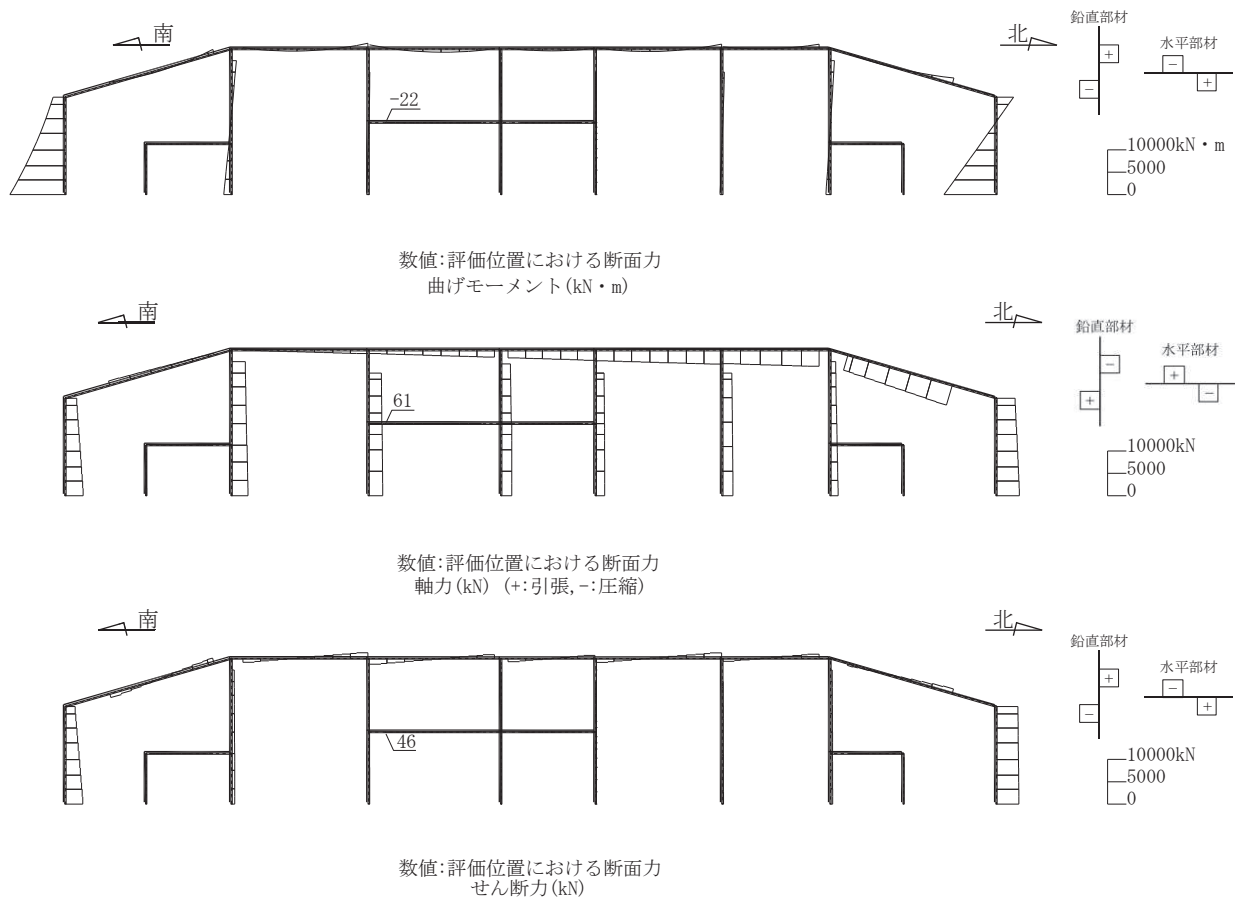
図 6-9 曲げ・軸力系の破壊に対する照査値最大時の断面力図 (断面②, 隔壁 (南北), 解析ケース①, S s - D 1 (-+))
