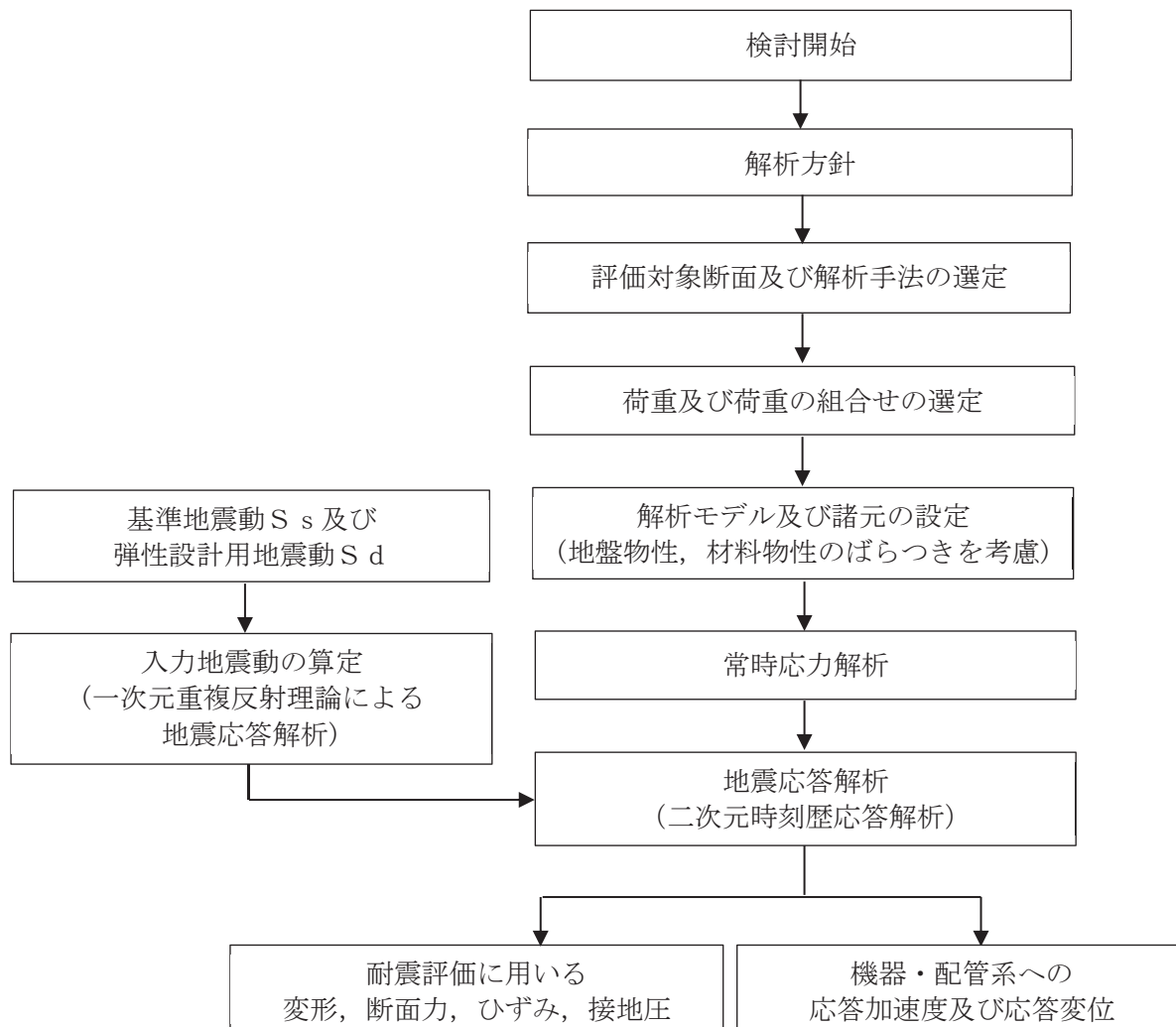
図 2-8 原子炉機器冷却海水配管ダクト（水平部）の地震応答解析フロー
