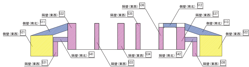
断面⑤
