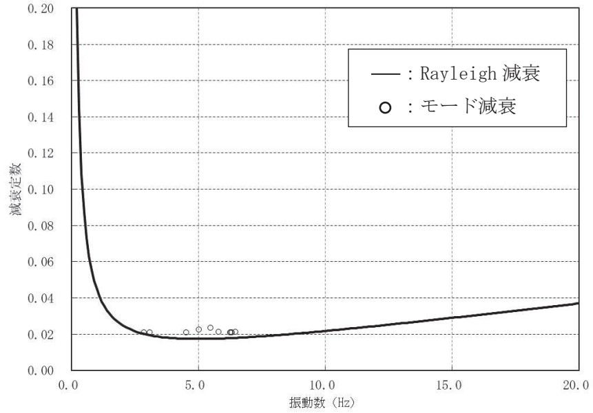
図 3-16 設定した Rayleigh 減衰 (A-A 断面 : 南北)
