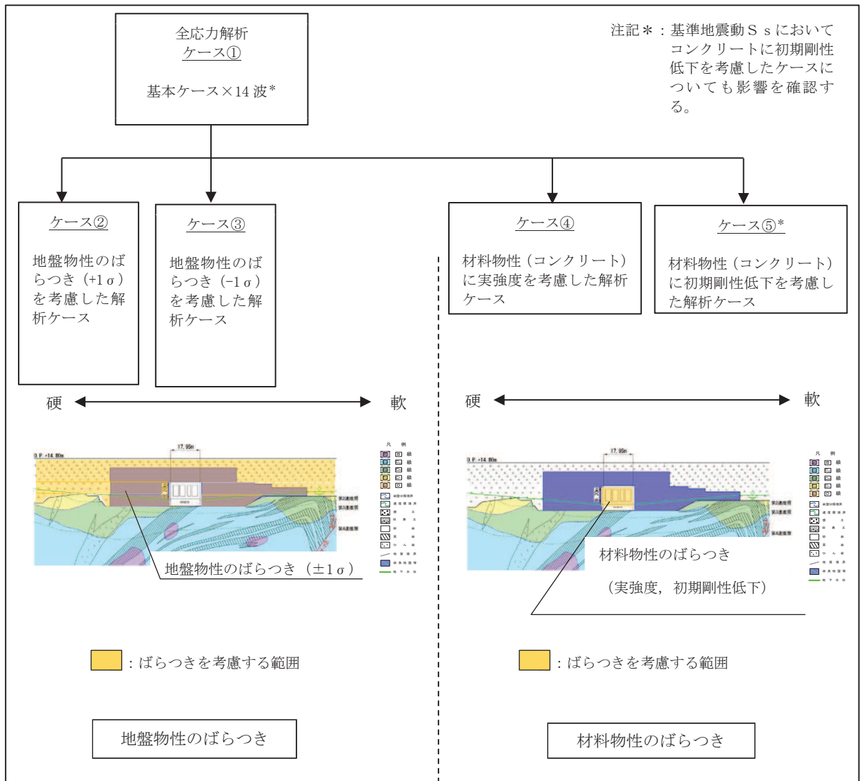
図 3-22 機器・配管系の耐震評価に適用する解析ケース
