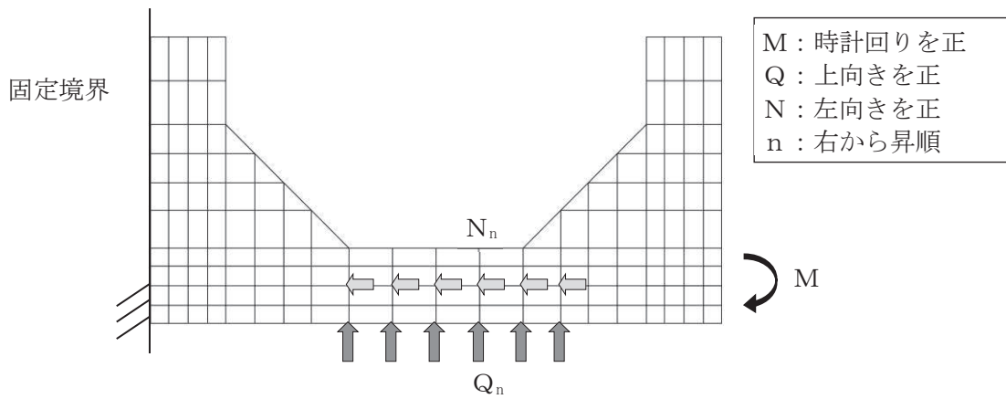
図 5-17 材料非線形解析における荷重状況（底版）
