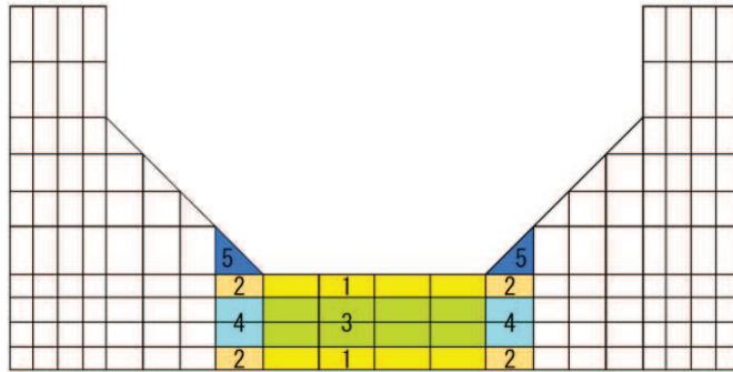
図 5-15 要素プロパティ番号図 (底版)
