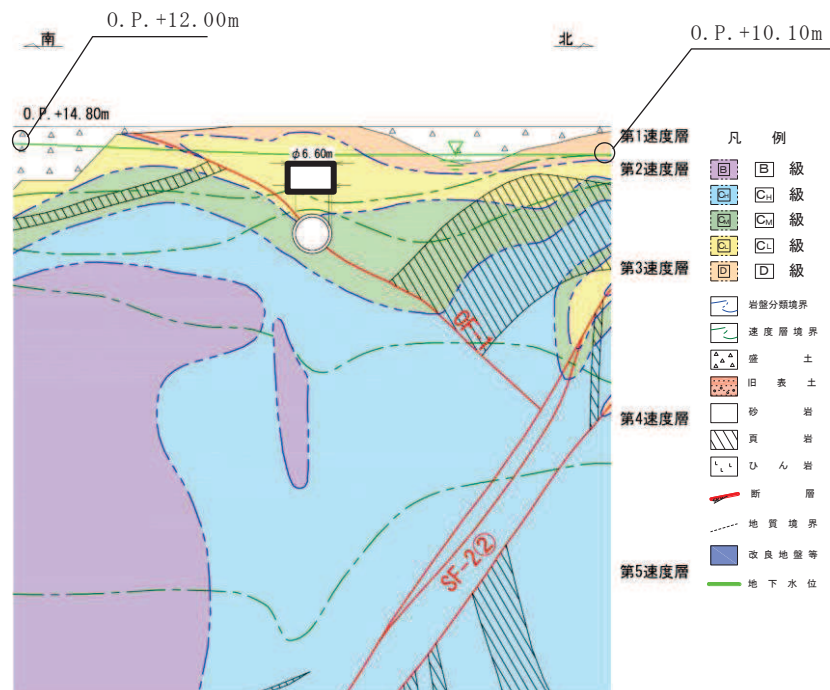
図 2-5 設計用地下水位 (岩盤部, (断面⑦))
