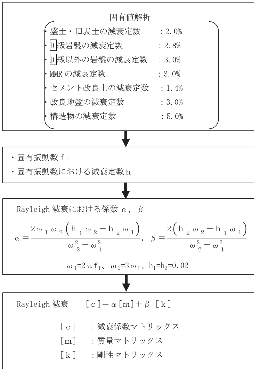
図 3-15 Rayleigh 減衰の設定フロー
