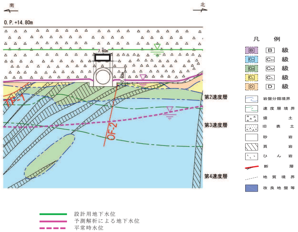
図 2-2 排気筒連絡ダクトにおける設計用地下水位と平常時水位の比較（横断(断面①)）
