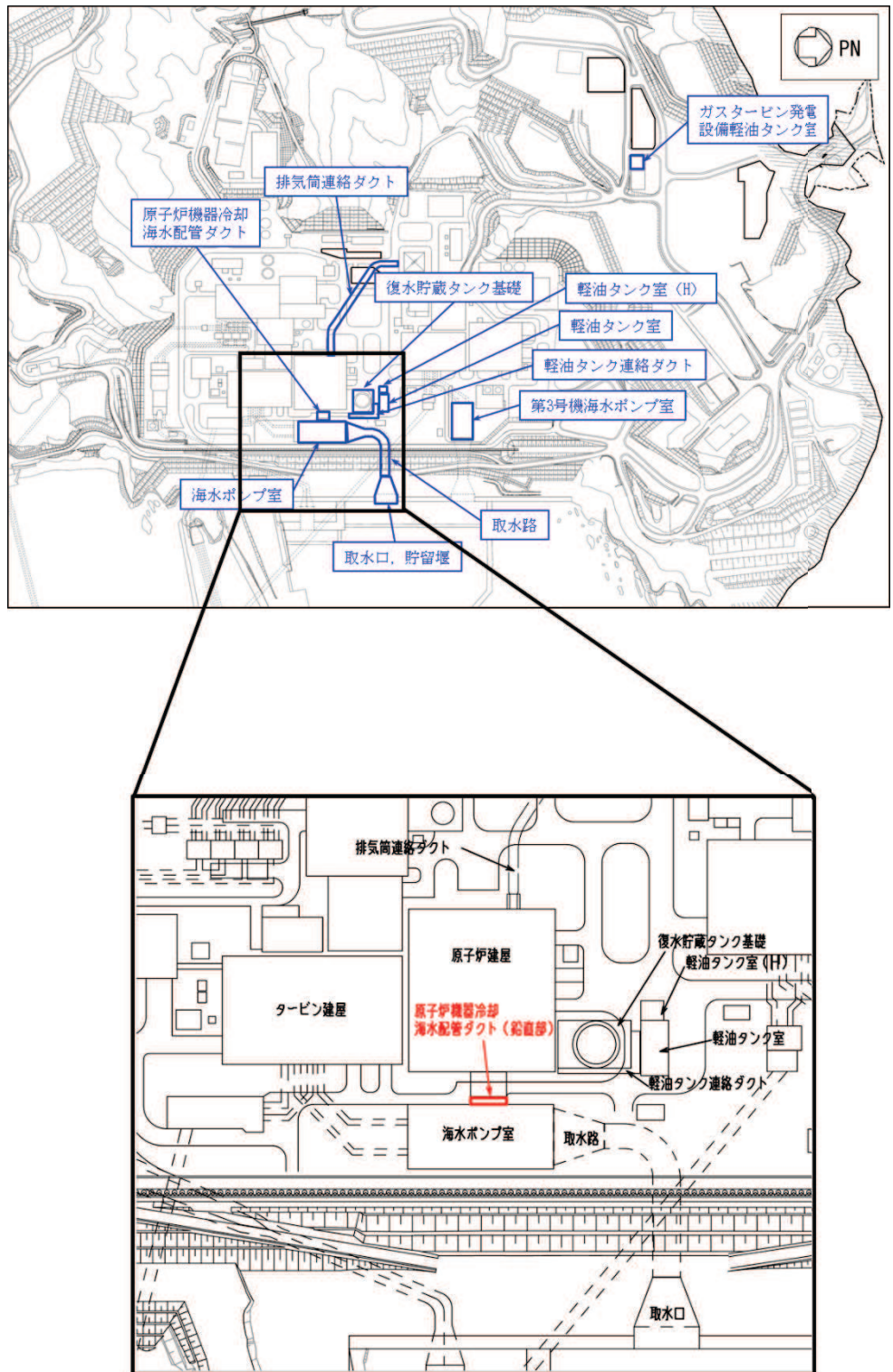
図 2-2 原子炉機器冷却海水配管ダクト（鉛直部）の位置図
