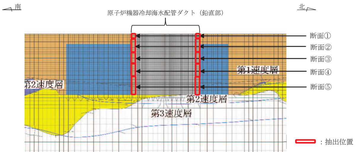
図 4-15 地震時土圧の抽出位置 (A-A 断面：南北)
