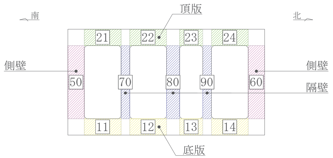
图 5-5 評価位置図
