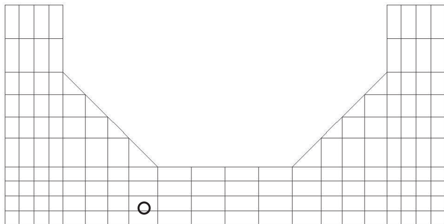
図 5-24 せん断補強筋の初期降伏箇所 (底版, 解析ケース④, S_s - N1 (++) 155STEP)
