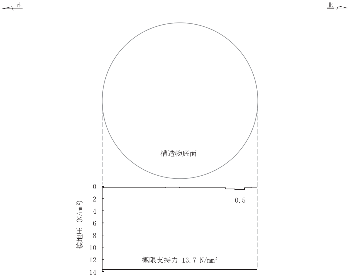
図 5-10 接地圧分布図 (S s -D 2 (++)) (解析ケース①：標準ケース)
