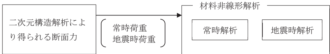
図 6-32 荷重の作用手順
