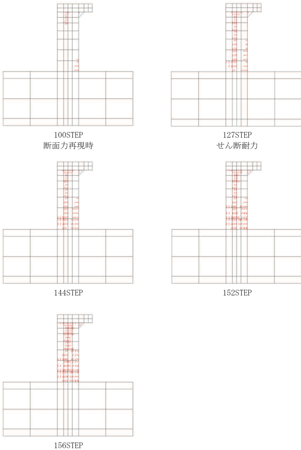
図 6-34 各ステップにおけるひび割れ図 (隔壁, 解析ケース④ 地震動 S s - D 2 (++) )
