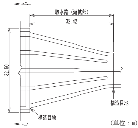
図 2-2 取水路 (漸拡部) 平面図
