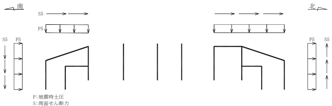
図 4-16(5) 土圧及び周面せん断力の载荷概念図 (断面⑤)
