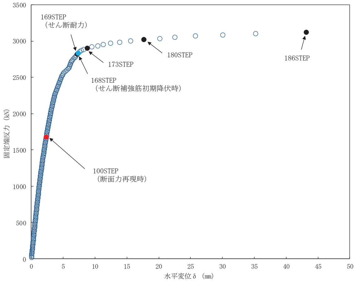
図 5-19 荷重-変位曲線 (側壁, 解析ケース③, S_s - N1 (++))
