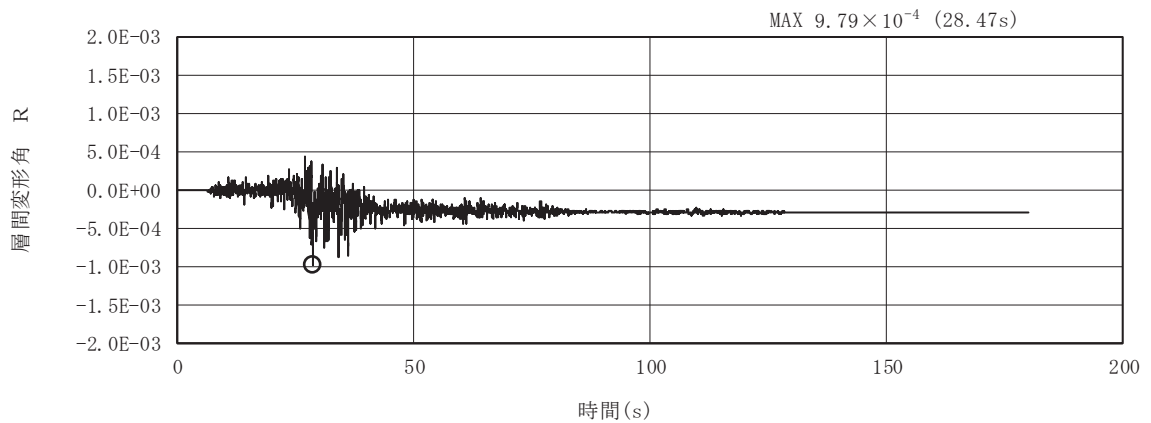
図5-1 曲げ・軸力系の破壊に対する照査が最も厳しくなるケースの層間変形角時刻歴波形（解析ケース④，地震動S s - F 2 (-+)）
