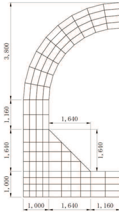
(a) 側壁
