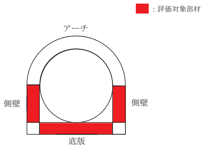
図 5-12 材料非線形解析における評価対象部材
