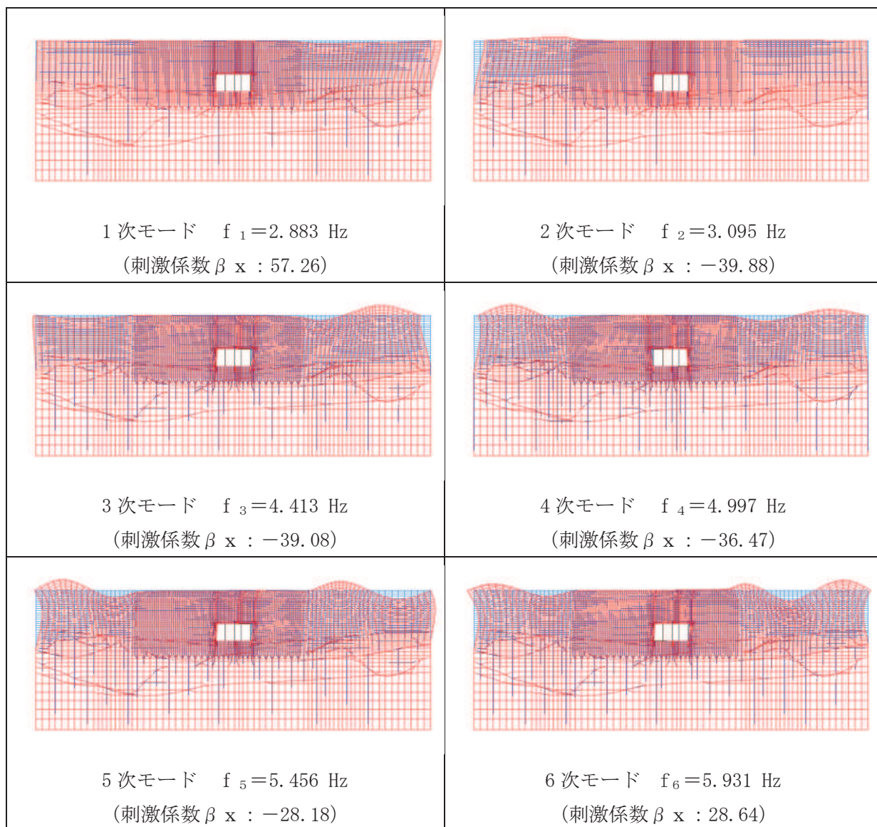
図3-16 固有値解析結果 (モード図) (1/2)
