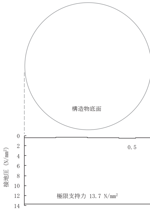
図 5-30 基礎地盤の最大接地圧分布図 (断面⑤) (解析ケース③, S s - D 2 (-+))
