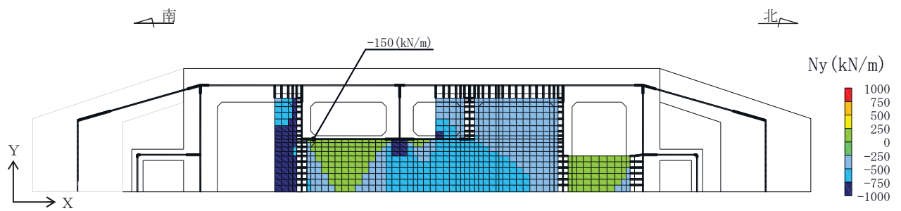
図 6-6 曲げ・軸力系の破壊に対する照査値最大時の断面力分布図 (軸力 (kN/m) : N_y ) (頂版, 解析ケース④, S_s - D_2 (++) )
