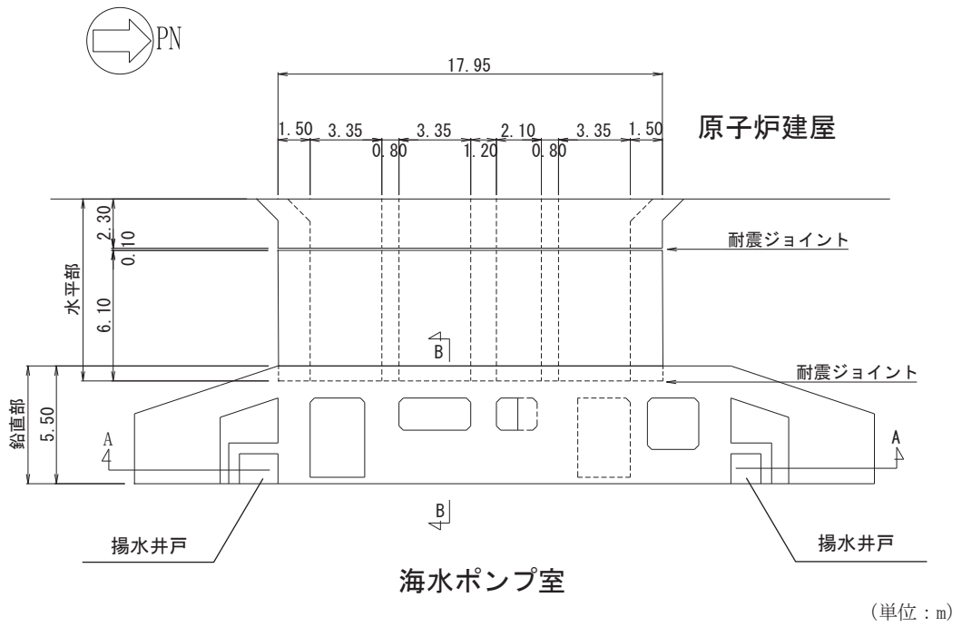
図 2-3 原子炉機器冷却海水配管ダクト（鉛直部）平面図
