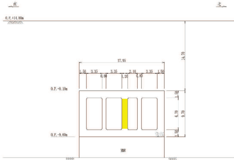
図 4-30 Ccb工法を用いる部材
