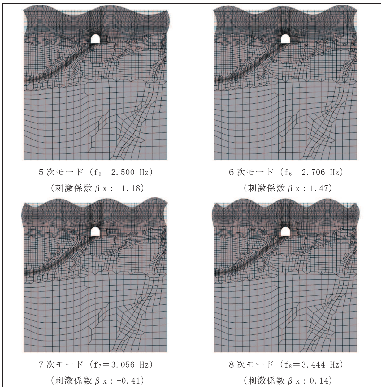
図 3-3(2) 固有値解析結果 (モード図) (断面②) (2/3)
