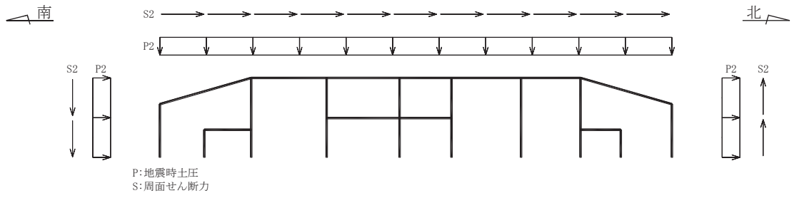
図 4-16(2) 土圧及び周面せん断力の载荷概念図 (断面②)
