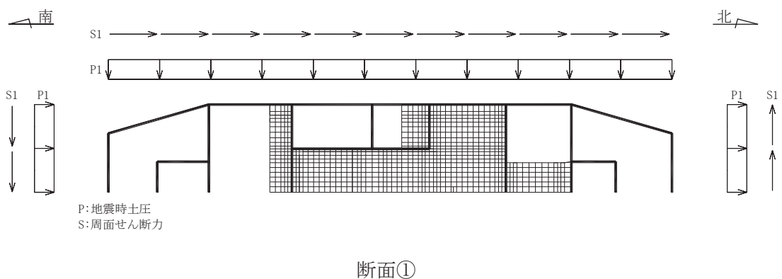
図 4-16(1) 土圧及び周面せん断力の载荷概念図 (断面①)
