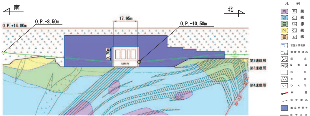
図 2-5 原子炉機器冷却海水配管ダクト（水平部）評価対象地質断面図（A-A 断面）
