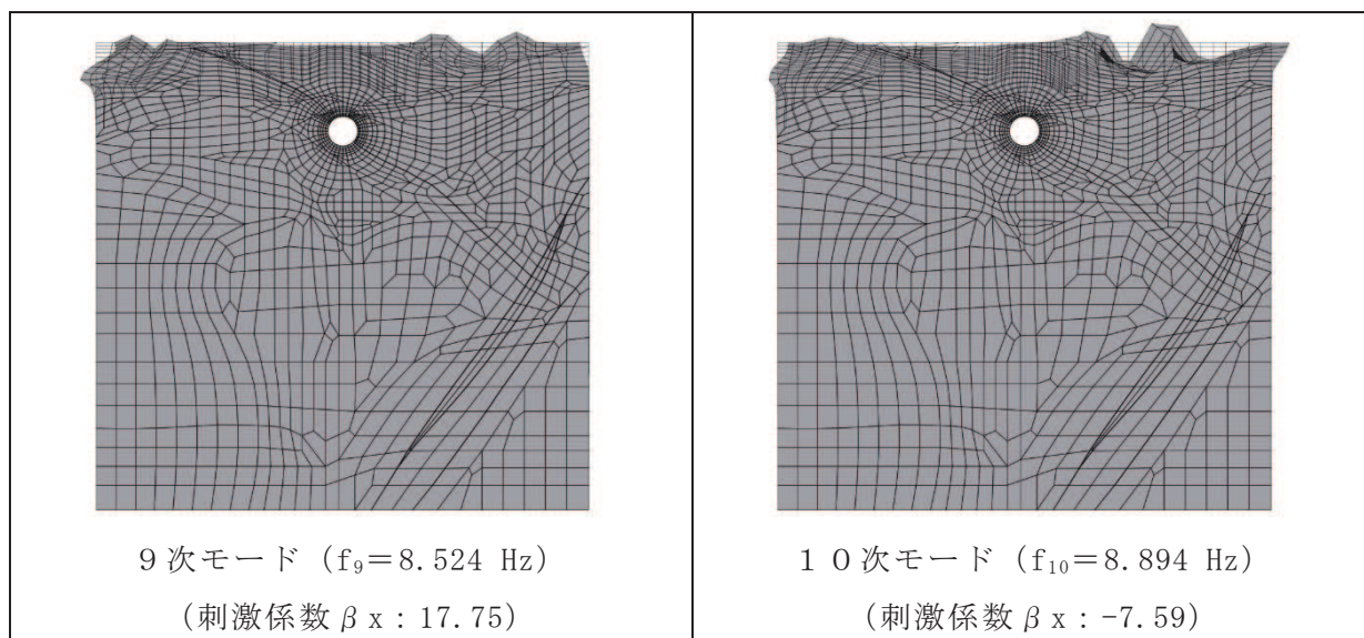
図 3-3(6) 固有値解析結果 (モード図) (断面⑦) (3/3)
