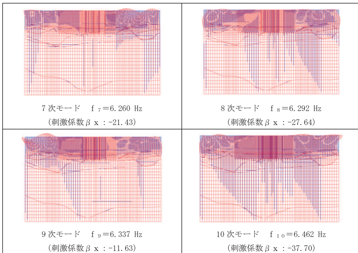
図 3-14(2) 固有値解析結果 (モード図) (A-A 断面 : 南北) (2/2)
