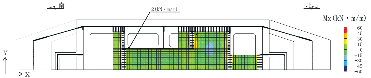
図 6-3 曲げ・軸力系の破壊に対する照査値最大時の断面力分布図 (曲げモーメント (kN・m/m) : M_x ) (頂版, 解析ケース④, S s - D 2 (++) )
