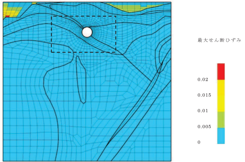
(a) 全体図
