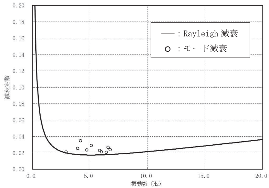
図 3-17 設定した Rayleigh 減衰 (B-B 断面 : 東西)
