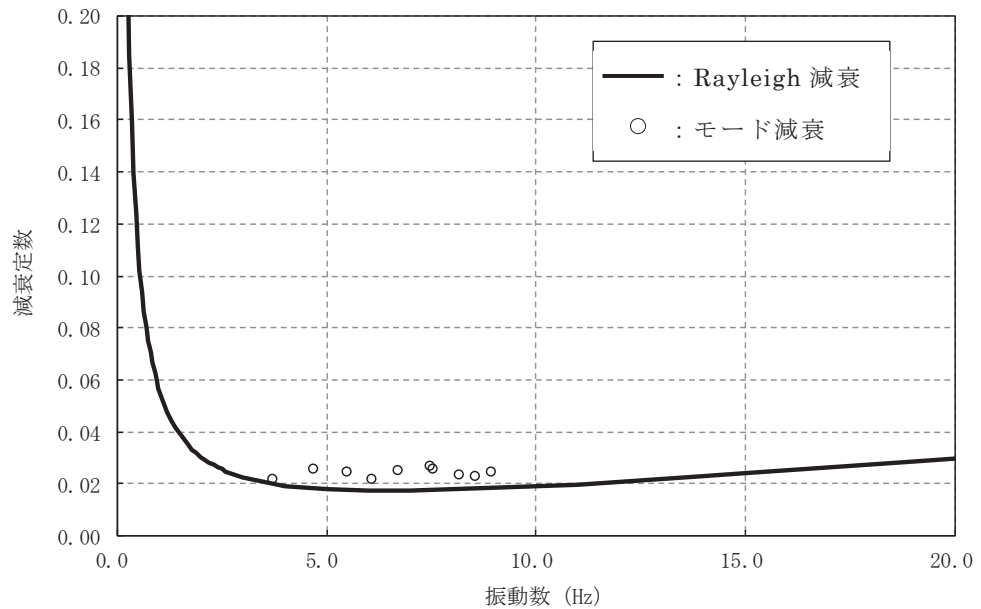
図 3-4(1) 設定した Rayleigh 減衰 (断面⑦)
