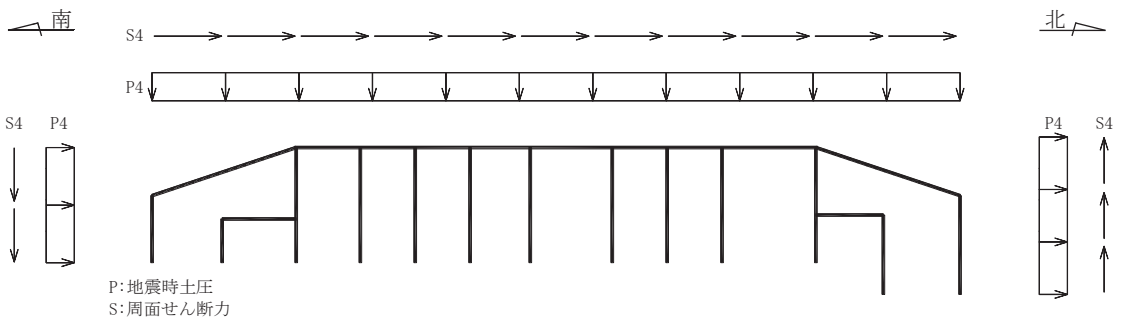
図 4-16(4) 土圧及び周面せん断力の载荷概念図 (断面④)
