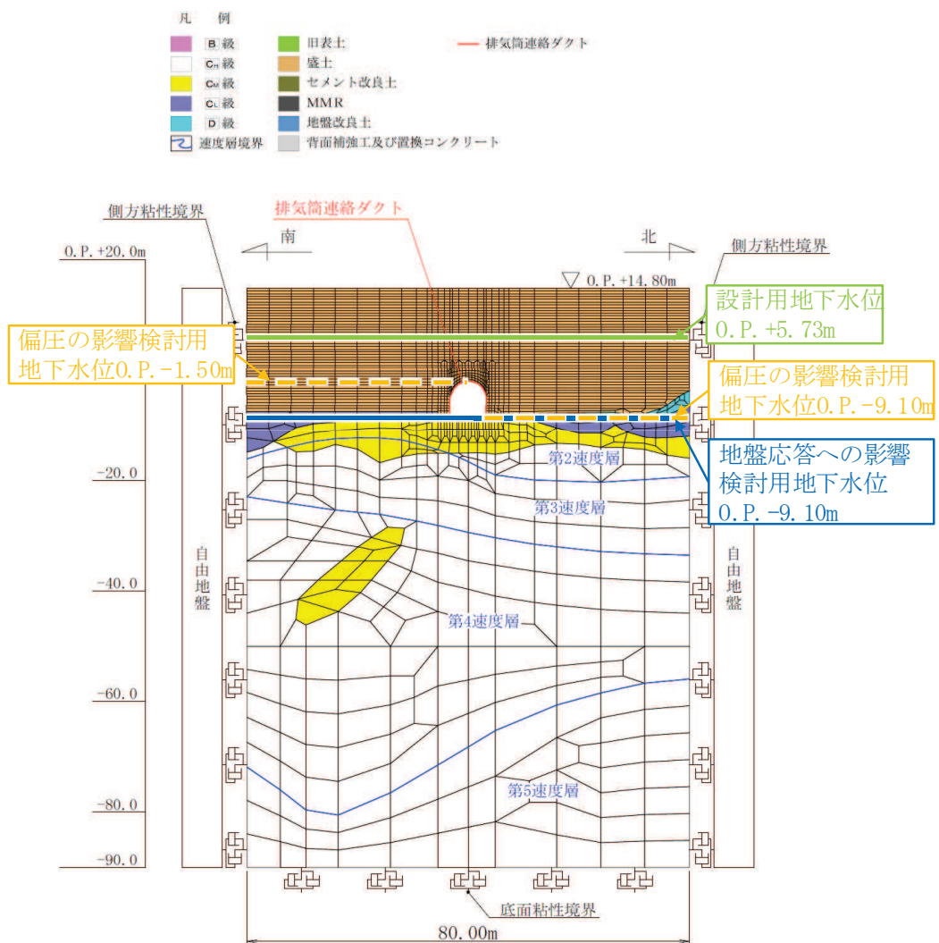
図 2-3 地震応答解析モデル図
