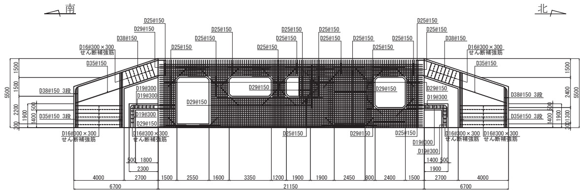
図 2-11 原子炉機器冷却海水配管ダクト（鉛直部）概略配筋図（断面①）
