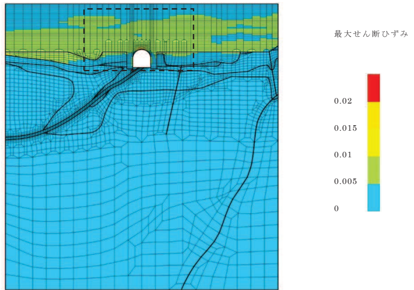
(a) 全体図
