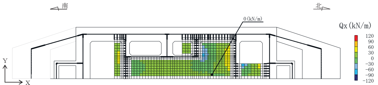
図6-17 せん断破壊に対する照査における照査値最大時の断面力分布図
