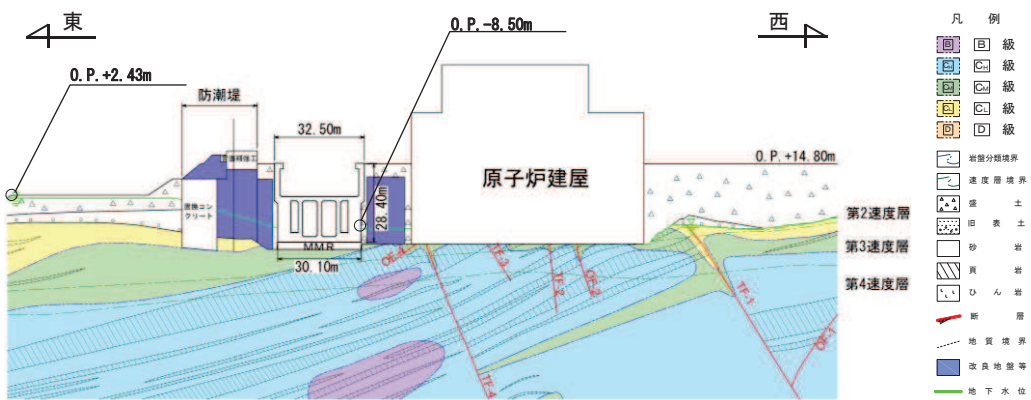
図 2-17 原子炉機器冷却海水配管ダクト(鉛直部) 地震時荷重算出用地質断面図(B-B断面:東西)
