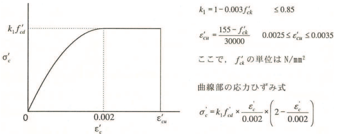
図 4-8 コンクリートの応力-ひずみ関係 (コンクリート標準示方書より引用)
