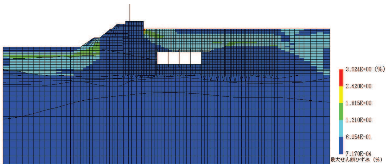
(a) 全体図
