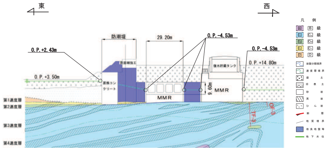
図 2-7 取水路（漸拡部）の設計用地下水位
