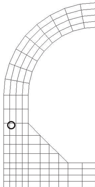
図 5-20 せん断補強筋の初期降伏箇所 (側壁, 解析ケース③, S_s - N1 (++) 168STEP)
