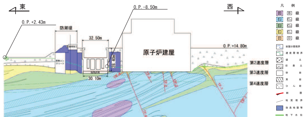
図 2-20 設計用地下水位 (B-B 断面)
