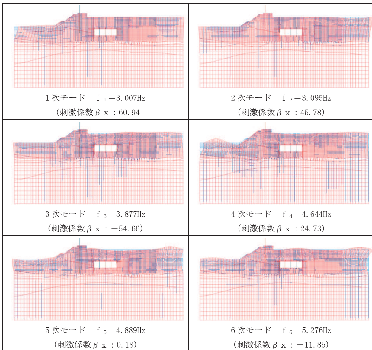
図 3-16 固有値解析結果 (モード図) (1/2)
