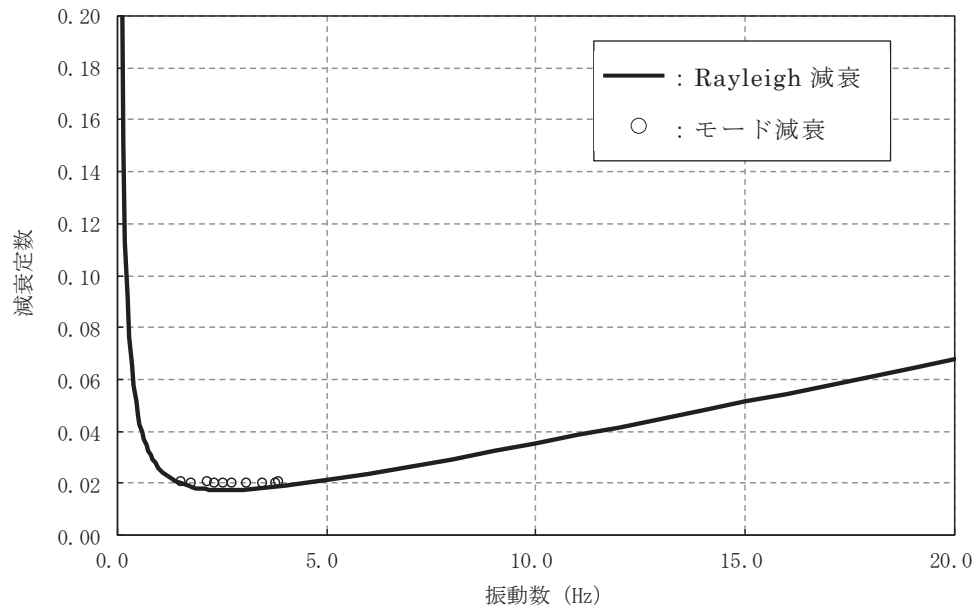
図 3-4(1) 設定した Rayleigh 減衰 (断面②)
