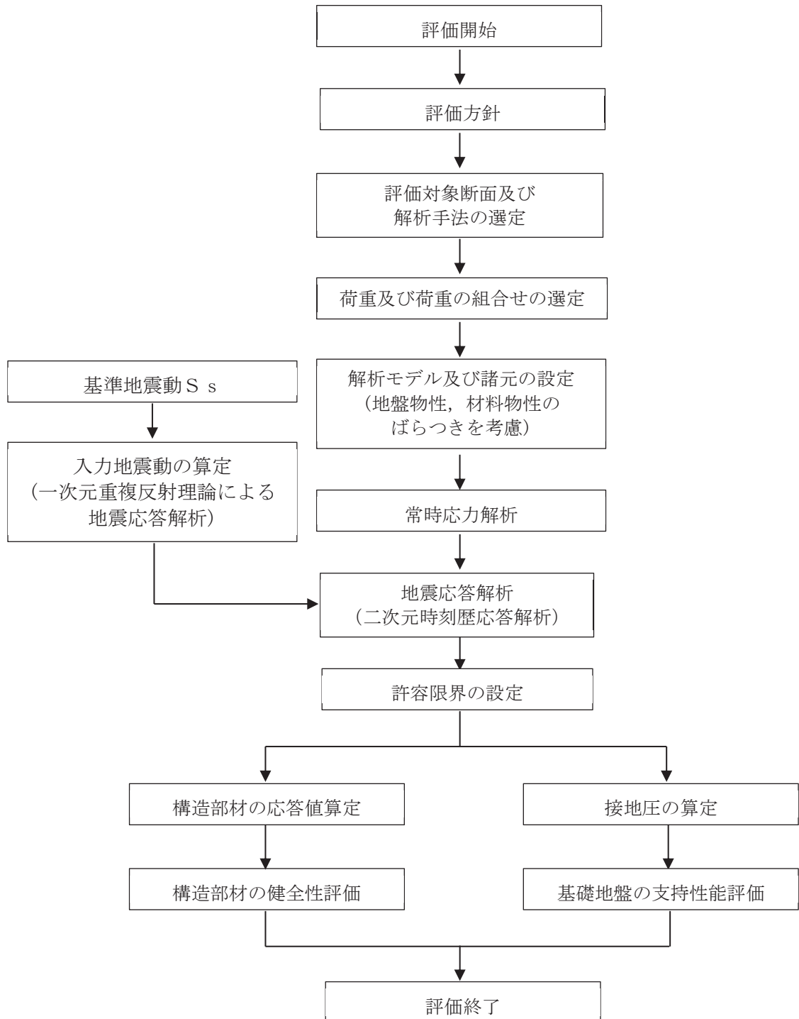
図 2-8 取水路（漸拡部）の耐震評価フロー
