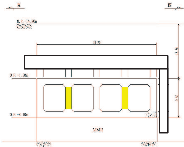
図 4-17 Ccb工法を用いる部材
