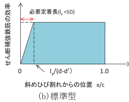
図 4-32 セラミックキャップバー (CCb) の有効率算定の概念図
