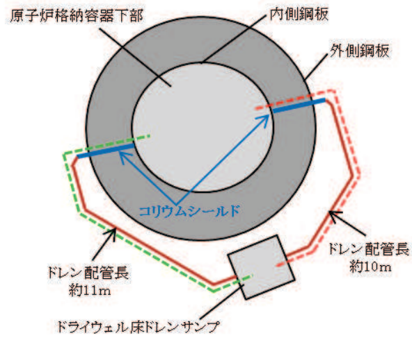
図9-5 ドライウェル床ドレンサンプルまでの流入経路
