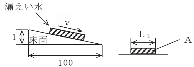
図9-3 床面概略図
