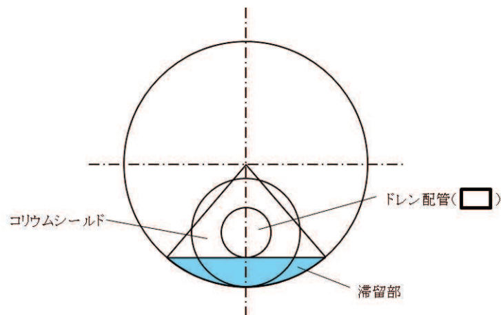
図9-4 ドレン配管受口滞留概念図
