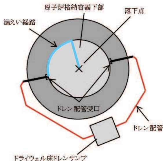
図9-2 原子炉格納容器下部床面からドレン配管受口までの漏えい経路
