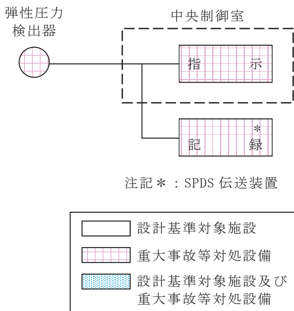
図 3.1.2-15 復水移送ポンプ出口圧力の概略構成図
