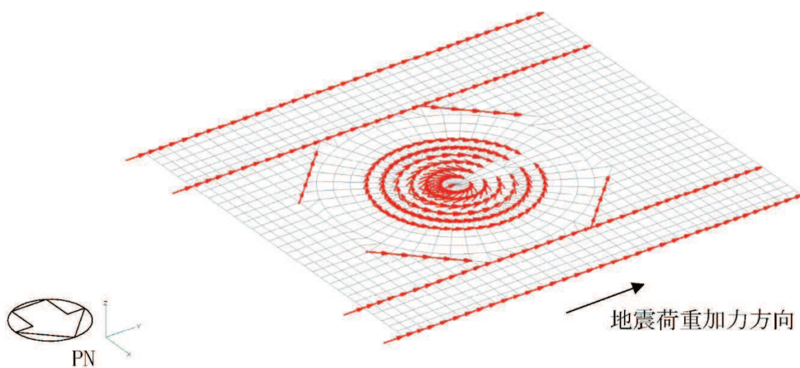
(b) 水平力 (EW 方向) 基礎版モデル部分
