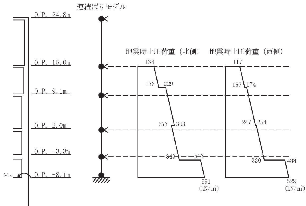
(e) 地震時土圧荷重 ( R_A 通り, R11 通りの R_A \sim R_C 間)
