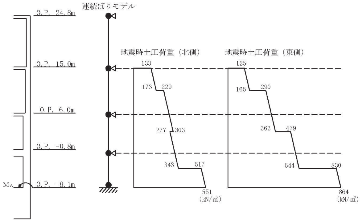
(d) 地震時土圧荷重 ( R_K 通り, R11 通りの R_C \sim R_K 間)
