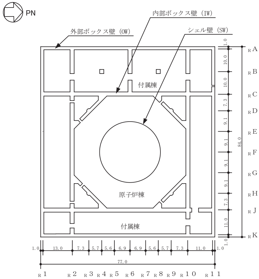
図 1-1 原子炉建屋基礎版の概略平面図 (0.P. -8.1 m)
