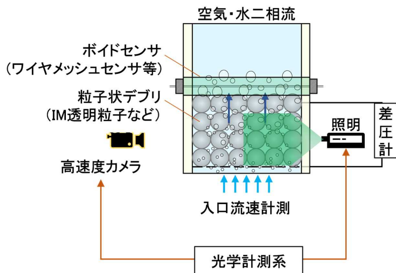
図3 個別効果試験(粒子状デブリ・構造物接触領域の流動可視化実験)の実験体系概念図
