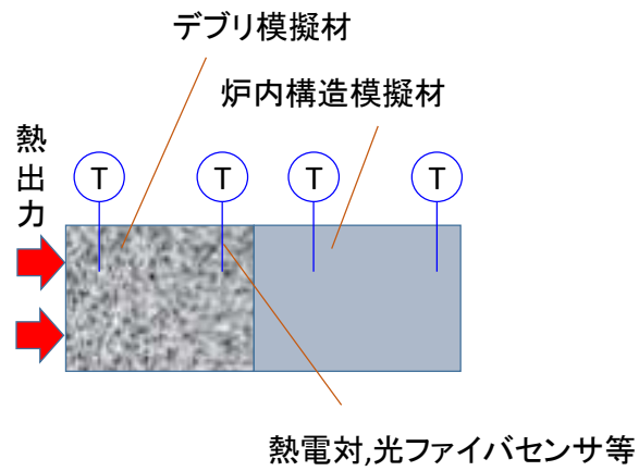
図2 個別効果試験(粒子状デブリ・構造物間の接触熱抵抗実験)の実験体系概念図
