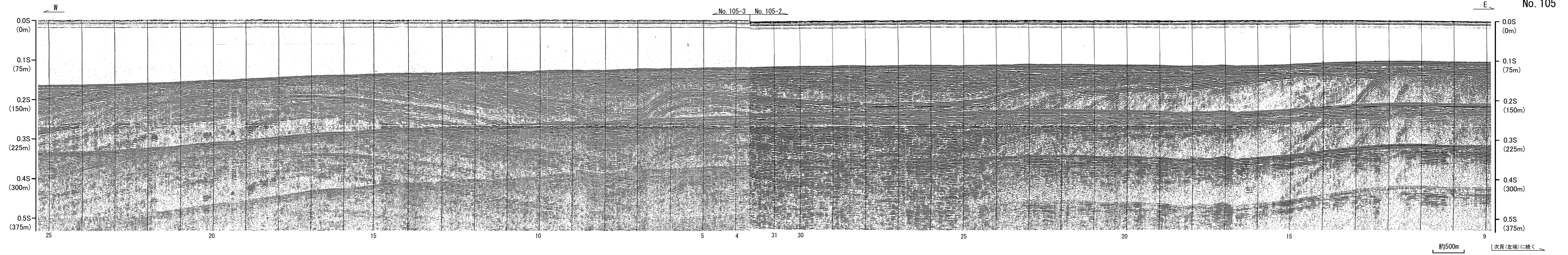
第3.2-32図(21) 敷地前面海域の音波探査記録 (No. 105・その1)
