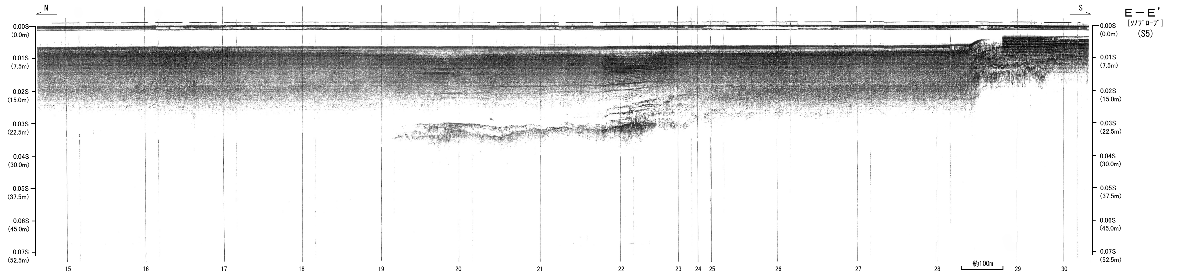
第3.2-9図(3) 宍道湖の音波探査記録(ソノプローブ・E-E')
