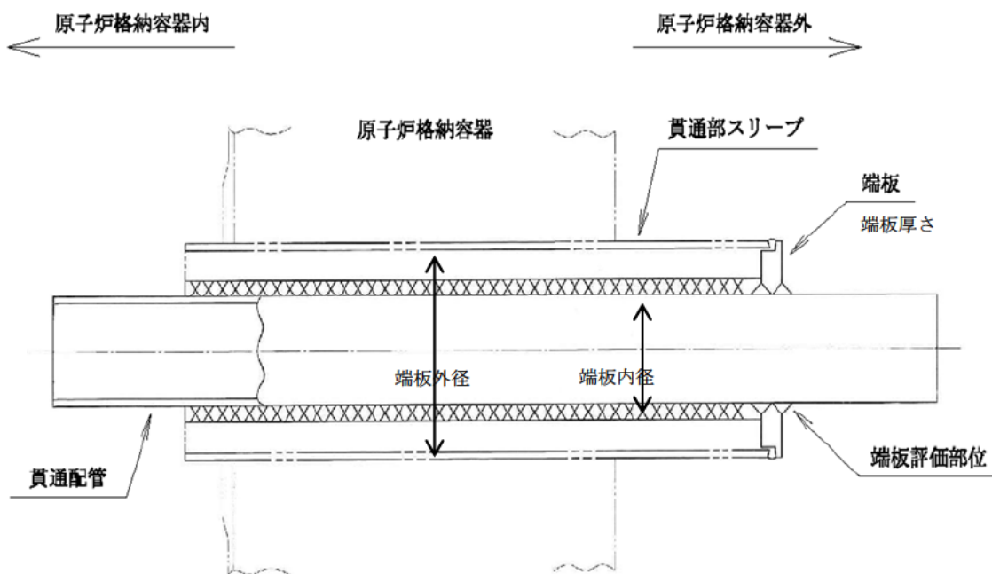
図1 余熱除去冷却器出口配管貫通部の基本寸法箇所
