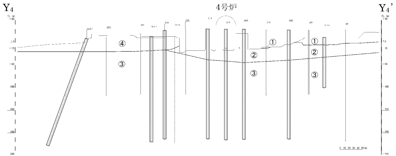
第7-2図 速度層断面図 (Y 4 -Y 4 ' 断面) (2/3)
