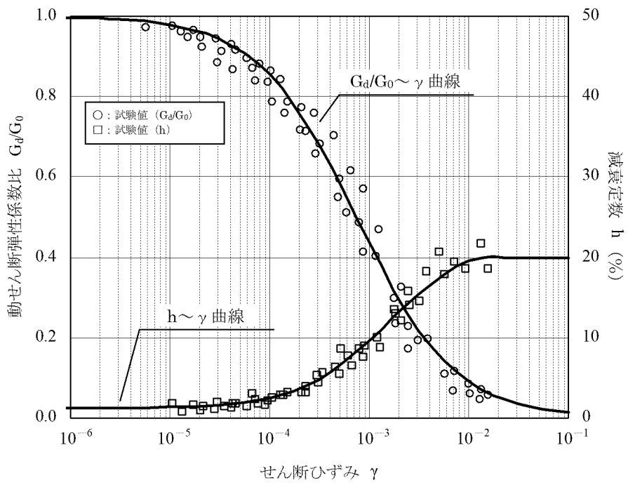
第 3-1 図 動せん断弾性係数及び減衰定数のひずみ依存性 (埋戻土 (碎石)) (5/5)
