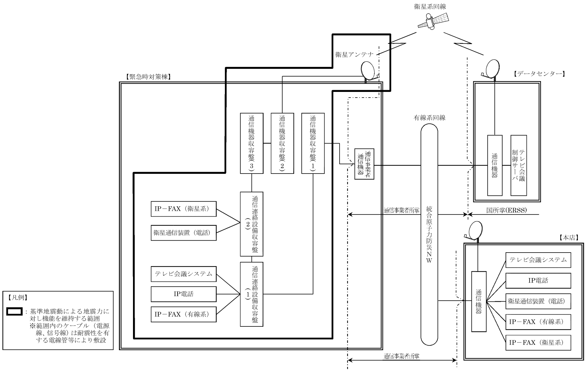
第5図 統合原子力防災ネットワークに接続する通信連絡設備の概略構成図
