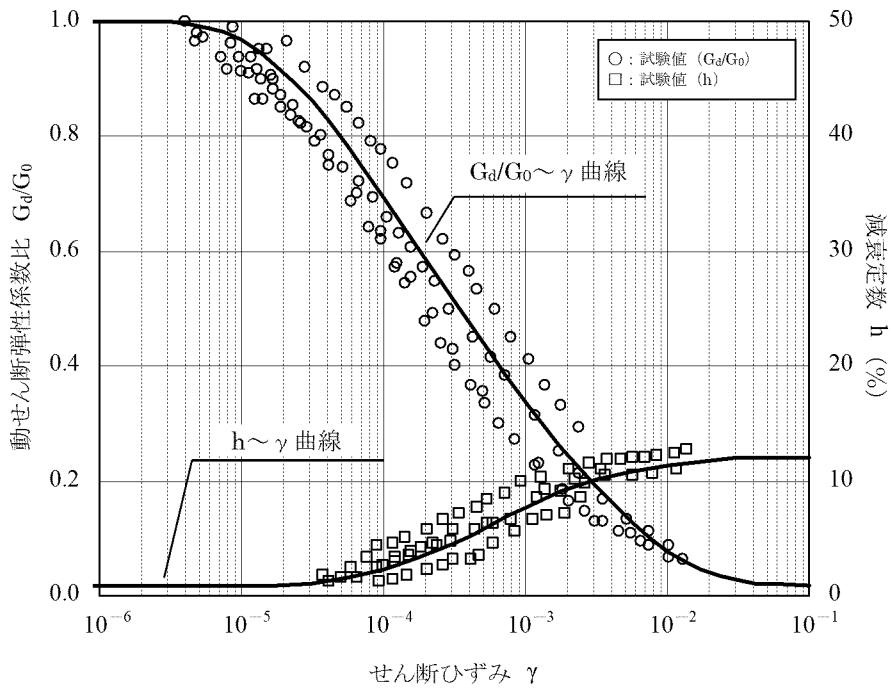
第 3-1 図 動せん断弾性係数及び減衰定数のひずみ依存性 (埋戻土 (ロック材)) (4/5)
