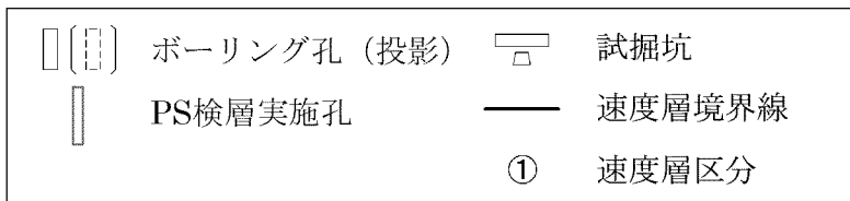
第7-2図 速度層断面図 (Y 3 -Y 3 ' 断面) (1/3)
