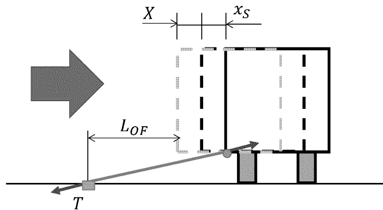
(c) 固縛対象物停止時（固縛装置作動終了）
