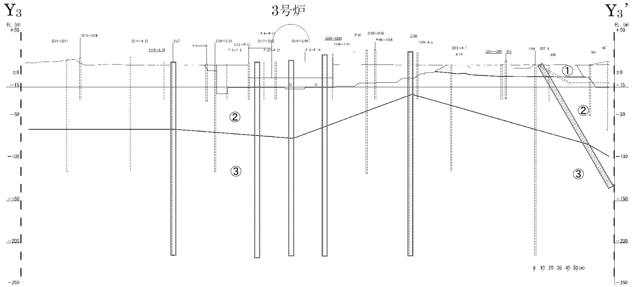
第7-2図 速度層断面図 (Y 3 -Y 3 ' 断面) (1/3)
