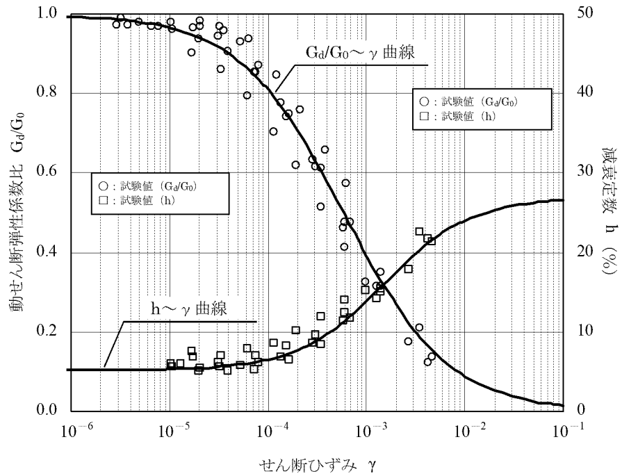
第 3-1 図 動せん断弾性係数及び減衰定数のひずみ依存性 (断層) (2/5)
