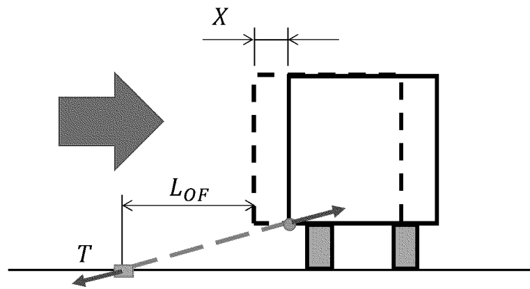
(b) 固縛装置展張時（固縛装置作動開始）
