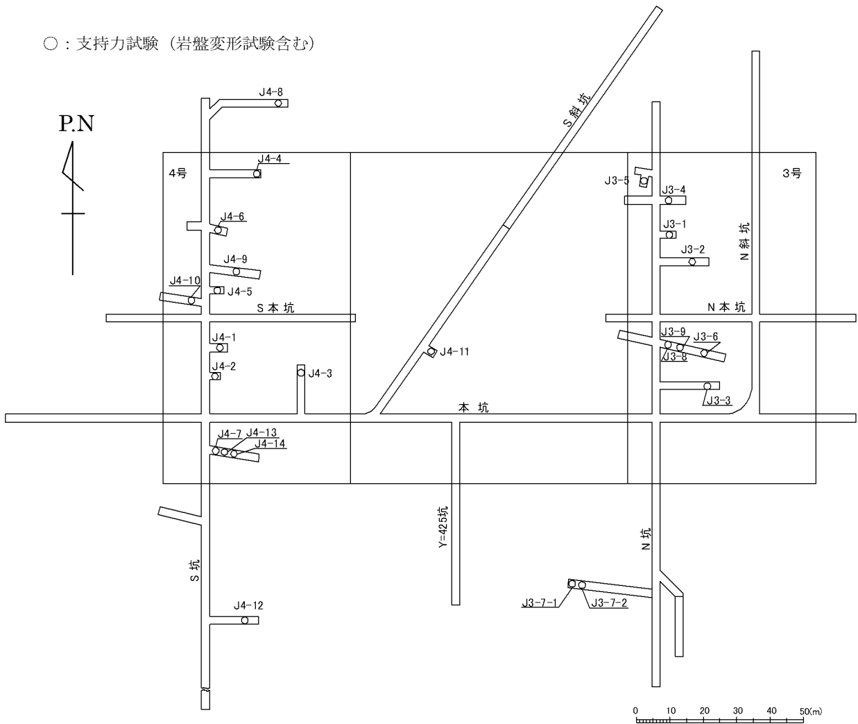
第 4-1 図 支持力試験実施位置
