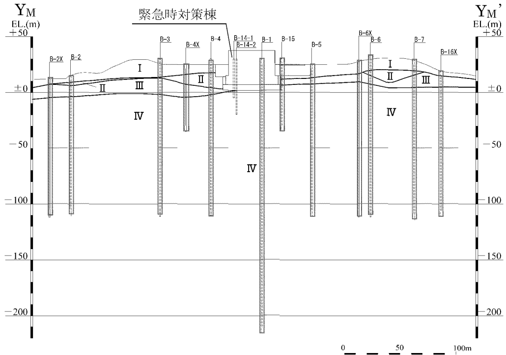
第 7-3 図 速度層断面図 ( Y_M - Y_M' 断面) (1/2)
