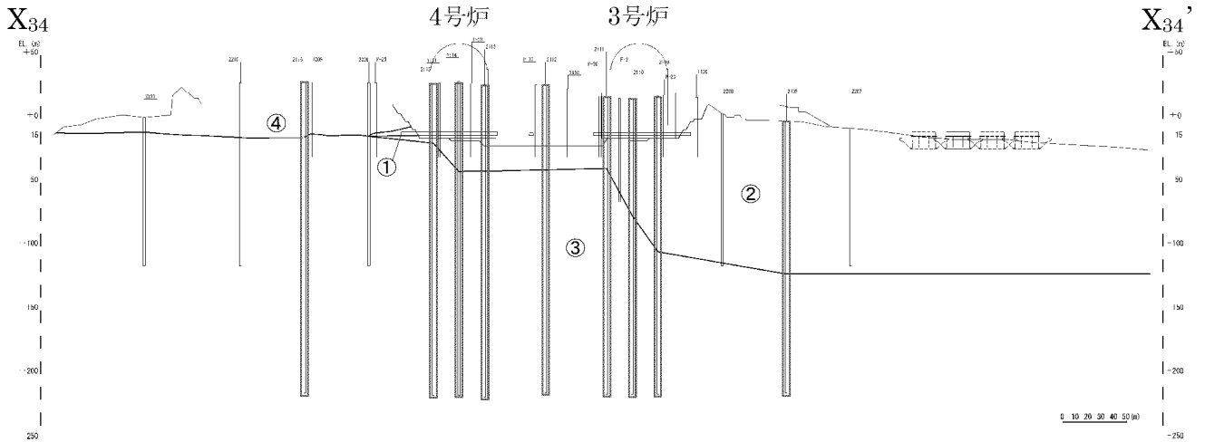
第7-2図 速度層断面図 (X 34 -X 34 ' 断面) (3/3)
