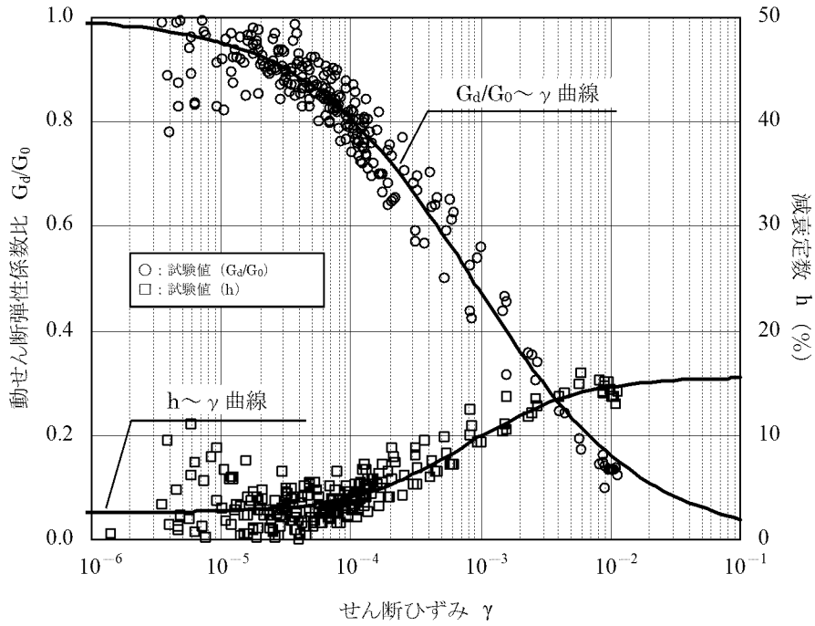
第 3-1 図 動せん断弾性係数及び減衰定数のひずみ依存性 (埋戻土 (まさ土)) (3/5)
