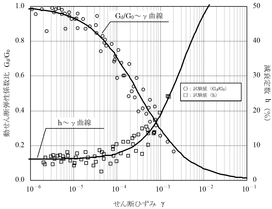
第 3-1 図 動せん断弾性係数及び減衰定数のひずみ依存性 (シーム) (1/5)
