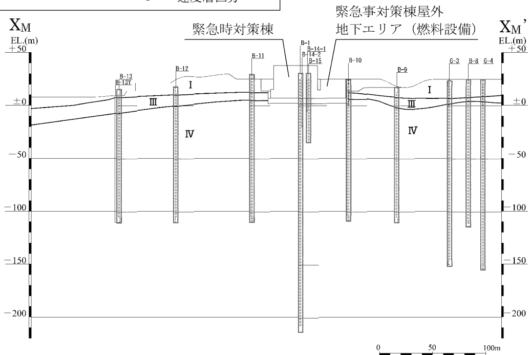
第 7-3 図 速度層断面図 ( X_M - X_M' 断面) (2/2)
