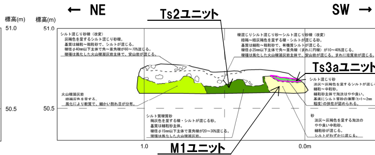
南側壁面
