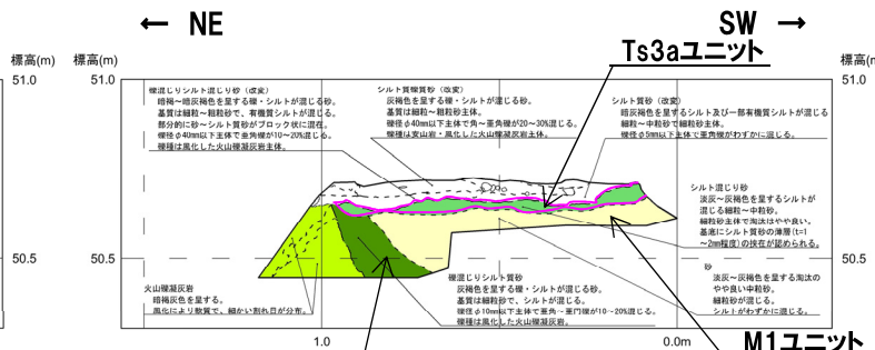
南側壁面
