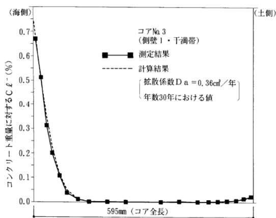
図-10 塩分浸透計算結果
