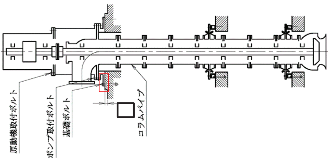
構造概要図
