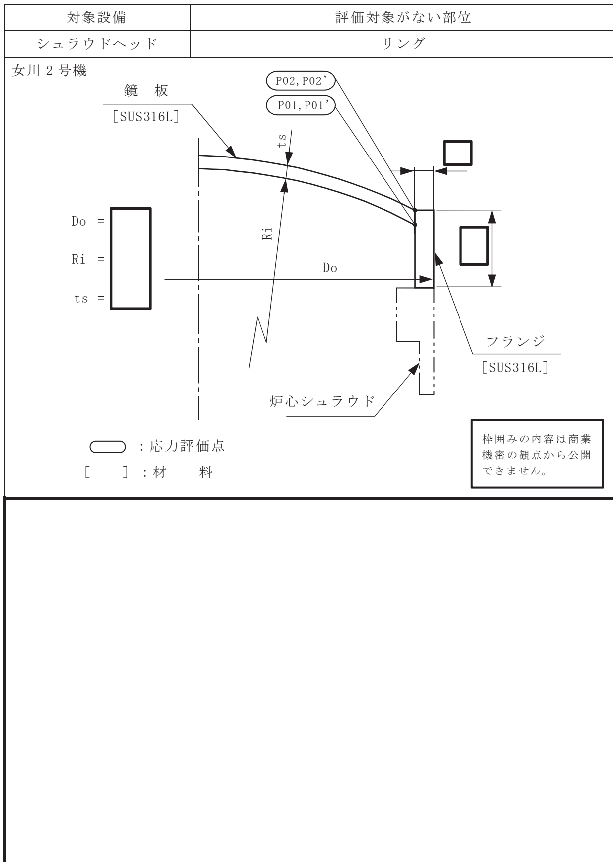
図 2 シュラウドヘッド概要図
