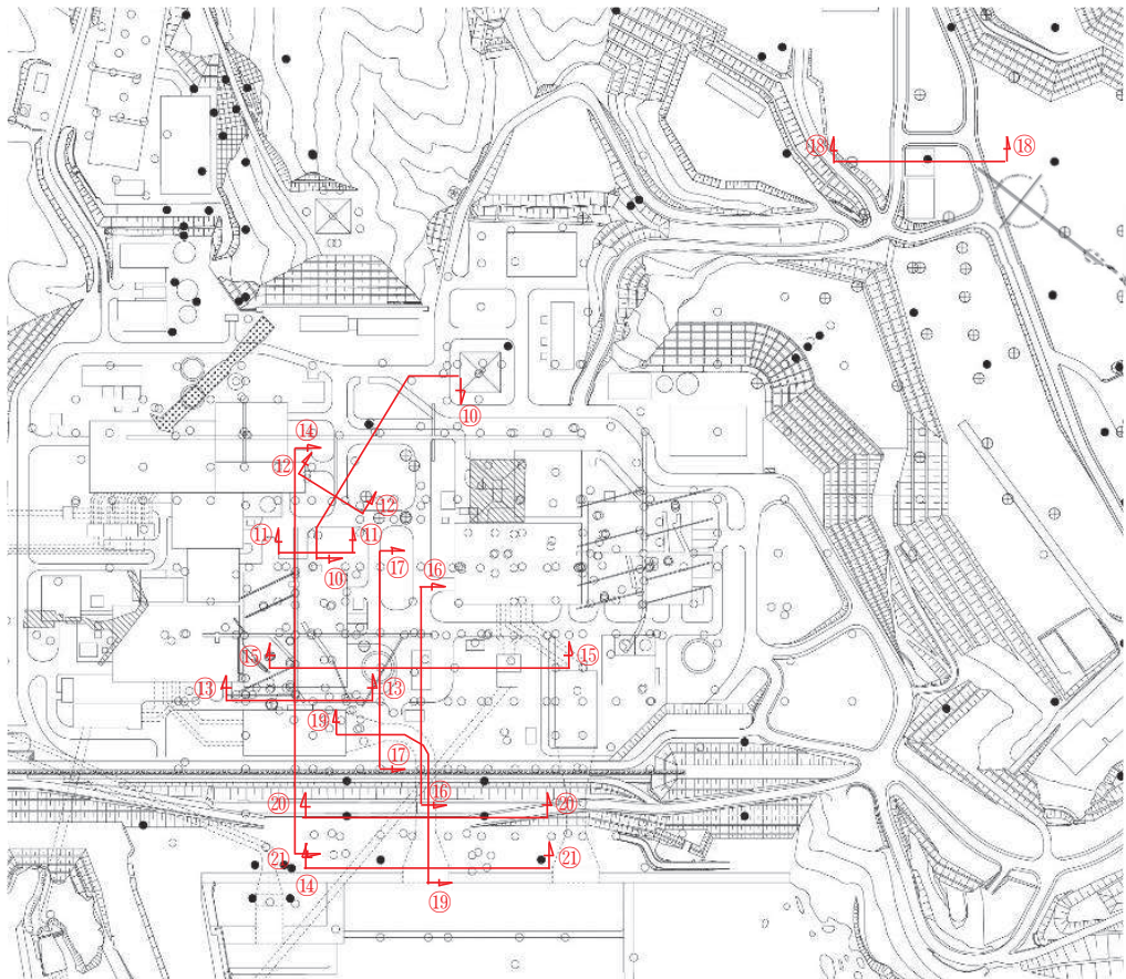
图 3.1-3(2) 地質断面图位置 (⑩—⑩断面~㉑—㉑断面)
