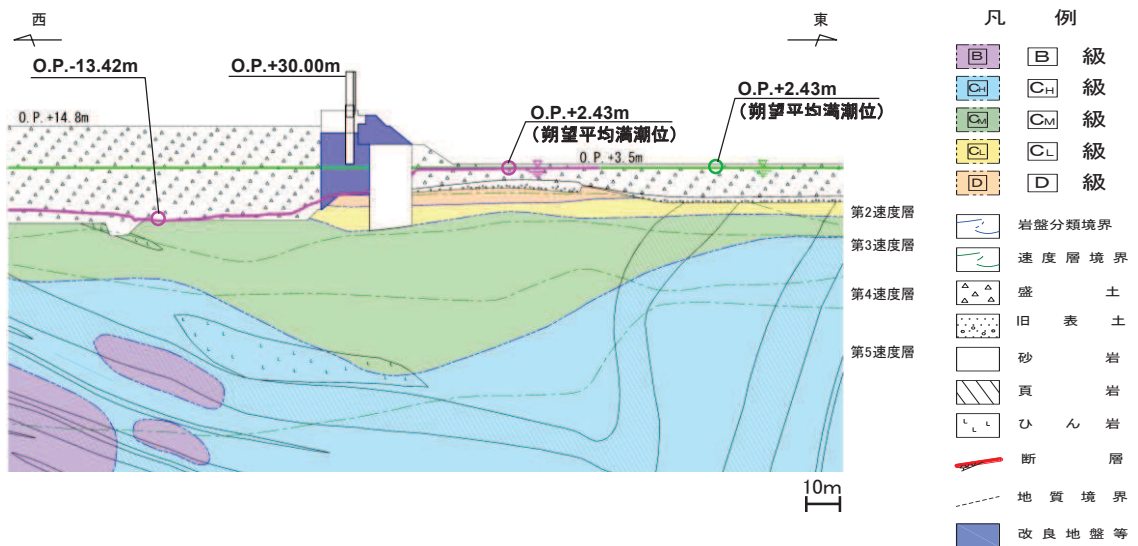
図 3.3-48(2) 防潮堤(鋼管式鉛直壁)の設計用地下水位(岩盤部②)
