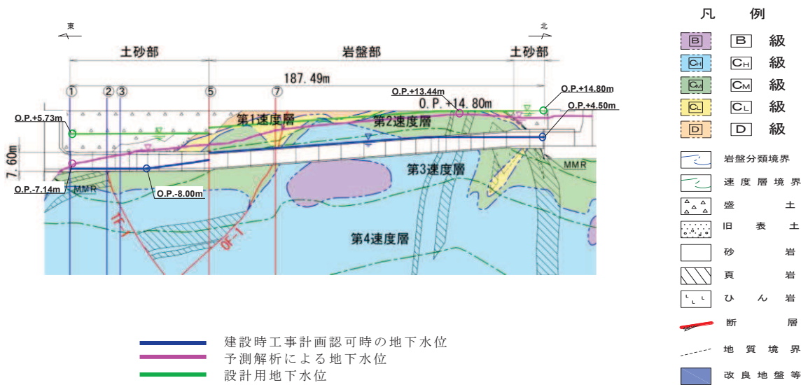
図 3.3-40(1) 排気筒連絡ダクトの設計用地下水水位 (縦断)
