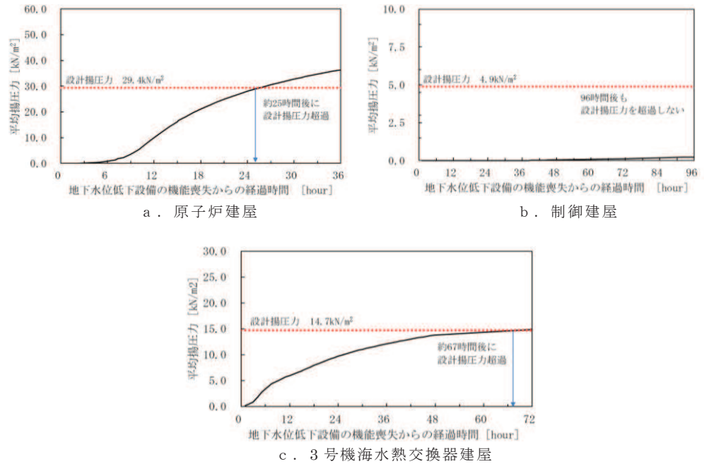
図 3.3-12 時間余裕の評価結果
