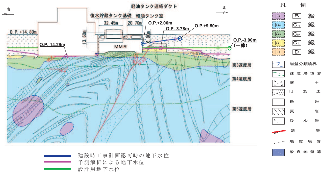
図 3.3-44 軽油タンク室の設計用地下水位（南北） （復水貯蔵タンク基礎の南北方向断面の設計用地下水位を含む）
