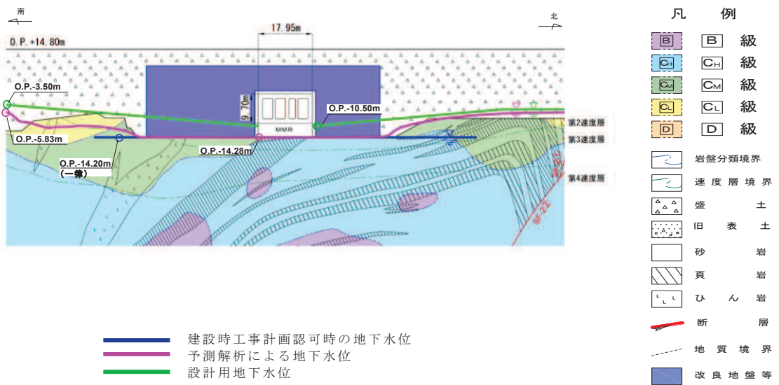
図 3.3-39 原子炉機器冷却海水配管ダクトの設計用地下水水位 (横断)
