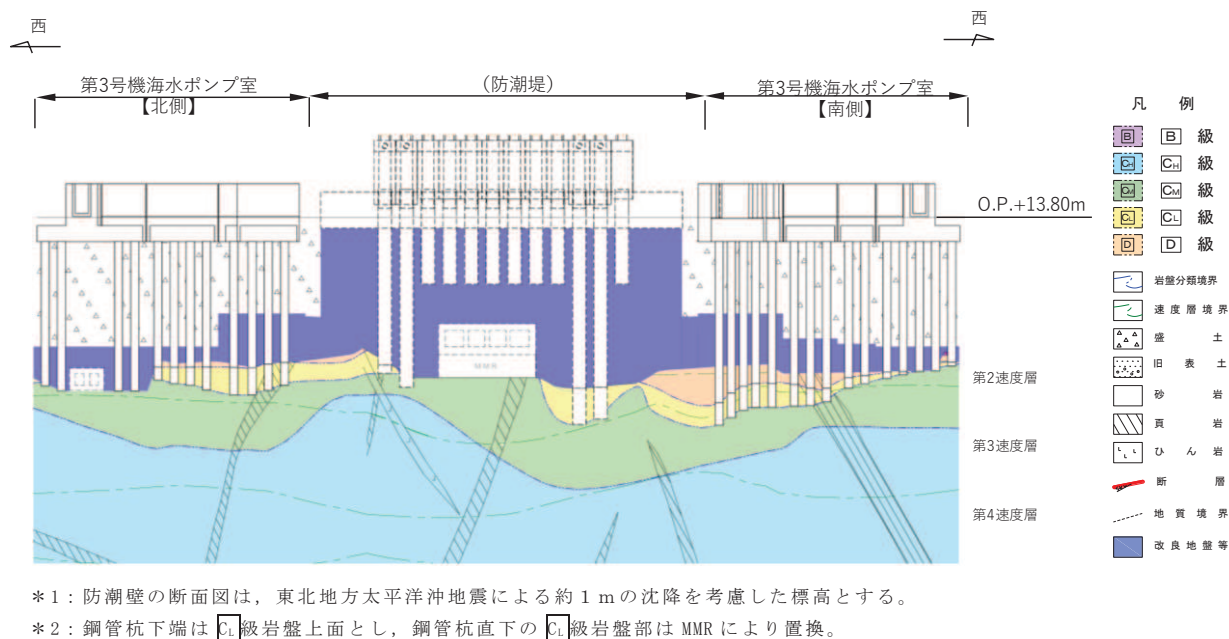
図 3.1-21(3) 防潮壁（第3号機海水ポンプ室）の地質断面図（㉕-㉕断面）
