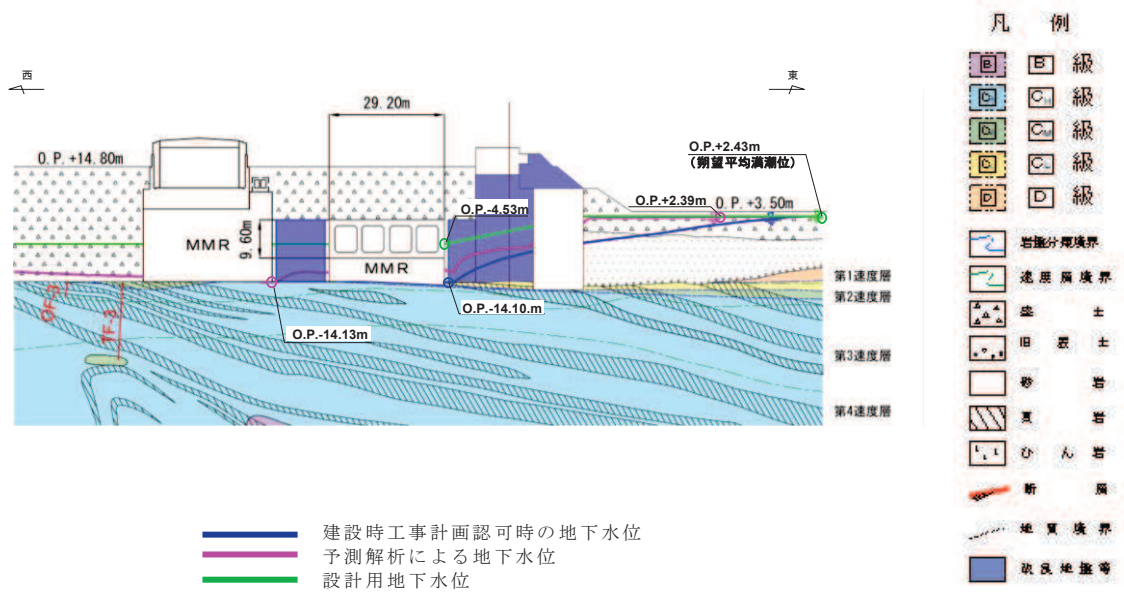
図 3.3-42(8) 取水路の設計用地下水水位（漸拡部）（東西）
