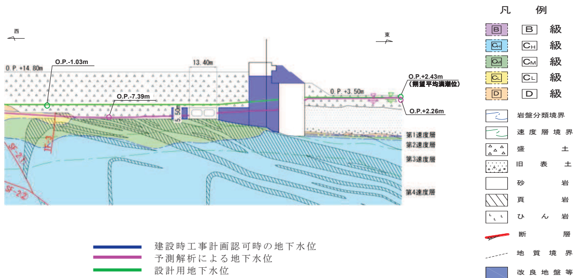
図 3.3-42(7) 取水路の設計用地下水水位（曲がり部）（東西）
