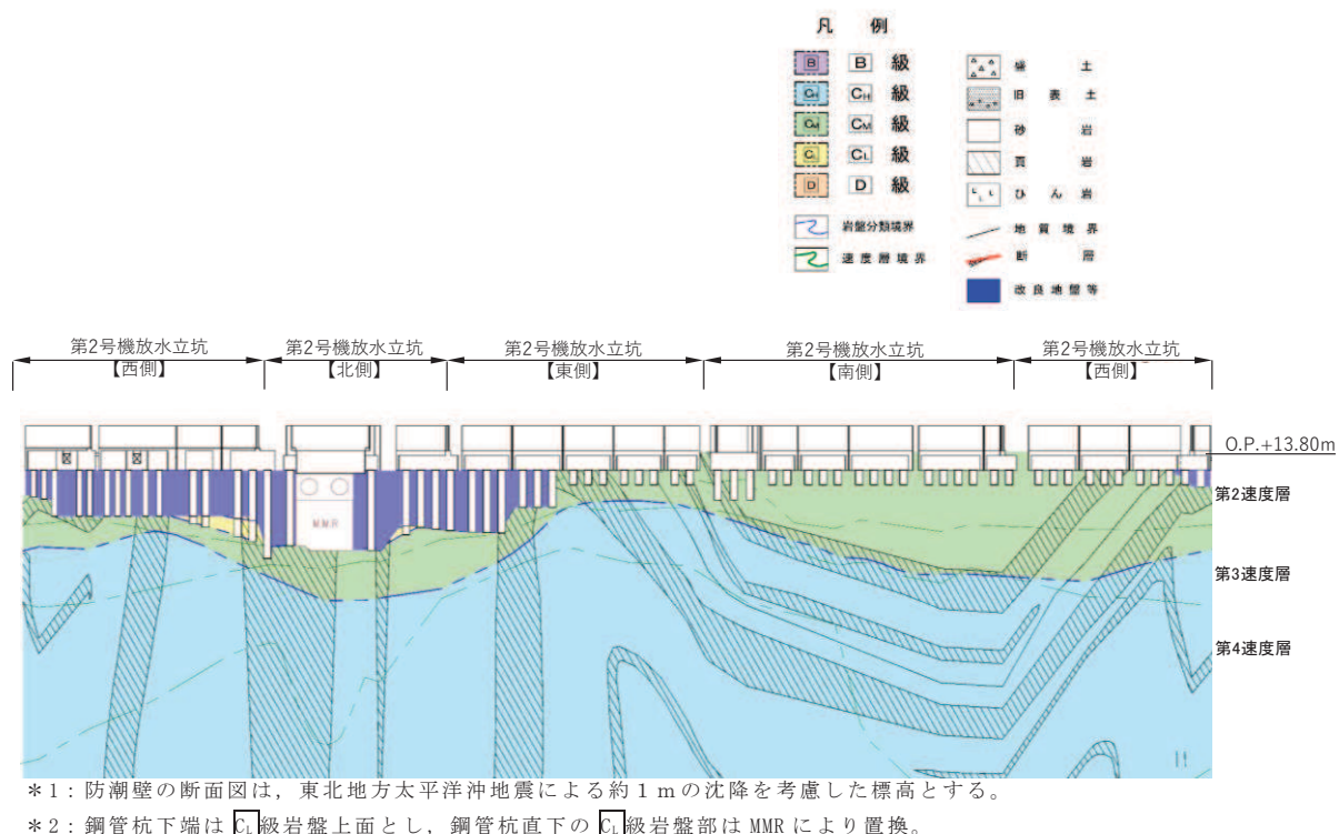
図 3.1-21(2) 防潮壁（第2号機放水立坑）の地質断面図（㉔-㉔断面）
