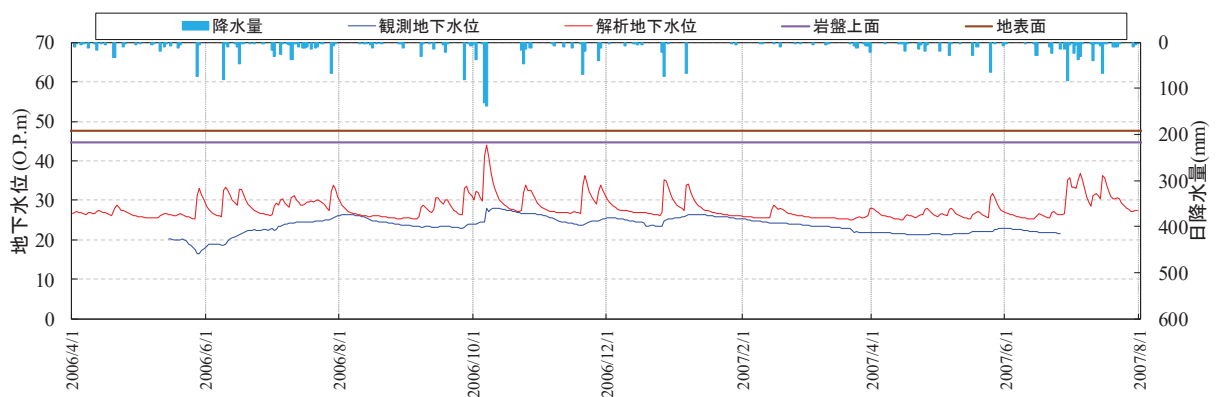
図 3.3-19 (5) 解析水位と観測水位の経時変化 (観測井⑪) (期間 1)
