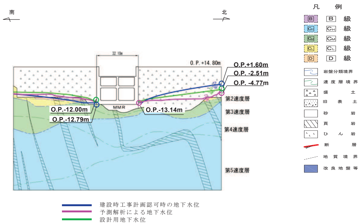
図 3.3-51(2) 第 3 号機海水ポンプ室の設計用地下水位 (横断)
