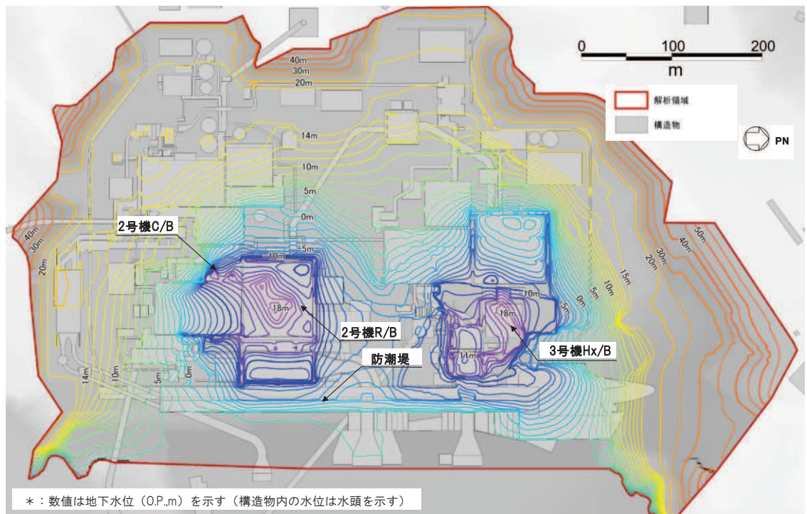
図3.3-32 設計用地下水位の設定において参照する敷地の地下水位分布 (ケース①～④の予測解析により求めた地下水位の包絡水位)
