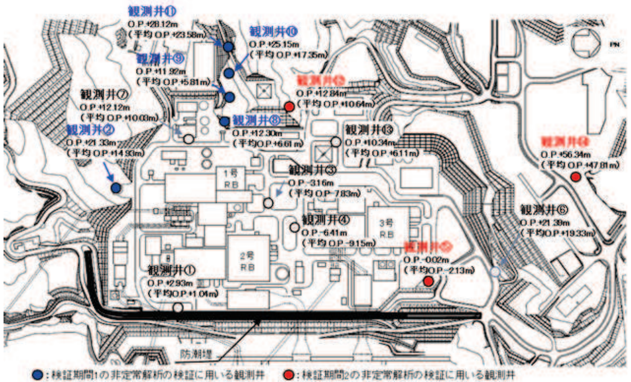
図 3.3-16 検証に用いる観測井位置
