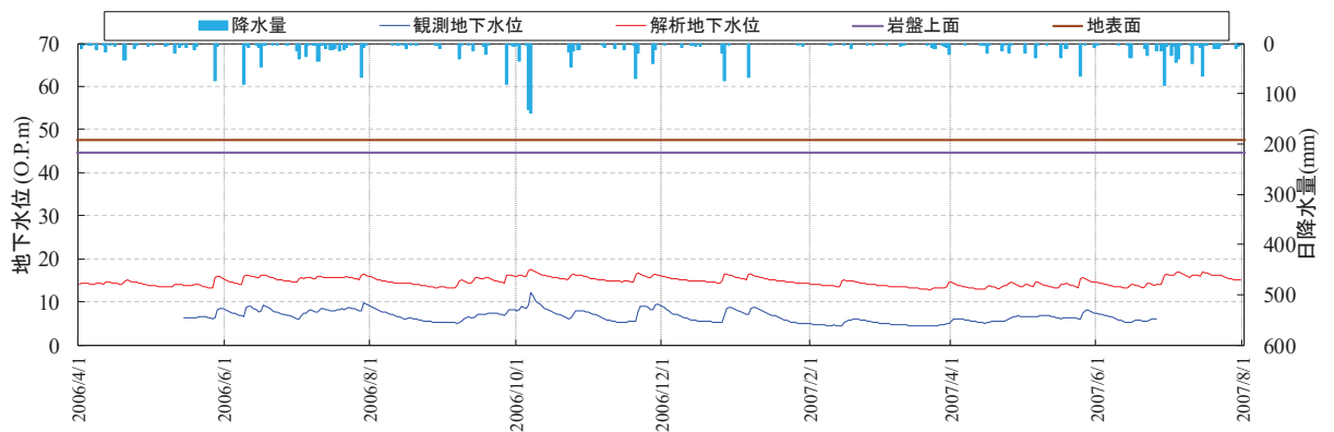
図 3.3-19 (2) 解析水位と観測水位の経時変化 (観測井⑧) (期間 1)
