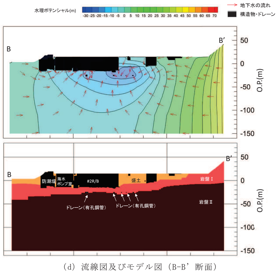
図3.3-28(2) 予測解析結果 (ケース①)
