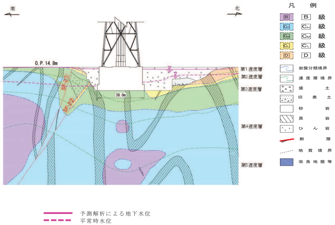
図 3.3-61 排気筒周辺における平常時水位分布(参考)
