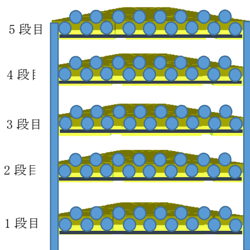
サポート試験（その2）のケーブル部詳細配置
