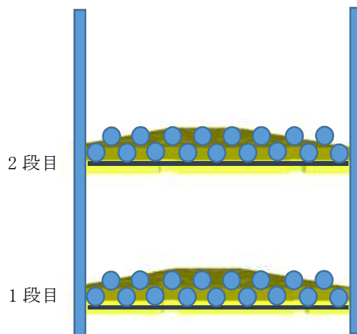
サポート試験（その3）のケーブル部詳細配置
