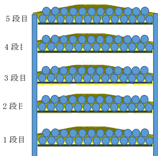
サポート試験（その1）のケーブル部詳細配置
