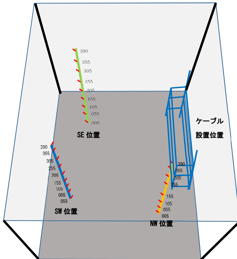
図 4. 2-3 本試験（その 1）の解析結果の過渡変化出力位置
