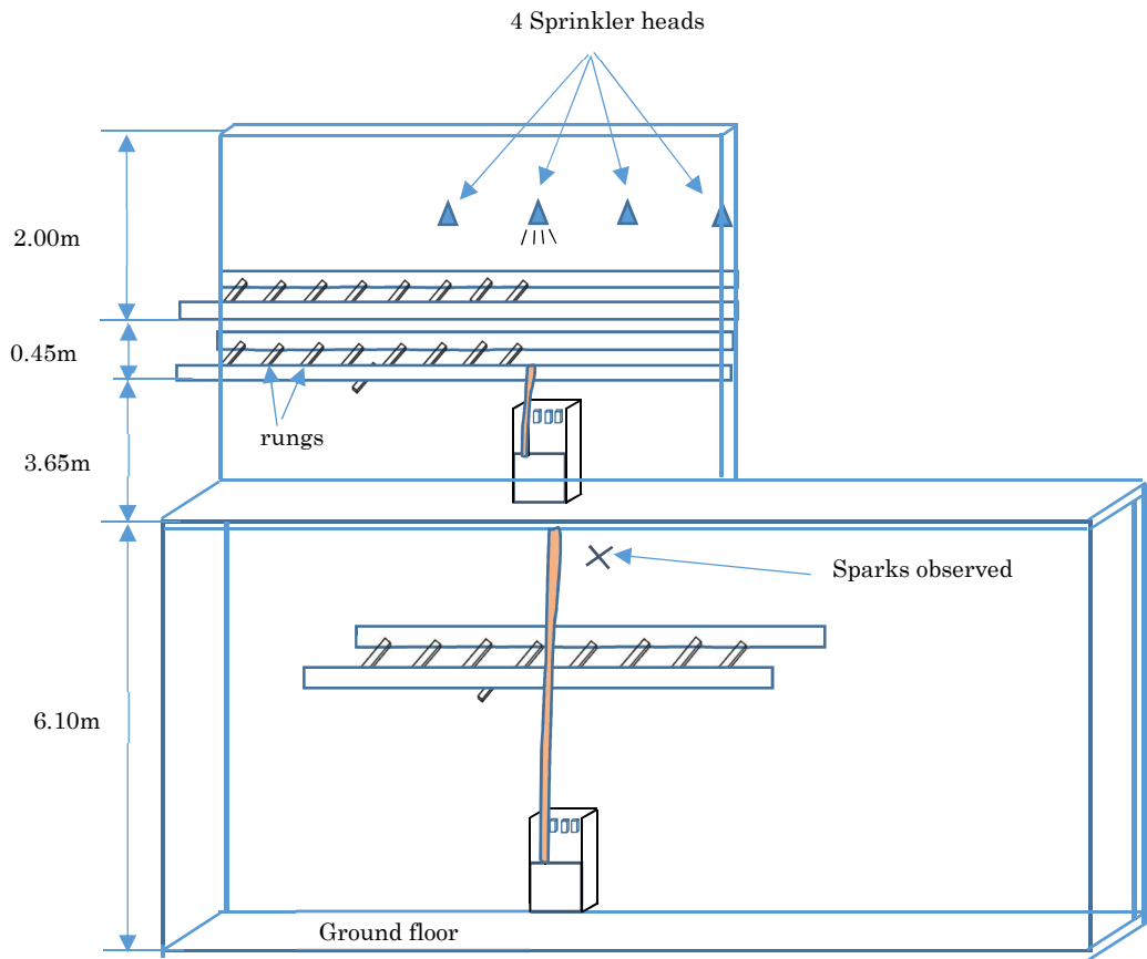
図 4. 3-2 実機火災対象の正面図
