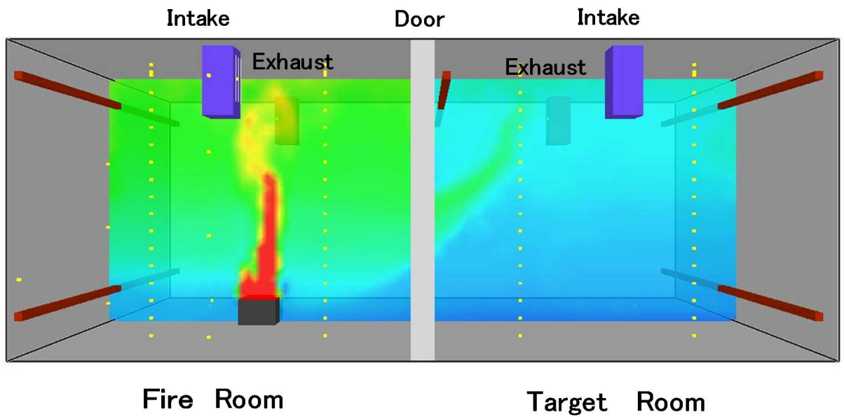
図 4. 2-2 本試験（その 1）の解析結果の温度分布出力例
