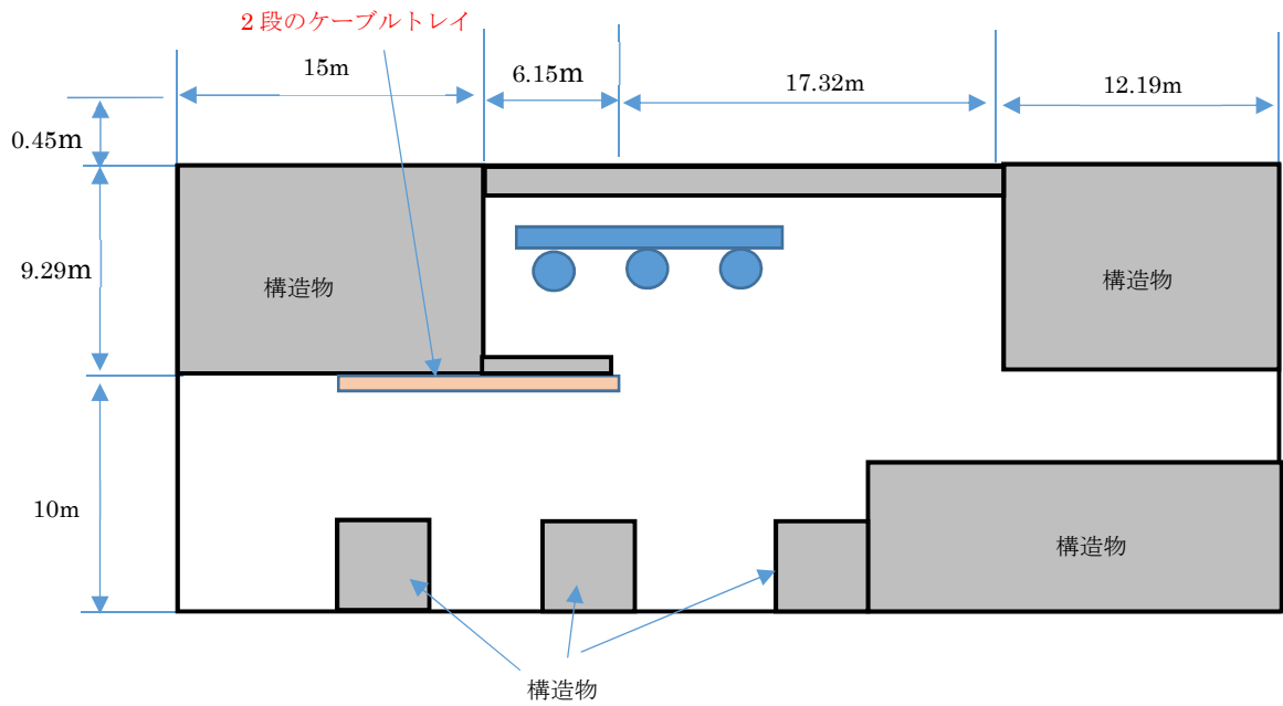
図 4. 3-1 実機火災対象の上面図
