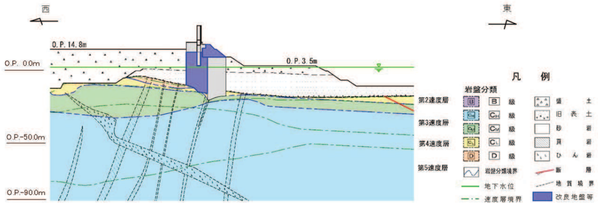
図 3.3.3-14 地質断面図
