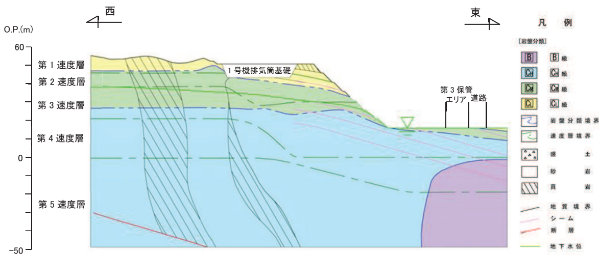
図 3.3.2-5 斜面 F の地質断面図
