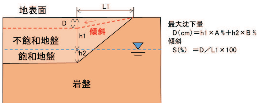
図 3.3.3-7 地山に勾配を設けて掘削した箇所の評価方法
