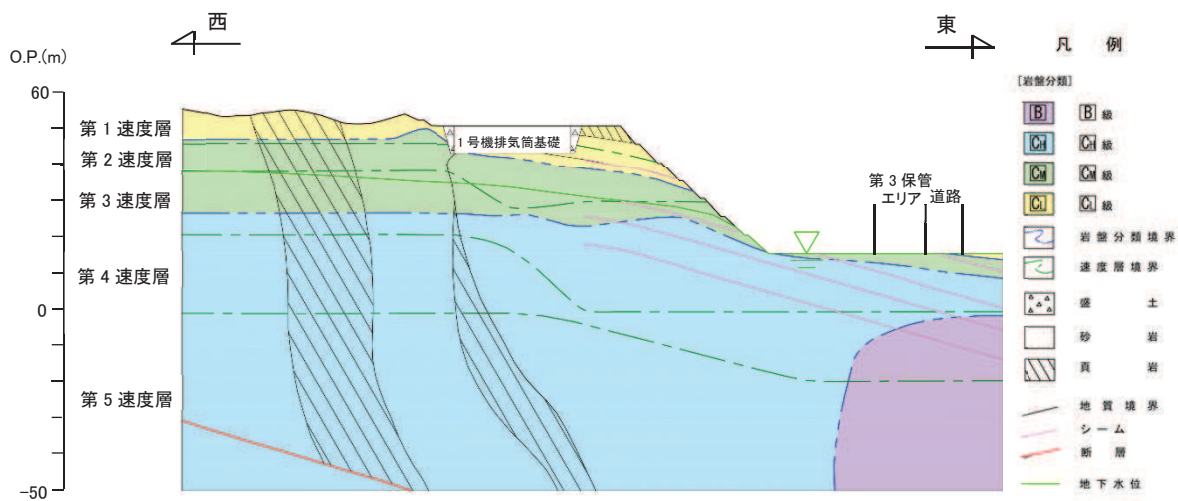
図 2.3.2-3 斜面 F の地質断面図
