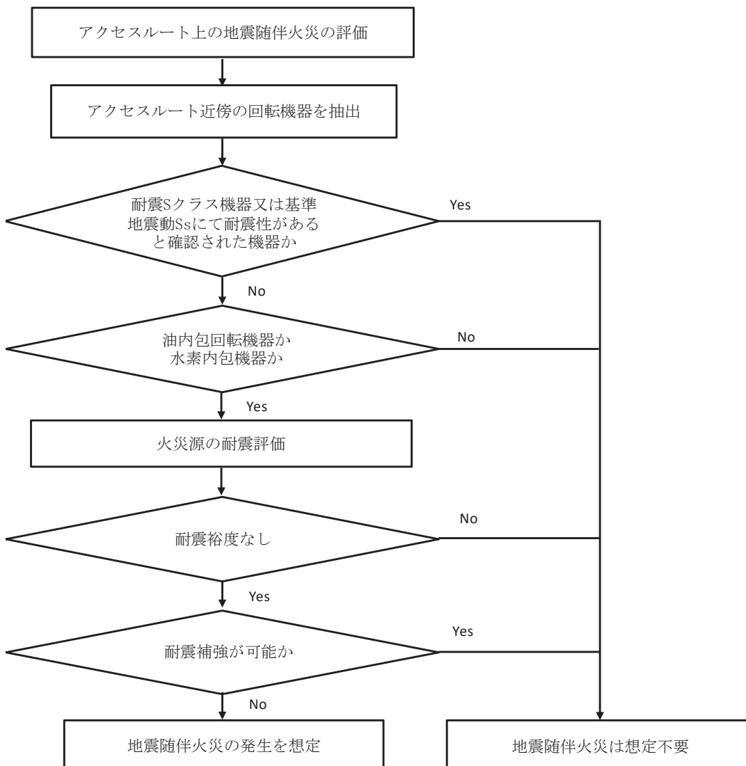
図 4.3.1-1 地震随伴火災評価対象機器抽出フロー
