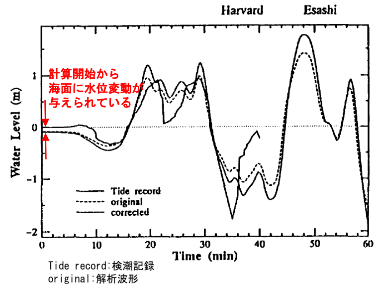
1993年北海道南西沖地震津波 江差地点の検潮記録と解析波形の比較 首藤 (1996) (31) に一部加筆
