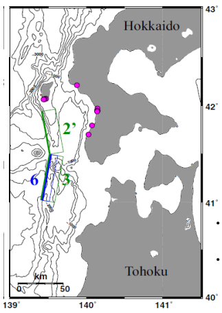
12世紀地震の断層モデル
