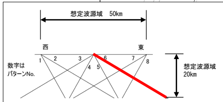
例示ケースの波源モデル
