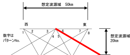
例示ケースの波源モデル
