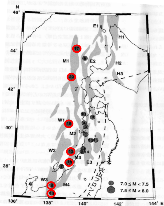
「主地震帯」で発生した地震 (○印)
