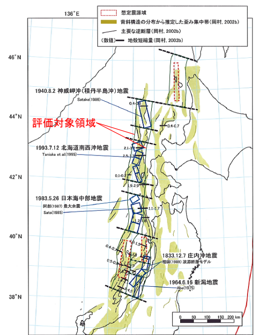
ひずみ集中帯と想定震源域の分布
