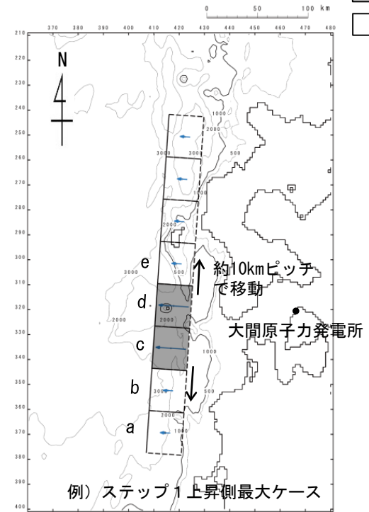
アスペリティ位置変化ケース (例)
