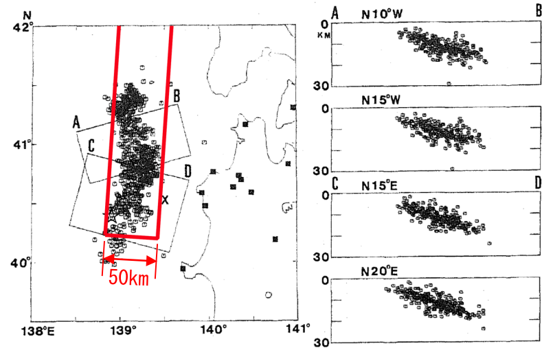
1983年日本海中部地震の余震分布
