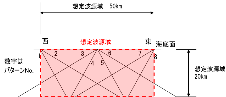
鉛直面内の断層形状
