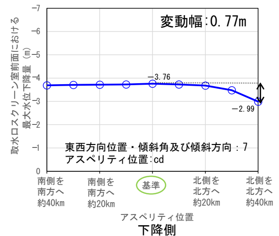
アスペリティ数と位置の影響
