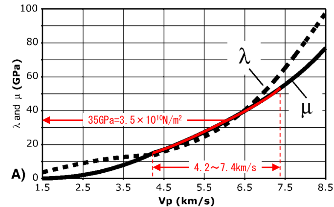
P波速度とラメ定数の経験的關係※2
