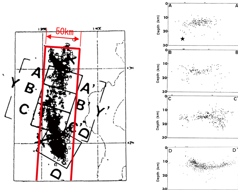
1993年北海道南西沖地震の余震分布
