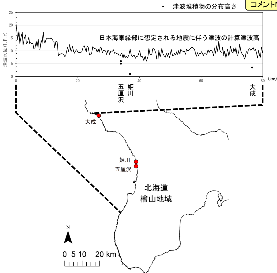
計算津波高と津波堆積物の分布高さ比較表
