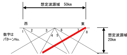
最大ケースの波源モデル
