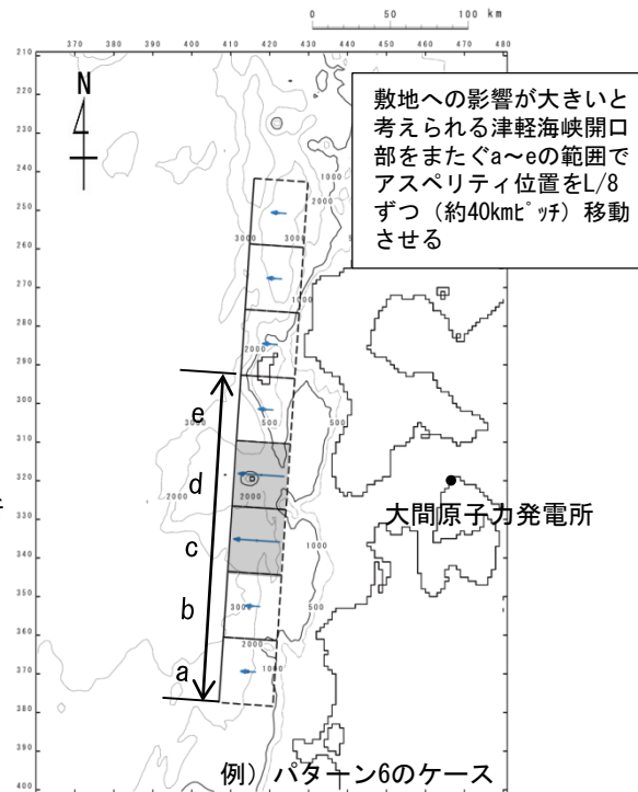
アスペリティ位置変化ケース (例)
