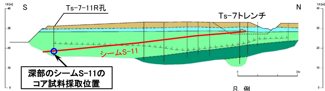
Ts-7-11R孔 試料採取位置図
