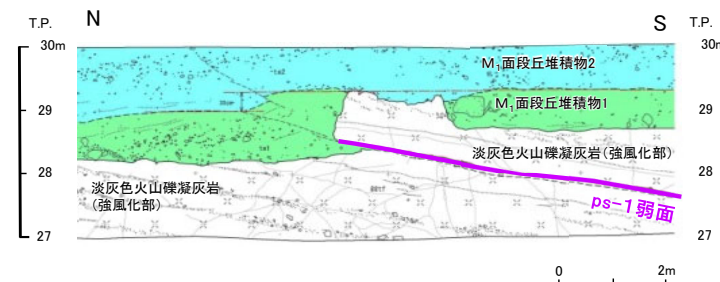
Ts-7トレンチ東側法面: 変状が認められる ps-1弱面が分布する (補足説明資料P.8-5参照)
