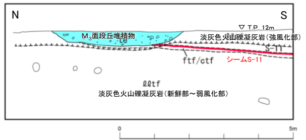
No.3法面: 変状が認められない (補足説明資料P.4-3参照)
