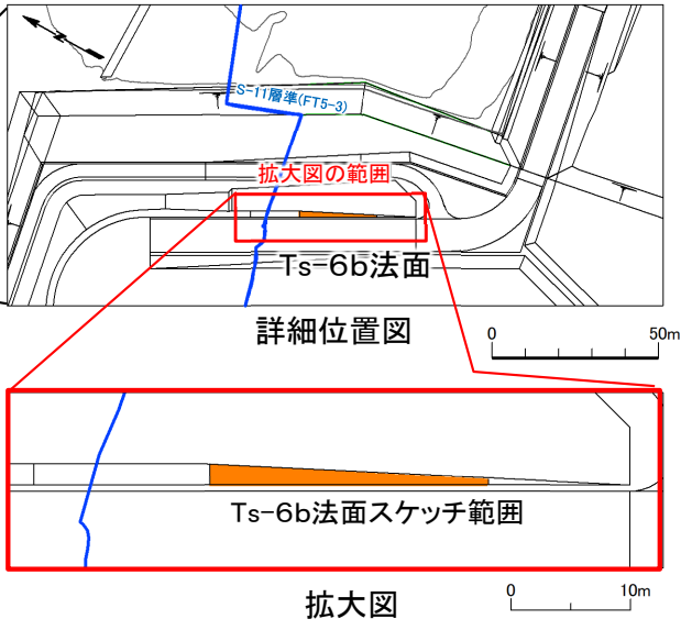
Ts-6b法面スケッチ
