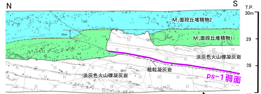
Ts-7トレンチ東側法面スケッチ
