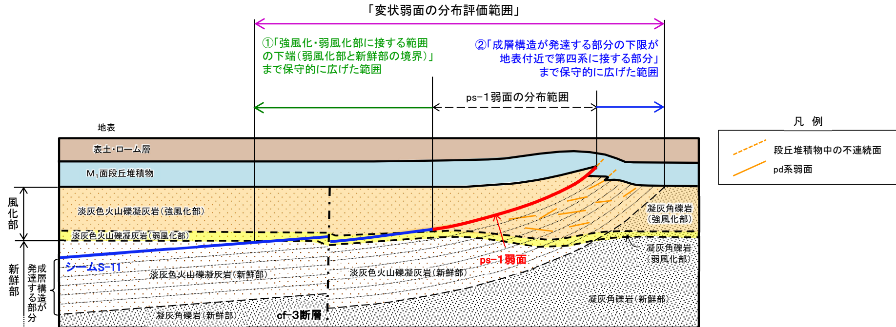
図1 変状弱面の分布評価範囲の概念断面図
