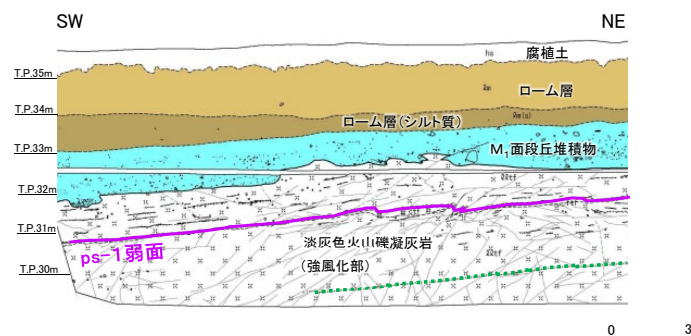
Ts-8トレンチ北側法面: 変状が認められる ps-1弱面が分布する (補足説明資料P.8-9, 8-10参照)
