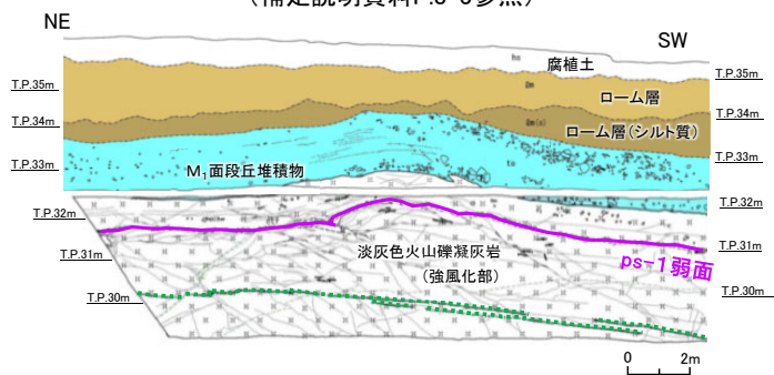
Ts-8トレンチ南側法面: 変状が認められる ps-1弱面が分布する (補足説明資料P.8-7, 8-8参照)
