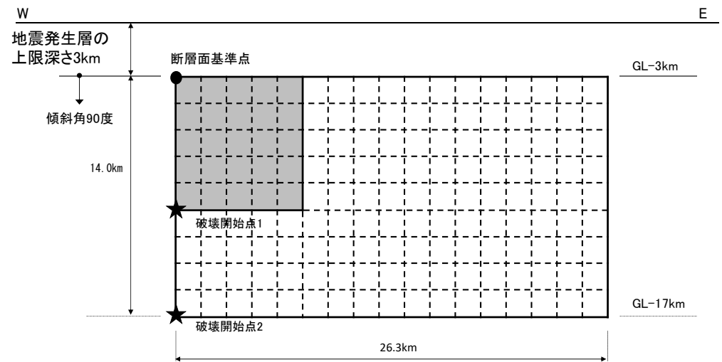
展開図
