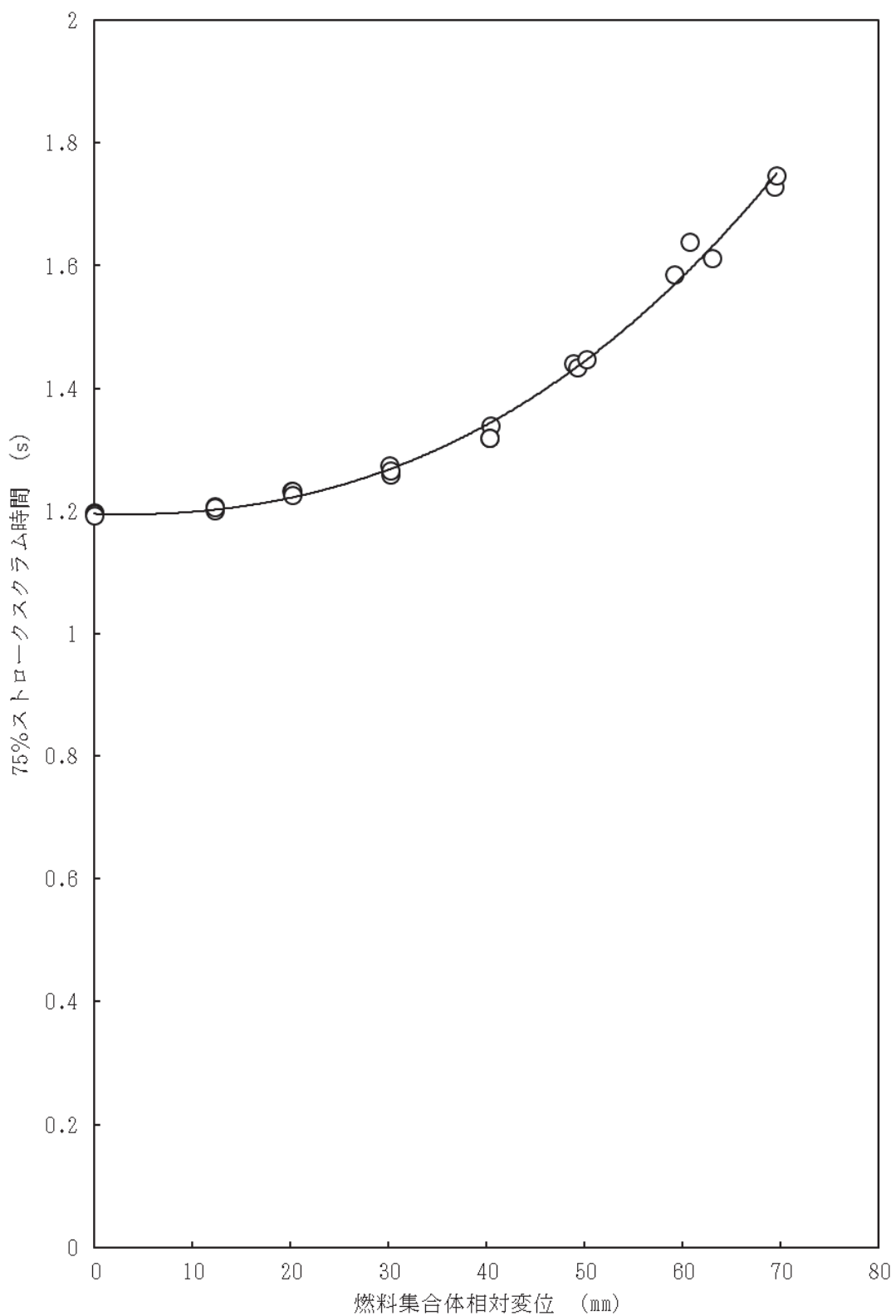
図 4-3 燃料集合体相対変位のスクラム時間に及ぼす影響
